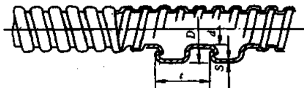
图 9.4.3 P3 型镀锌金属软管 (GB 3641—83)
