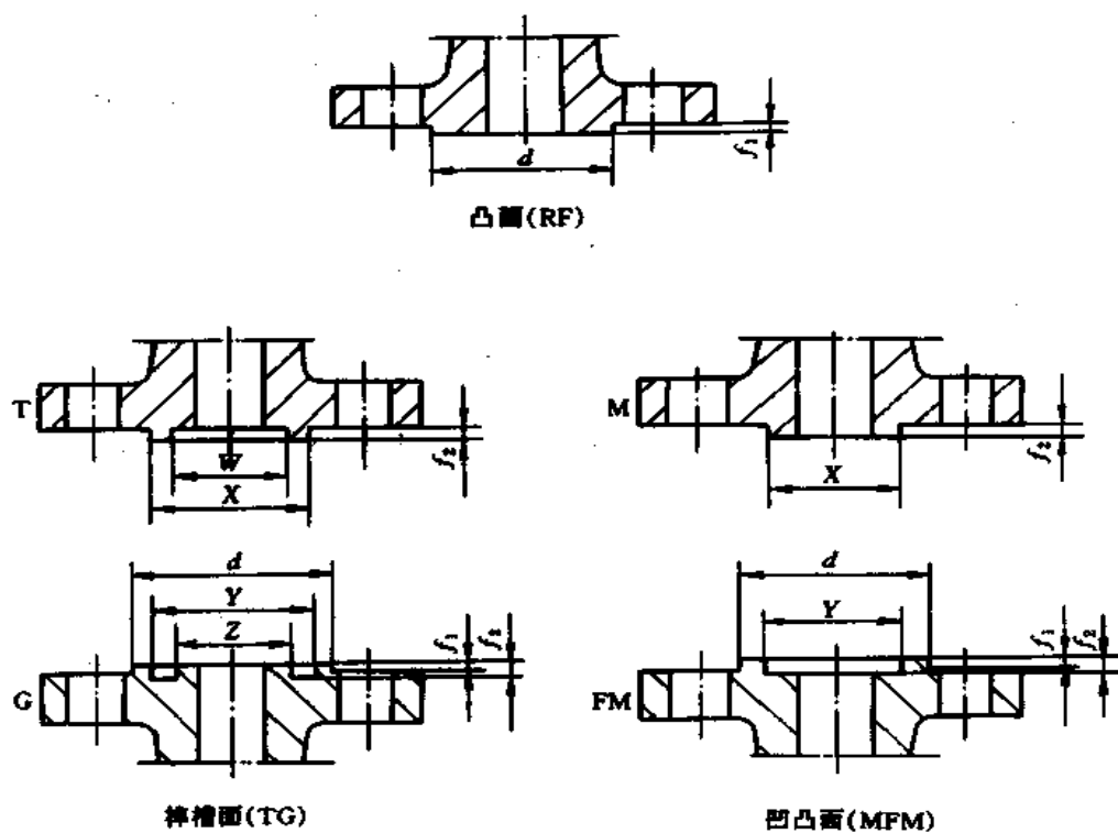
图 10.2.3.1-2 HGJ 44~76 密封面尺寸示意图
