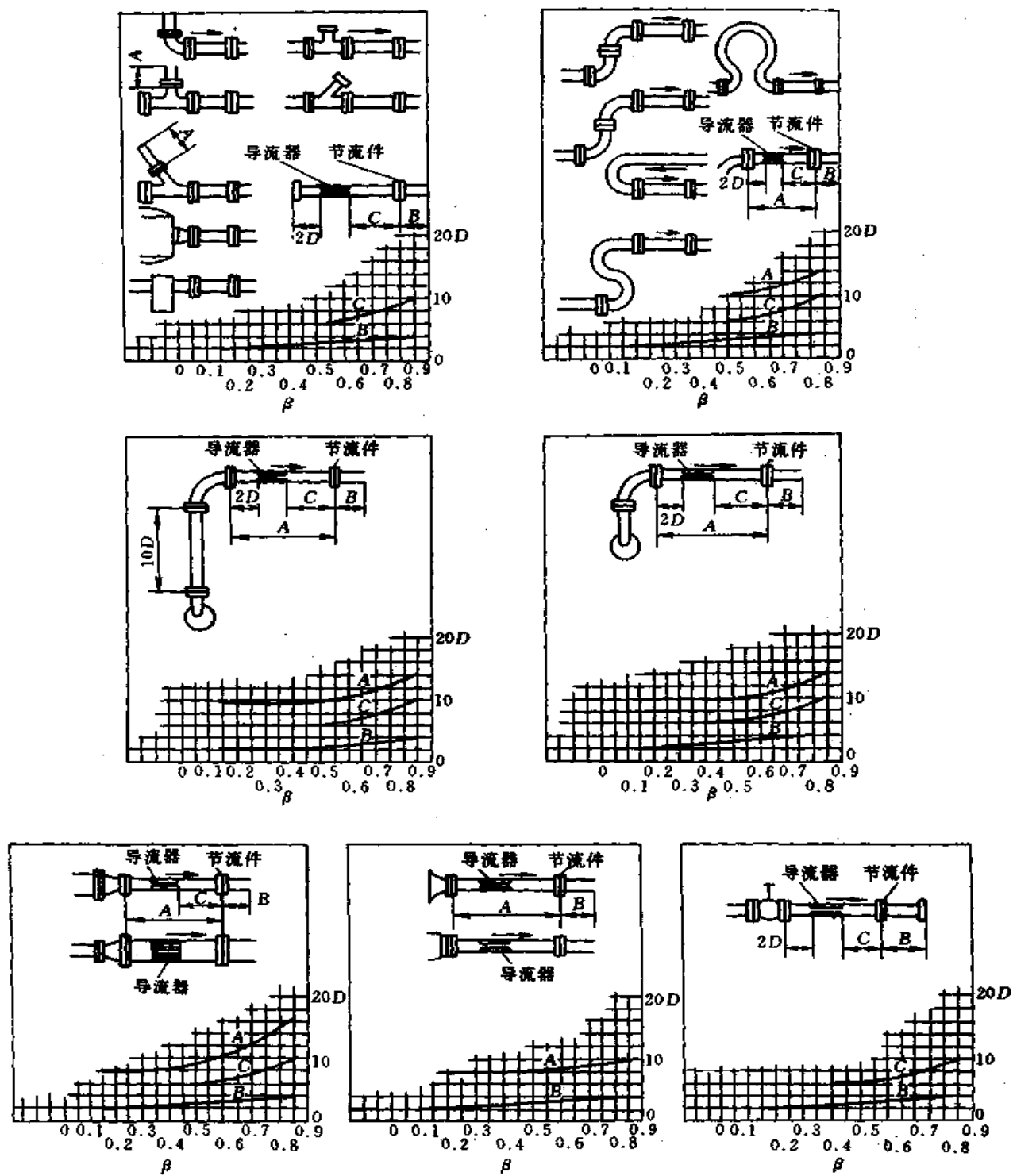
图 4.1.7-3 加装导流器后最小直管段长度图
