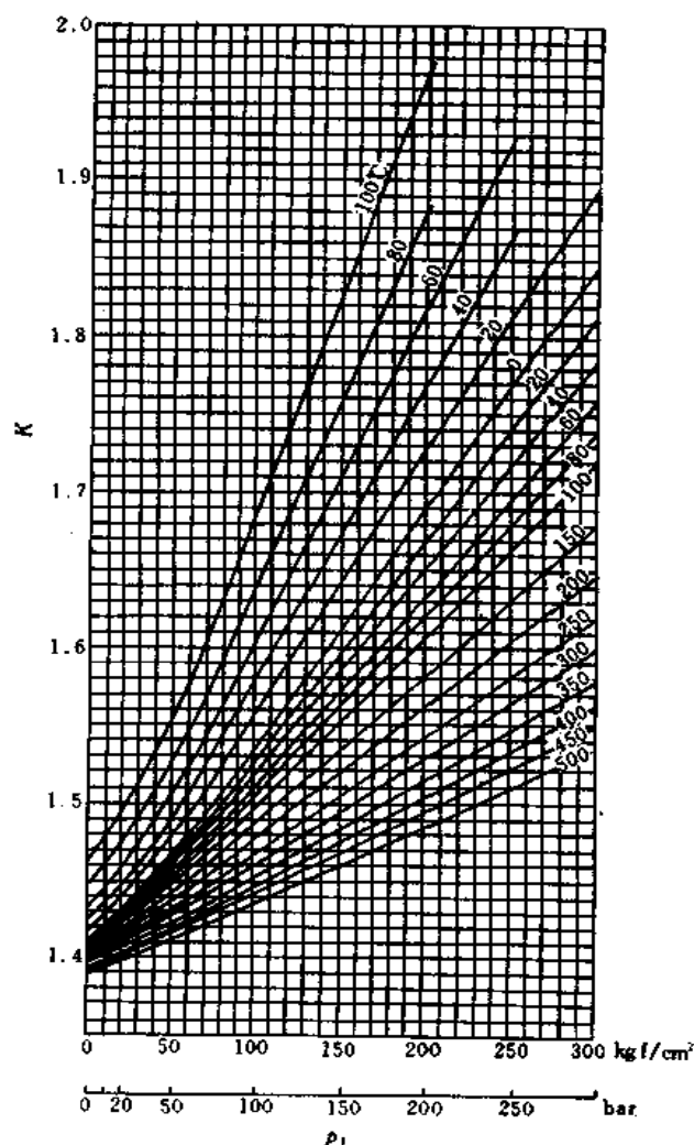
图 5.1.6-7 氢气 ( H_2 ) 的等熵指数图 K
