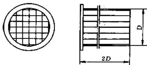
图 4.1.7-2 网格式导流器示意图
