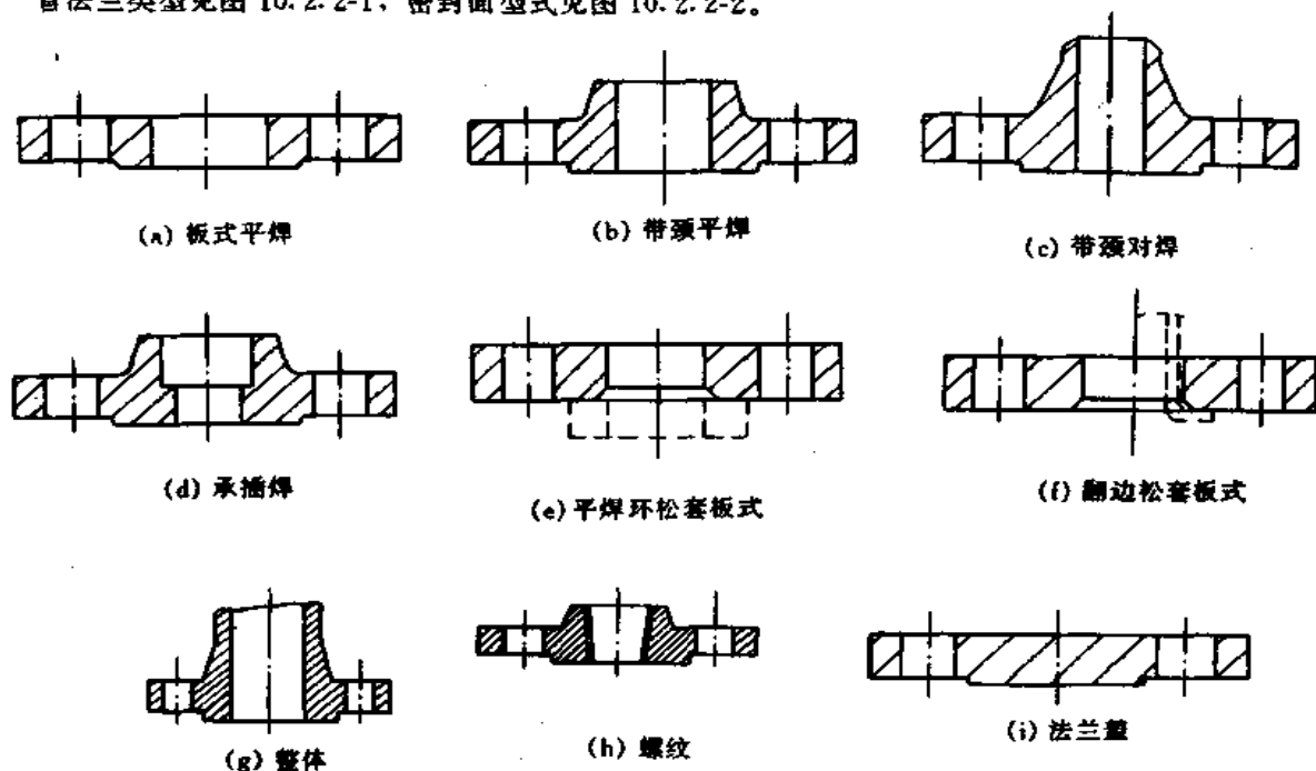
图 10.2.2-1 法兰类型
