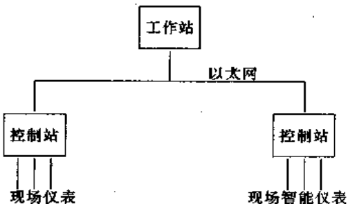
图 7.7 Delta V 系统构成图
