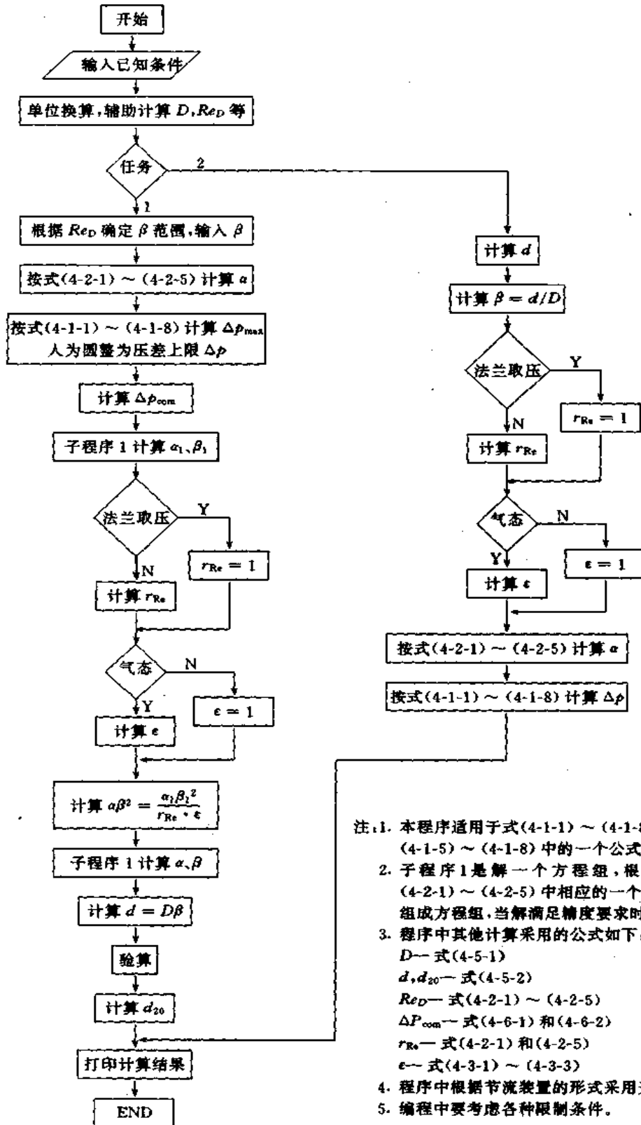
图 4.1.3 计算程序框图
