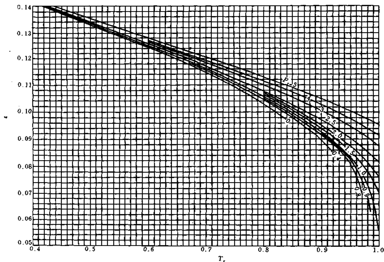
图 5.2.3 液体的膨胀系数图 W
