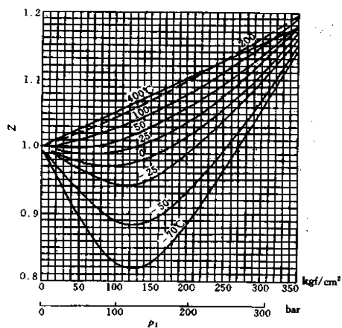
图 5.1.5-9 甲烷 ( \text{CH}_4 ) 的压缩系数图 Z
