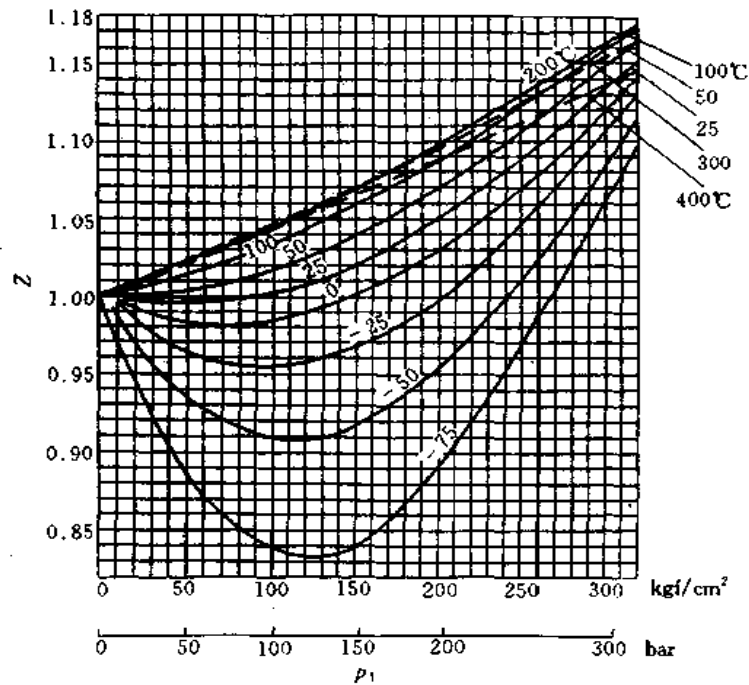
图 5.1.5-4 氮气 ( \text{N}_2 ) 的压缩系数图 Z
