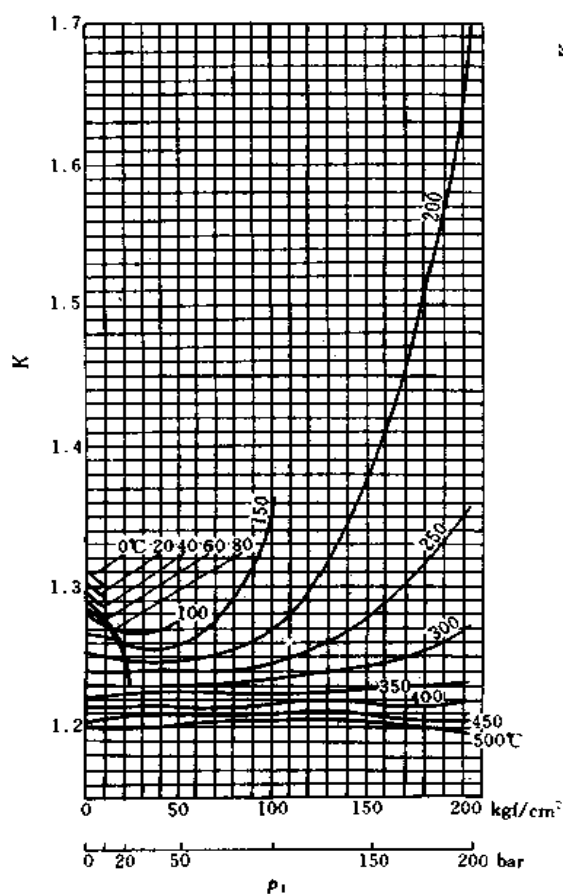
图 5.1.6-5 氨气 ( \text{NH}_3 ) 的等熵指数图 K
