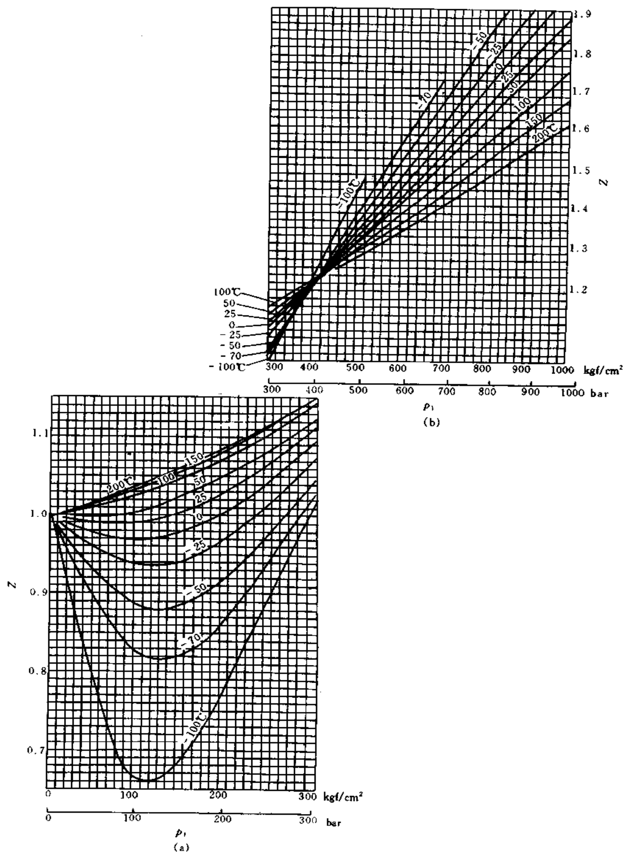
图 5.1.5-1 空气的压缩系数图 Z
