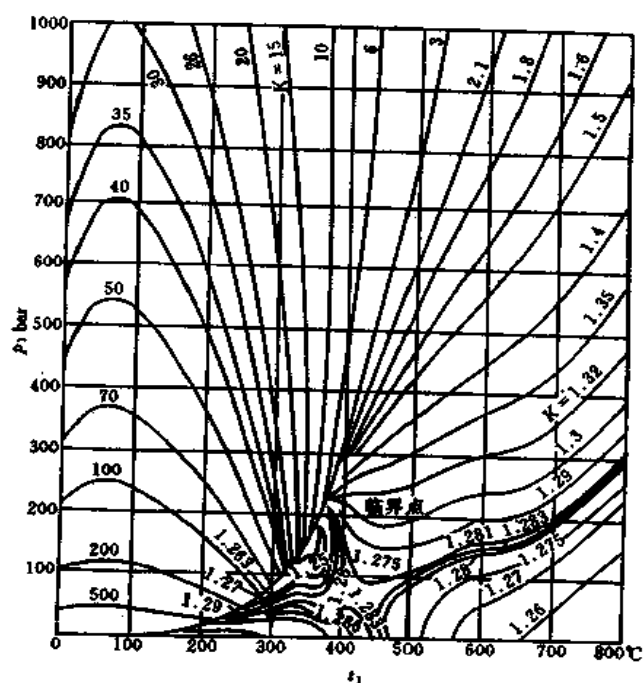
图 5.1.6-8 水蒸气的等熵指数图 K
