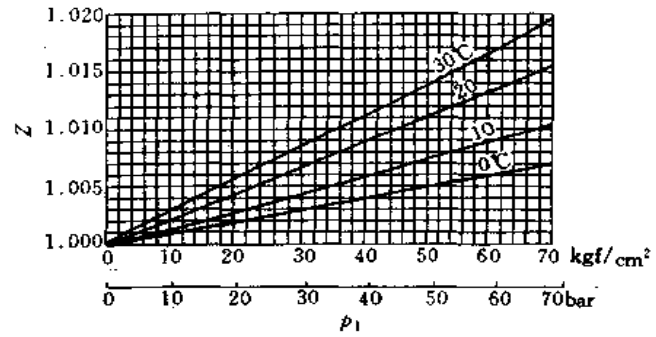
图 5.1.5-2 焦炉煤气的压缩系数图 Z
