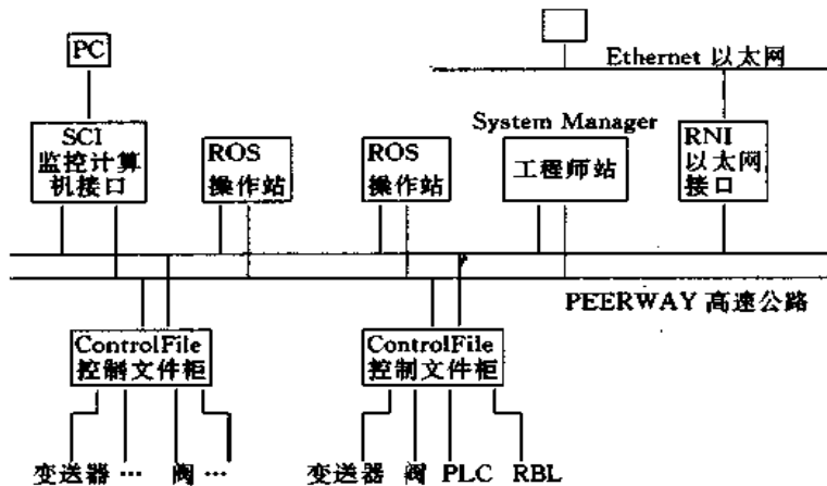
图 7.6 RS3 系统构成图
