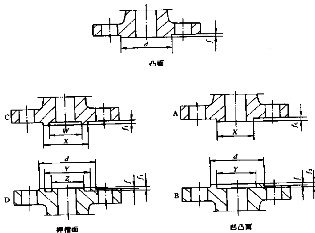
图 10.2.3.1-1 GB 9112~9131 和 JB/T 74~90 密封面尺寸示意图
