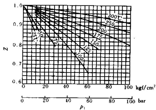
图 5.1.5-6 氨气 ( \text{NH}_3 ) 的压缩系数图 Z
