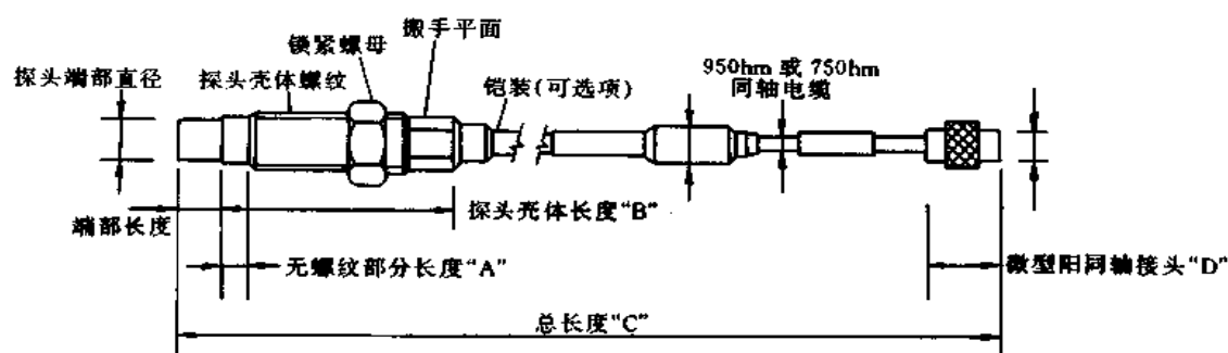
图 12.1.1 探头外形和尺寸示意图 (标准安装式)
