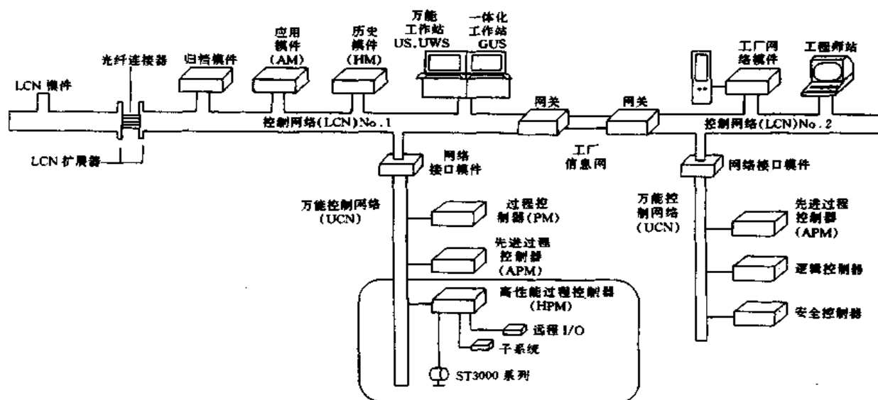
图 7.3 TDC 3000 (TPS) 系统构成
