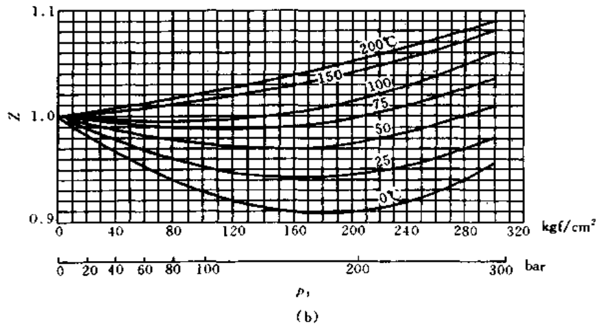
图 5.1.5-3 氧气 ( \text{O}_2 ) 的压缩系数图 Z
