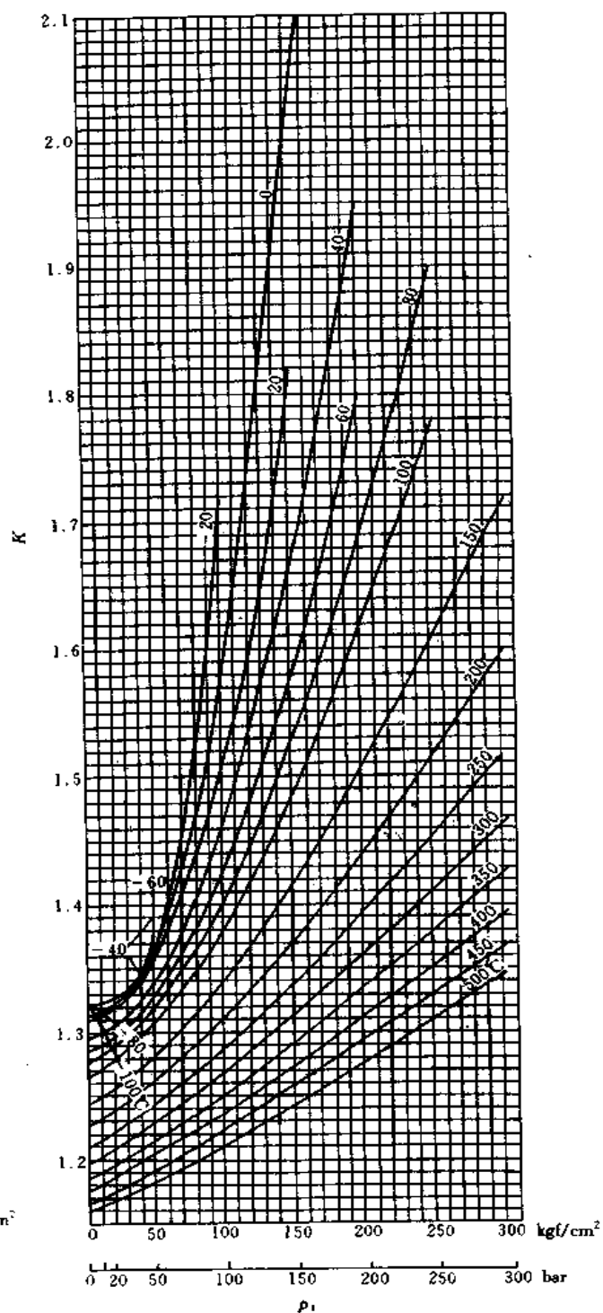
图 5.1.6-6 甲烷 ( \text{CH}_4 ) 的等熵指数图 K
