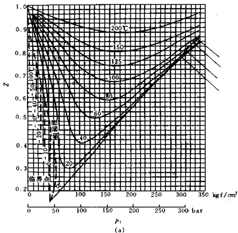
图 5.1.5-10 天然气的压缩系数图 Z
