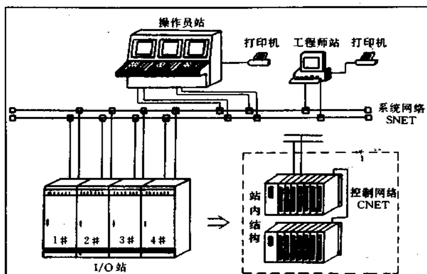
图 7.1 HS2000M 中型分布式控制系统
