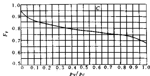
图 4.2.1.1-1 F_F \sim p_v/p_c 关系曲线
