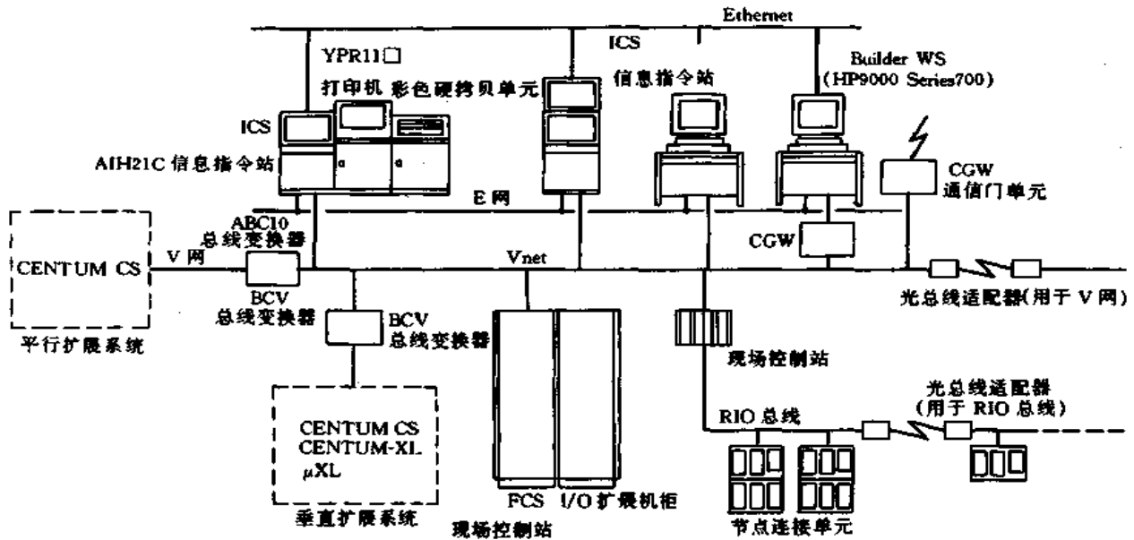
图 7.5 CENTUM-CS 系统构成图
