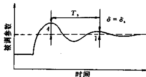
图 12.10.2-1 4:1 衰减过程曲线
