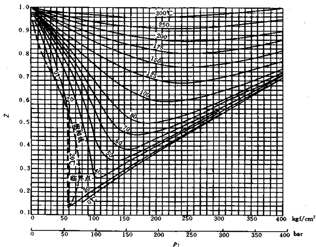
图 5.1.5-8 二氧化碳 ( \text{CO}_2 ) 的压缩系数图 Z
