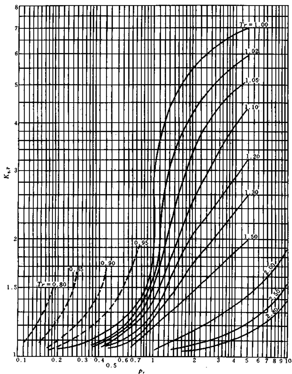
图 5.1.2-2 气体粘度的压力修正系数图 K_{\eta, p}
