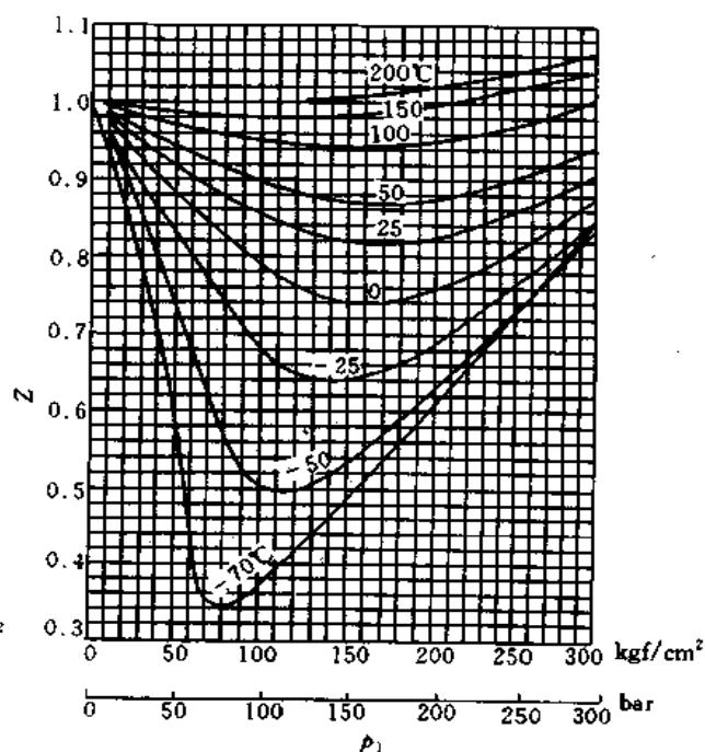
图 5.1.5-7 一氧化碳 ( \text{CO} ) 的压缩系数图 Z
