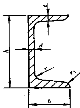
图 9.2.5 常用热轧槽钢
