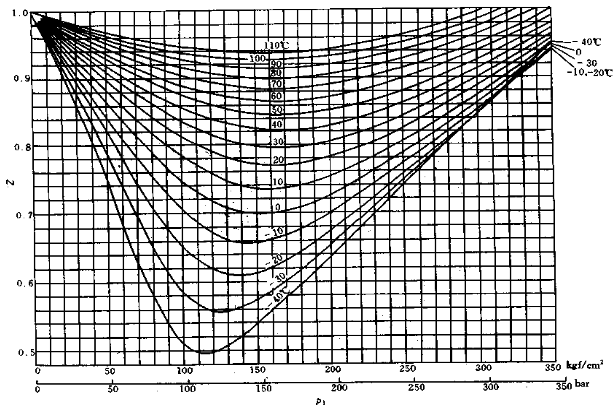
图 5.1.5-10 天然气的压缩系数图 Z
