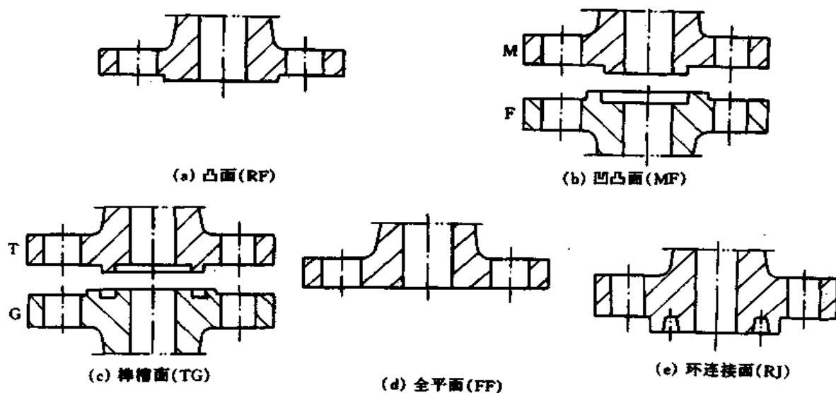
图 10.2.2-1 法兰类型
