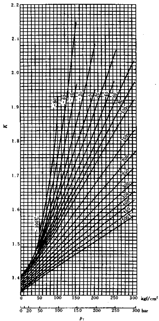
图 5.1.6-1 空气的等熵指数图 K
