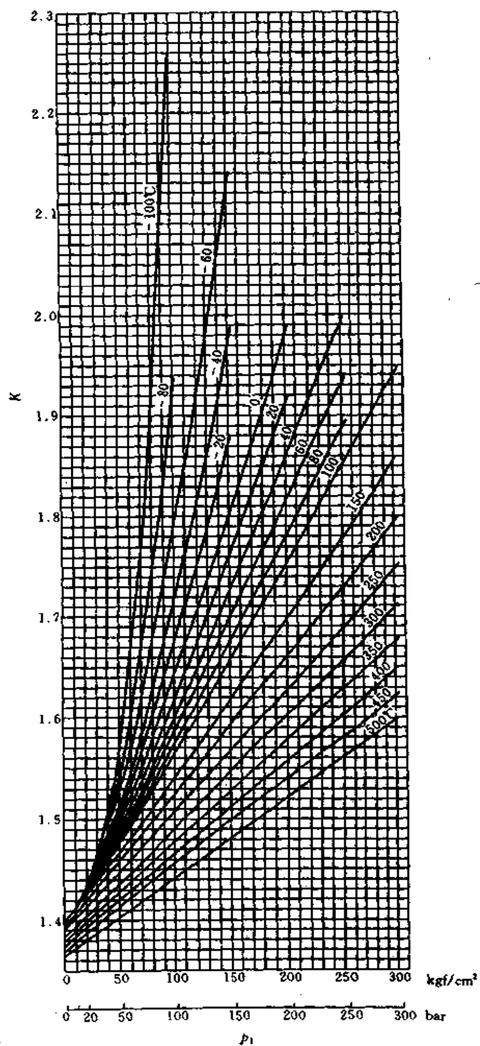
图 5.1.6-3 氮气 ( \text{N}_2 ) 的等熵指数图 K
