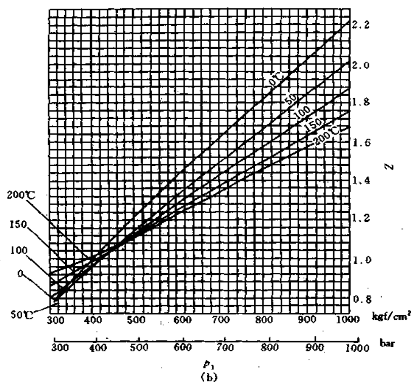
图 5.1.5-11 乙烯 ( C_2H_4 ) 的压缩系数图 Z
