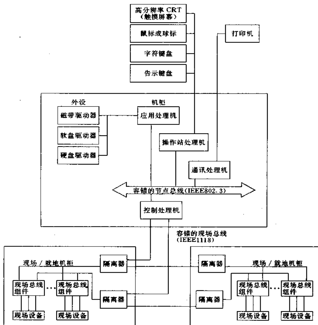
图 7.8 典型的 I/A S 单节点系统
