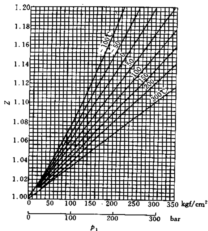
图 5.1.5-5 氢气 ( \text{H}_2 ) 的压缩系数图 Z
