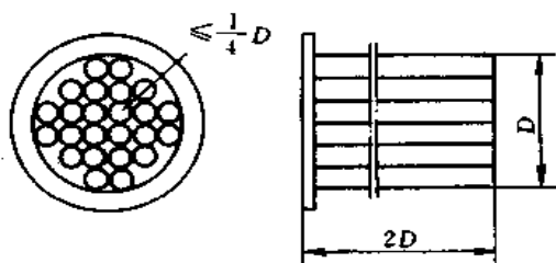
图 4.1.7-1 管式导流器示意图
