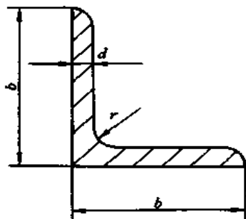
图 9.2.4 常用热轧等边角钢
