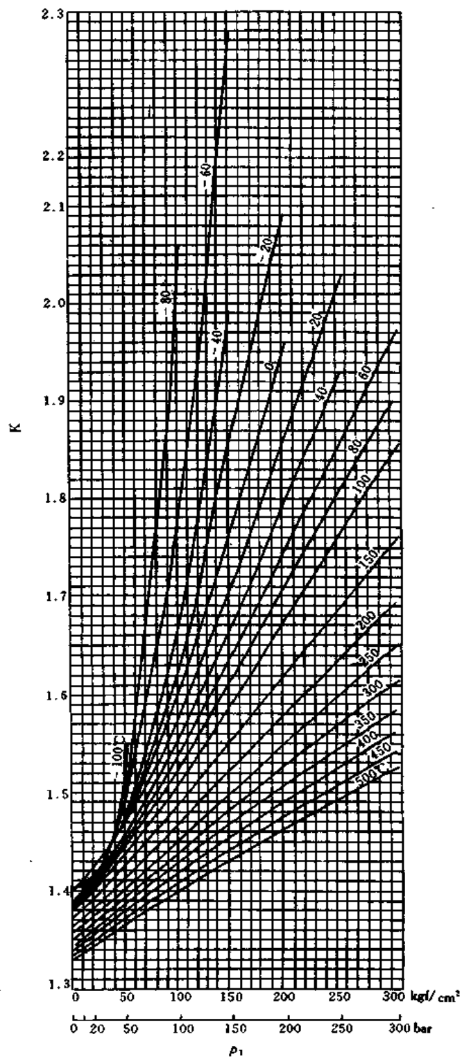
图 5.1.6-2 氧气 ( O_2 ) 的等熵指数图 K
