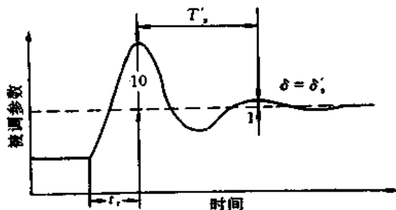
图 12.10.2-2 10:1 衰减过程曲线
