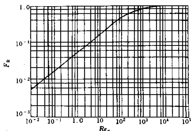
图 4.2.1.1-2 F_R \sim Re_v 关系曲线
