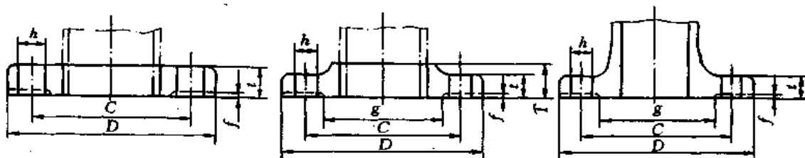
图 10.2.5.3 JIS 10K RF 管法兰
