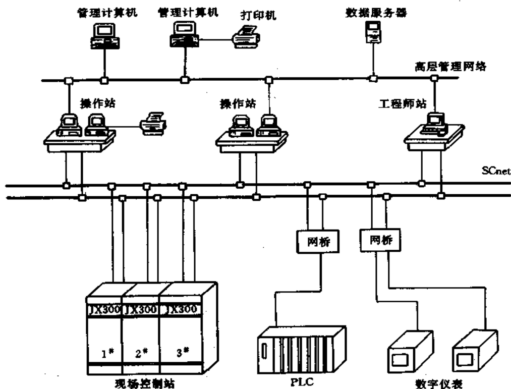
图 7.2 SUPCON JX-300 系统构成图
