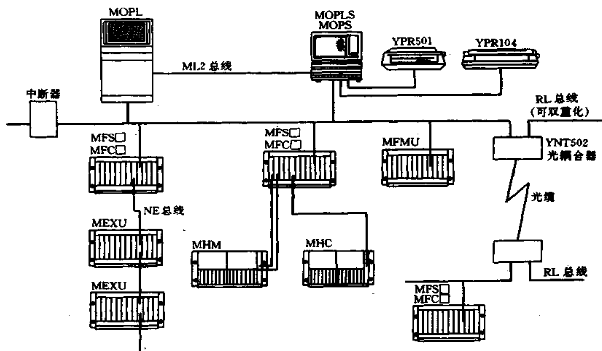
图 7.4 \mu XL 系统构成
