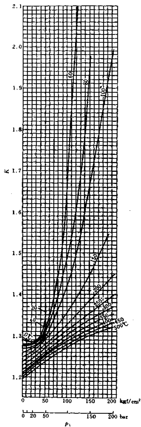
图 5.1.6-4 二氧化碳 ( \text{CO}_2 ) 的等熵指数图 K
