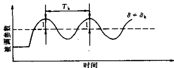
图 12.10.1 临界振荡过程曲线
