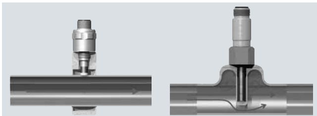
Siemens clamp-on
