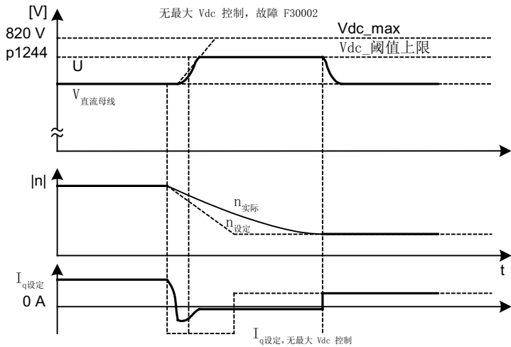
图 3-17 最大 Vdc 控制的激活/取消
