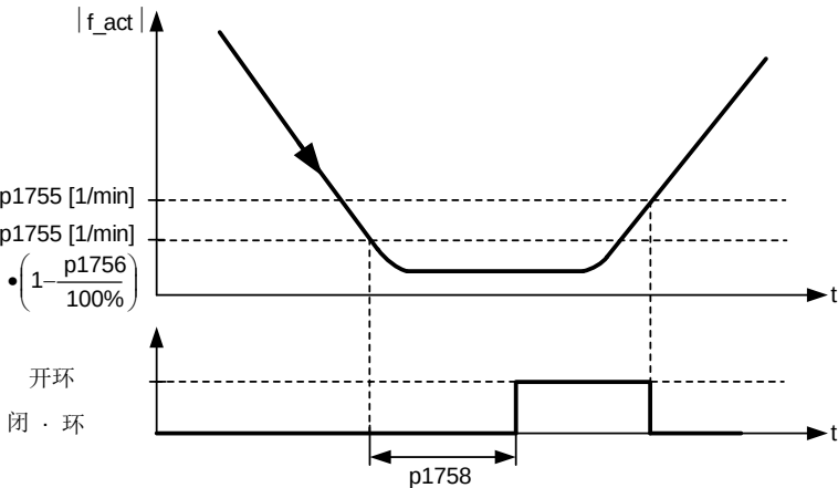
图 4-1 SLVC 的切换条件
