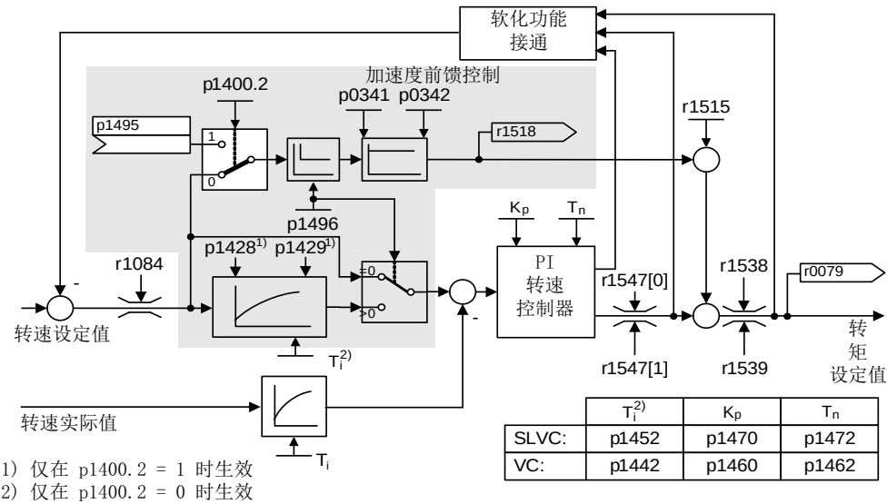
图 4-9 带前馈控制的转速控制器
