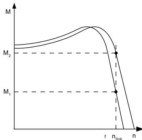
图 5-5 转差补偿
