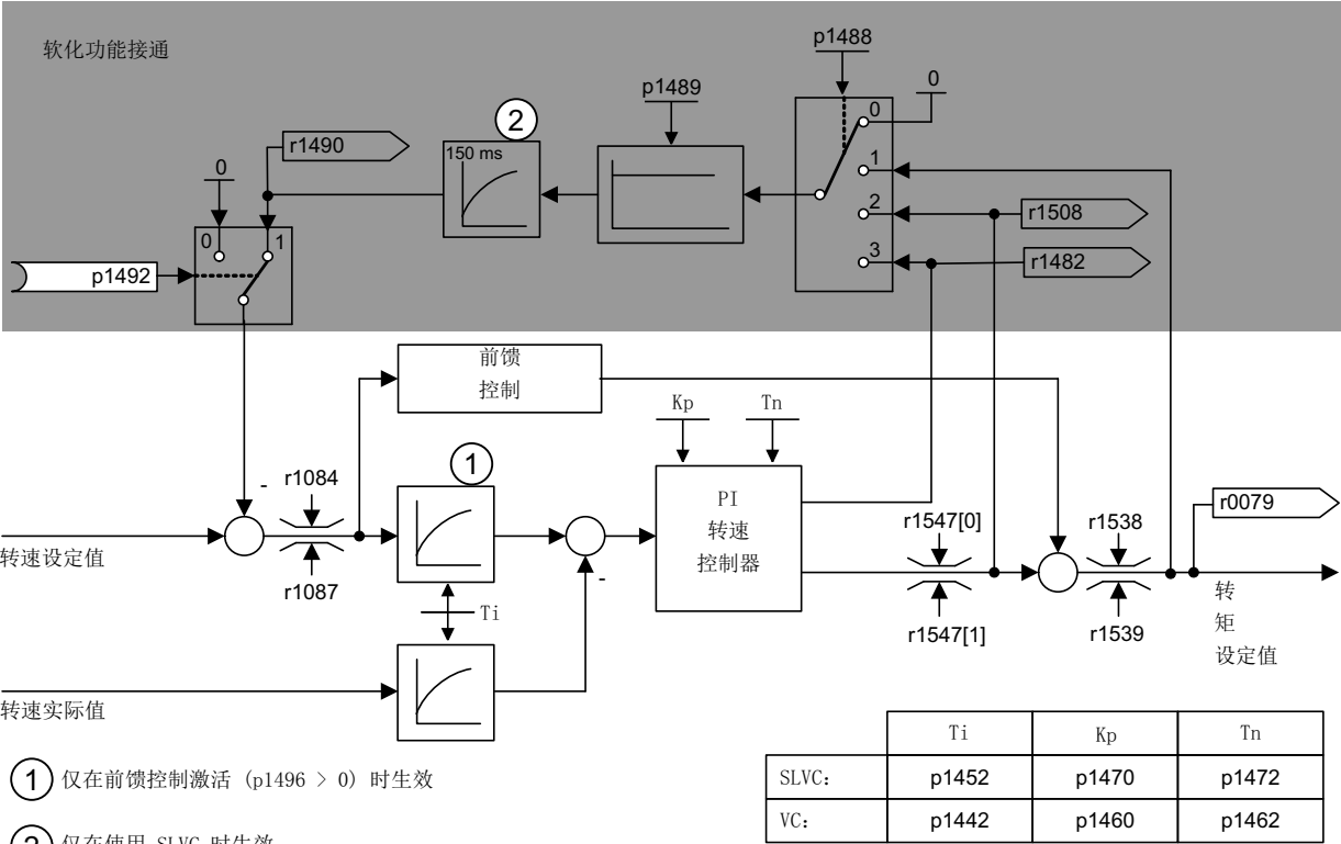
图 4-11 带有软化功能的转速控制器
