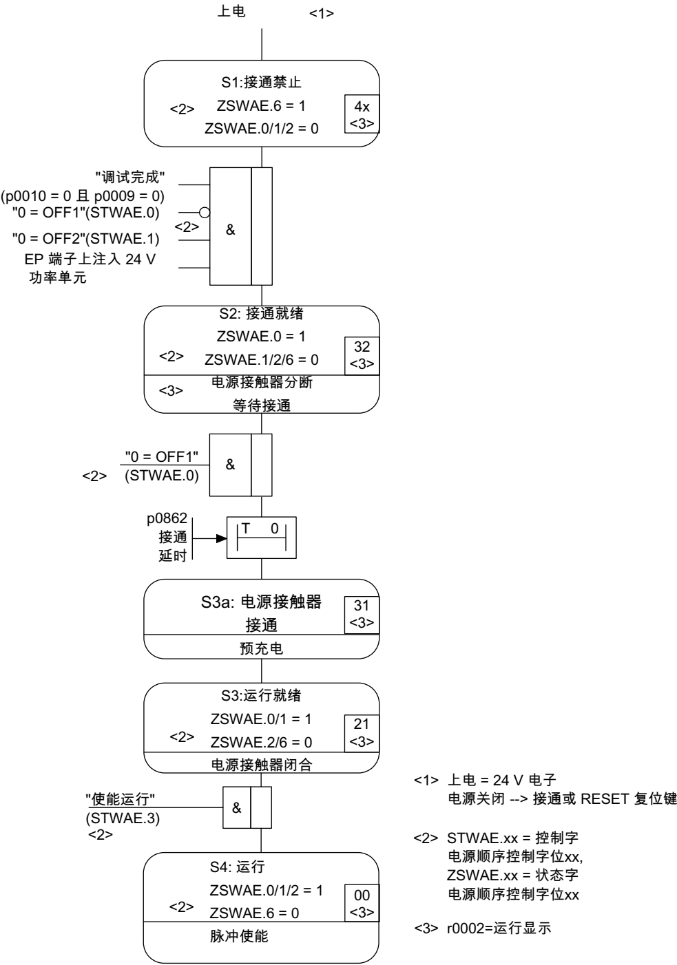
图 1-6 非调节型电源的启动过程
