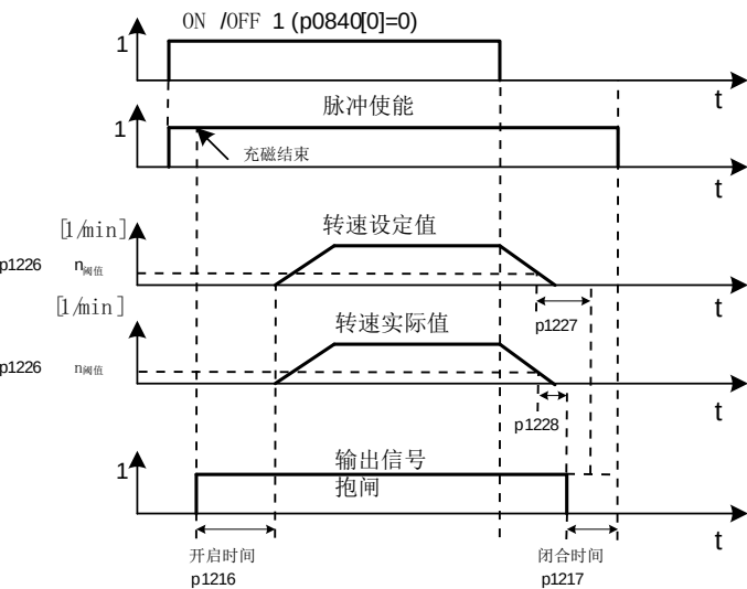
图 6-7 简单制动控制的时序图
