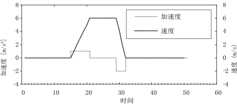
图 7-15 没有加加速度限制
