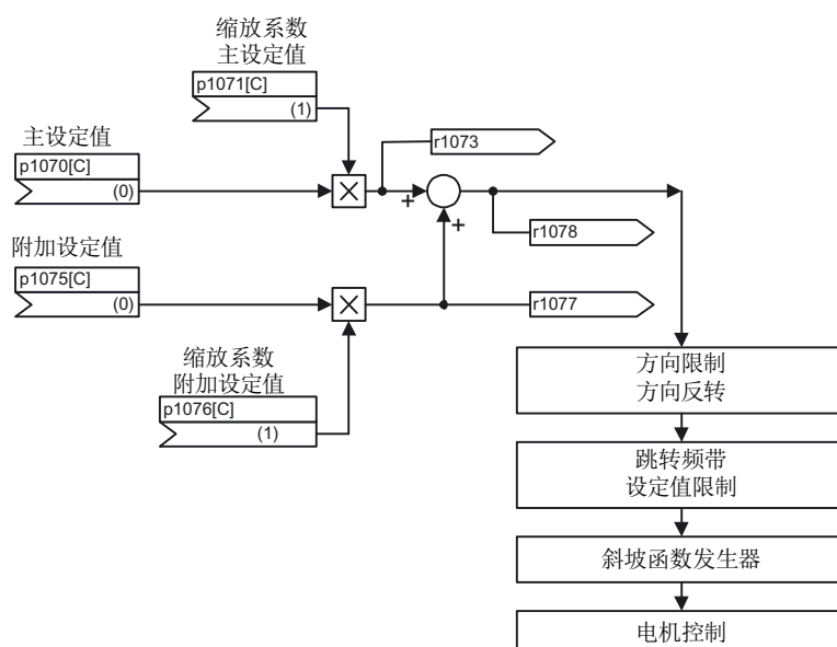
图 2-5 设定值相加，设定值比例系数
