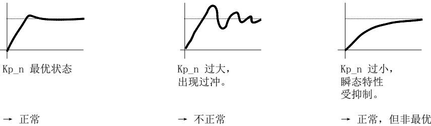
图 3-12 比例增益 Kp 的设置
