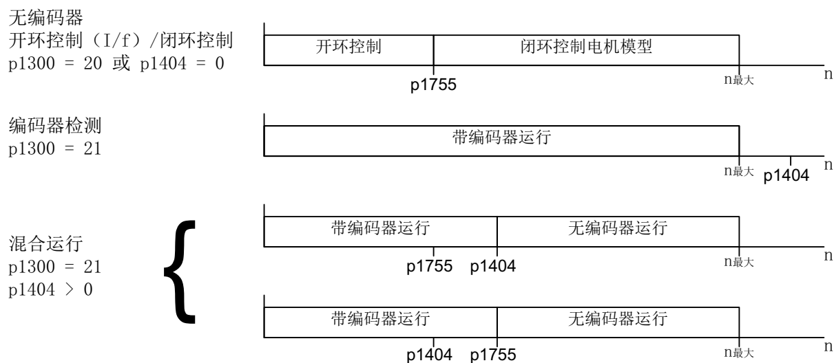
图 3-13 区域切换
