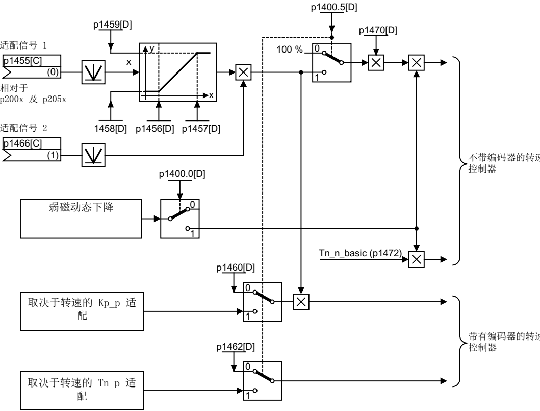
图 3-3 自由 Kp_n 适配
