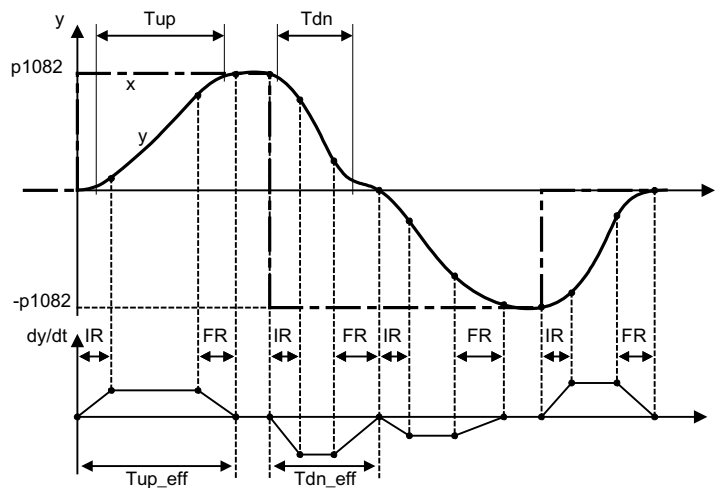
图 2-9 扩展斜坡函数发生器
