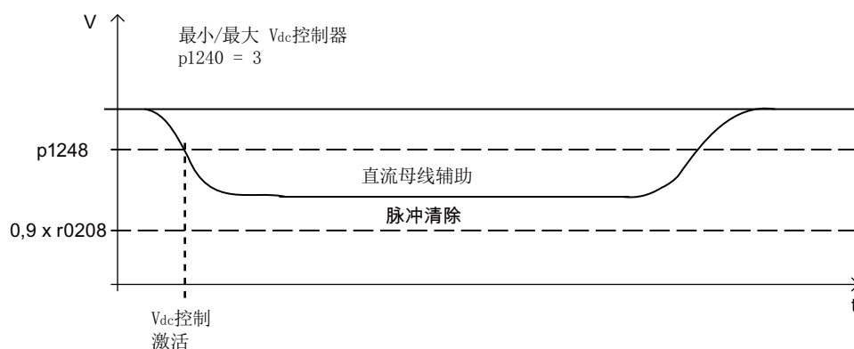
图 7-31 直流母线电压设定值
