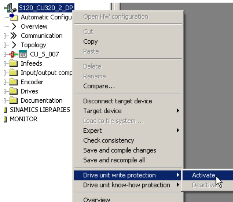
图 12-27 激活写保护
