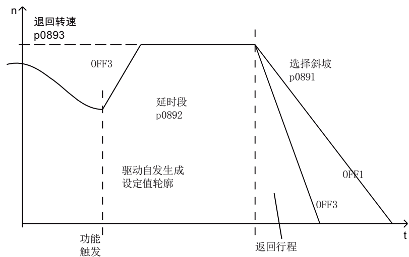
图 7-29 含“扩展退回”的 OFF 斜坡
