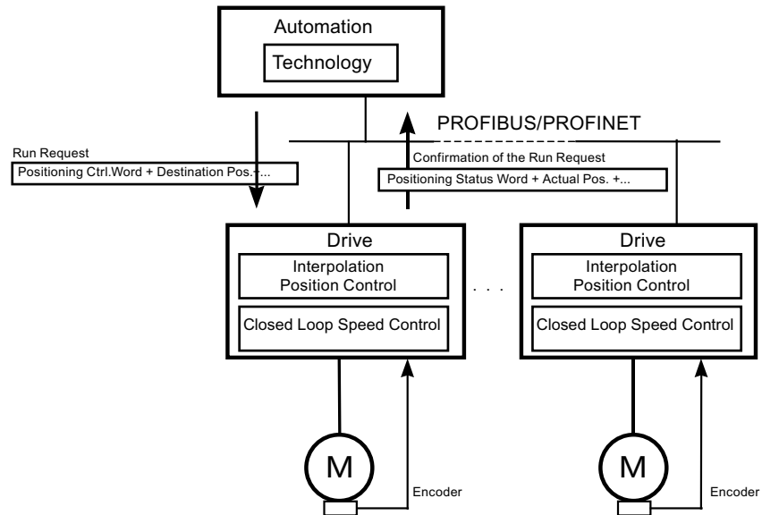
图 10-3 应用等级 3
