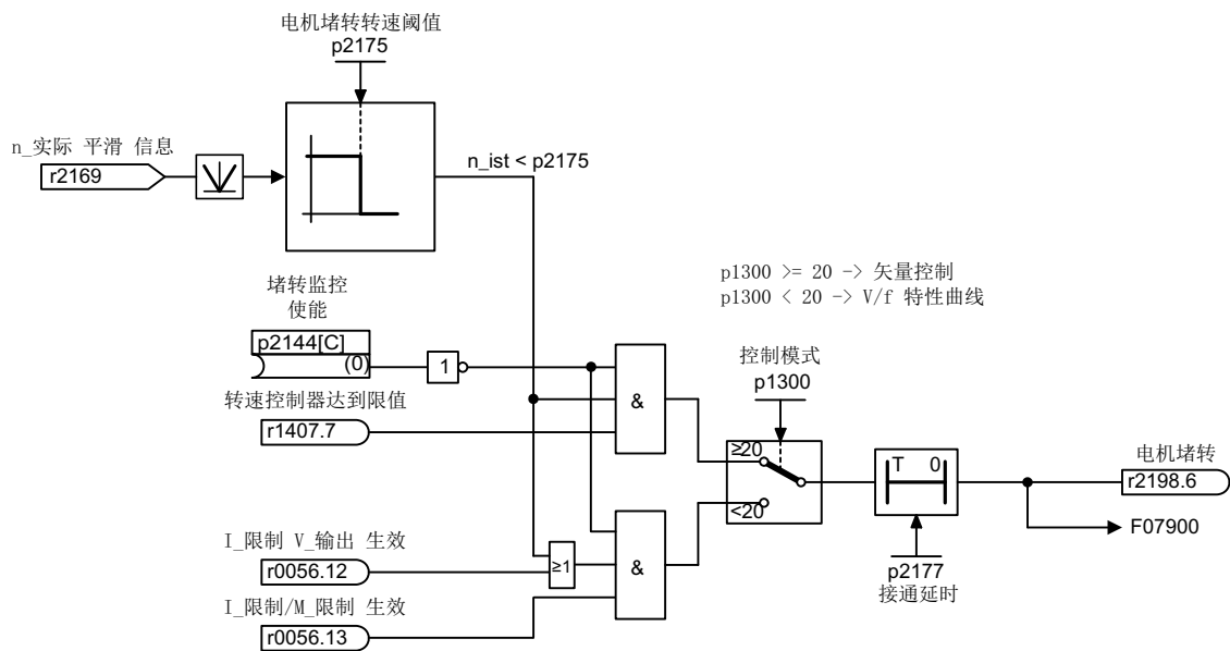
图 8-1 堵转保护
