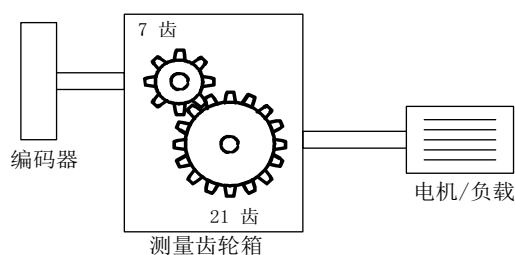
图 6-14 测量齿轮箱
