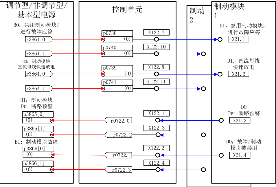
图 7-5 示例：控制两个书本型制动模块
