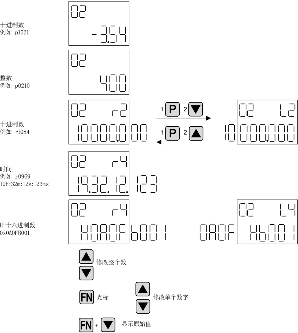
图 12-11 数值显示
