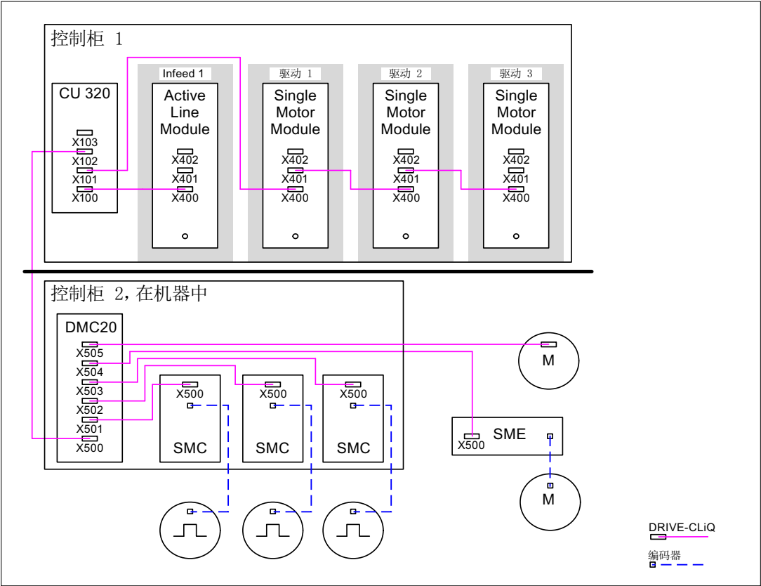
图 11-4 示例：带 DMC20 的分散拓扑结构
