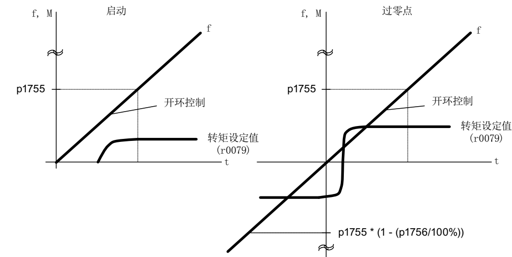
图 4-4 低速区内开环控制中的过零点和启动
