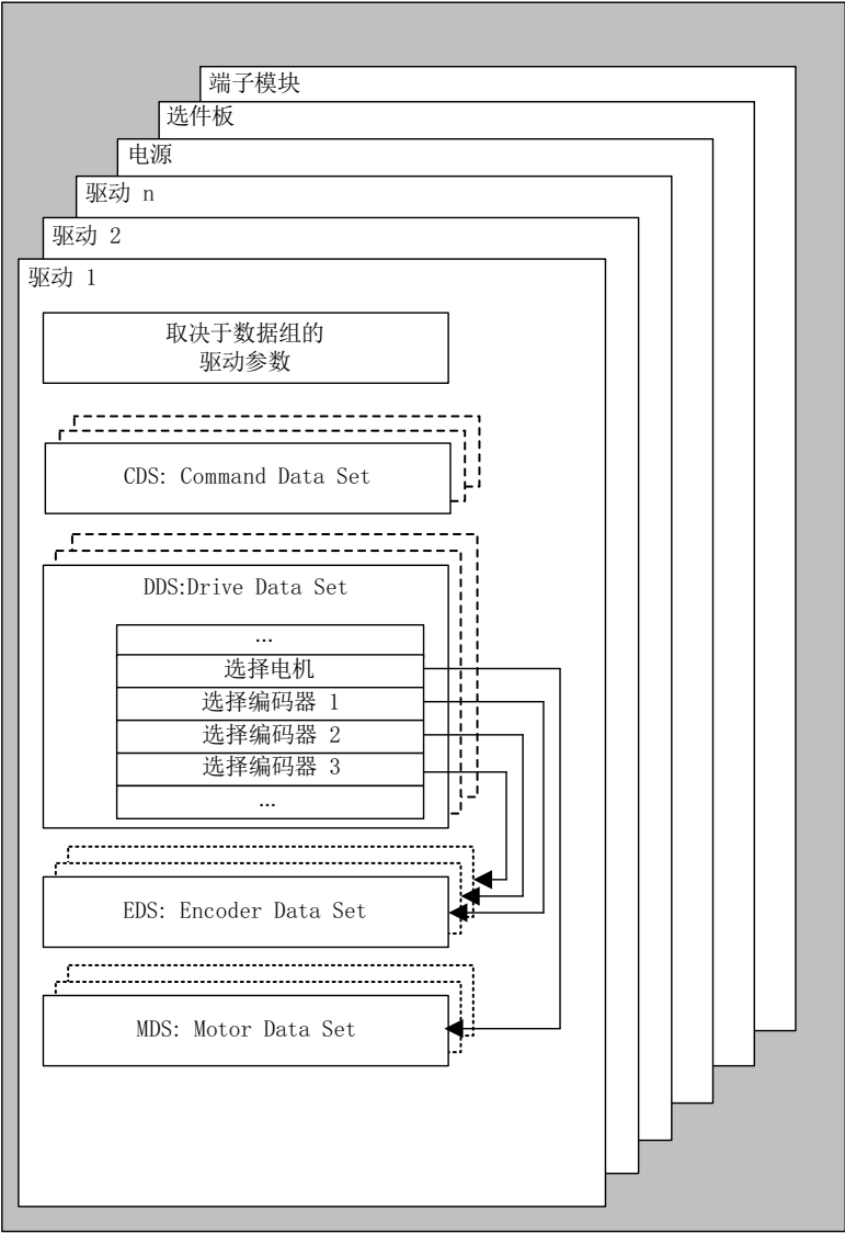
图 12-2 参数分类
