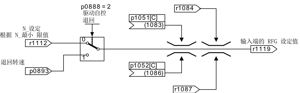
图 7-30 将设定值通道连接至斜坡函数发生器
