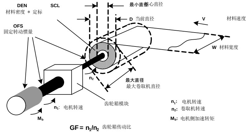
图 11-6 轴卷取机的结构
