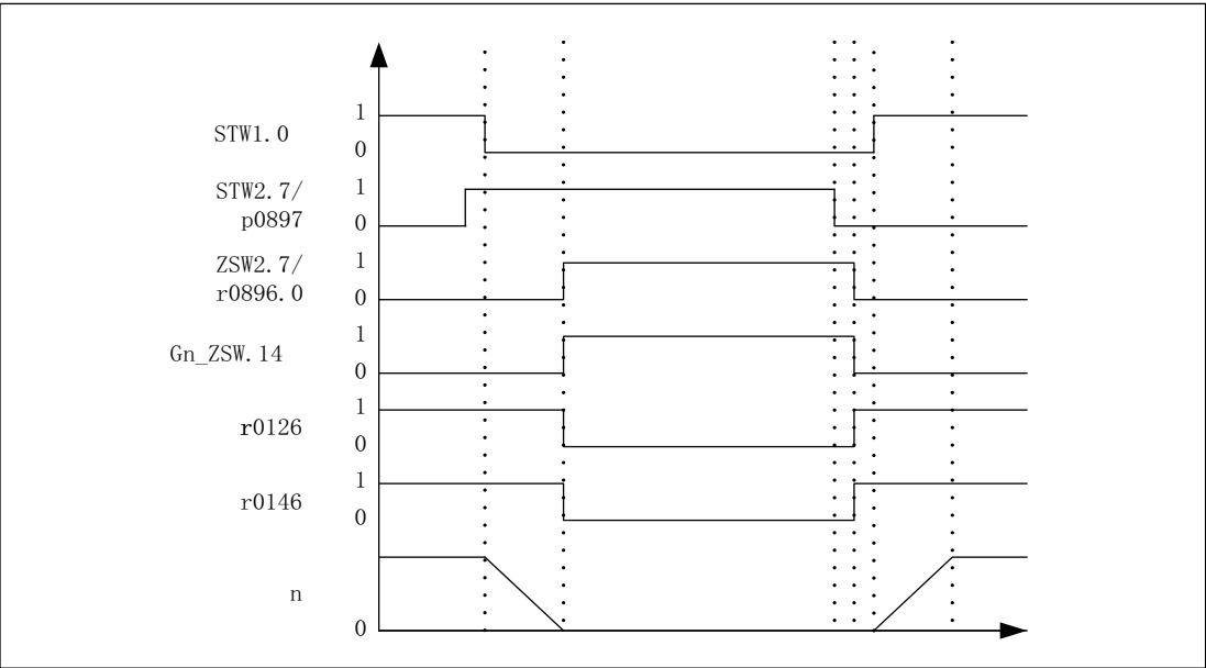
图 6-11 驻留轴的时序图
