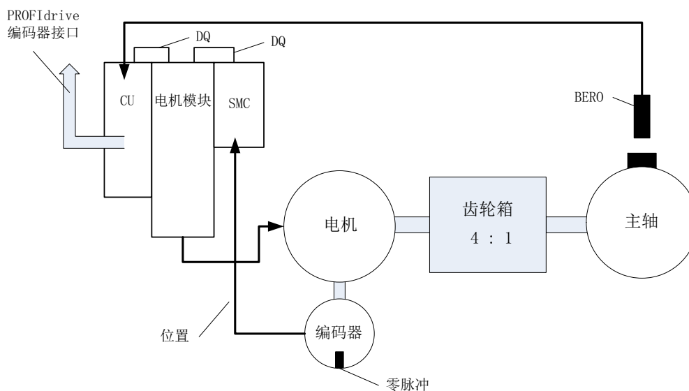
图 7-18 电机和主轴间存在齿轮箱的结构
