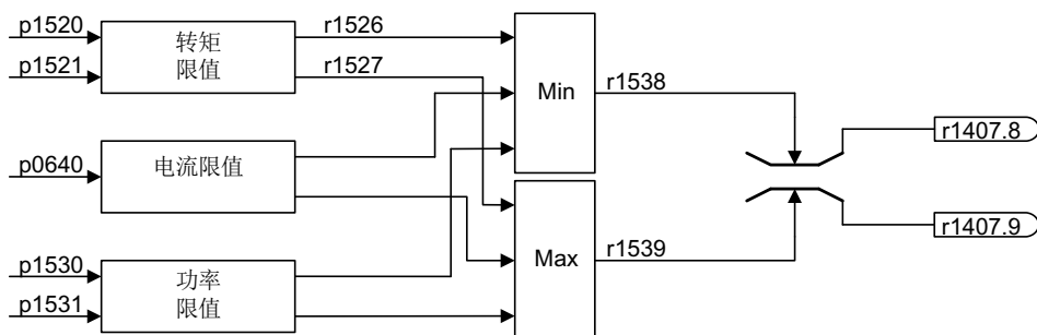
图 4-14 转矩限制
