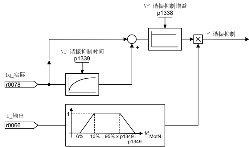
图 5-6 谐振抑制
