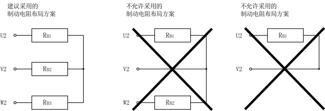
图 6-5 制动电阻
