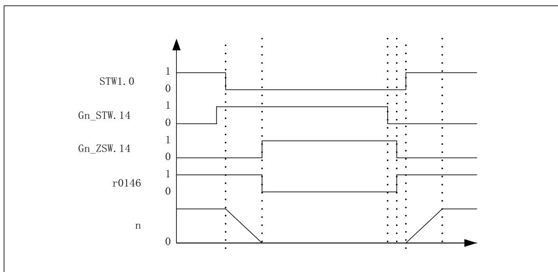
图 6-12 驻留编码器的时序图
