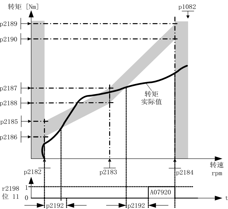
图 7-3 负载监控
