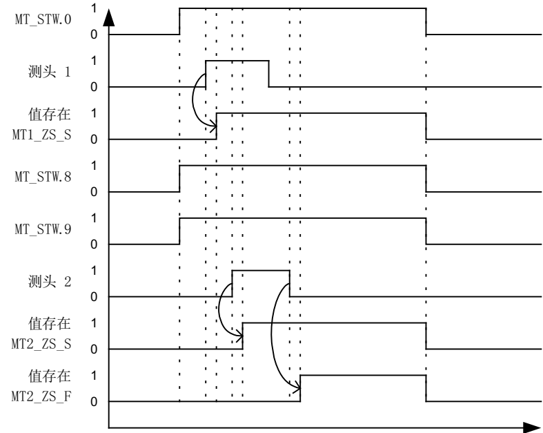
图 10-13 中央测头示例的时序图
