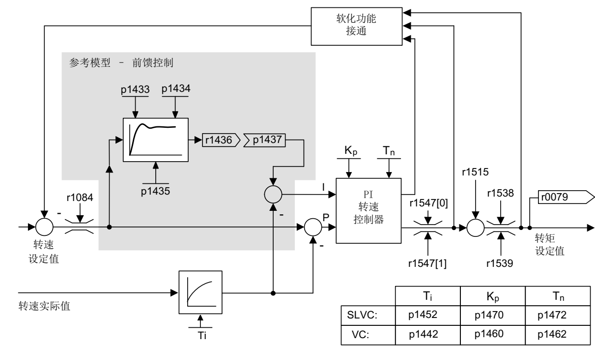
图 4-10 参考模型
