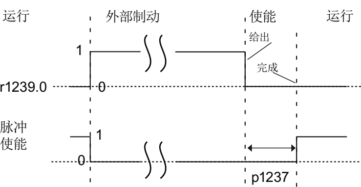
图 6-3 脉冲使能 - 使用无接触器反馈的外部电枢短路制动时的信号特性
