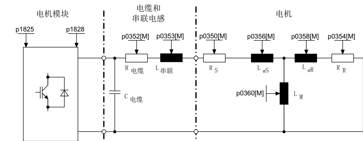
图 4-23 异步电机和电缆的等效电路图
