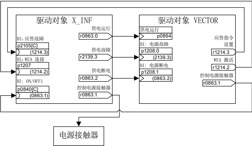
图 11-1 BICO 互联
