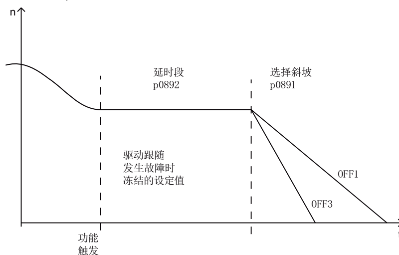
图 7-28 包含延时段的 OFF 斜坡
