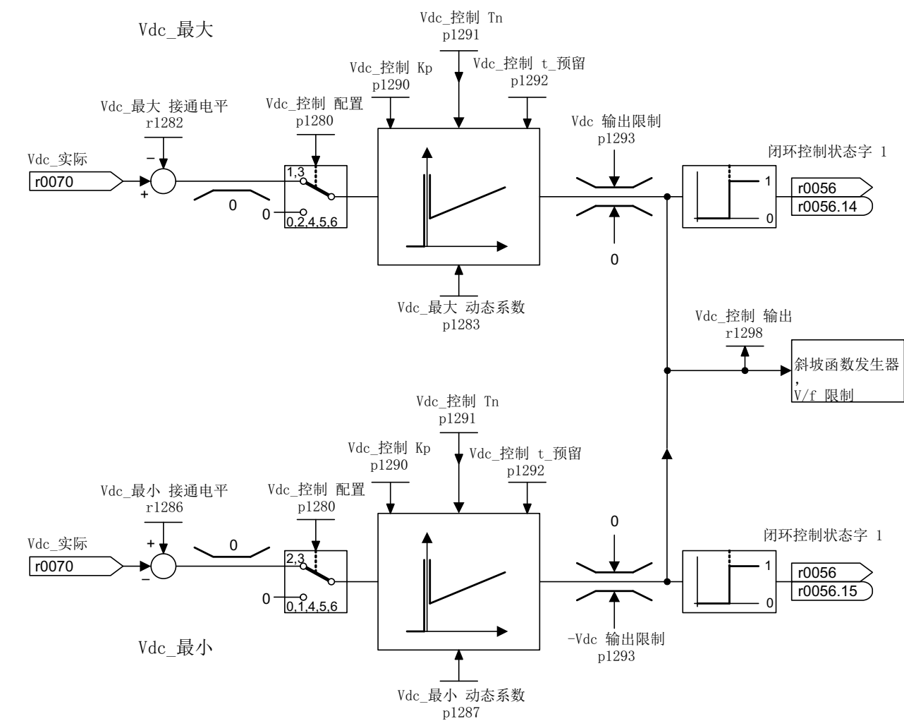
图 5-7 Vdc 控制 V/f
