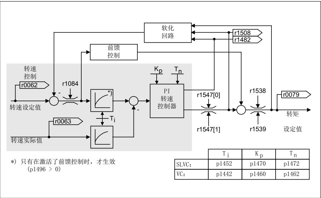
图 4-6 转速控制器
