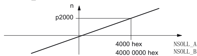
图 10-5 转速定标
