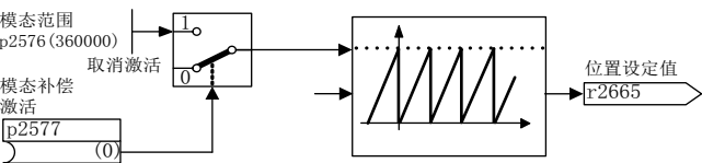
图 7-14 模态补偿
