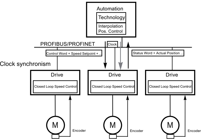
图 10-4 应用等级 4
