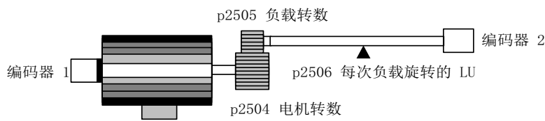
图 7-6 使用旋转编码器采集位置实际值
