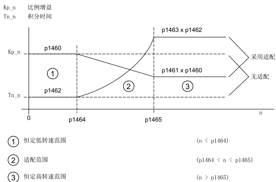
图 3-4 转速控制器 Kp\_n/Tn\_n 适配
