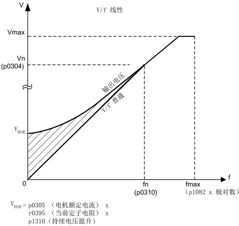
图 5-3 持续电压提升（示例：p1300 = 0, p1310 > 0）
