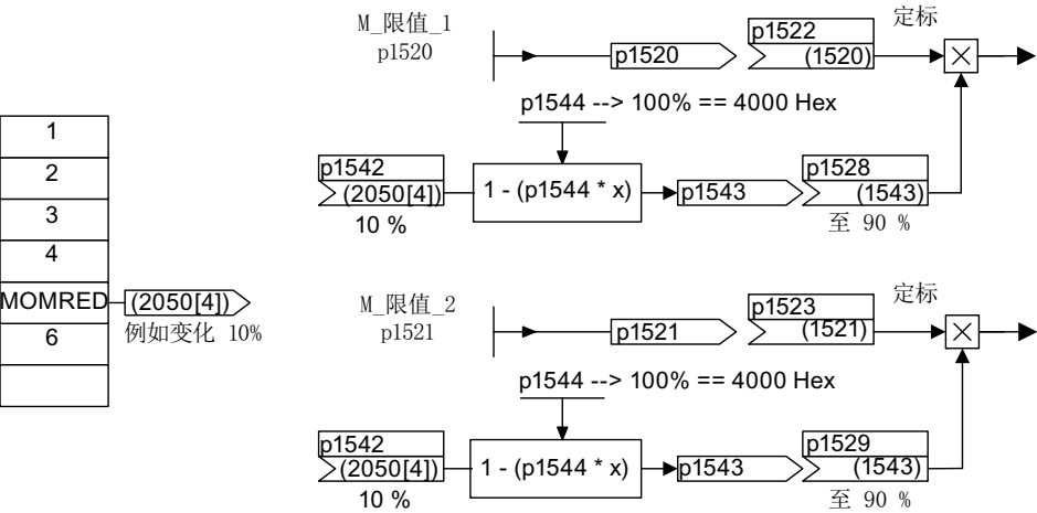
图 10-6 设定值 MOMRED
