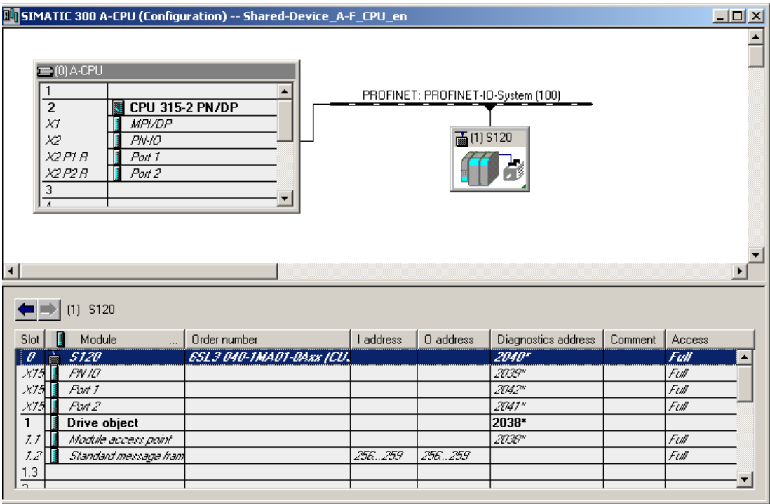
图 10-50 已在 HW-Config 中创建驱动控制系统
