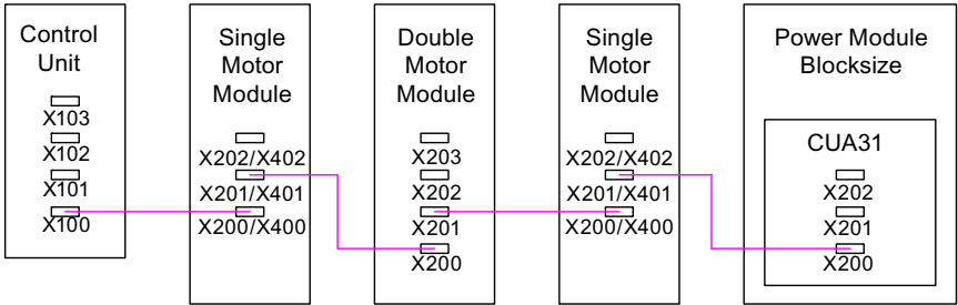
图 12-18 DRIVE-CLiQ 支路示例
