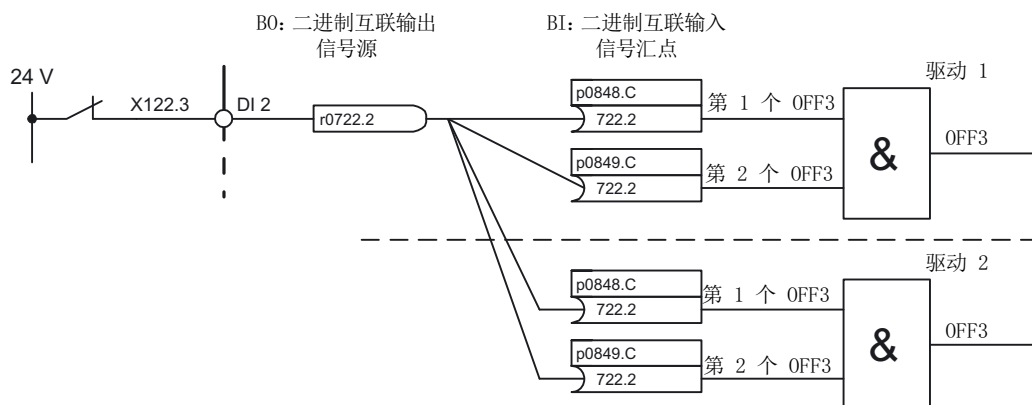
图 12-8 “OFF3”互联到多个驱动（示例）
