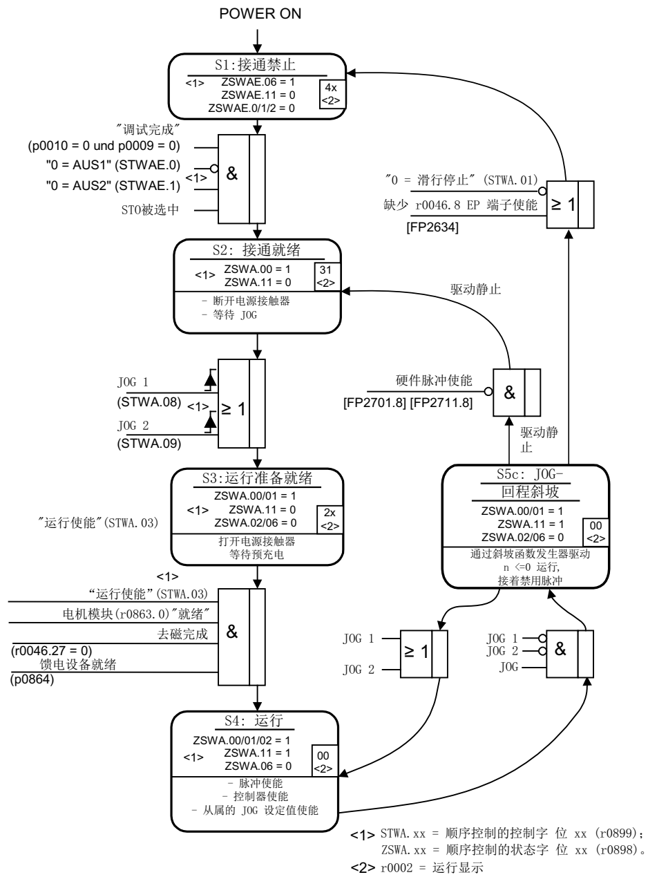
图 2-4 JOG 流程图
