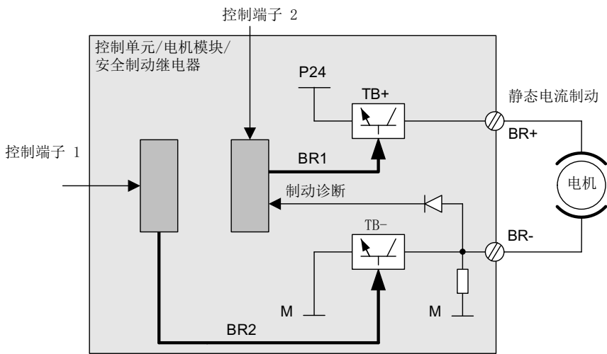
图 9-1 双通道式制动控制 模块型（示例）
