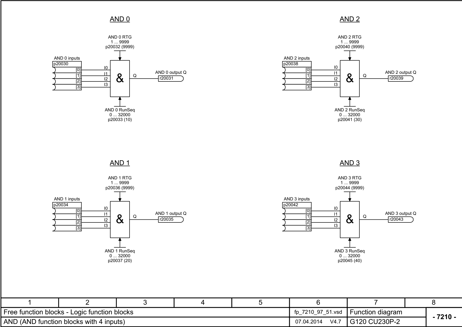
图 3-101 7210 - AND (有 4 个输入的“与”功能块)
