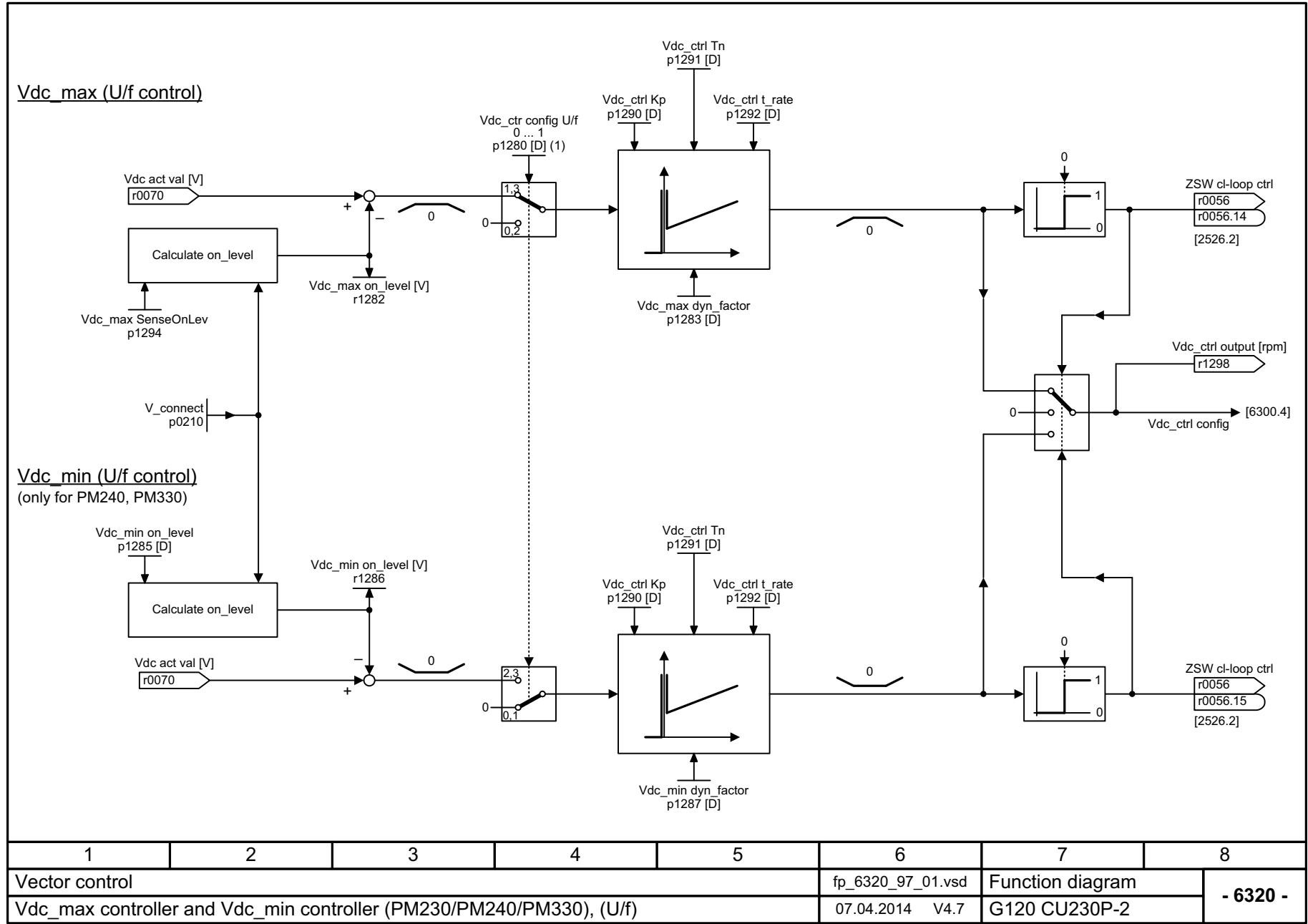
图 3-80 6320 - Vdc_max 控制器和 Vdc_min 控制器 (PM230/PM240/PM330), (V/f)
