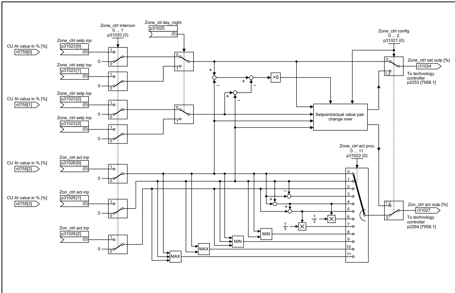
图 3-95 7032 - 多区域控制
