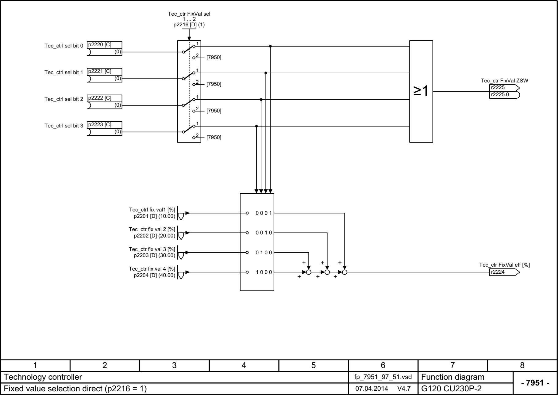
图 3-121 7951 - 固定值, 直接选择 (p2216 = 1)
