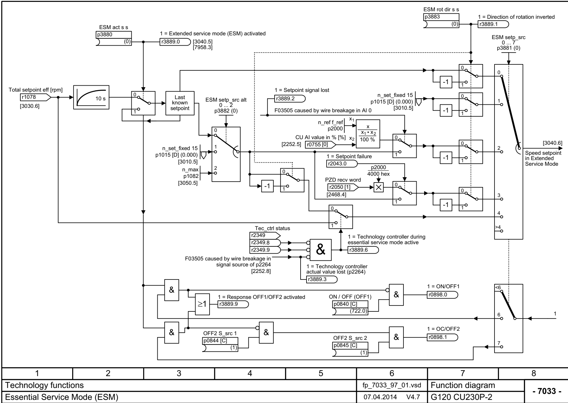
图 3-96 7033 - 紧急运行 (ESM, Essential Service Mode)
