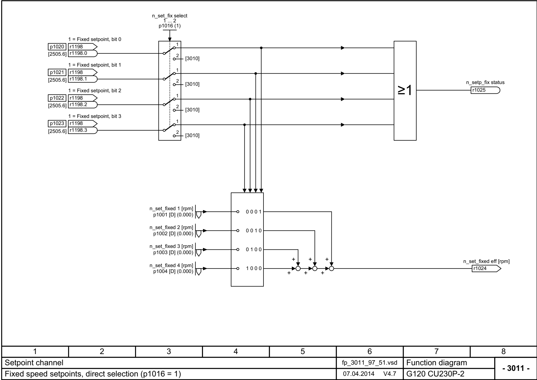
图 3-63 3011 - 转速固定设定值, 直接选择 (p1016 = 1)
