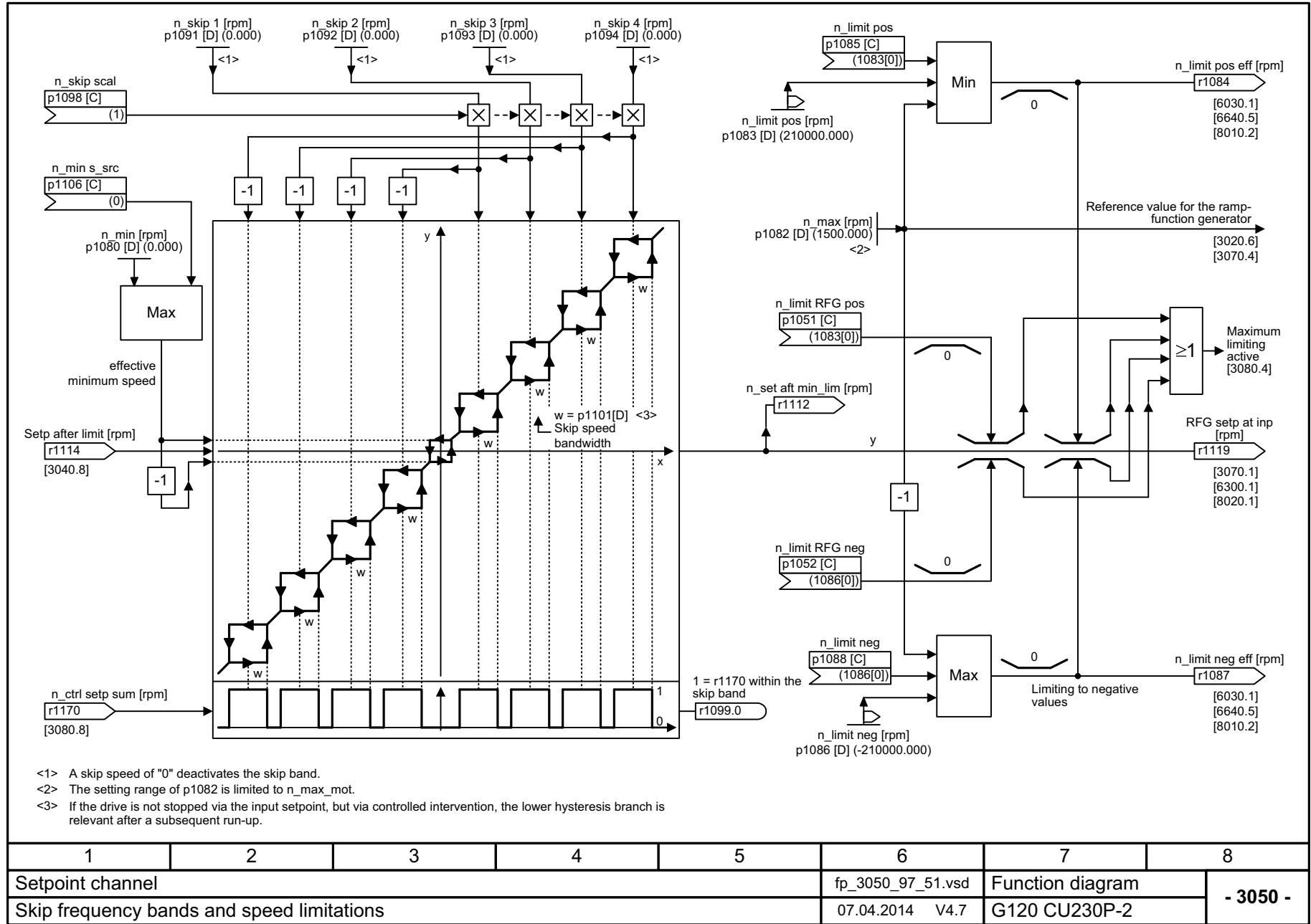
图 3-67 3050 - 跳转频带和转速限制
