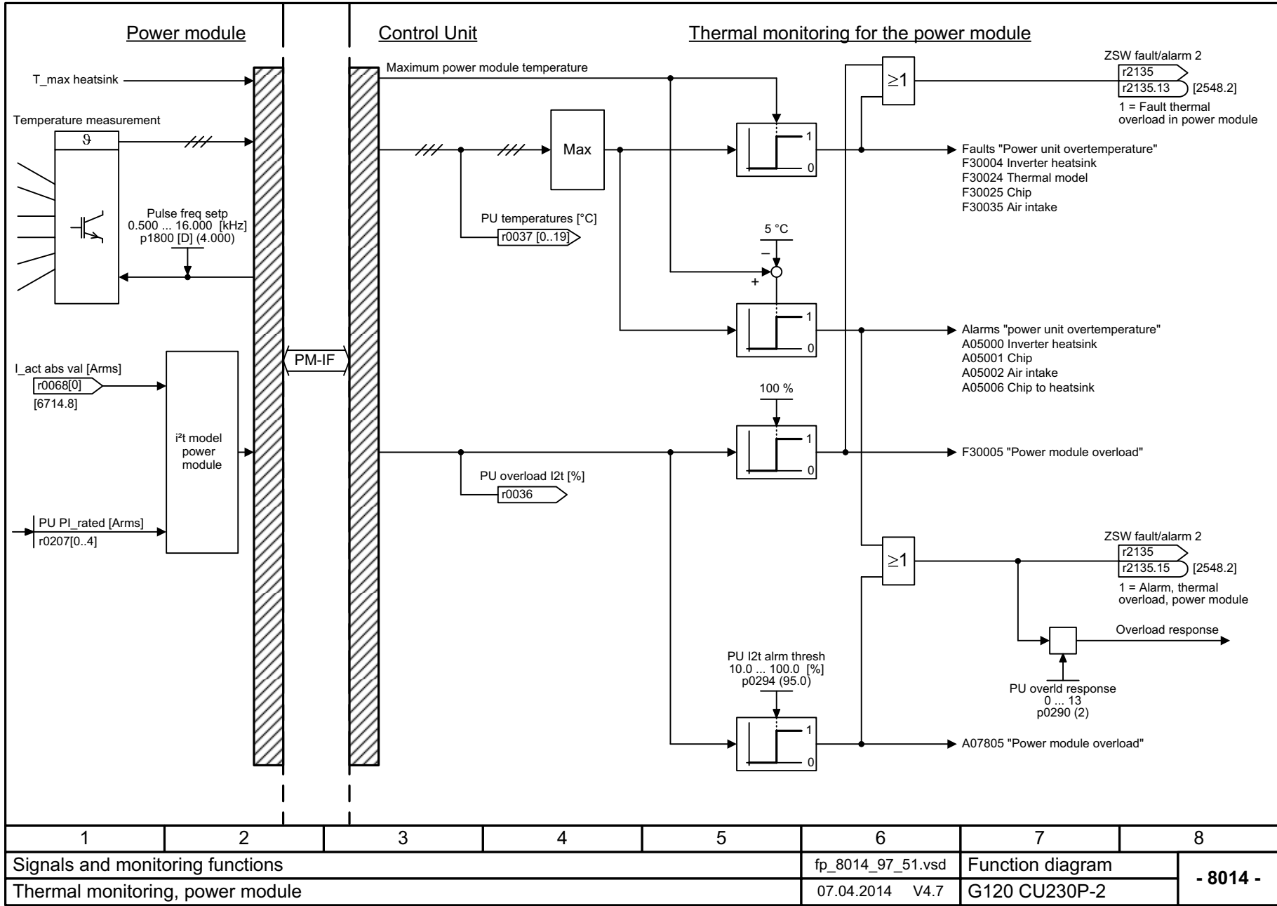
图 3-129 8014 - 功率单元热负荷监控
