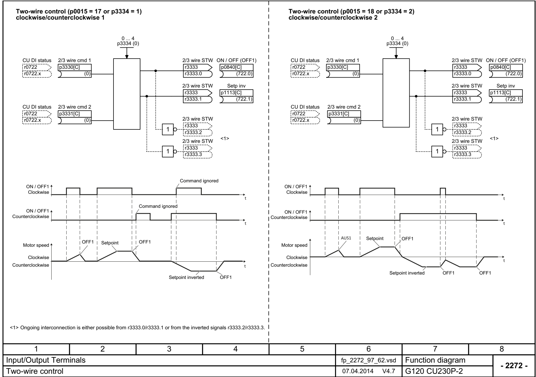
图 3-13 2272 - 双线制控制
