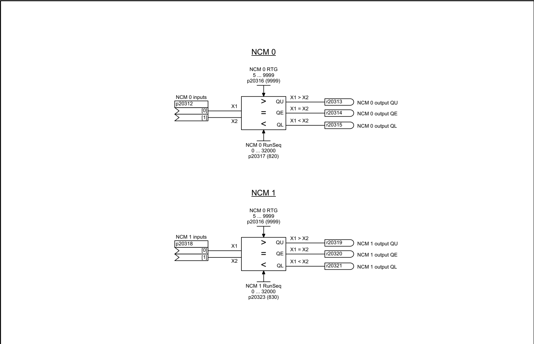
图 3-108 7225 - NCM (数字比较器)
