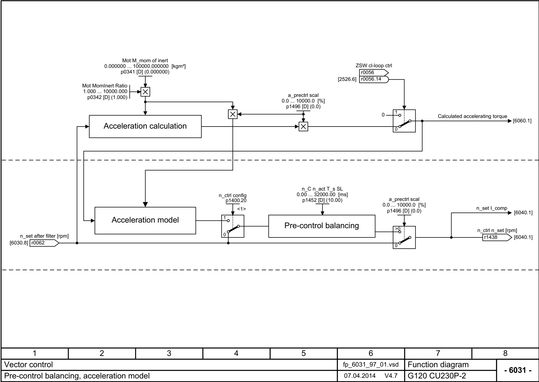
图 3-72 6031 - 前馈对称性, 加速度模型
