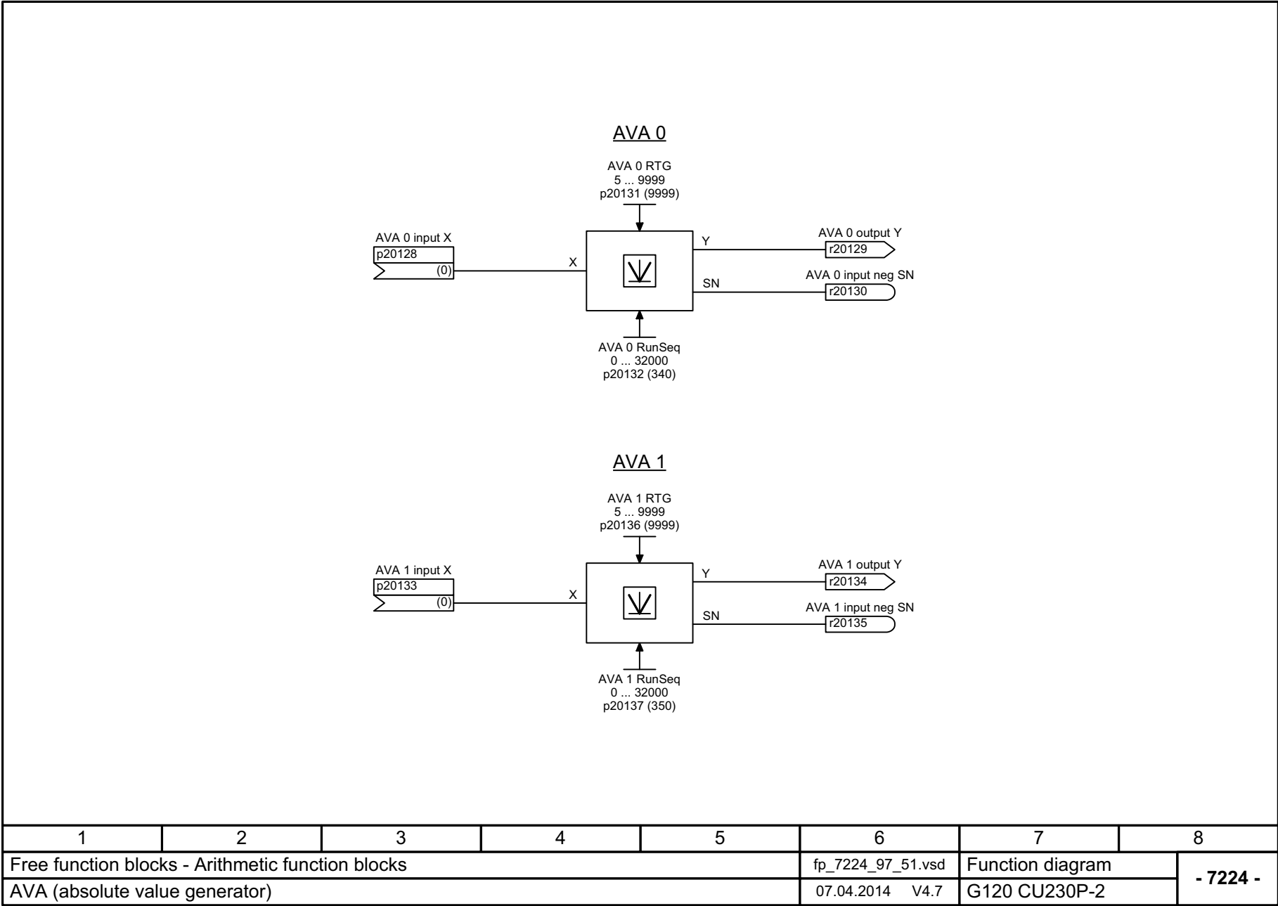
图 3-107 7224 - AVA (绝对值计算器)
