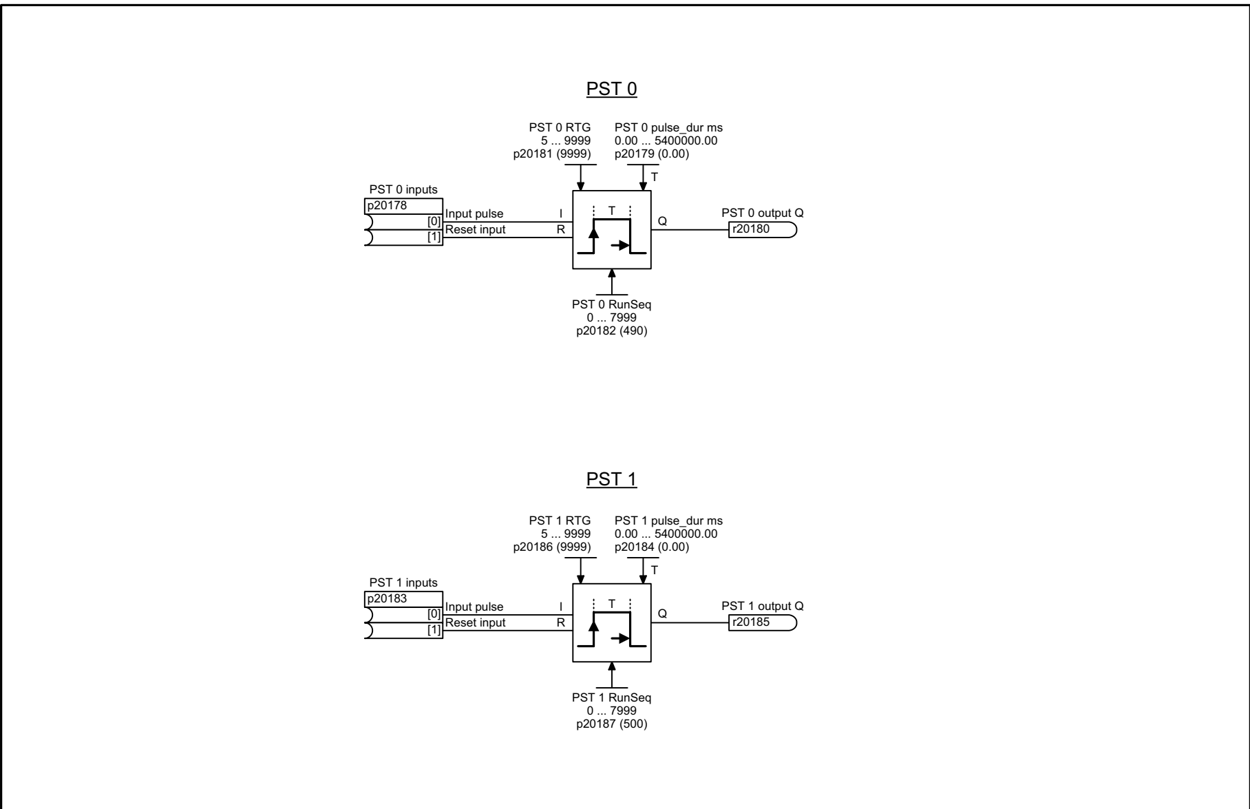
7234 - PST (脉冲延长器)
