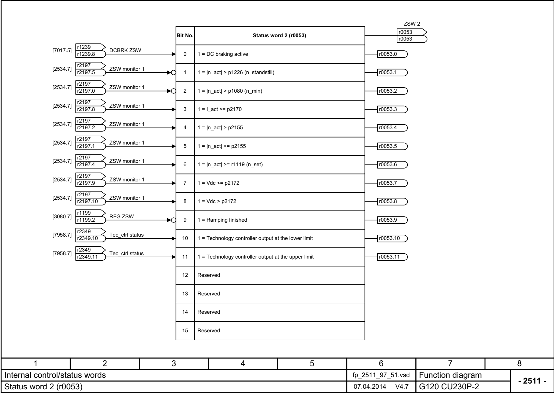
图 3-48 2511 - 状态字 2 (r0053)
