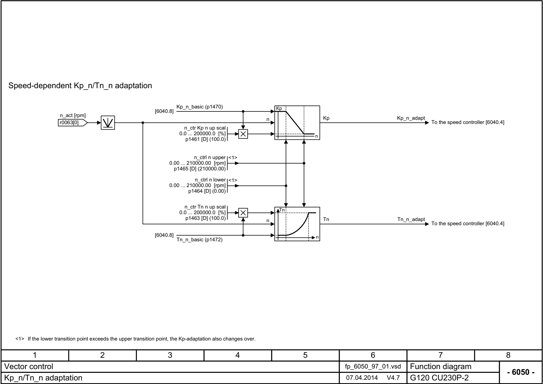
图 3-74 6050 - Kp_n-/Tn_n 适配
