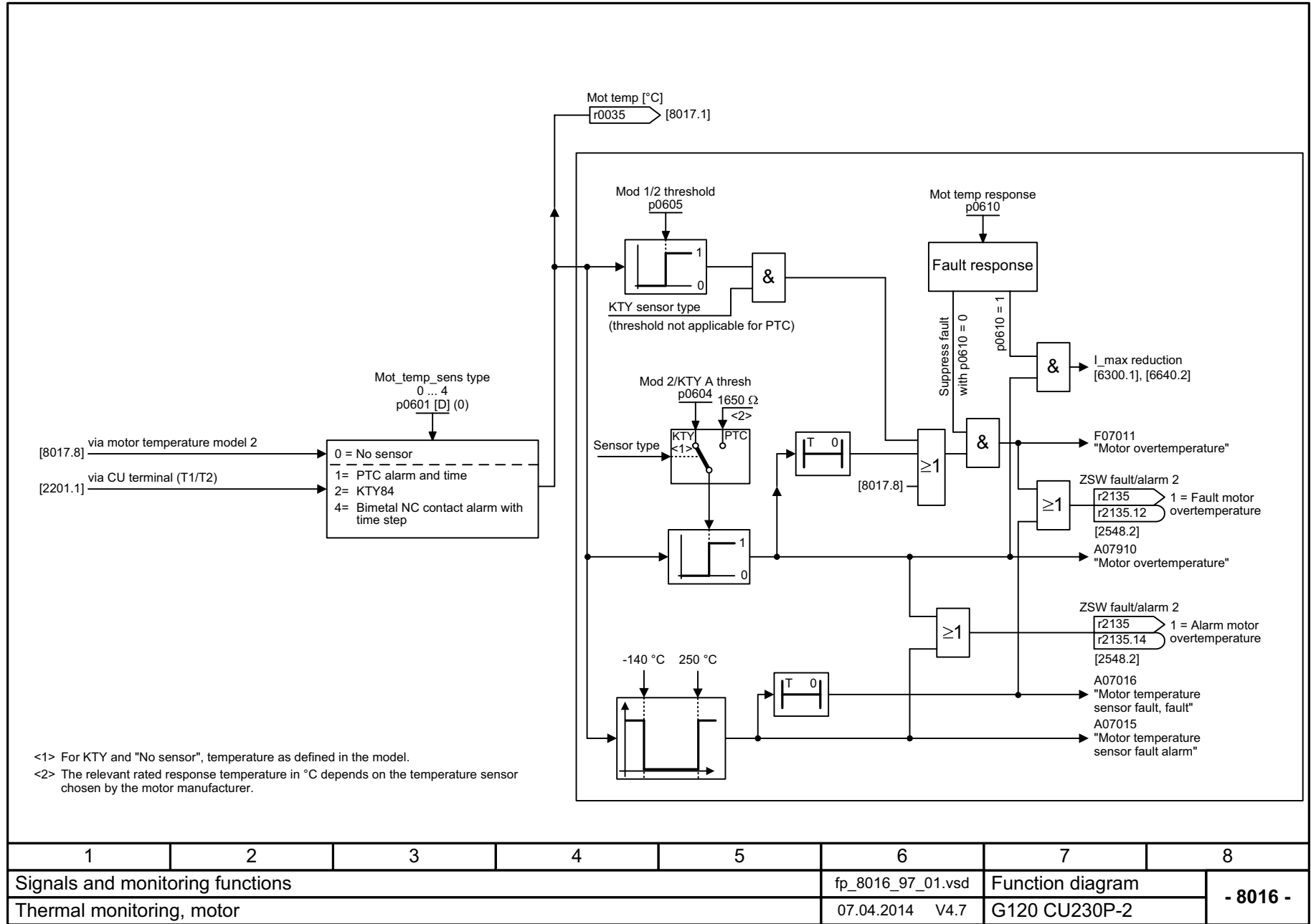
图 3-130 8016 - 电机热负荷监控
