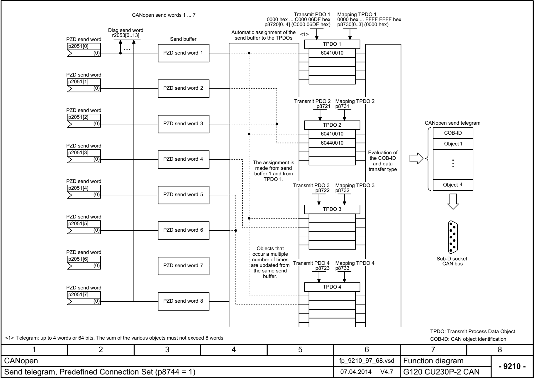
图 3-35 9210 - 预定义连接组发送电文 (p8744 = 1)
