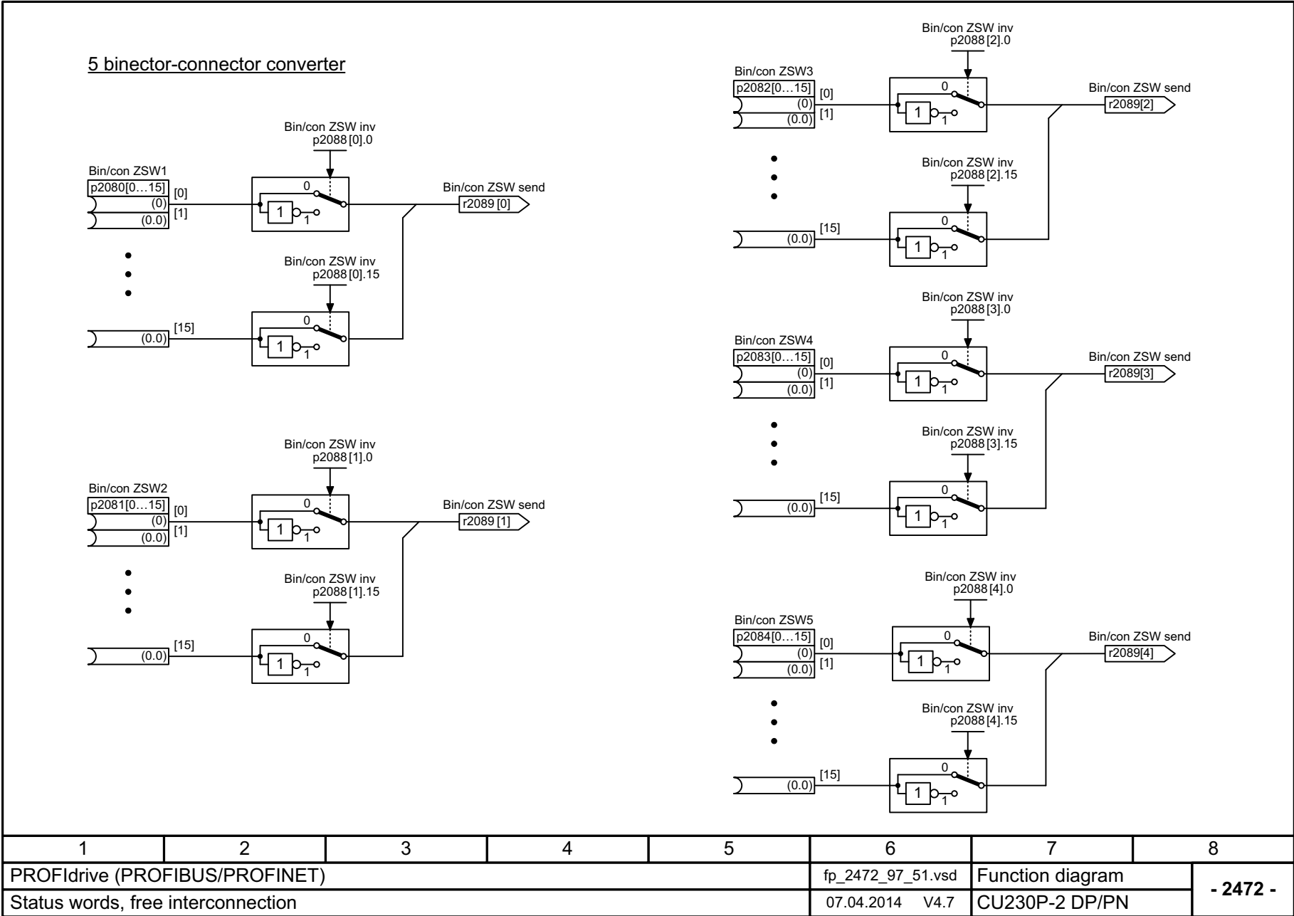
图 3-31 2472 - 自由互联状态字
