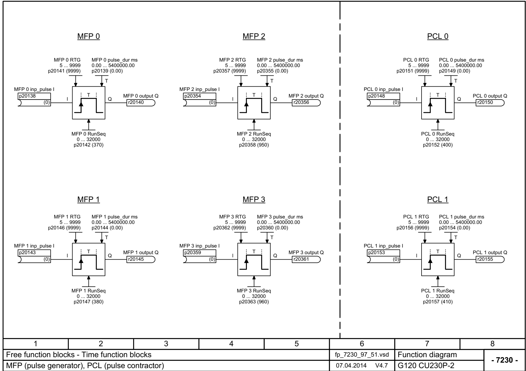
图 3-110 7230 - MFP (脉冲发生器), PCL (脉冲缩短器)
