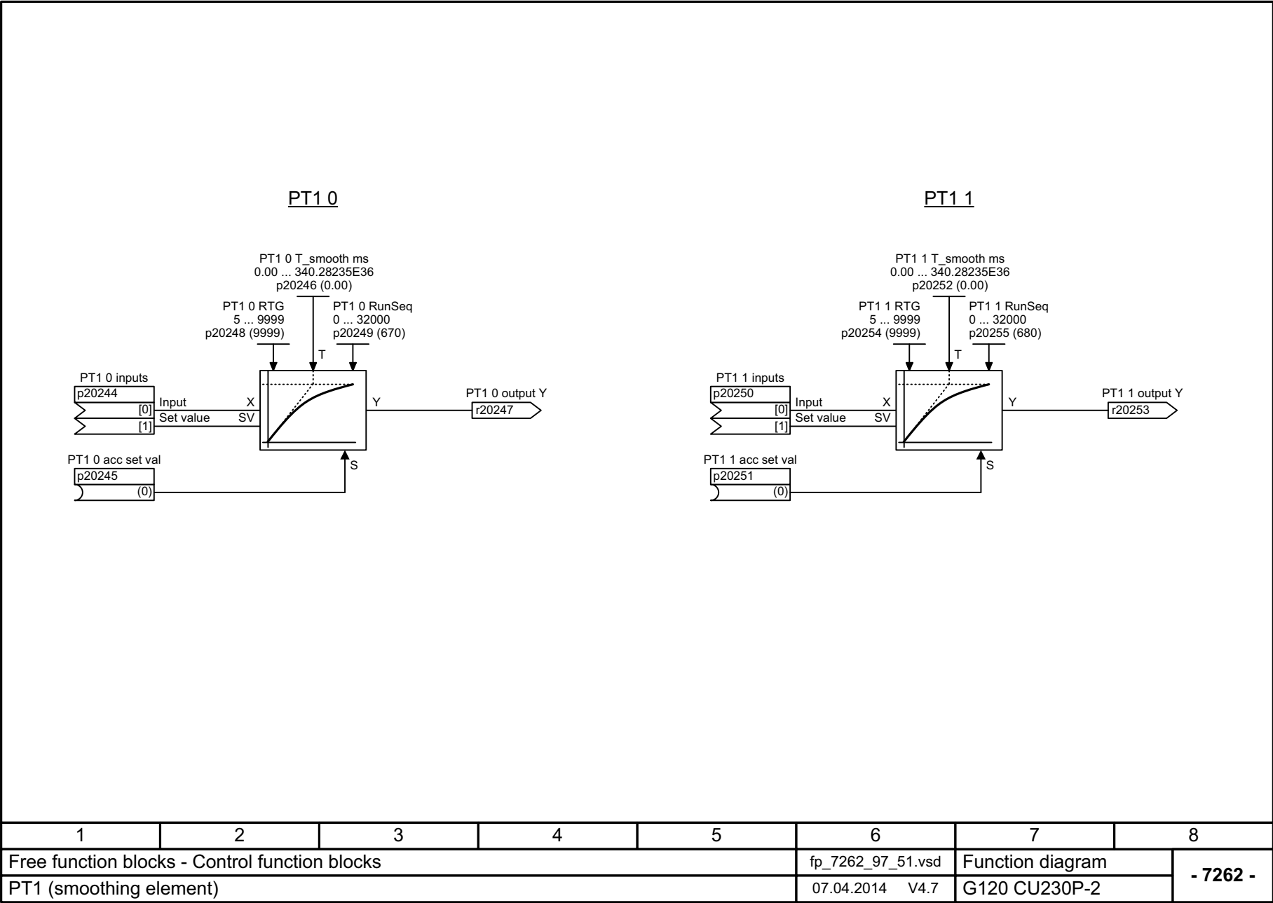
图 3-117 7262 - PT1 (平滑元件)
