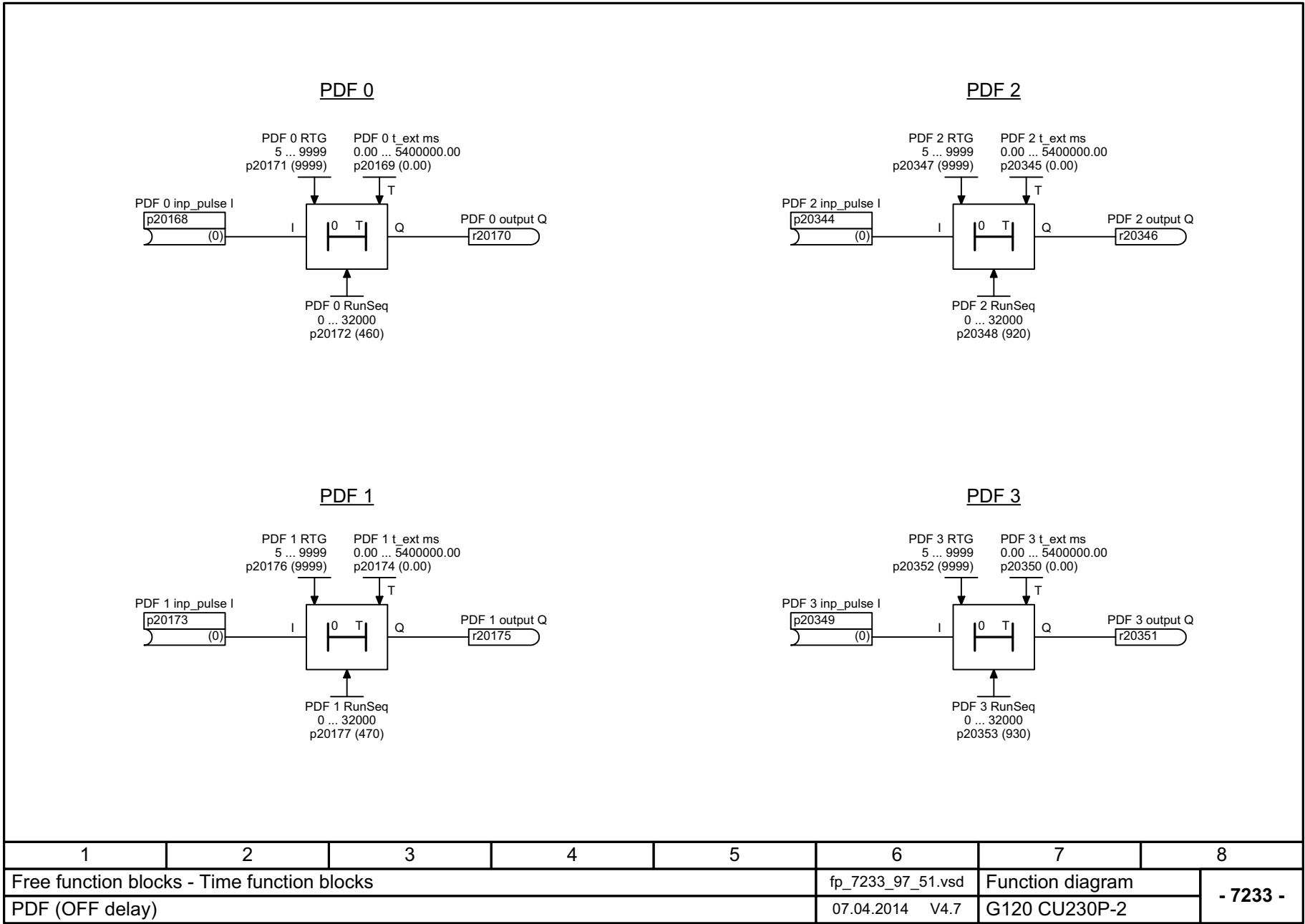
图 3-112 7233 - PDF (关闭延迟)
