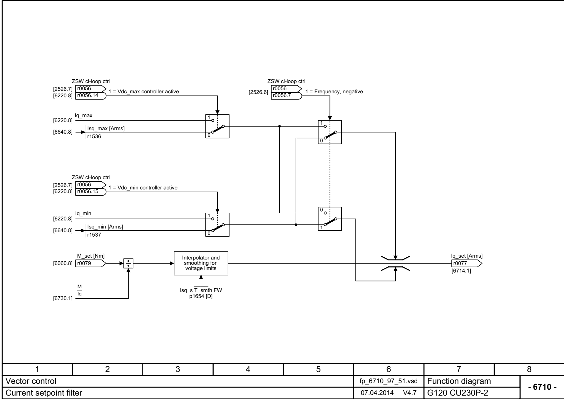
图 3-86 6710 - 电流设定值滤波器
