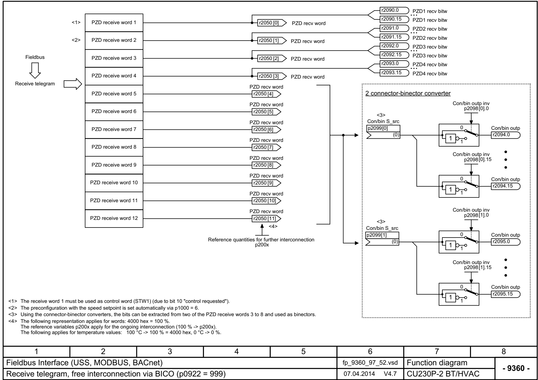
图 3-41 9360 - 通过 BICO 自由互连接收报文 (p0922 = 999)
