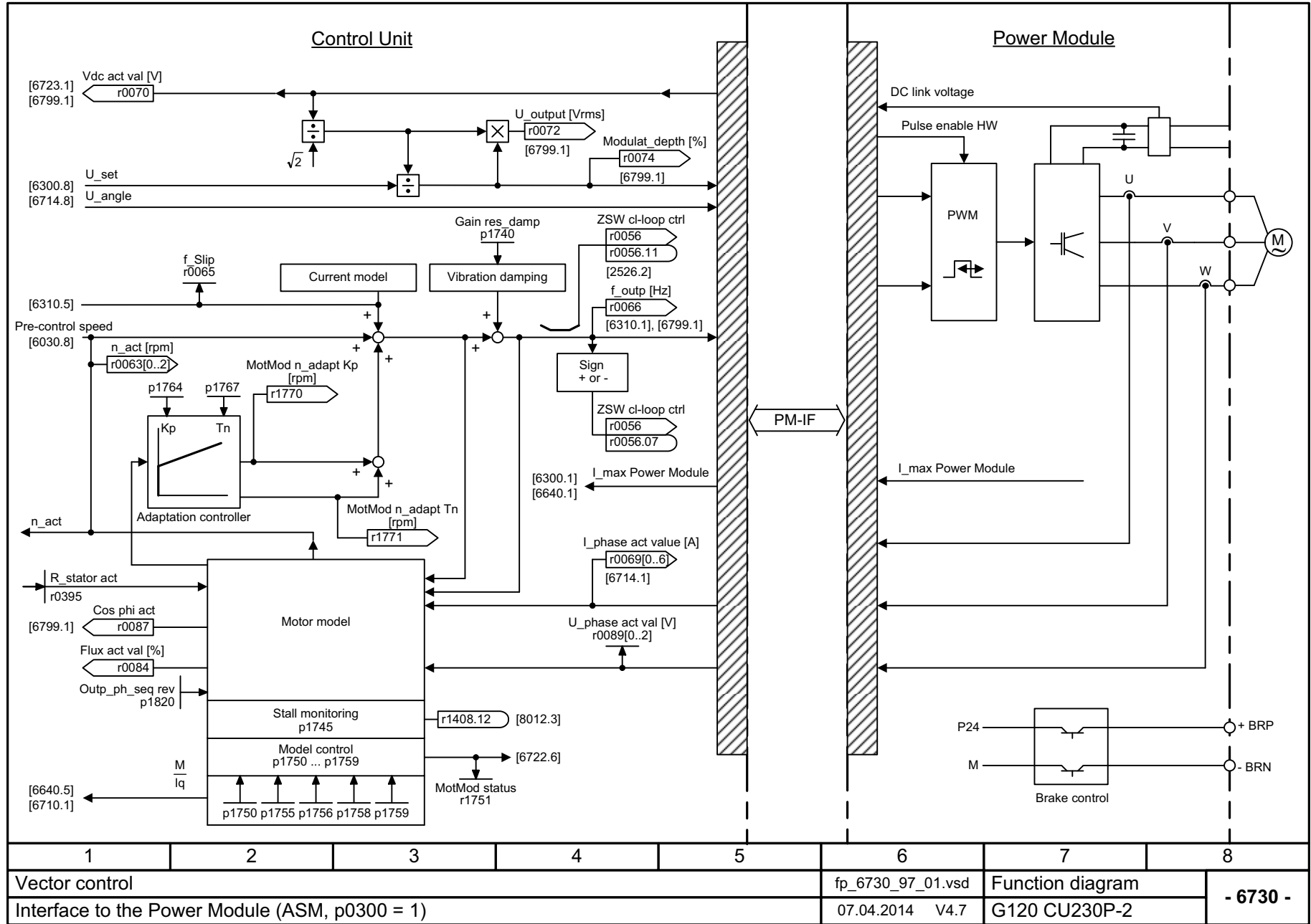
图 3-90 6730 - 和功率模块的接口 (ASM, p0300 = 1)
