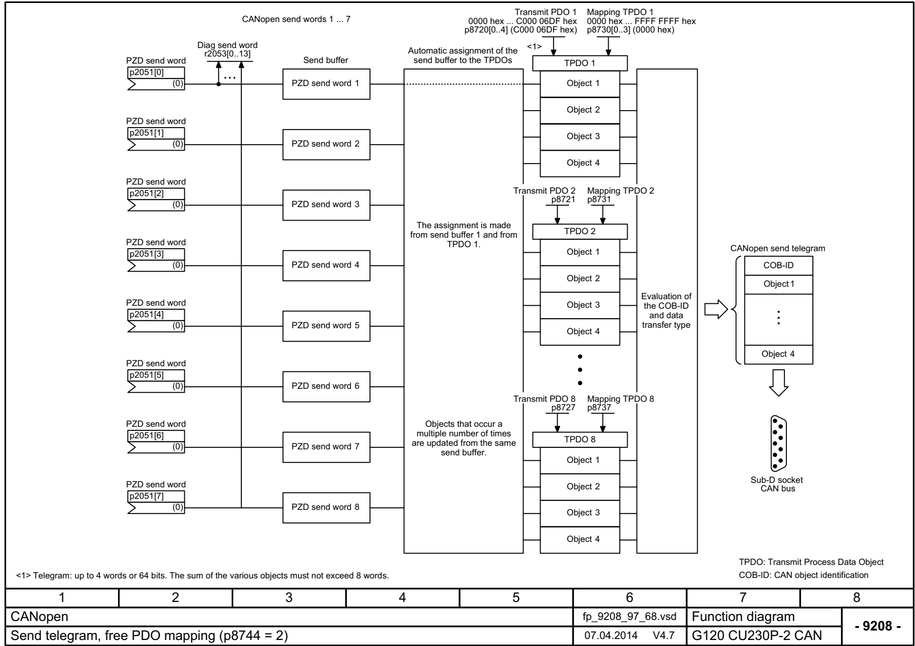
图 3-34 9208 - 由 PDO 映射发送电文 (p8744 = 2)
