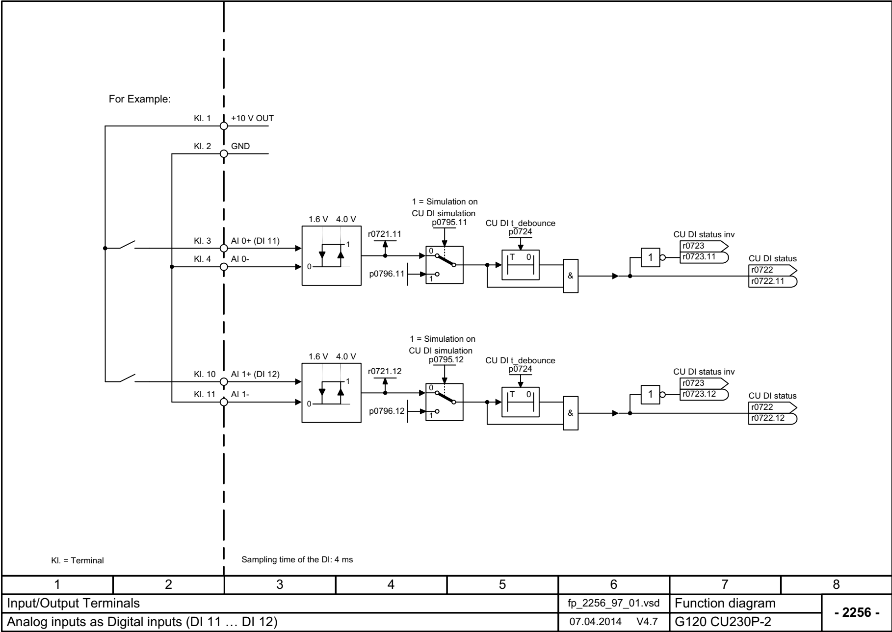
图 3-10 2256 - 模拟量输入用作数字量输入 (DI 11 ... DI 12)
