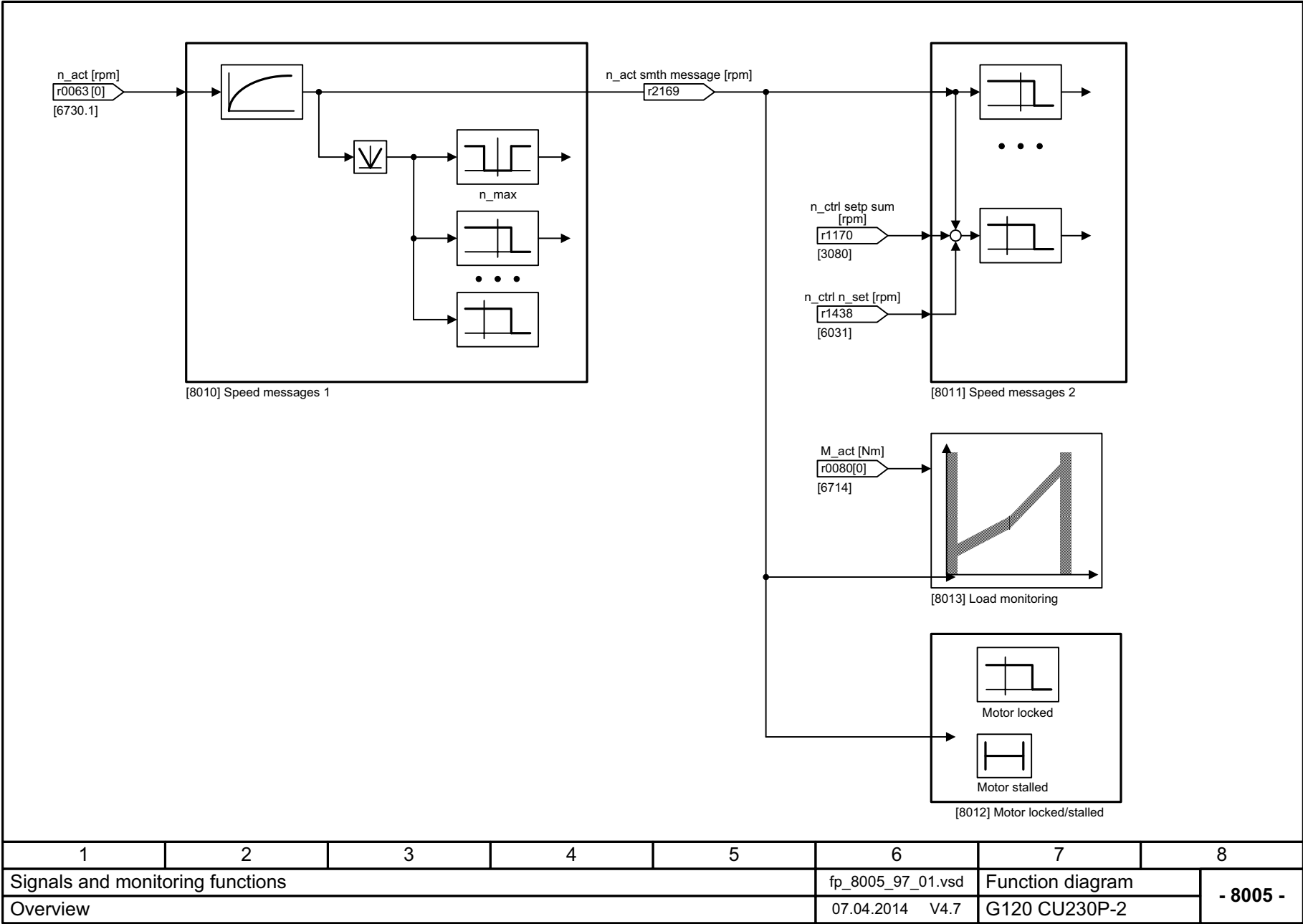
图 3-124 8005 - 一览
