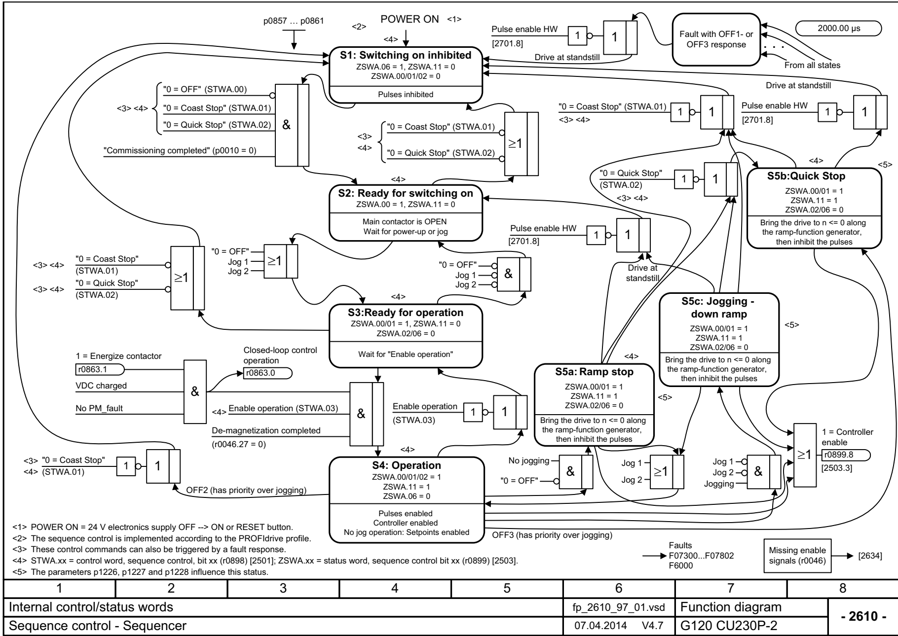
图 3-59 2610 - 顺序控制 - 控制器
