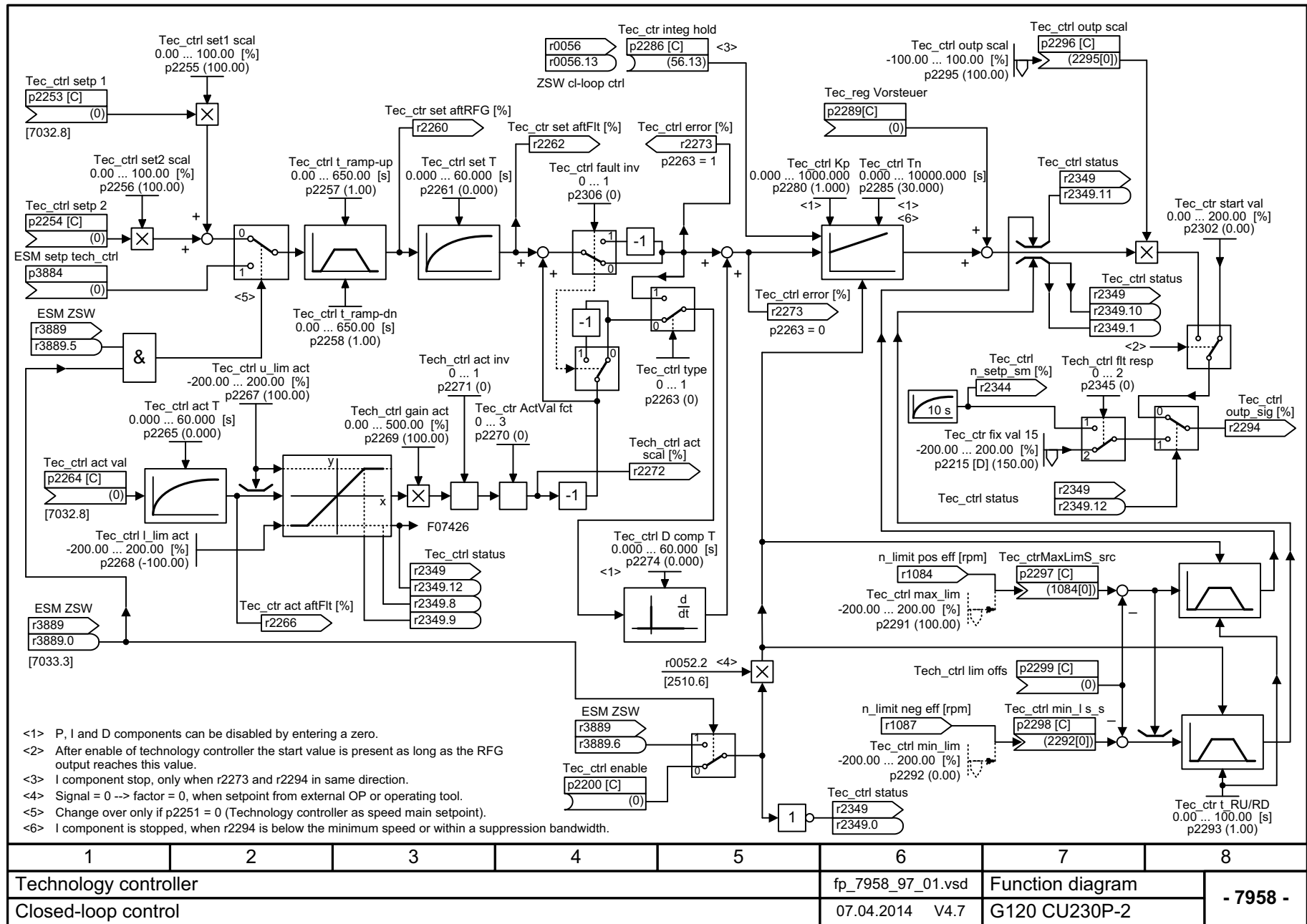
图 3-123 7958 - 闭环控制
