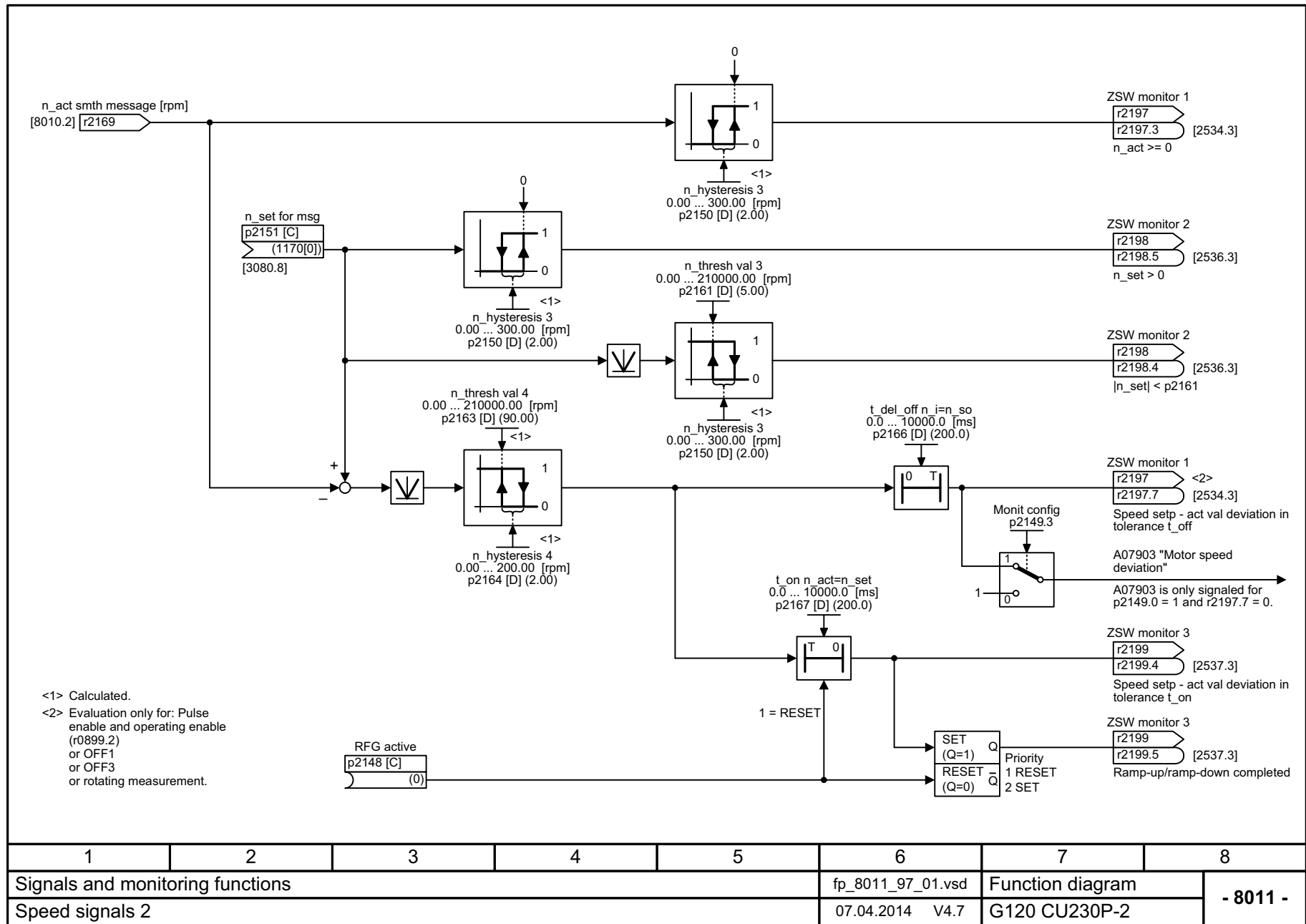
图 3-126 8011 - 转速信息 2
