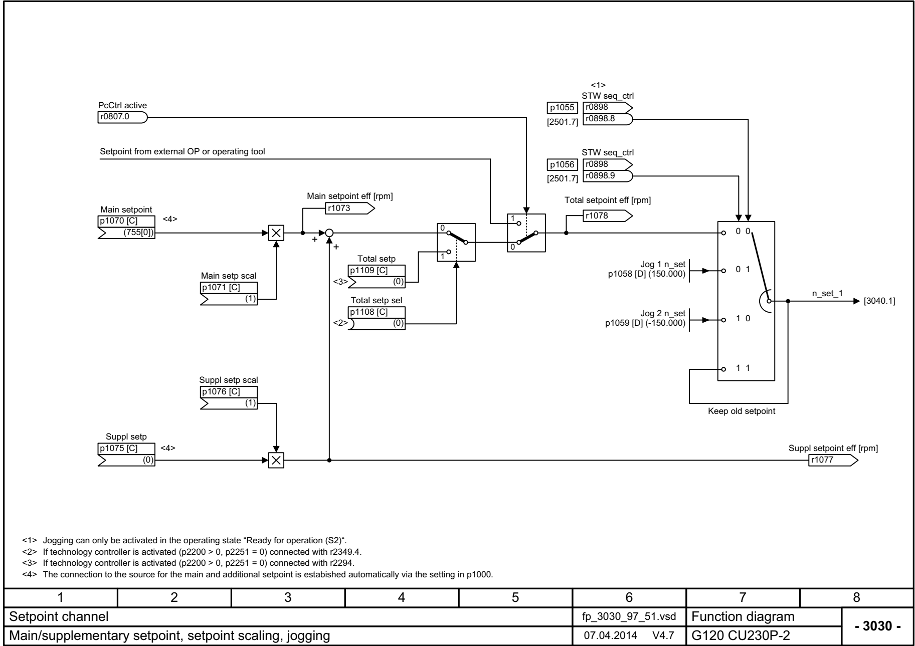
图 3-65 3030 - 主设定值 / 附加设定值, 设定值比例缩放, 点动
