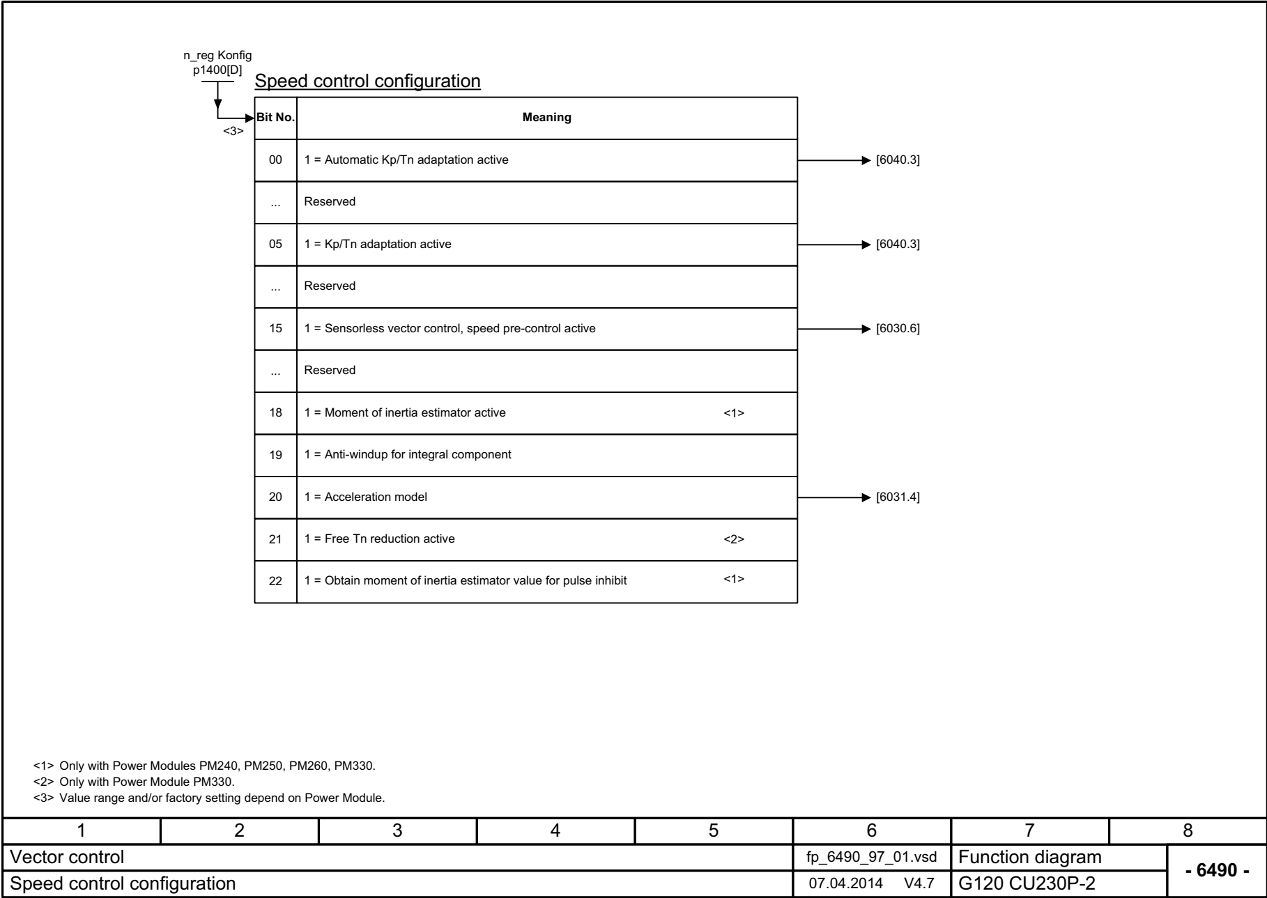
图 3-81 6490 - 转速控制配置
