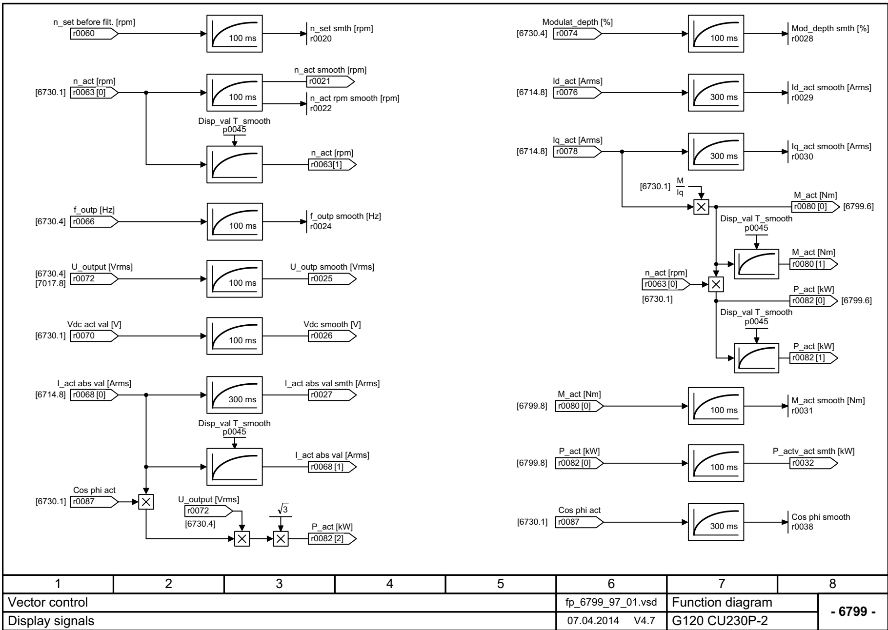
图 3-92 6799 - 显示信号
