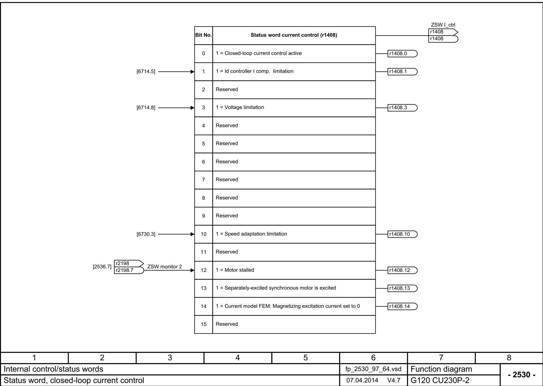
图 3-53 2530 - 电流控制状态字
