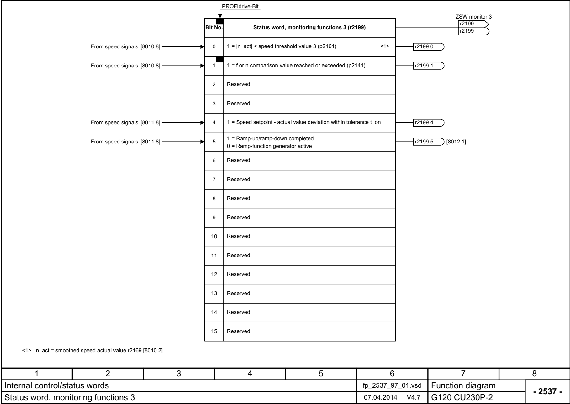
图 3-56 2537 - 监控状态字 3
