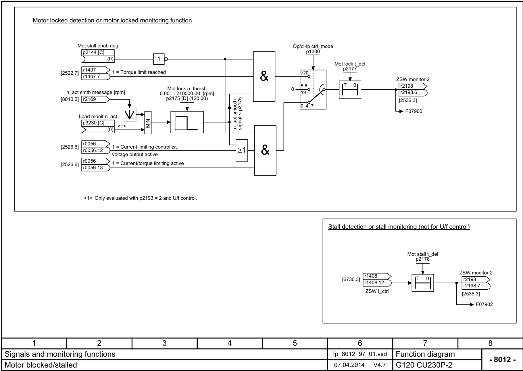
图 3-127 8012 - 转矩信息, 电机堵转 / 失步
