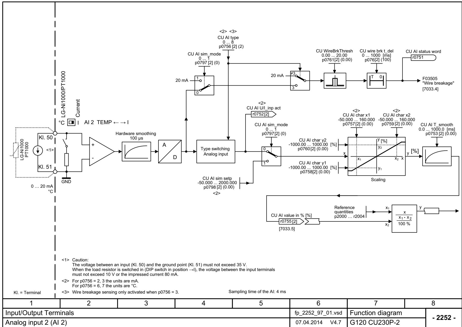
图 3-9 2252 - 模拟输入端 2 (AI 2)
