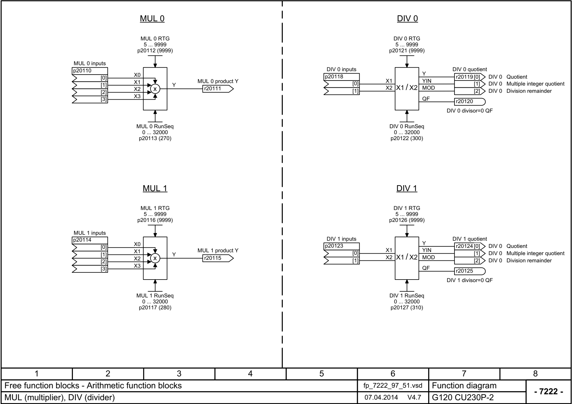
图 3-106 7222 - MUL (乘法器), DIV (除法器)
