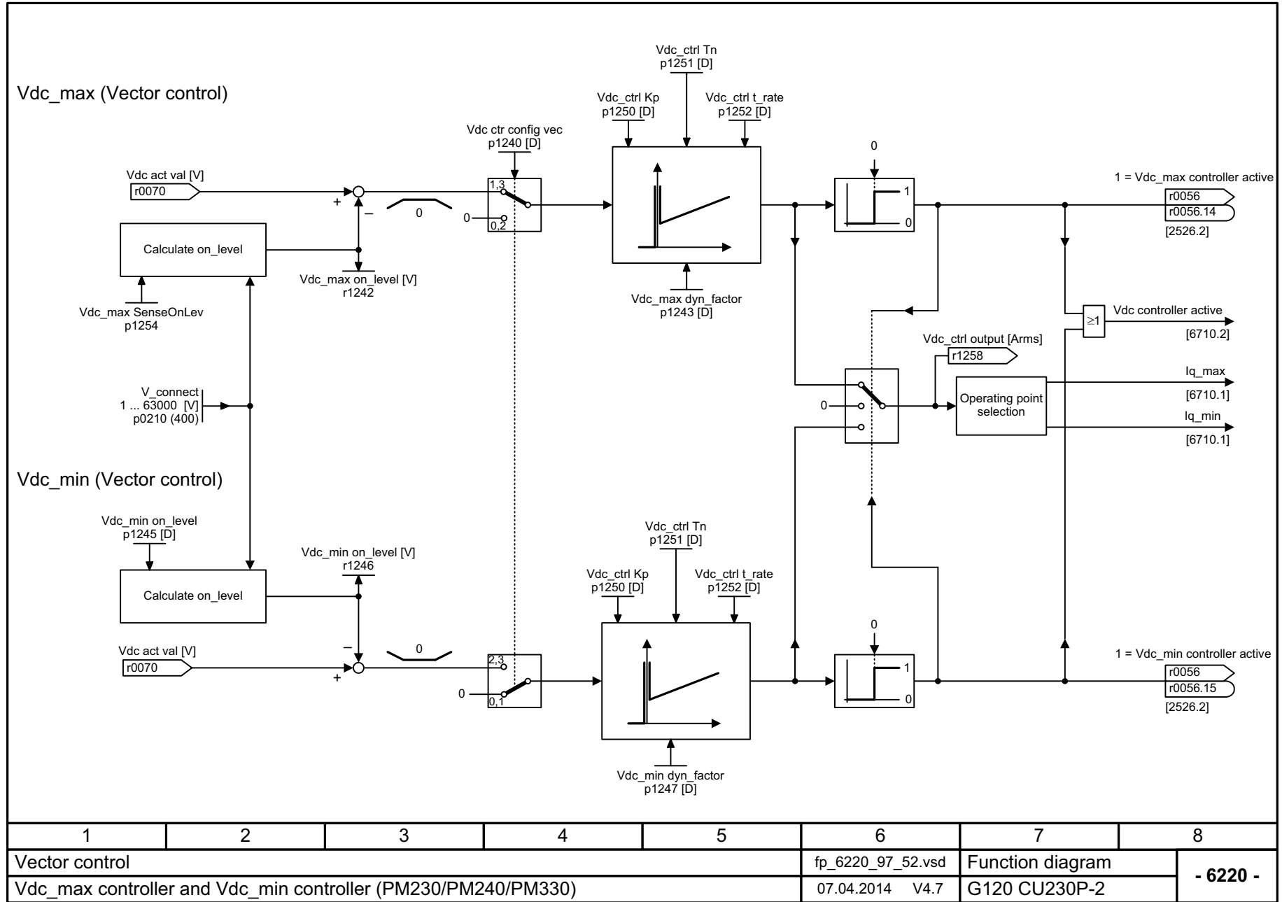
图 3-76 6220 - 直流母线电压控制器 (矢量控制、PM230/PM240/PM330)
