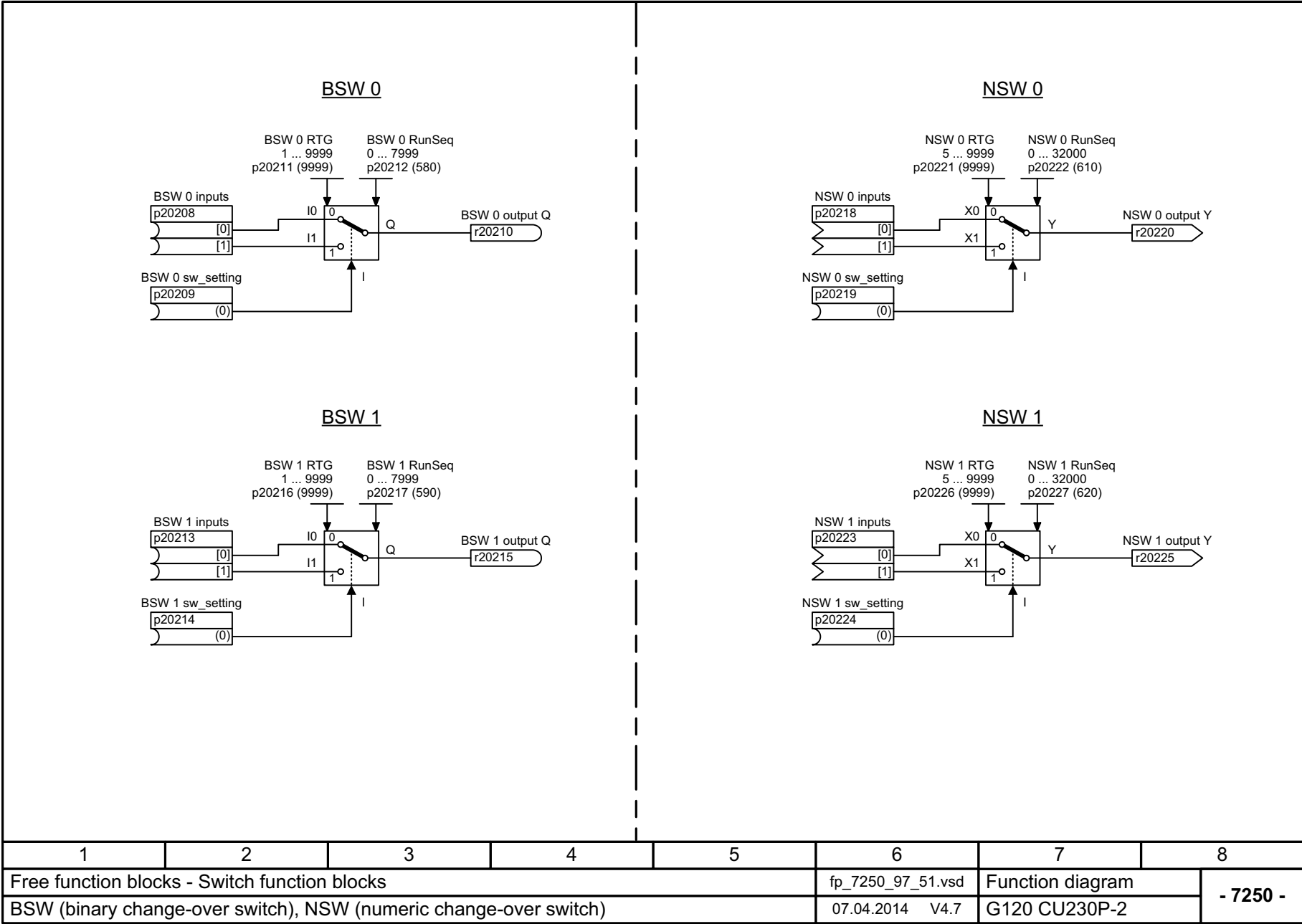
图 3-115 7250 - BSW (二进制转换器), NSW (数字转换器)
