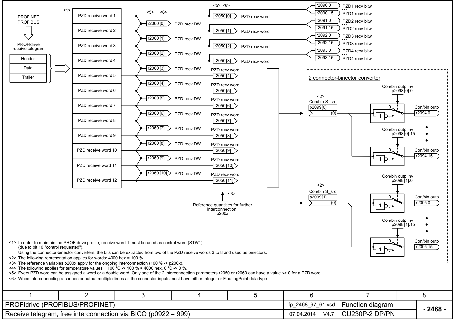
图 3-29 2468 - 通过 BICO 自由互接收报文 (p0922 = 999)
