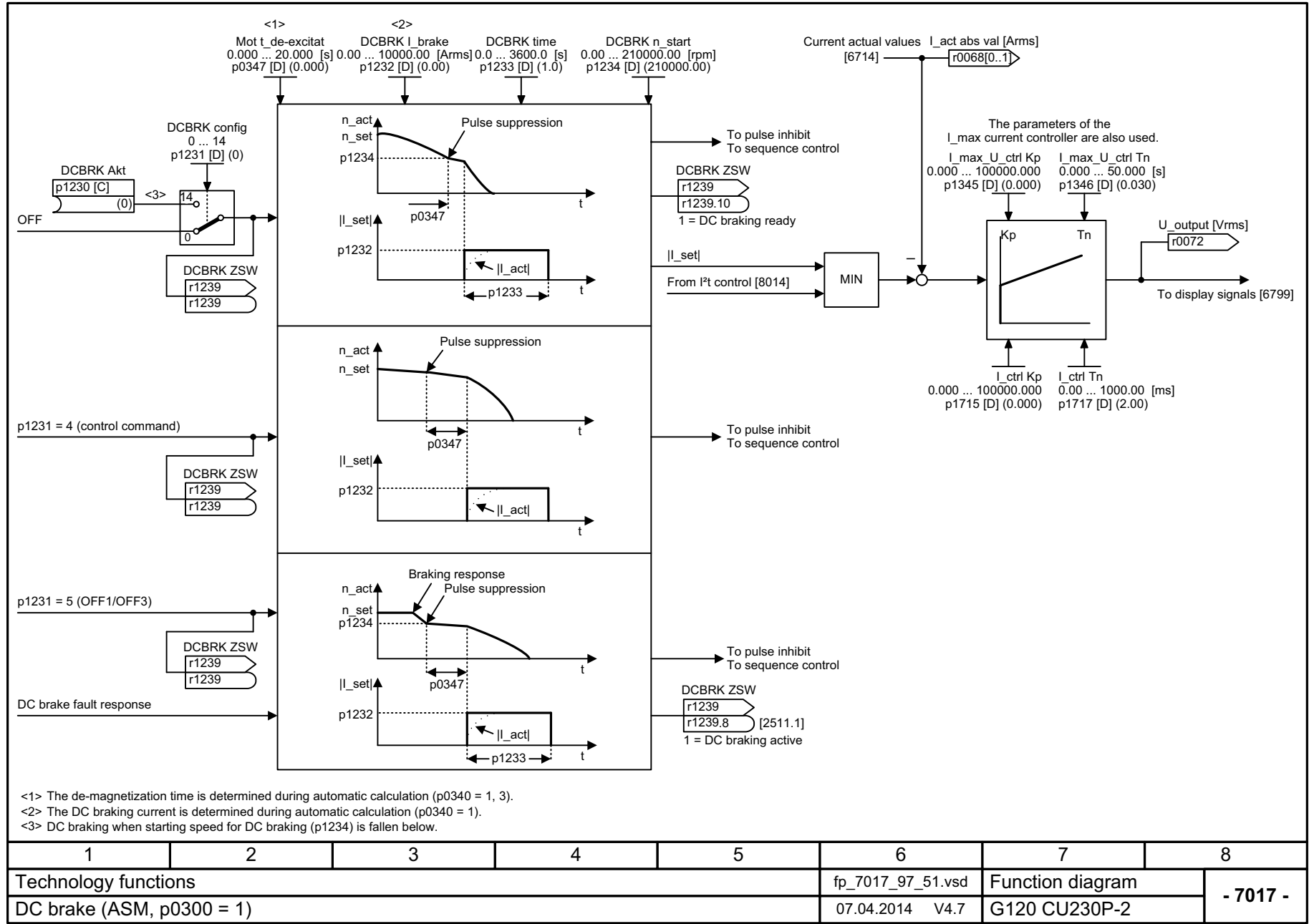
图 3-93 7017 - 直流制动 (p0300 = 1)
