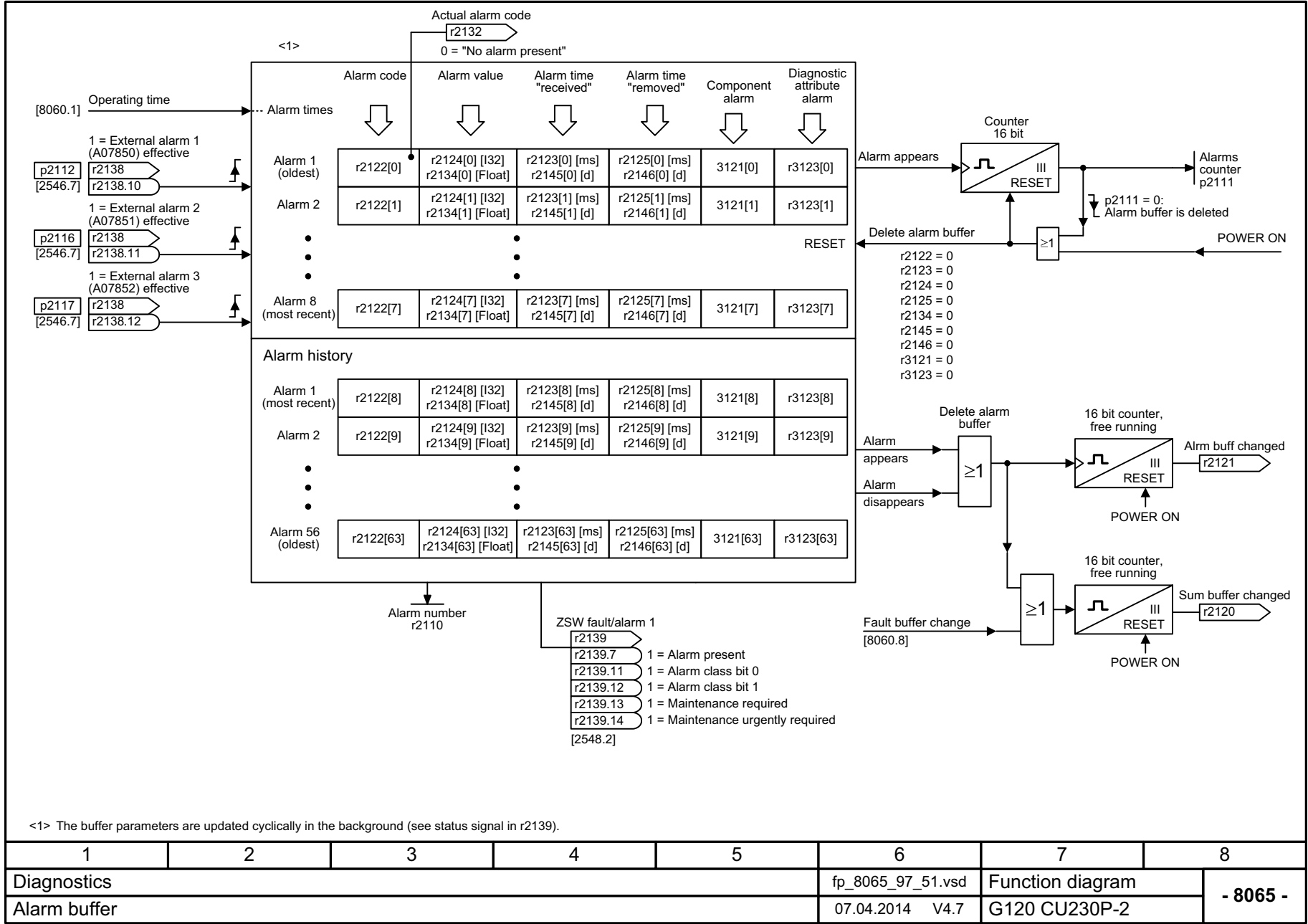
图 3-135 8065 - 报警缓冲器
