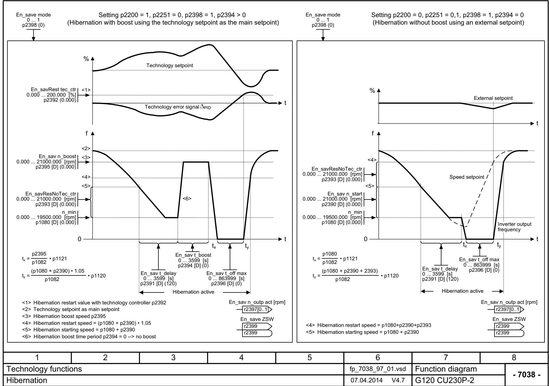
图 3-99 7038 - 节能模式
