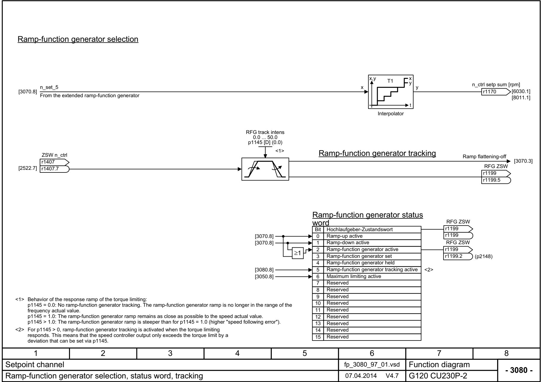
图 3-69 3080 - 斜坡函数发生器选择, 斜坡函数发生器状态字, 斜坡函数发生器跟踪
