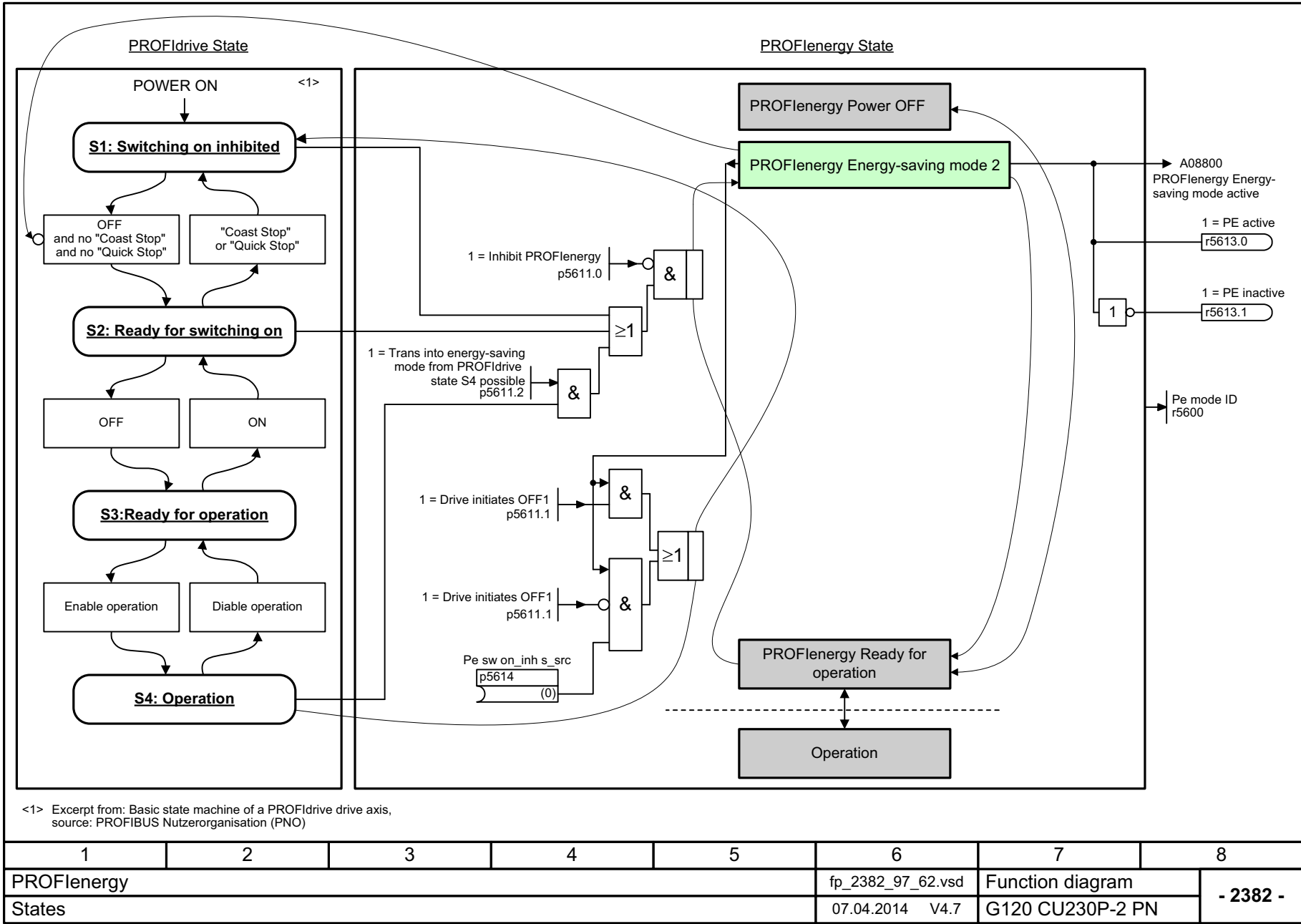
图 3-17 2382 - 状态
