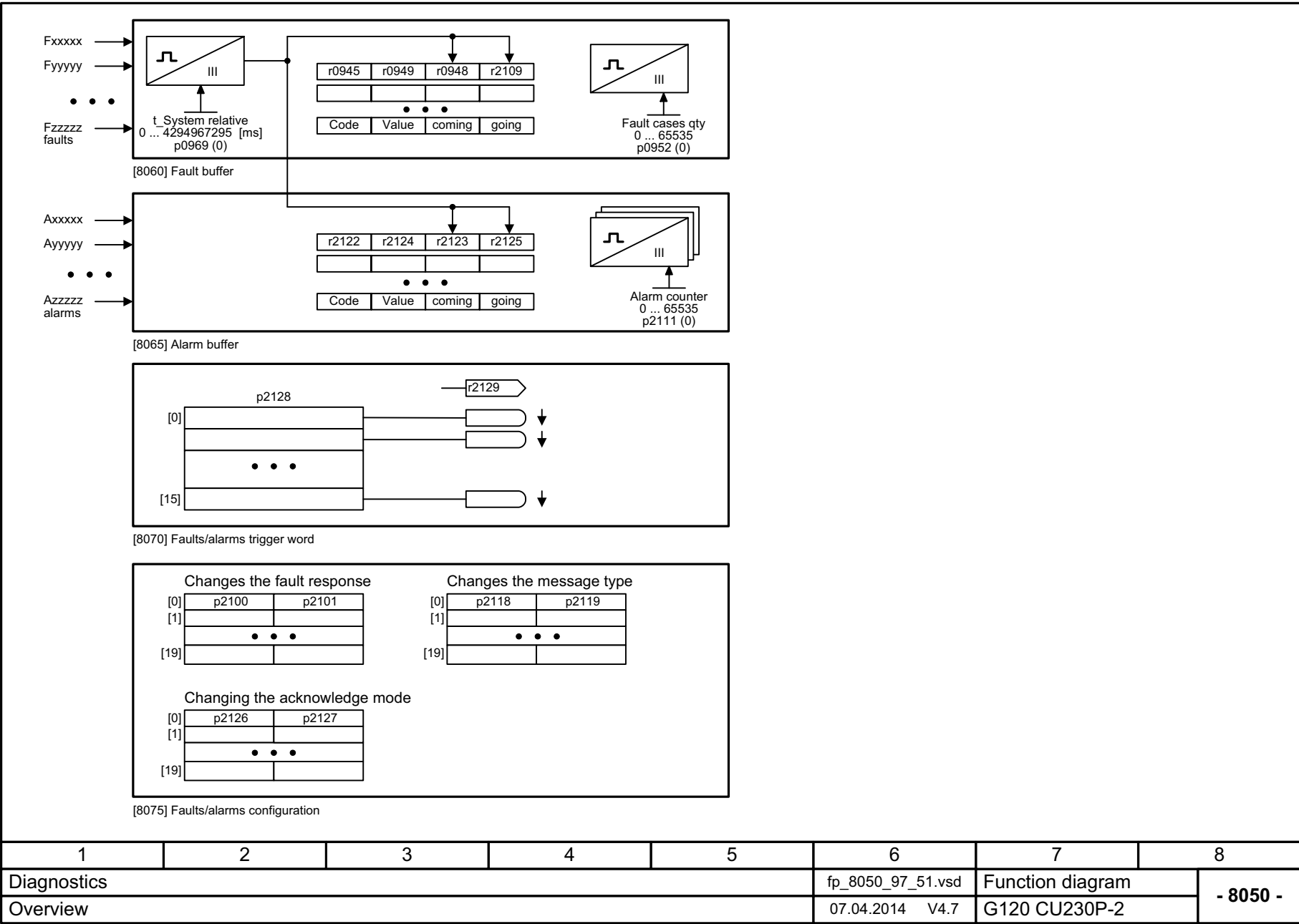
图 3-133 8050 - 一览
