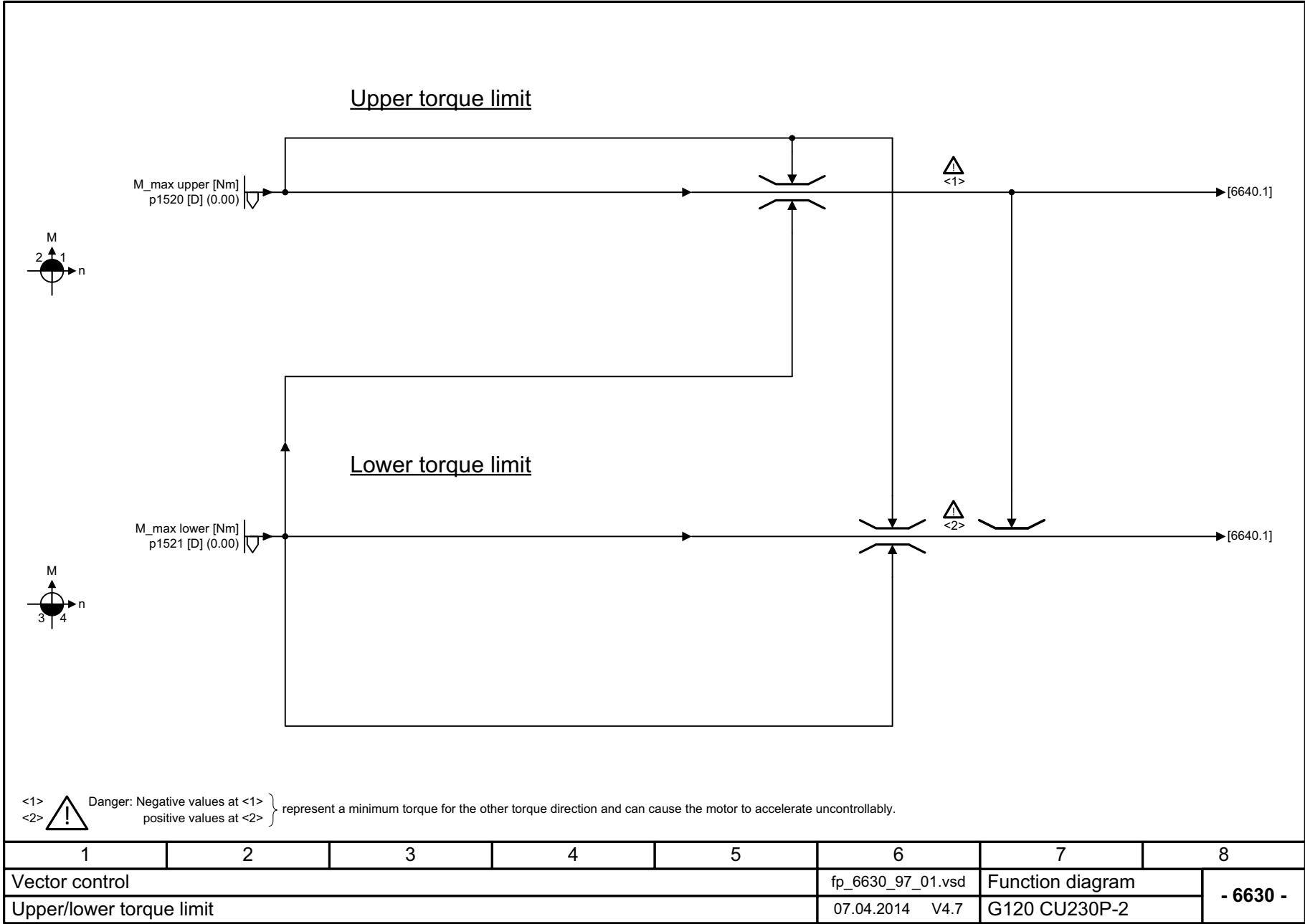
图 3-83 6630 - 转矩上限 / 转矩下限
