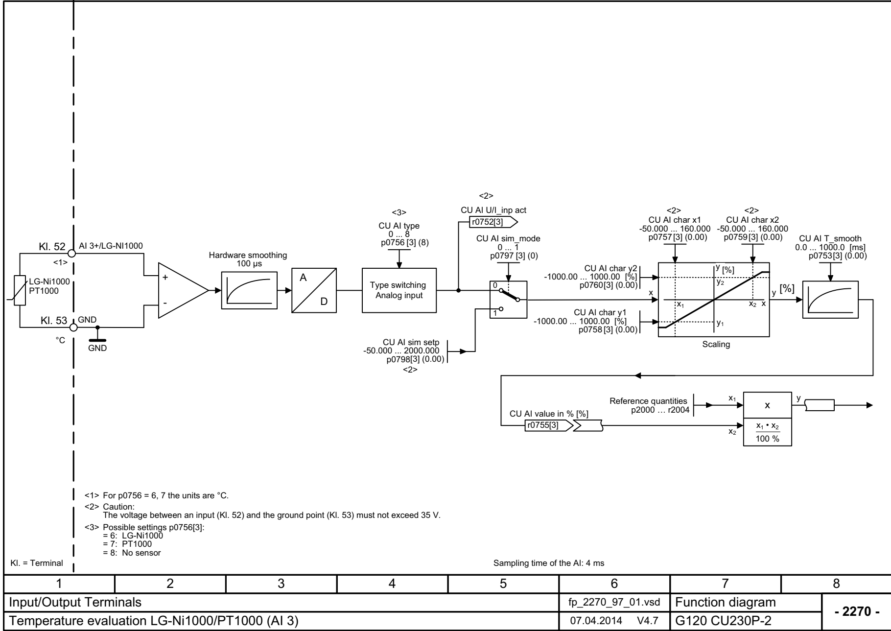
图 3-12 2270 - 温度检测 LG-Ni1000/PT1000 (AI 3)
