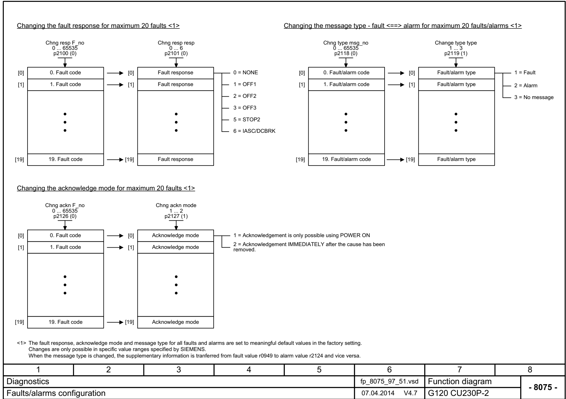
图 3-137 8075 - 故障 / 报警配置
