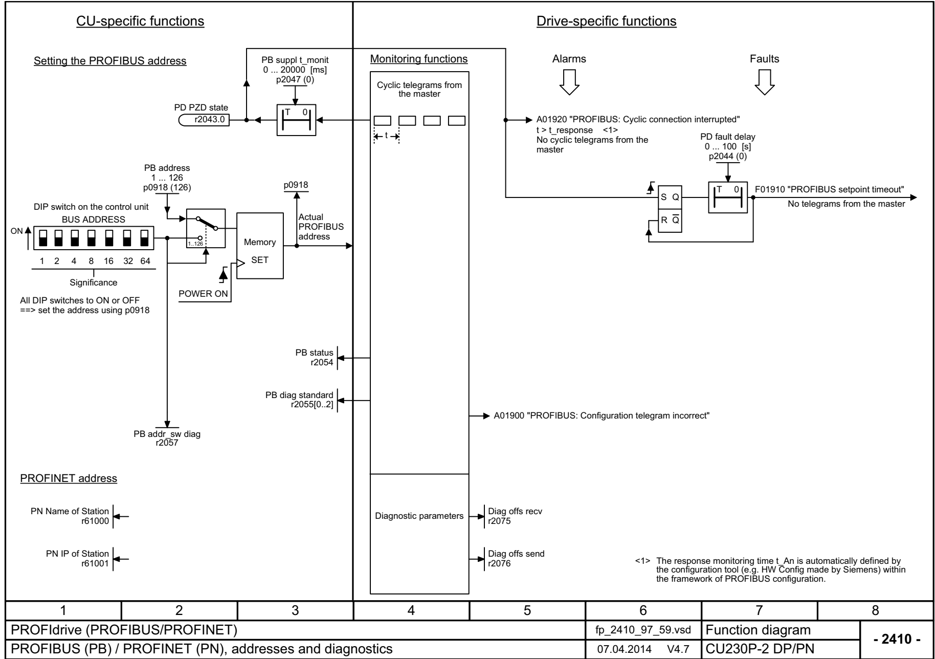
图 3-19 2410 - PROFIBUS (PB) / PROFINET (PN), 地址和诊断
