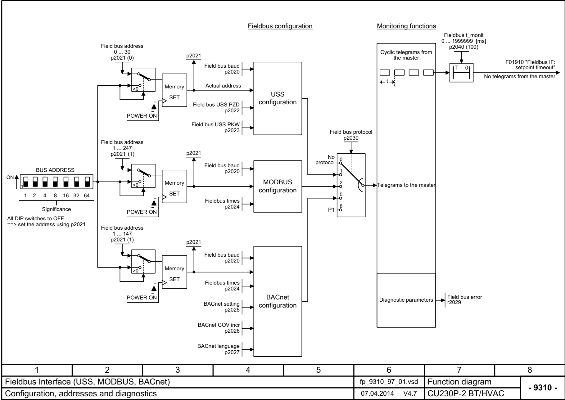
图 3-38 9310 - 配置，地址及诊断
