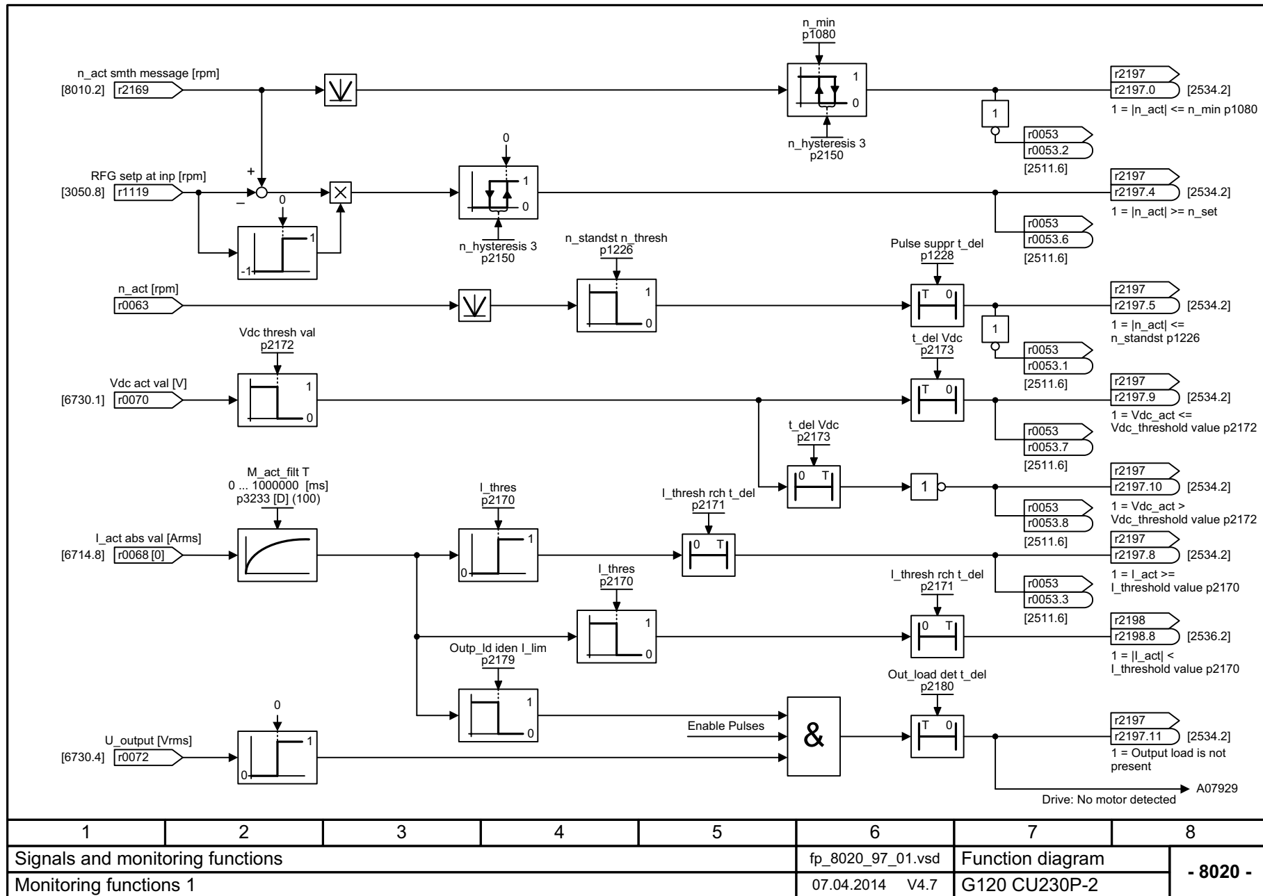
图 3-132 8020 - 监控功能 1
