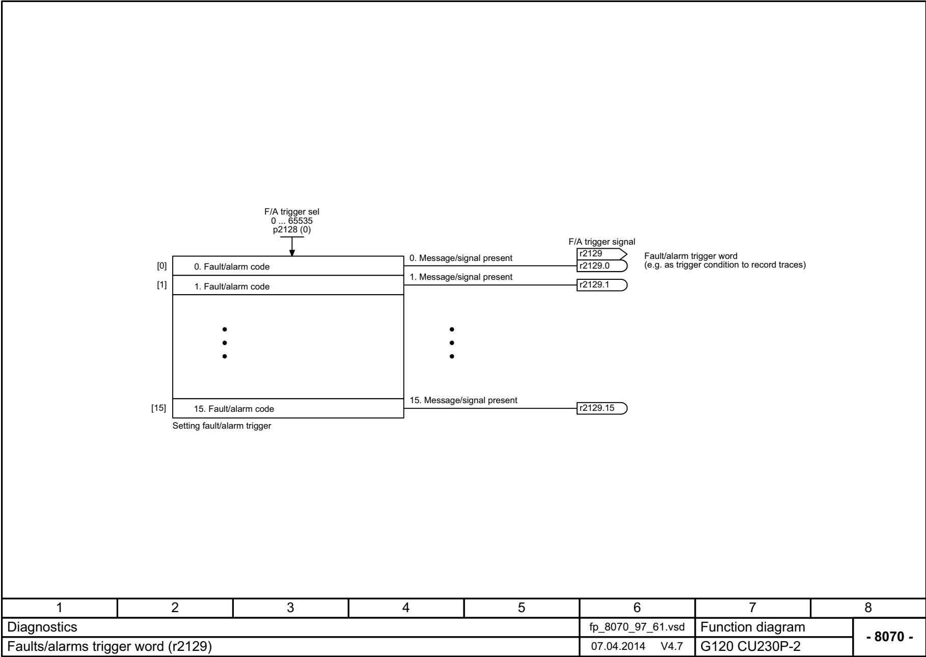
图 3-136 8070 - 故障 / 报警触发字 (r2129)
