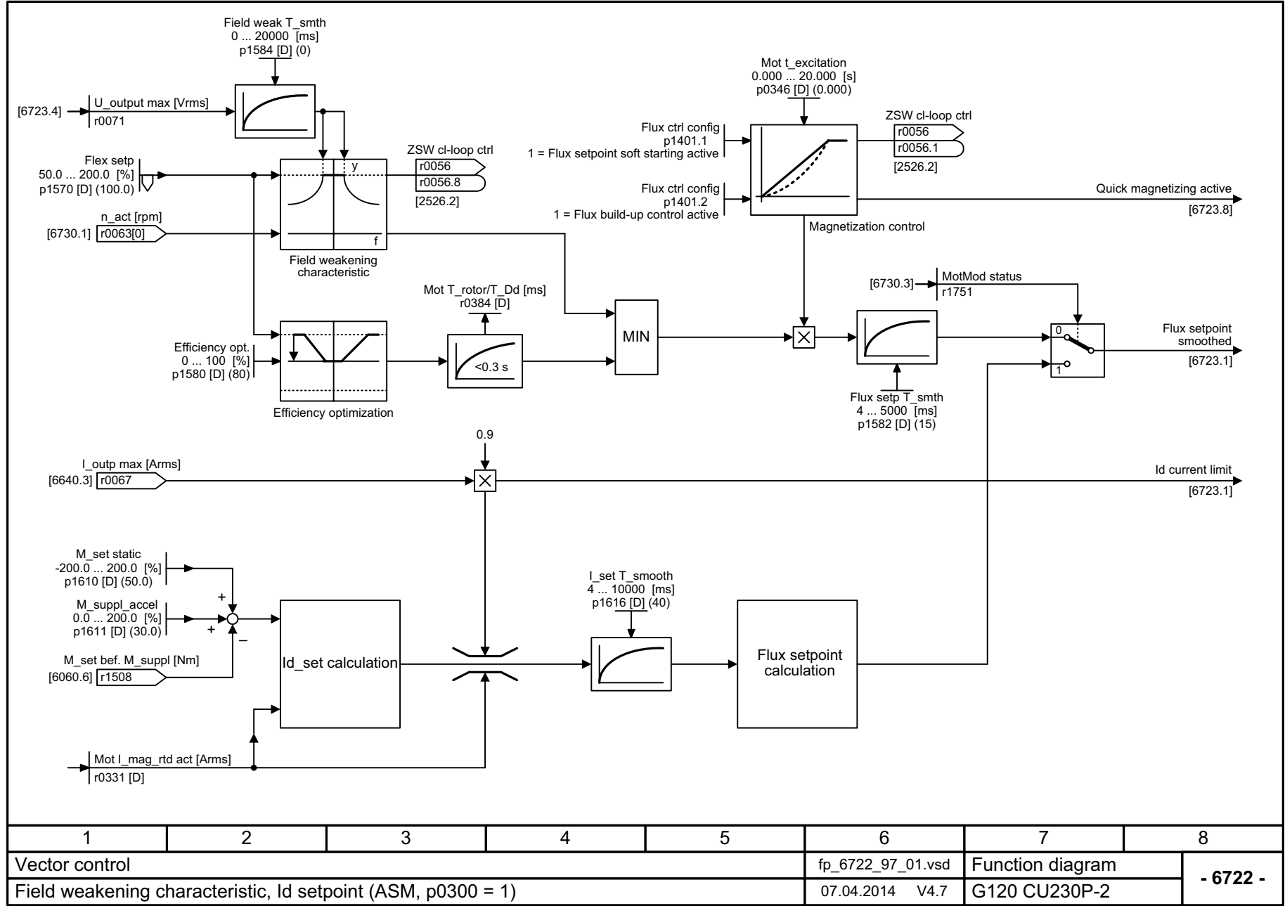
图 3-88 6722 - 弱磁特性曲线, Id 设定值 (ASM, p0300 = 1)
