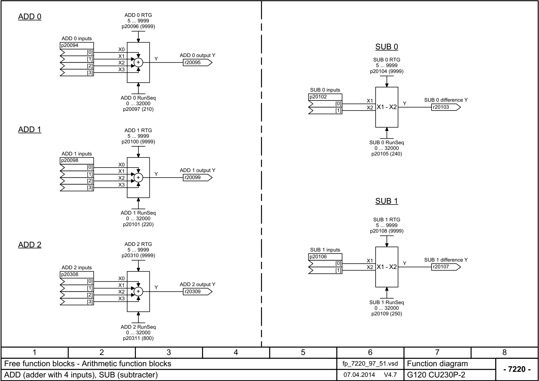
图 3-105 7220 - ADD (有 4 个输入的加法器), SUB (减法器)
