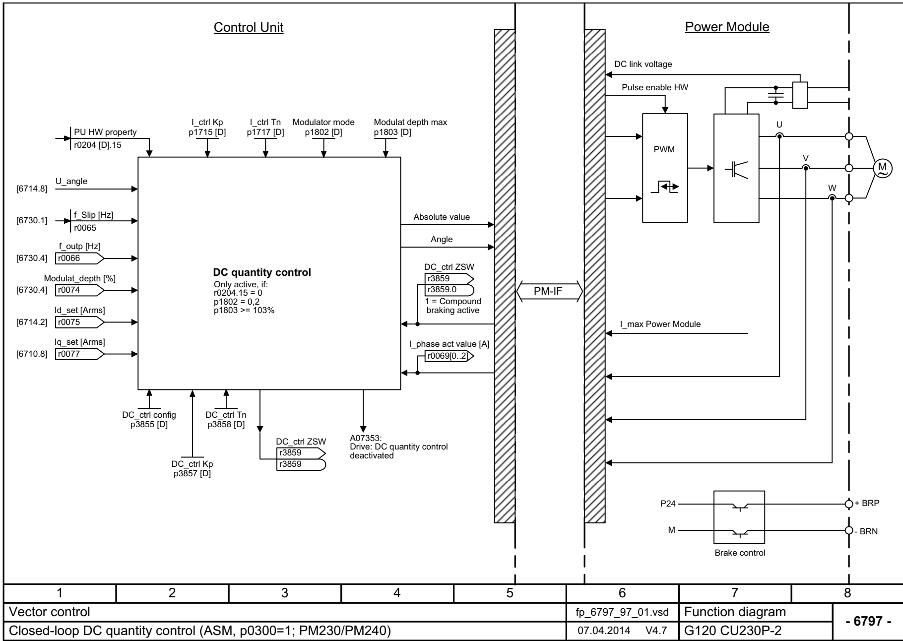
图 3-91 6797 - 恒定参数控制
