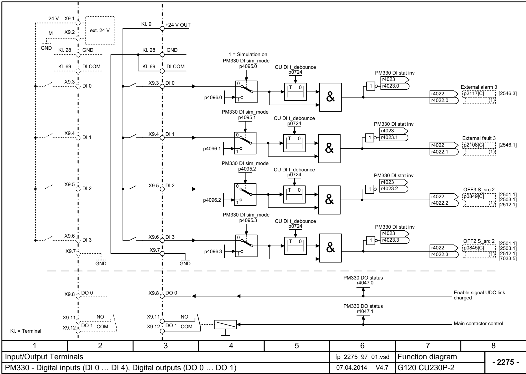
图 3-15 2275 - PM330 - 数字量输入 (DI 0 ... DI 4), 数字量输出 (DO 0 ... DO 1)
