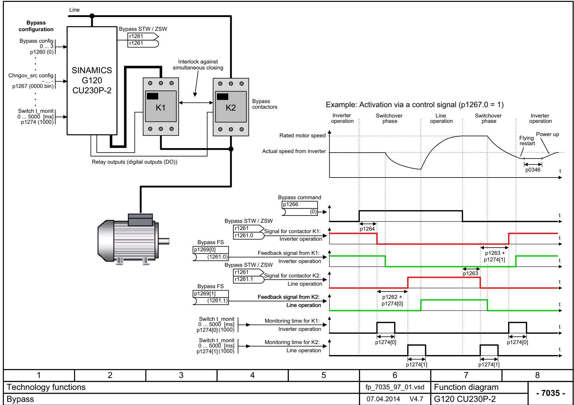
图 3-97 7035 - 旁路
