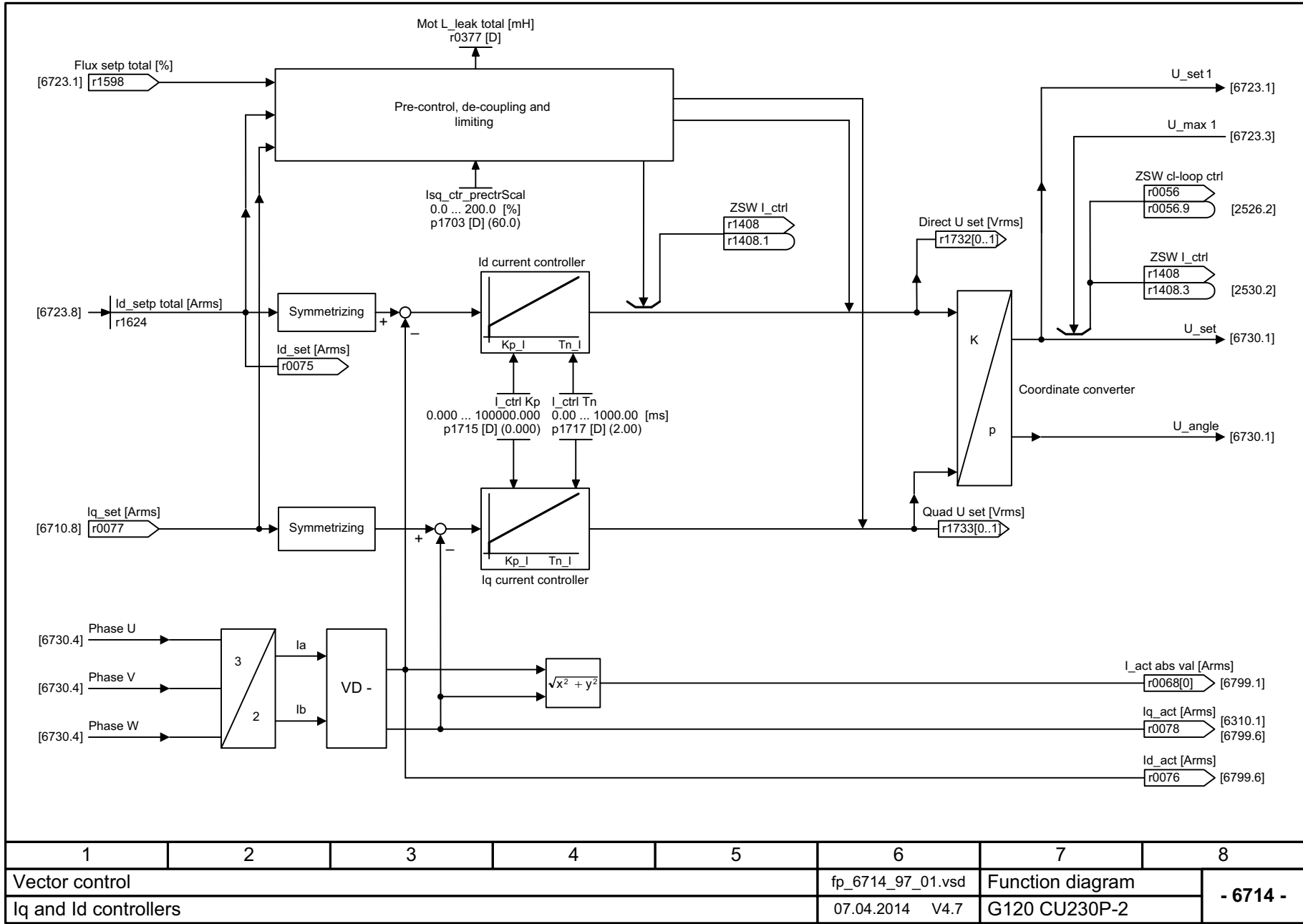
图 3-87 6714 - Iq 控制器和 Id 控制器
