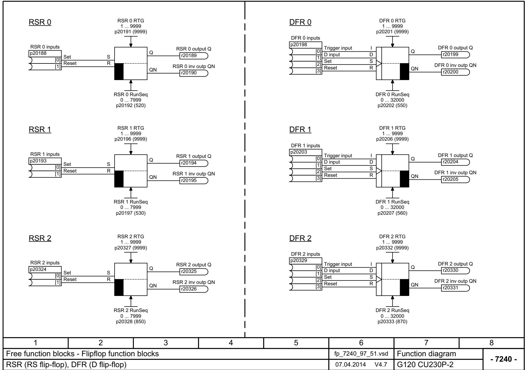
图 3-114 7240 - RSR (R 主导的 RS 触发), DFR (R 主导的 D 触发器)
