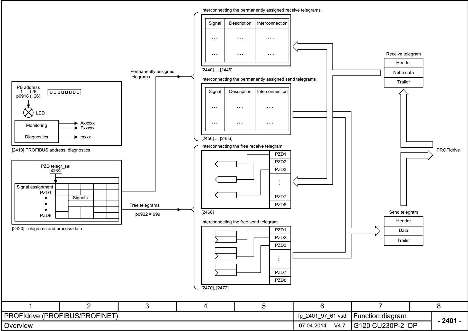
图 3-18 2401 - 一览
