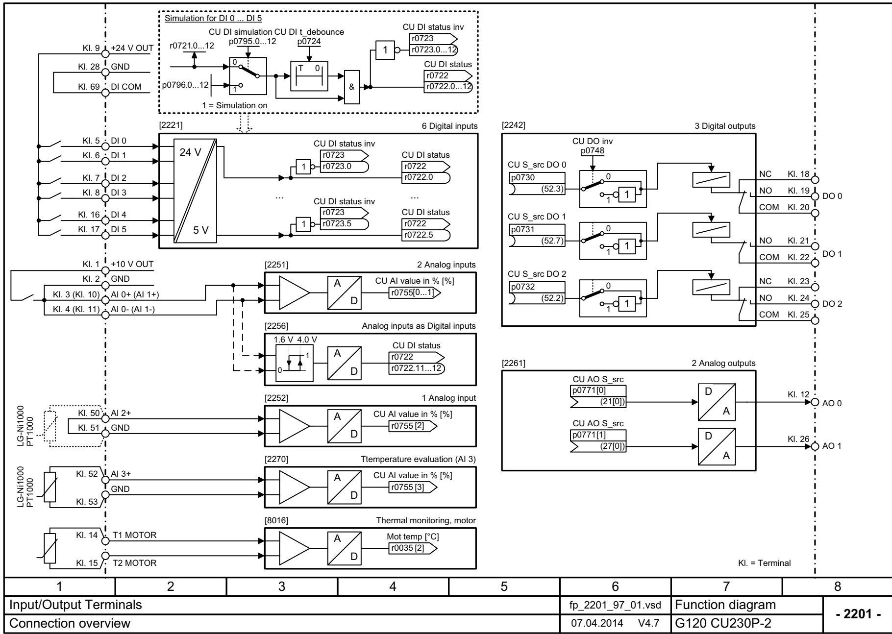
图 3-5 2201 - 接口一览
