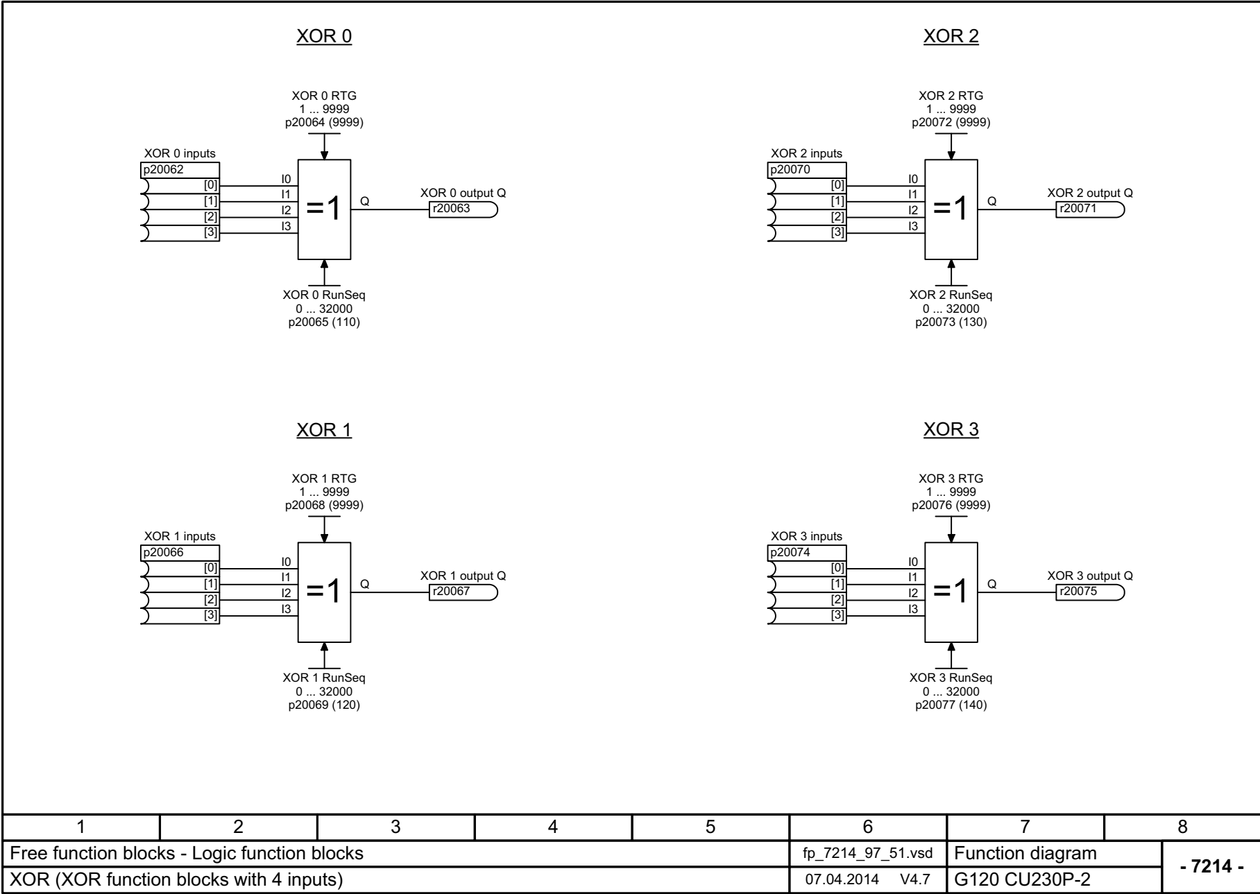
图 3-103 7214 - XOR (有 4 个输入的“异或”功能块)
