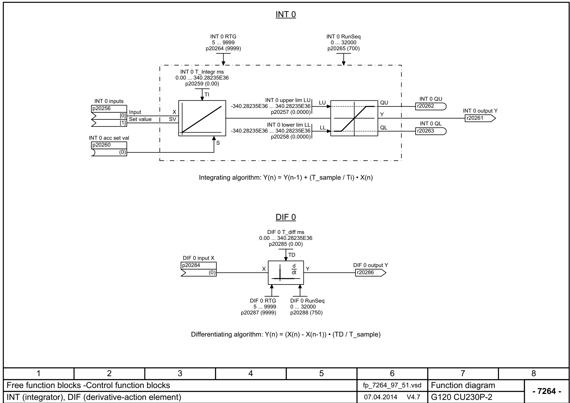
图 3-118 7264 - INT (积分器), DIF (微分器)
