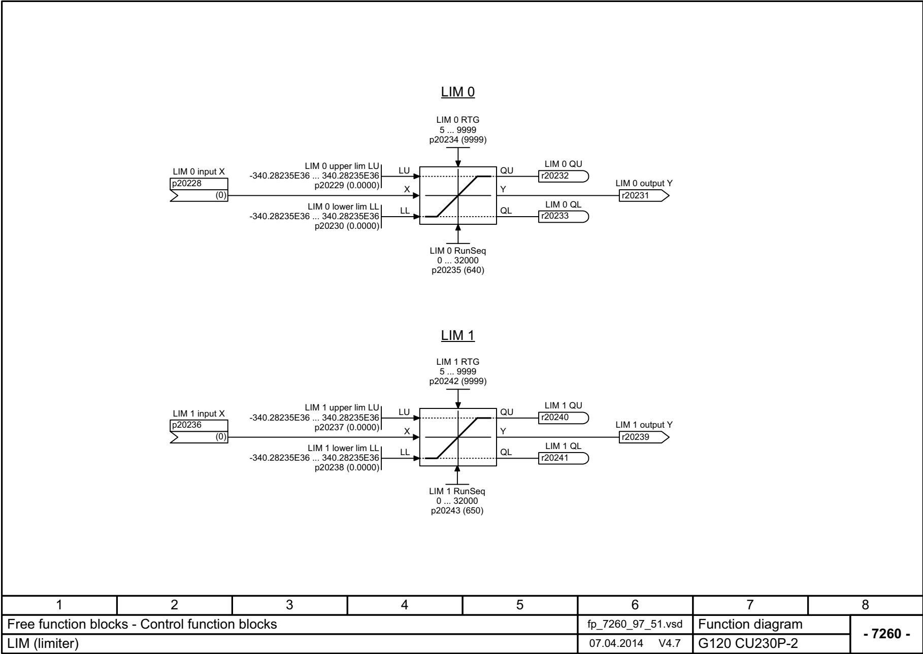
图 3-116 7260 - LIM (限制器)
