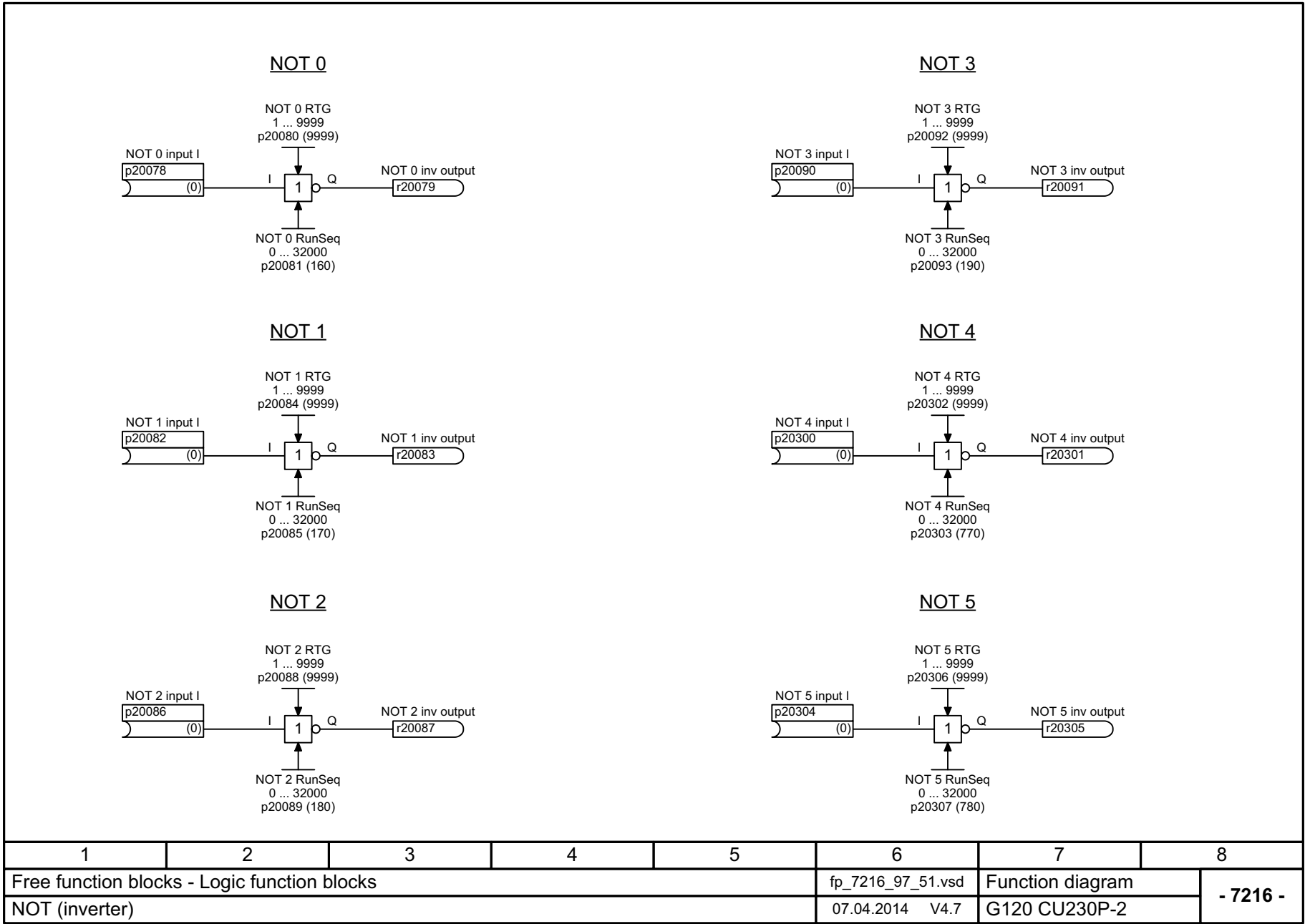
图 3-104 7216 - NOT (非)
