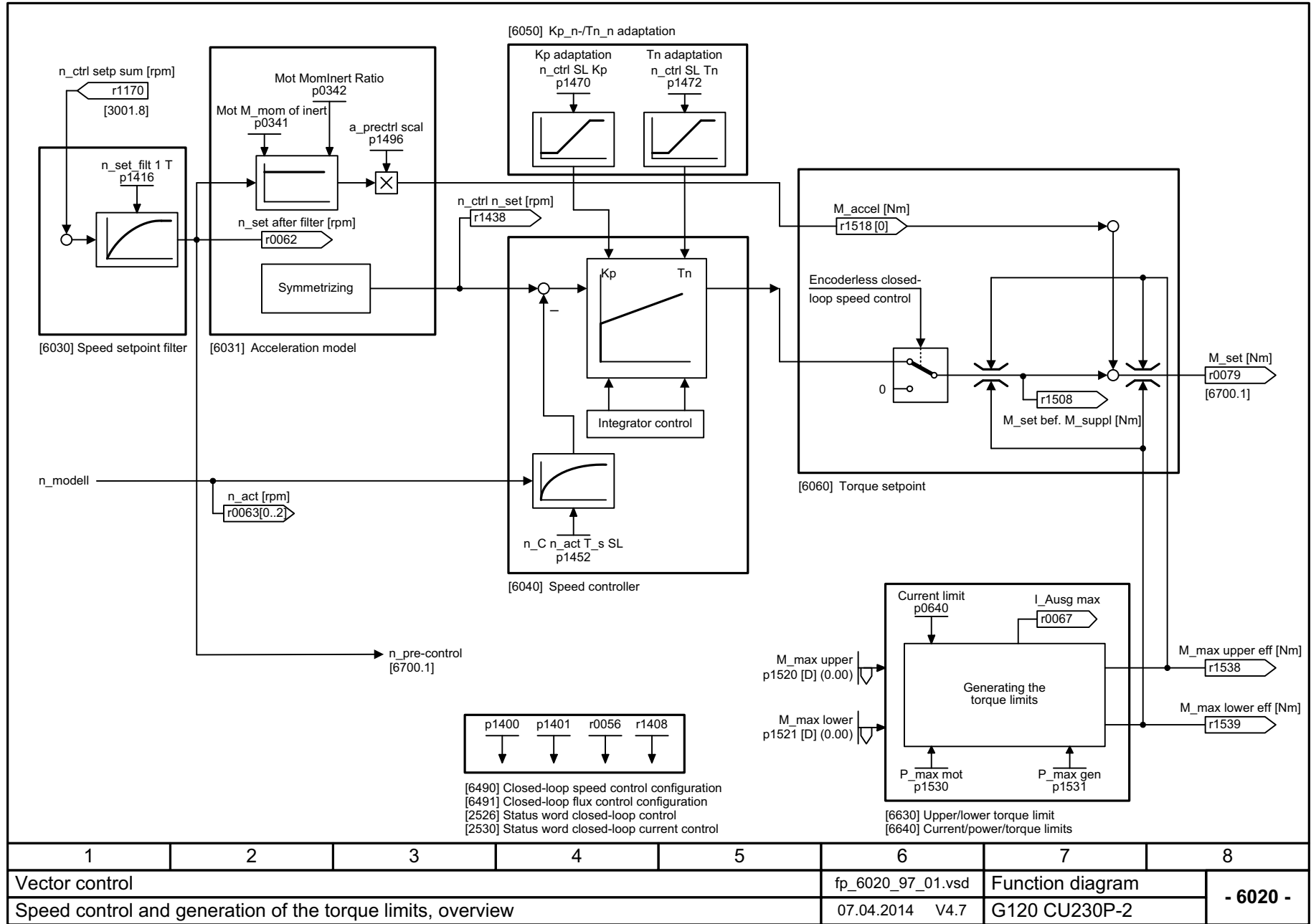
图 3-70 6020 - 转速控制和转矩限值形成, 一览
