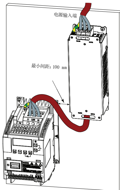
连接进线电抗器到变频器
