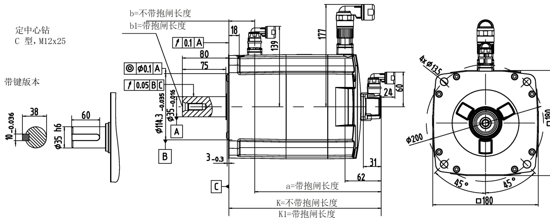
轴高 90 mm，带绝对编码器（单位：mm）
