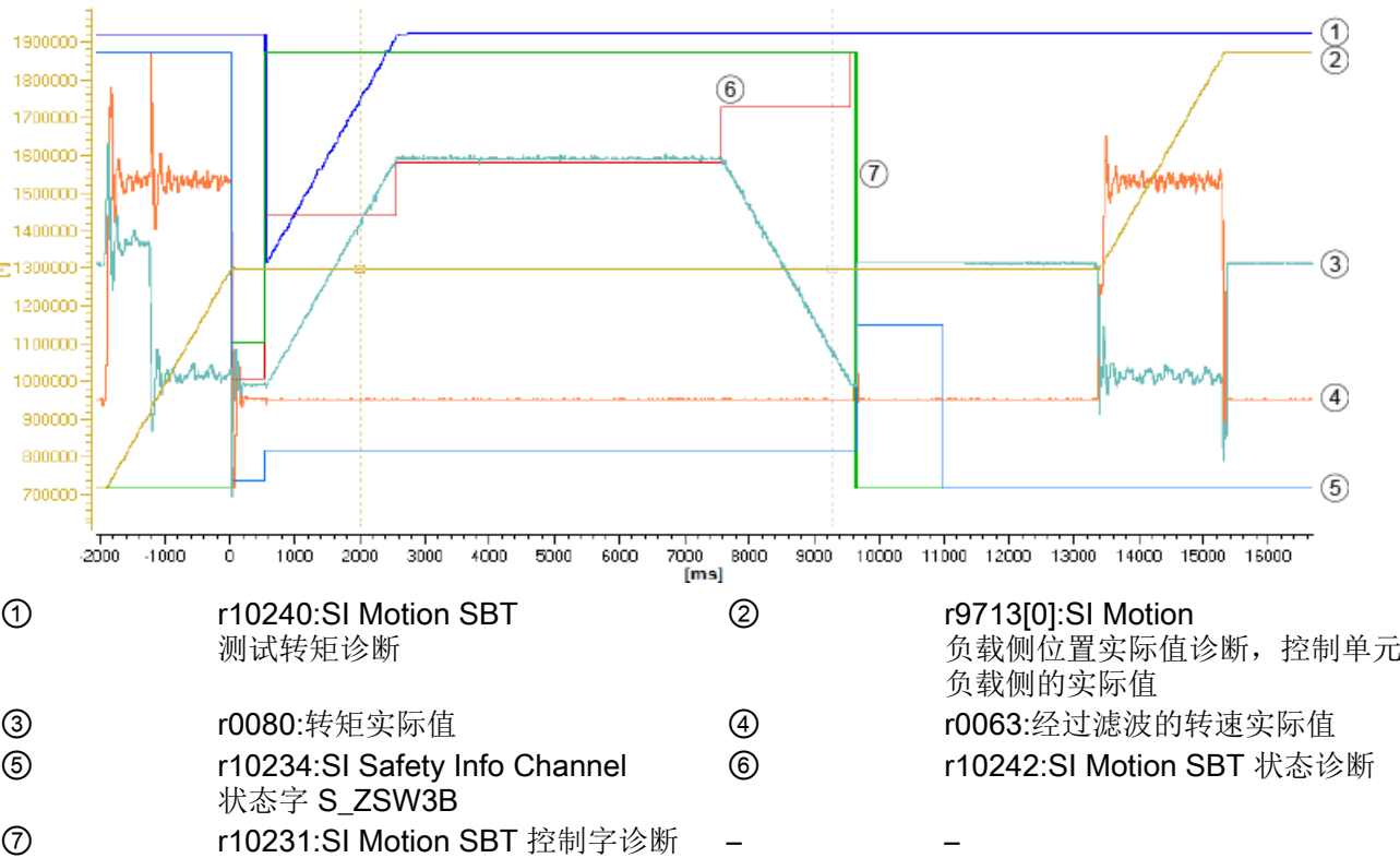
图 A-16 曲线图示例：SBT
