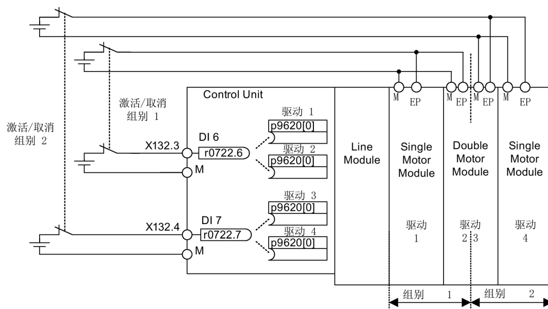
图 5-2 示例：端子分组：以书本型电机模块和 CU320-2 为例
