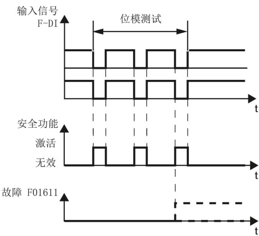
图 5-3 变频器对位模测试作出响应
