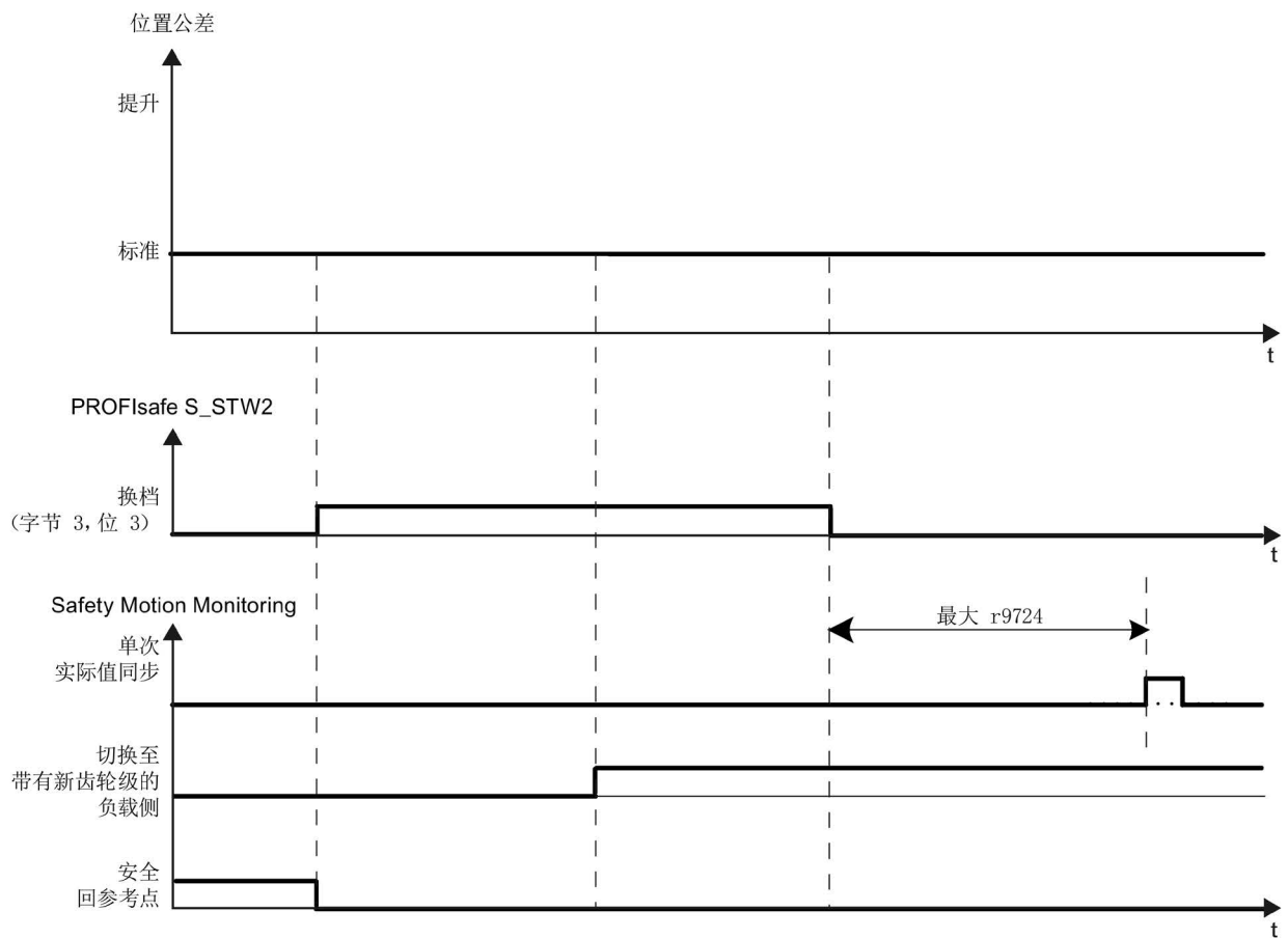
图 4-20 不提升位置公差的齿轮级切换，从“0”到“1”
