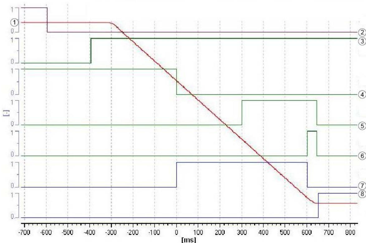
曲线图示例：带编码器、停止响应为“STOP D”的“SDI+”
