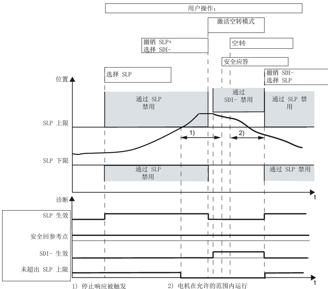
图 4-12 SLP 和回退的工作时序
