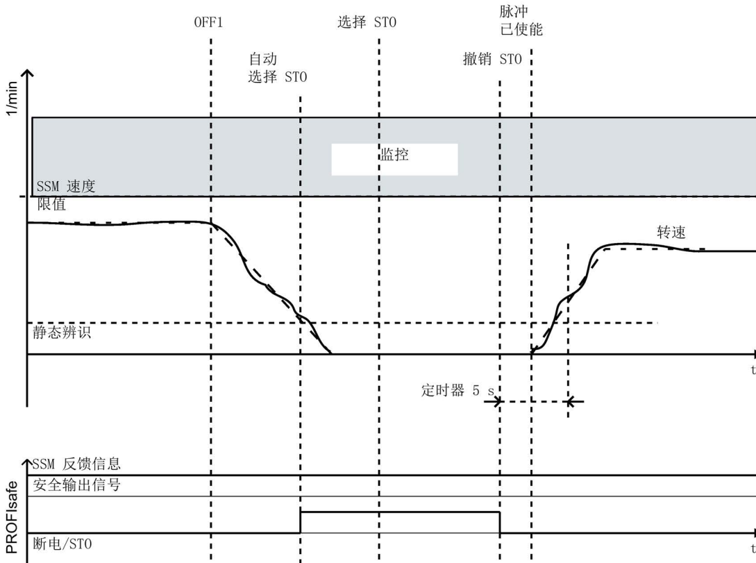
图 4-9 不带编码器的SSM ( p9509.0 = 0 )
