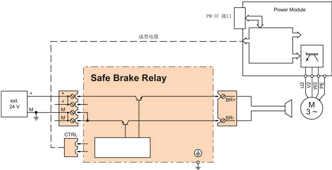
图 3-1 模块型设备上的安全制动继电器接线示例
