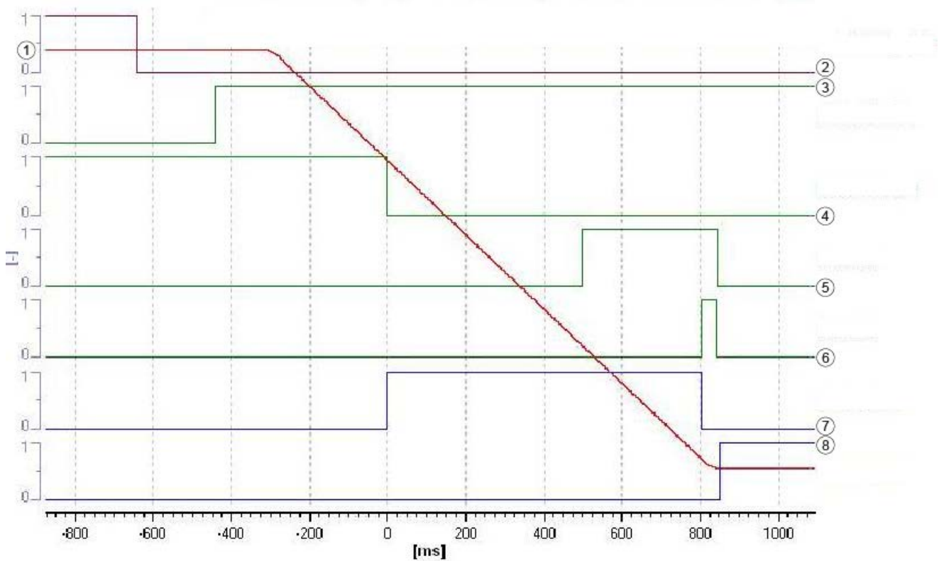
曲线图示例：带编码器、停止响应为“STOP E”的“SDI+”
