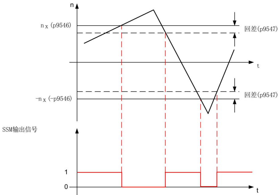
图 4-8 回差使能后 SSM 的安全输出信号
