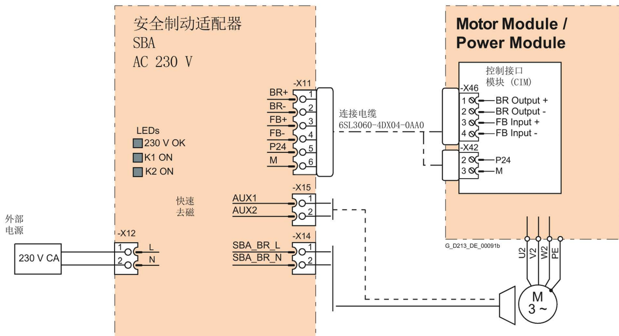
图 3-2 安全制动适配器接线图
