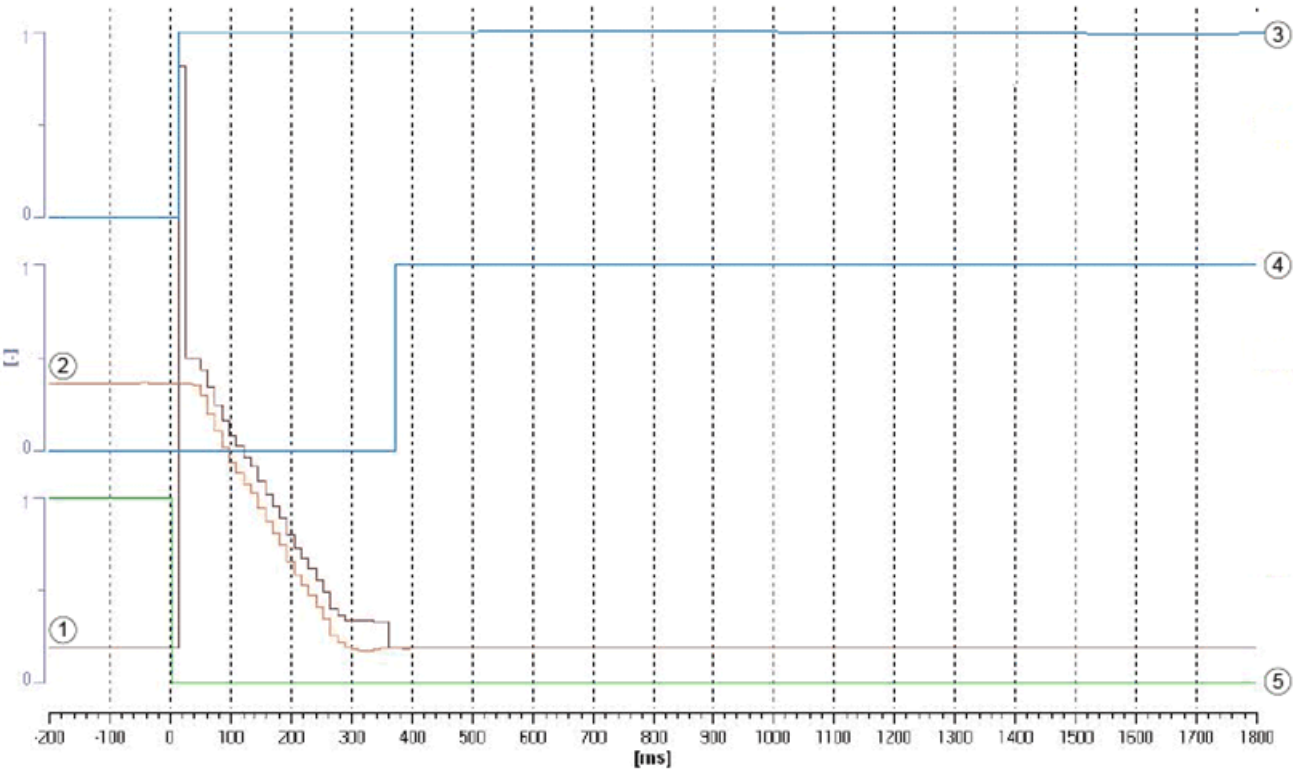
曲线图示例：SS1（带编码器）
