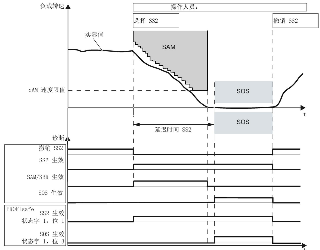
图 3-4 安全功能 SS2 的制动时序图与诊断信号（带 SAM 的 SS2）
