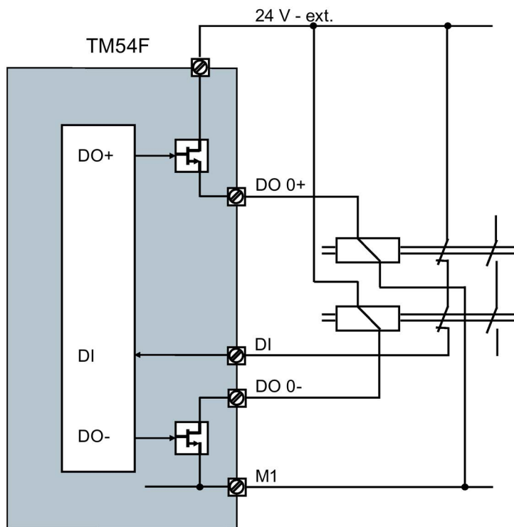
图 6-21 F-DO 回路的“检查模式 2: F-DO 在 DI 中回读 (继电器回路)”
