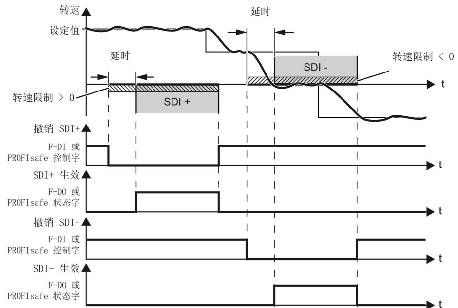
图 3-6 SDI (Safe Direction) 安全功能的工作时序
