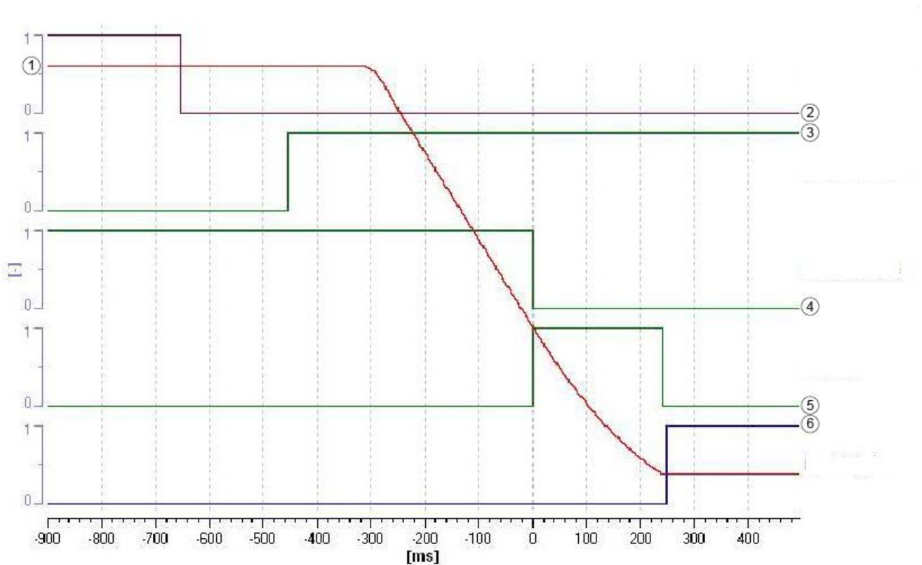
曲线图示例：带编码器、停止响应为“STOP B”的“SDI+”
