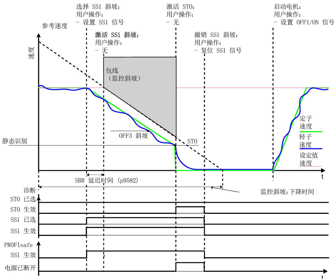
图 4-3 不带编码器，带 SBR 监控的 SS1 控制时序图 (p9506 = 1)
