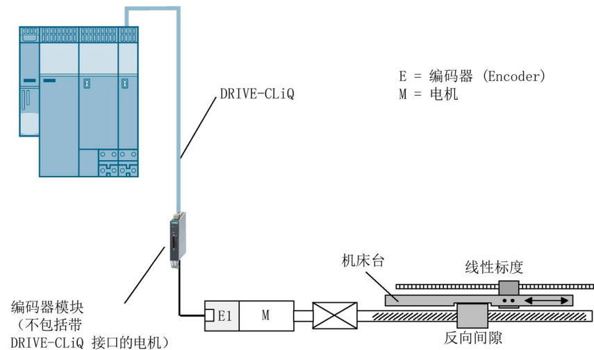
图 4-15 示例：单编码器系统
