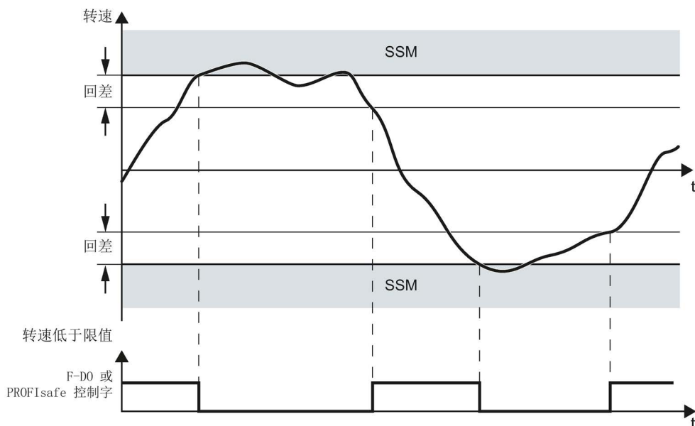
图 3-5 SSM (Safe Speed Monitor) 安全功能的工作时序
