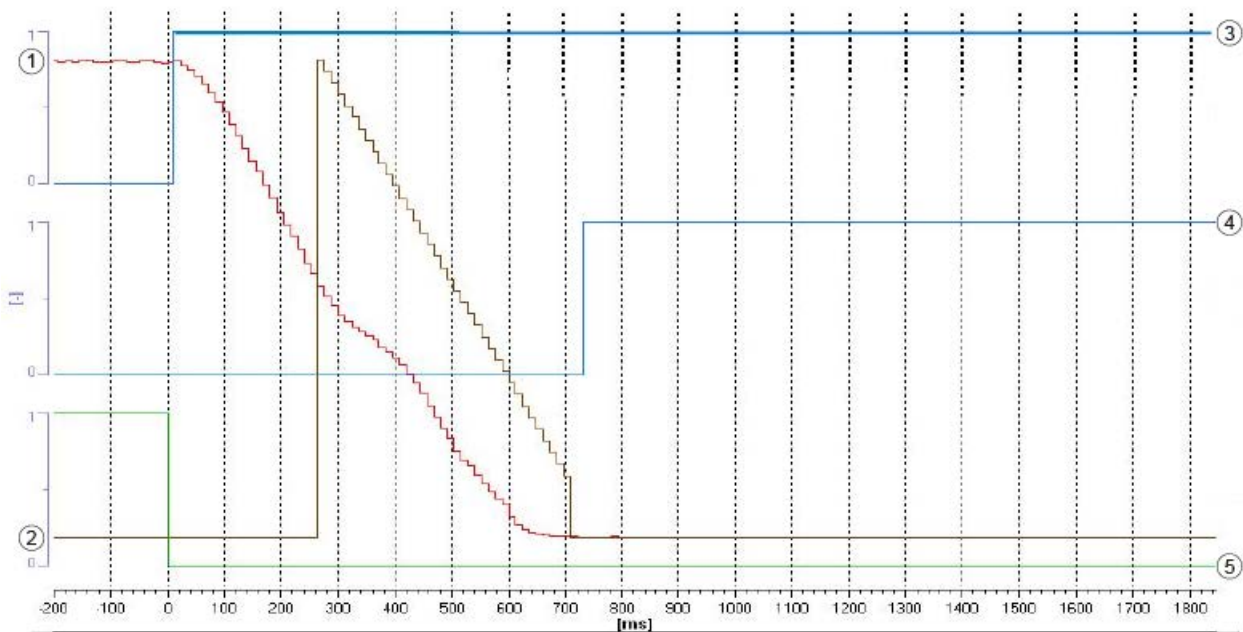
曲线图示例：不带编码器的SS1
