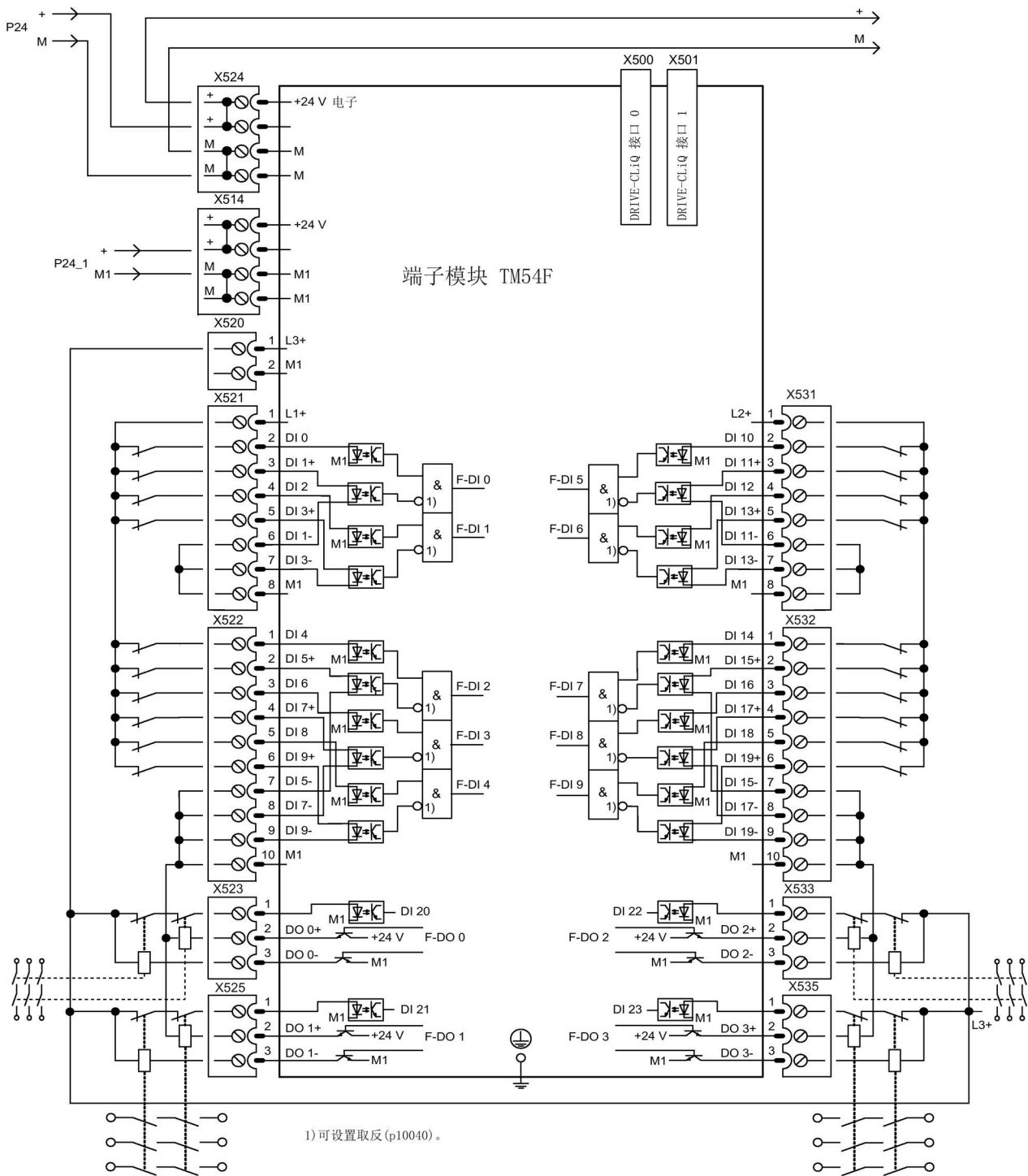
图 4-22 TM54F 接线示例
