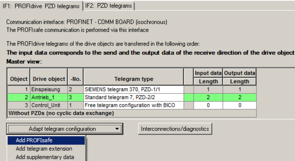
图 6-41 报文配置 3
