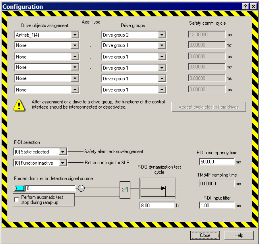
图 6-16 配置TM54F
