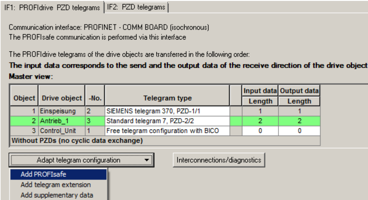
图 6-36 报文配置 3
