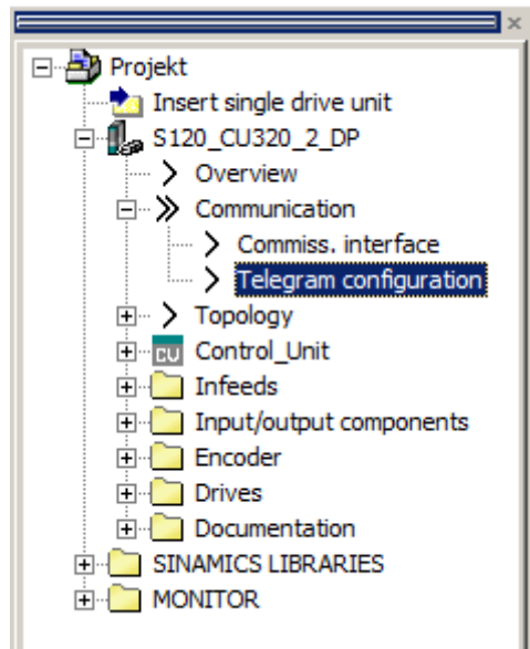
图 6-39 报文配置 1
