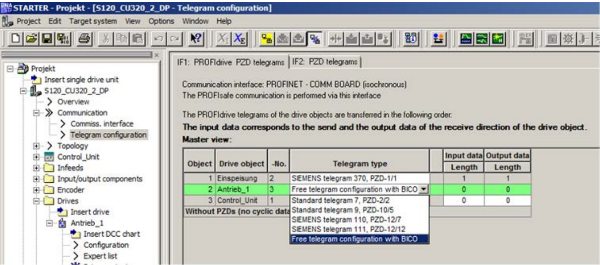
图 6-35 报文配置 2
