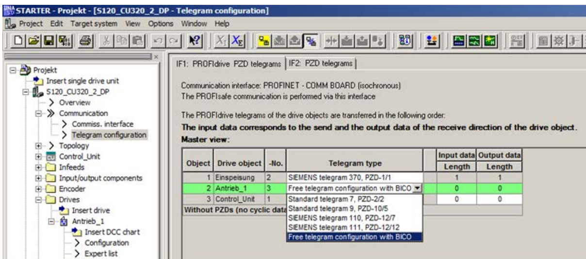
图 6-40 报文配置 2
