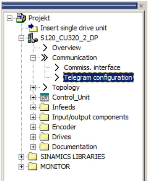
图 6-34 报文配置 1
