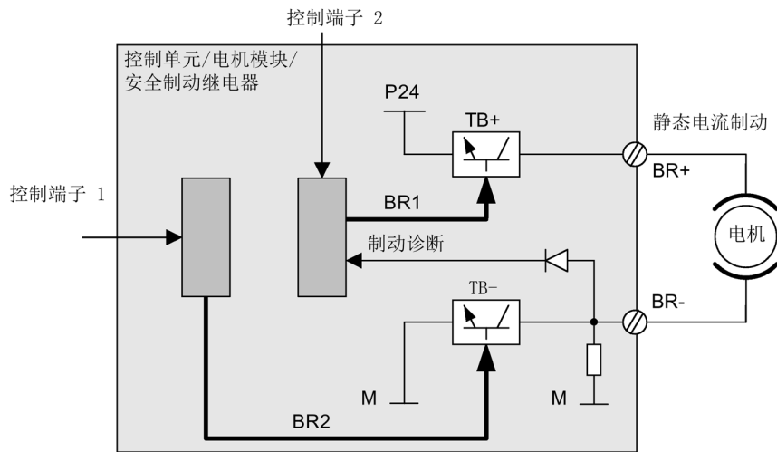
图 4-2 双通道式制动控制 模块型（示例）
