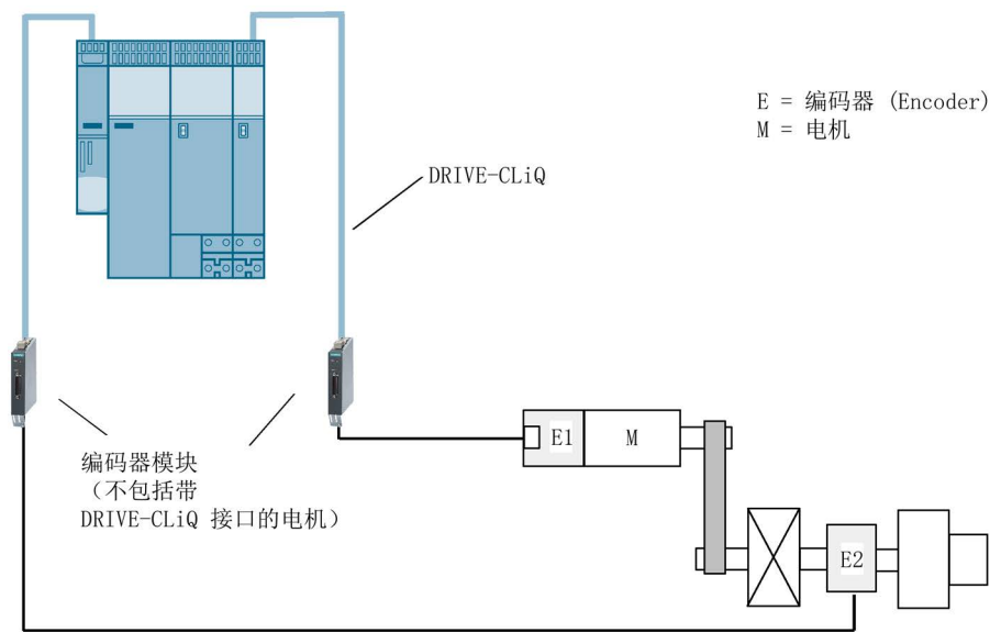
图 4-17 示例：回转轴上的双编码器系统
