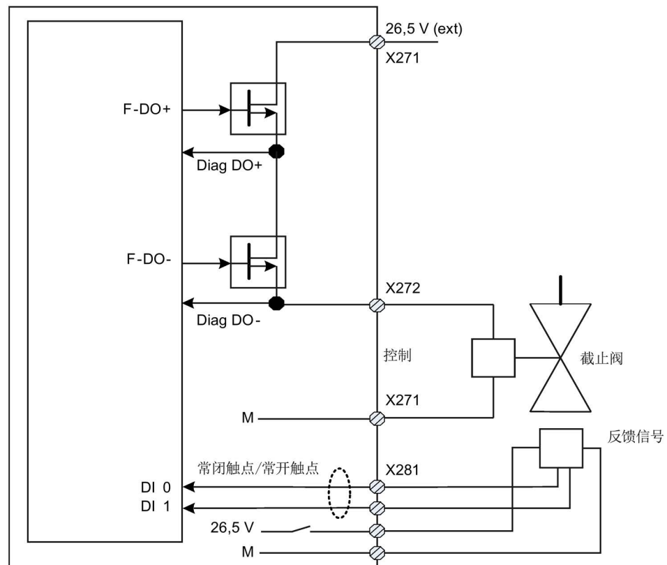
图 4-1 (为一根轴) 连接截止阀
