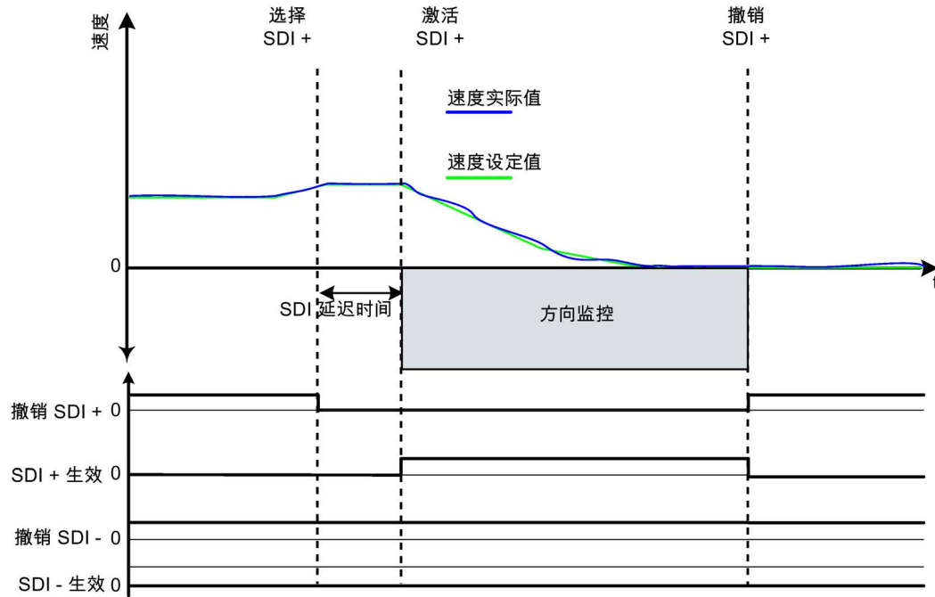
图 4-10 带编码器的 SDI 的工作原理
