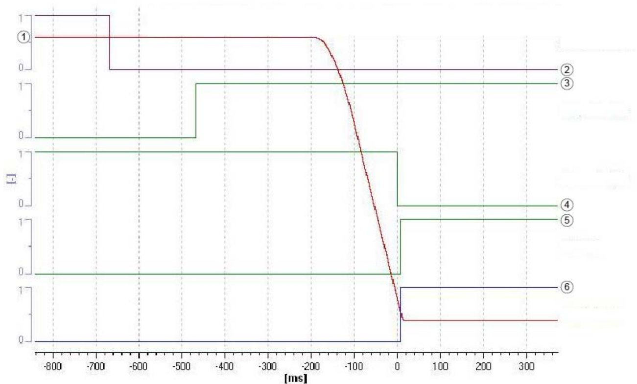
曲线图示例：带编码器、停止响应为“STOP A”的“SDI+”
