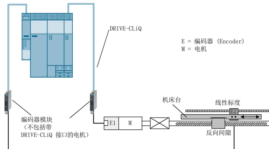
图 4-16 示例：滚珠丝杠上直线轴的双编码器系统
