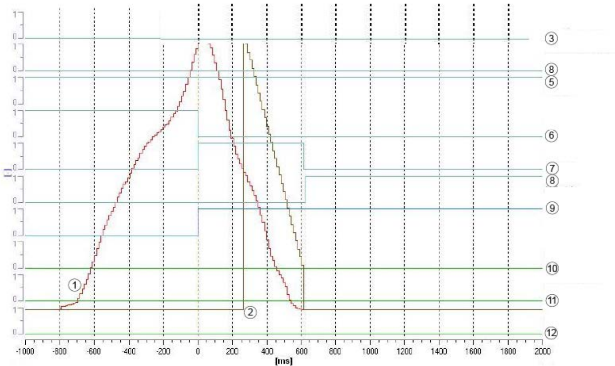
曲线图示例：不带编码器的 SLS，停止响应为“STOP B”
