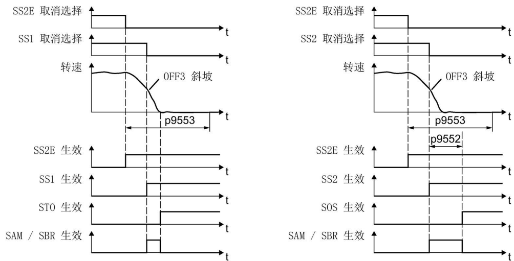
图 4-6 通过功能 SS1（左图）和 SS2（右图）中断功能 SS2E。
