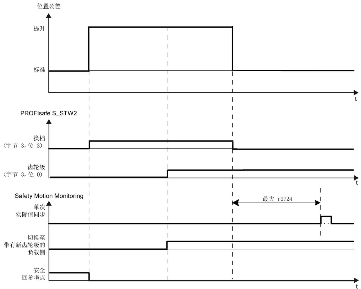
图 4-21 提升位置公差时的齿轮级切换
