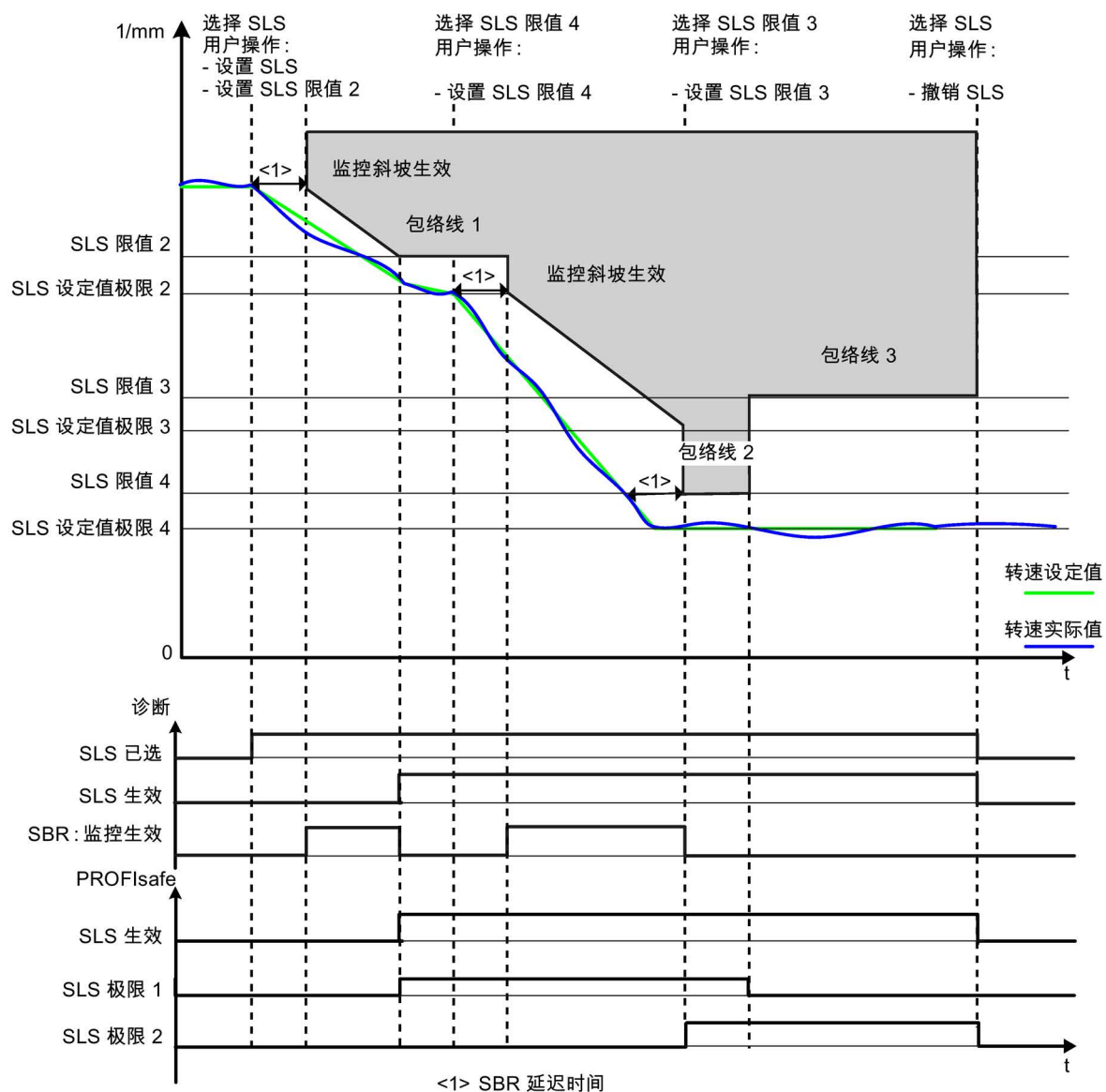
图 4-14 不带编码器的“Safe Brake Ramp”（执行 SLS 时）
