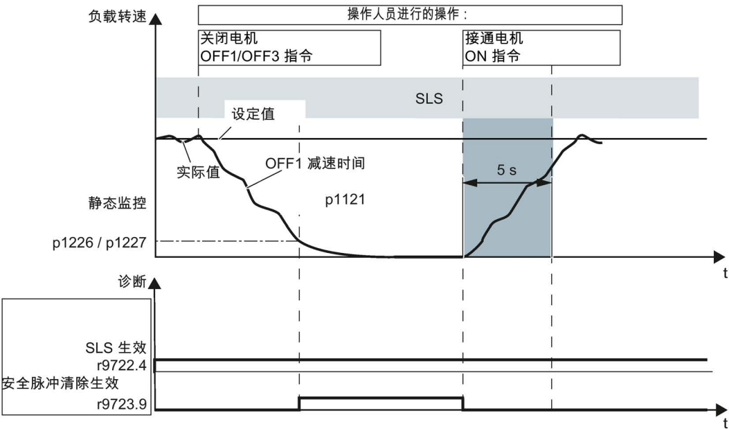
图 4-7 自动生效的 SLS 的工作时序，以关闭并重启电机为例（不带编码器）
