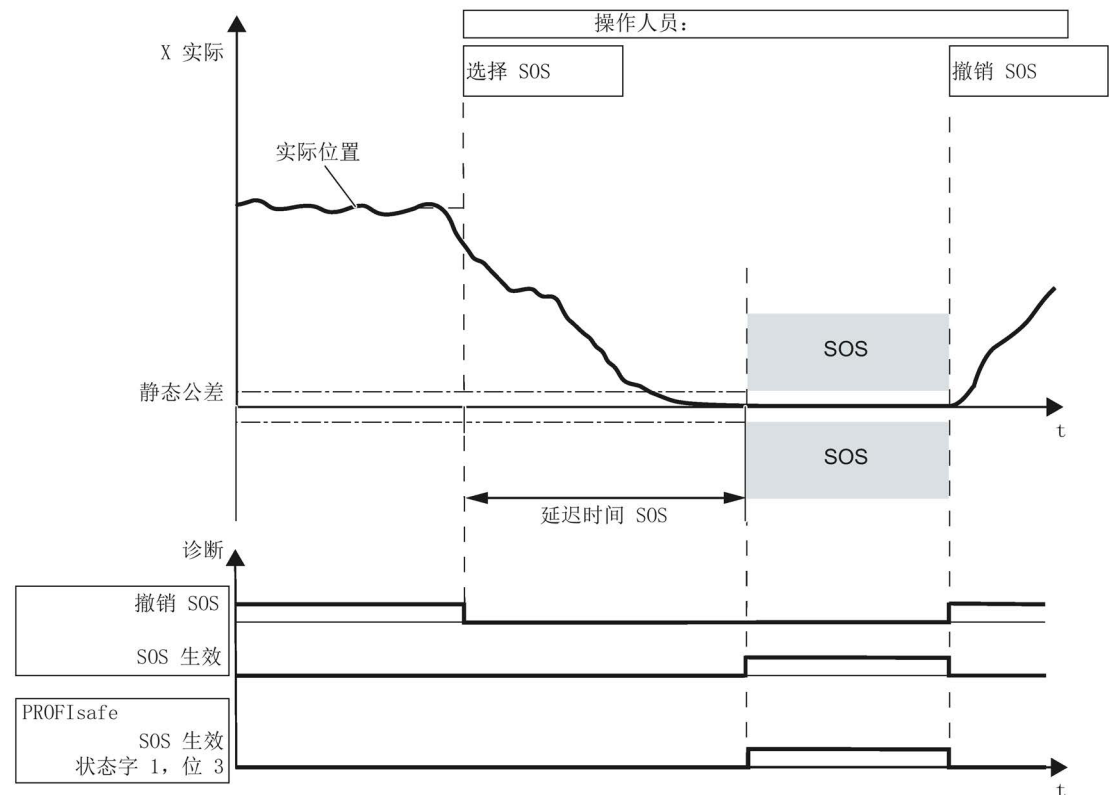
图 3-3 静态公差
