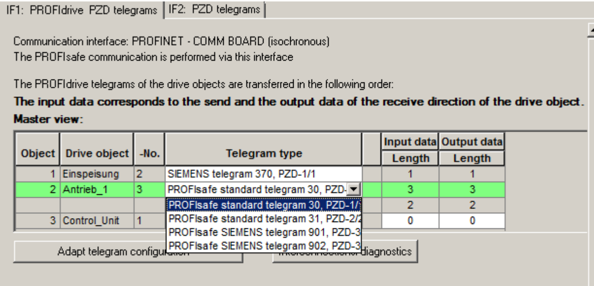
图 6-42 报文配置 4
