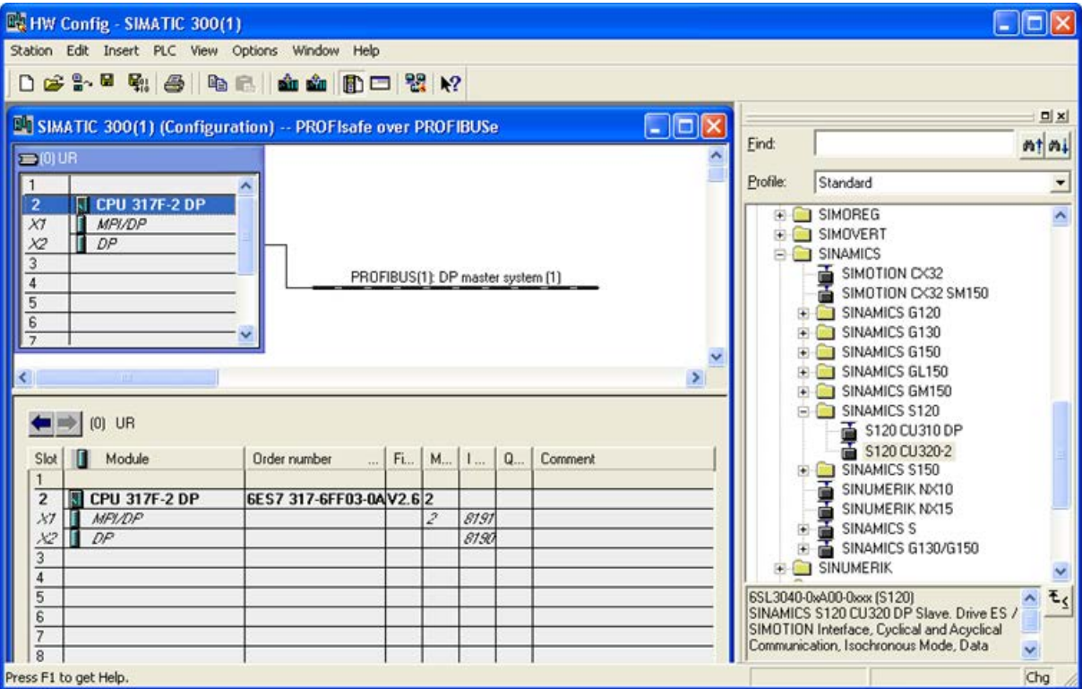
图 6-31 选择驱动器
