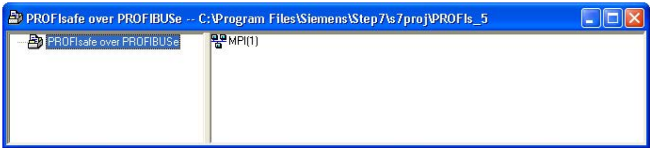
图 6-24 创建新项目
