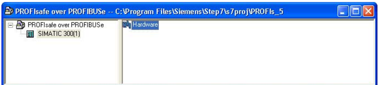
图 6-26 调用 HW-Config
