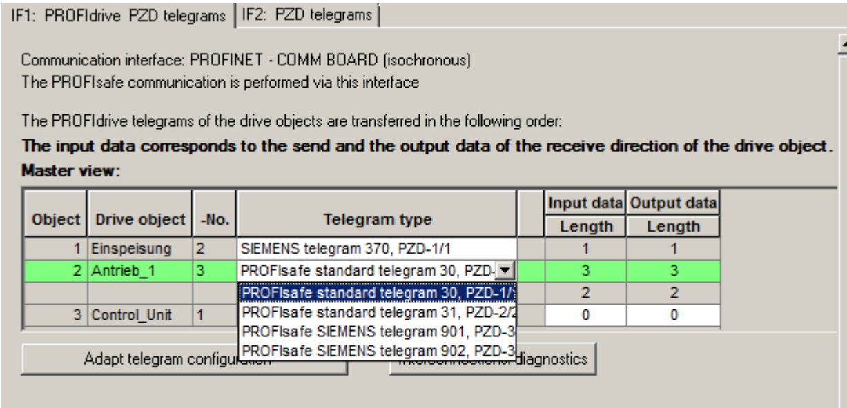
图 6-37 报文配置 4
