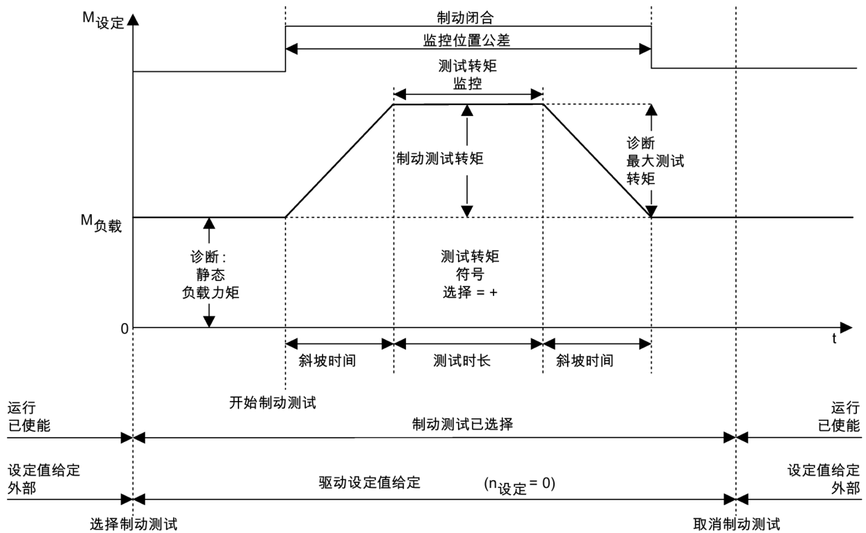
图 4-13 SBT: 时序
