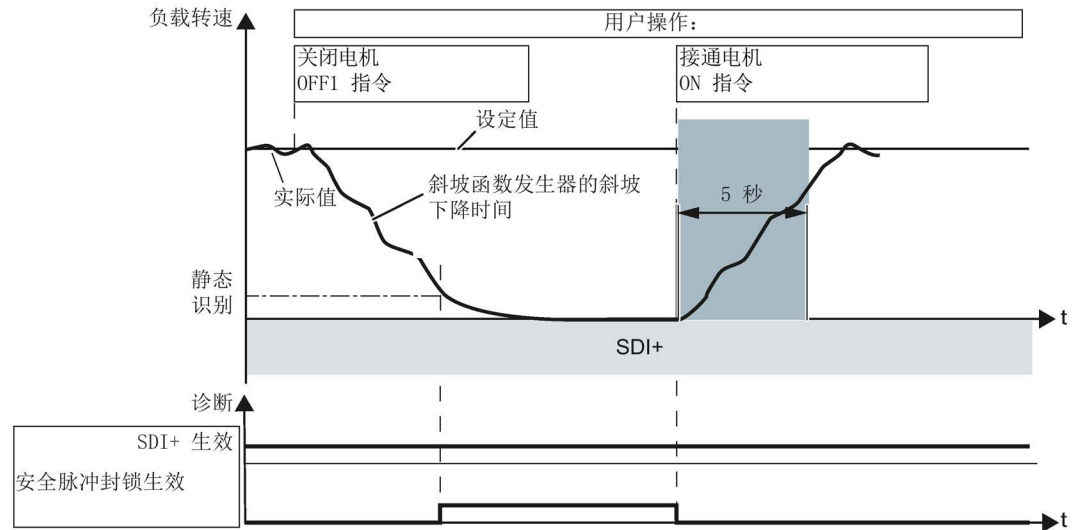
图 4-11 自动生效的 SDI 的工作时序，以关闭并重启电机为例（不带编码器）
