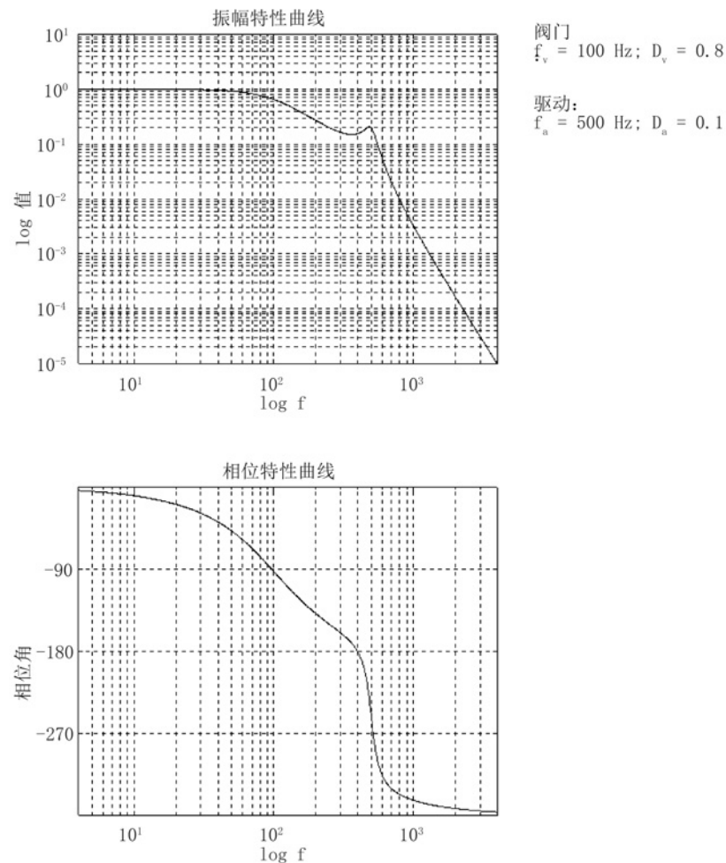
图 4-43 被控对象的频率响应特性 ( f_{\text{阀门}} \ll f_{\text{液压缸}} )
