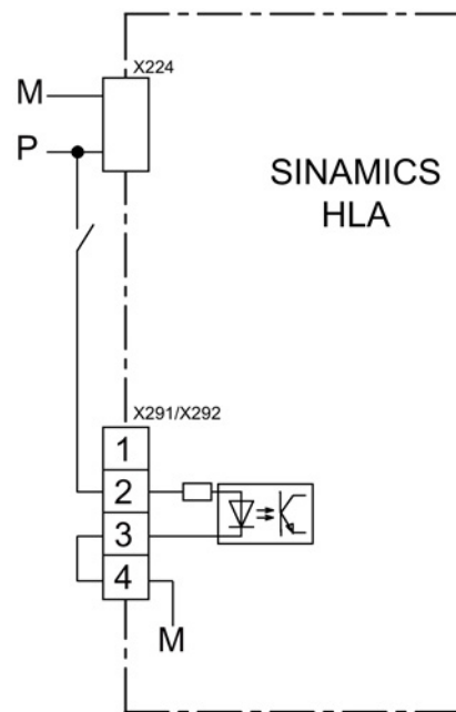
图 6-2 使能端子的布线，含内部光电耦合器
