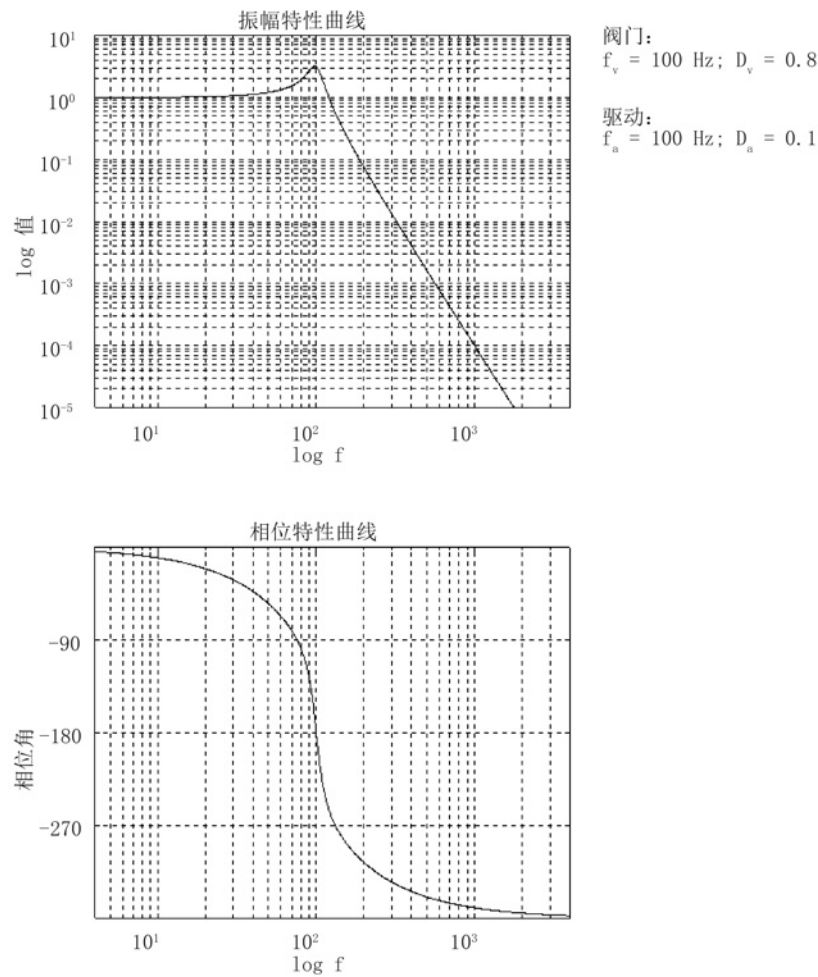
图 4-44 被控对象的频率响应特性 ( f_{\text{阀门}} \approx f_{\text{液压缸}} )
