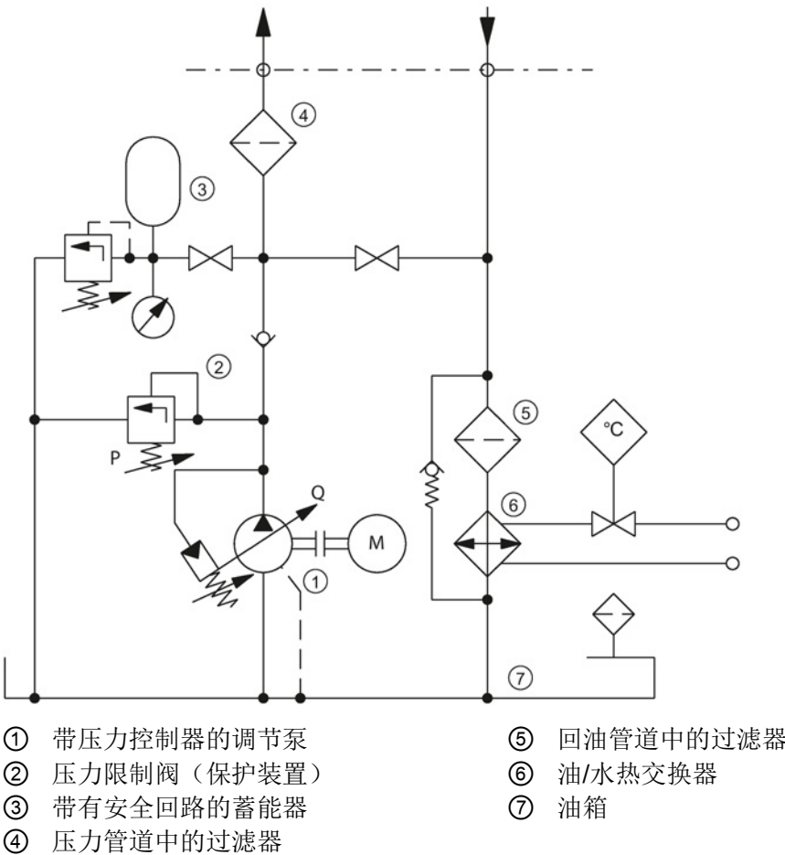
图 3-6 典型液压装置一览
