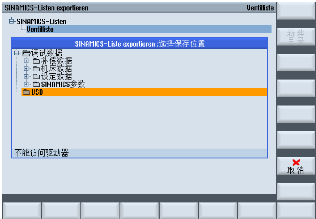
图 4-22 选择存档
