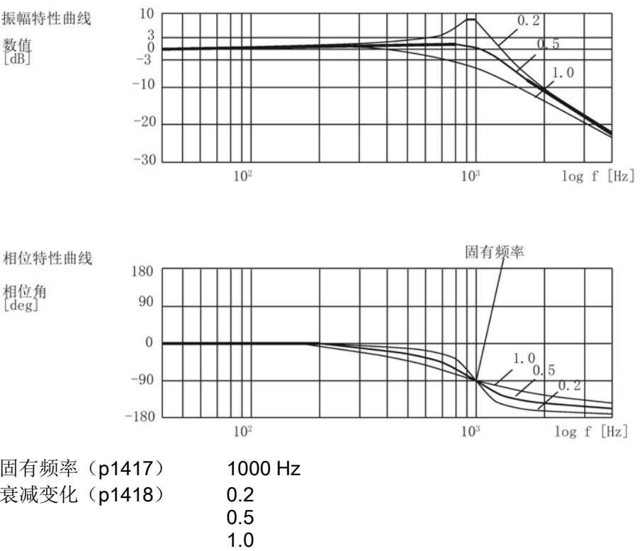
图 5-3 低通滤波器性能 (PT2)
