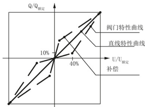
图 A-10 电气阀门拐点补偿
