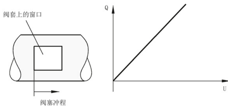
图 A-7 阀套上的控制窗口
