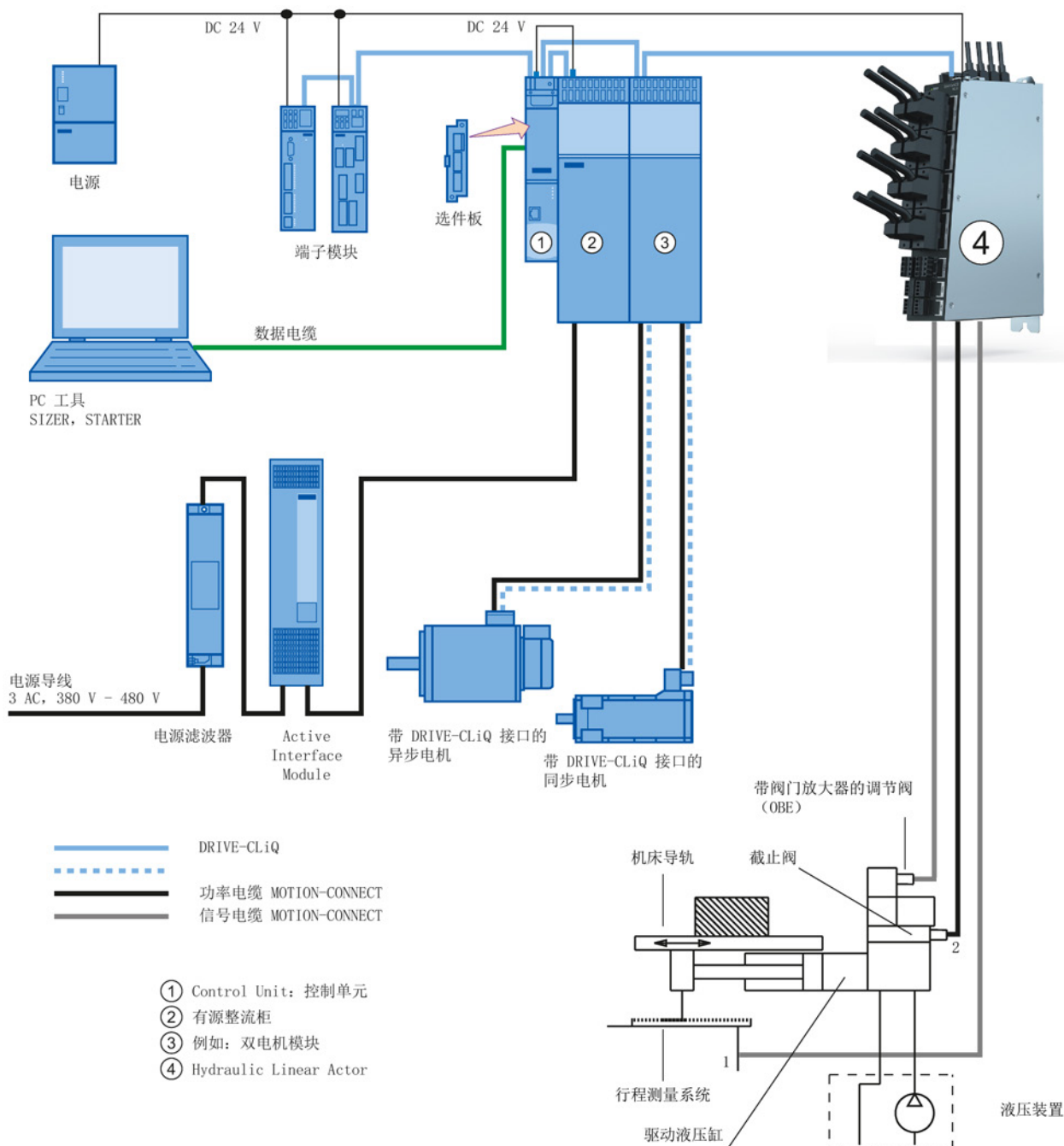
图 2-1 包含电气组件和液压组件的 SINAMICS 驱动系统示例
