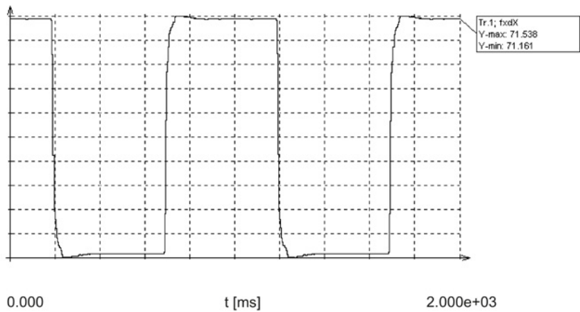
图 4-56 在信号类型为“方波”时，“位置实际值”到位置设定值的跟踪
