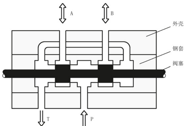
图 A-1 阀塞原理
