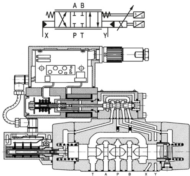
图 A-15 前馈控制的调节阀
