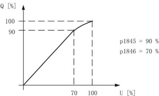
图 5-17 拐点补偿示例
