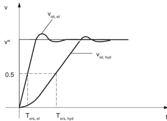
图 4-46 液压/电气插补
