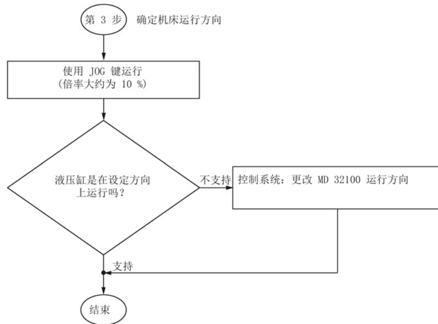
图 4-41 NC 运行方向定义的调试顺序图
