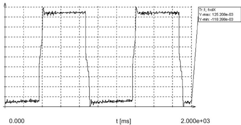
图 4-55 在信号类型为“方波”时，“速度实际值”到速度设定值的跟踪
