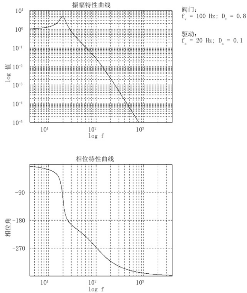
图 4-45 被控对象的频率响应特性 ( f_{\text{阀门}} \gg f_{\text{液压缸}} )
