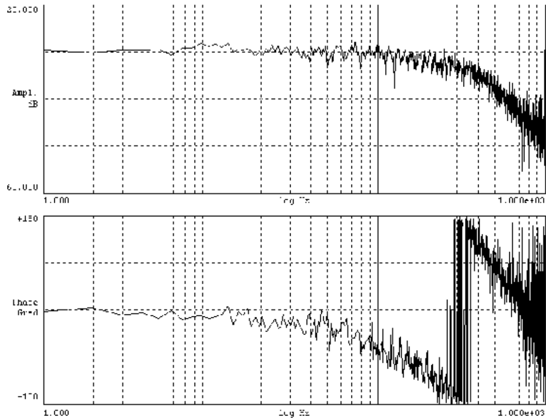
图 4-47 HR 调节阀阀门频率响应（示例）
