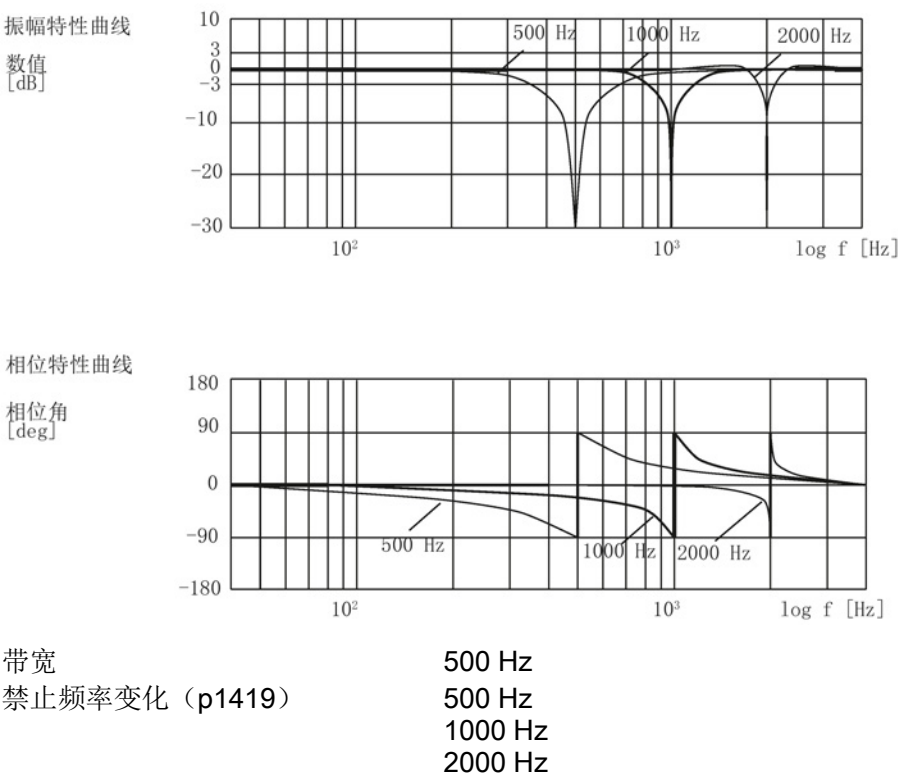
图 5-4 未衰减带阻的频率响应
