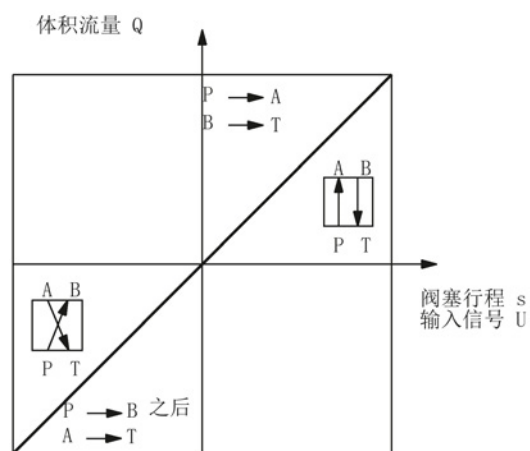
图 A-6 线性体积流量特性曲线
