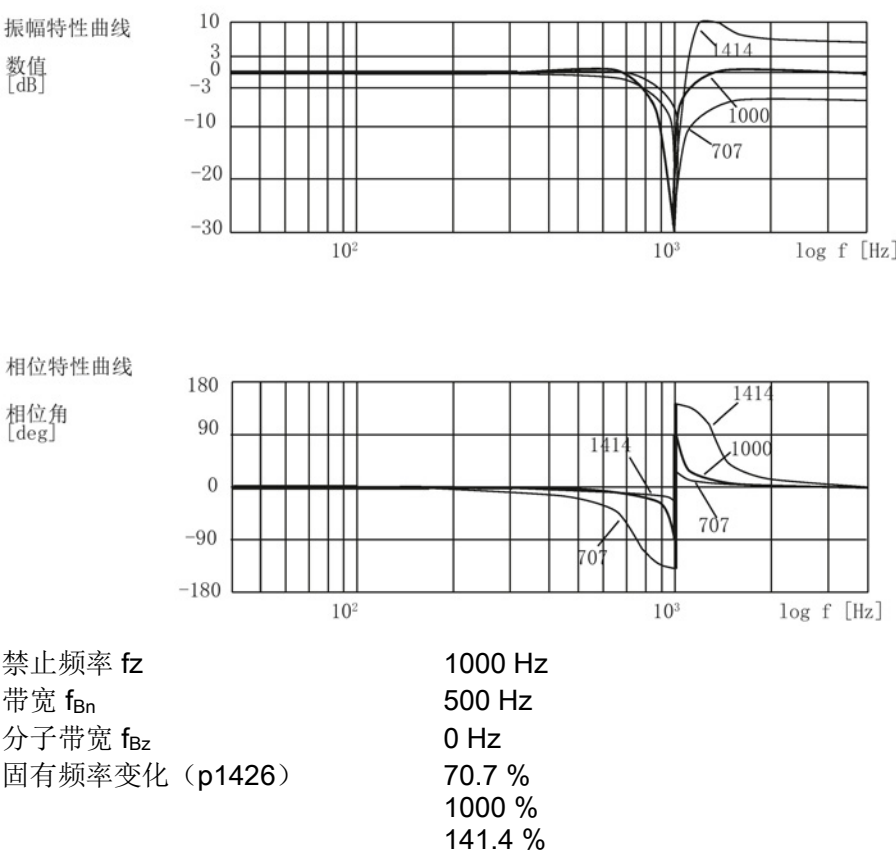
图 5-6 通用带阻的频率响应
