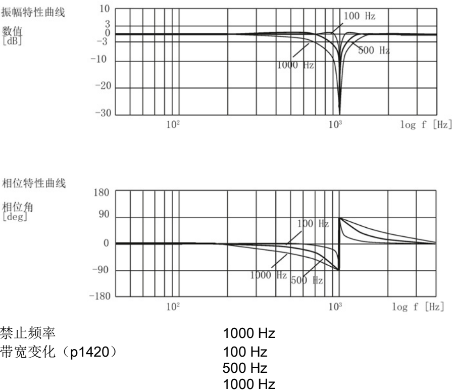
图 5-5 未衰减带阻的频率响应
