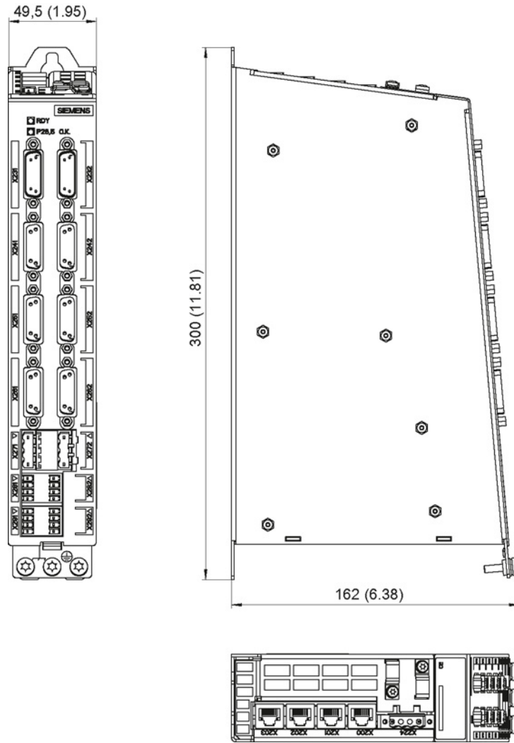
图 6-3 HLA 模块外形尺寸图，所有数据单位：mm 和(inch)
