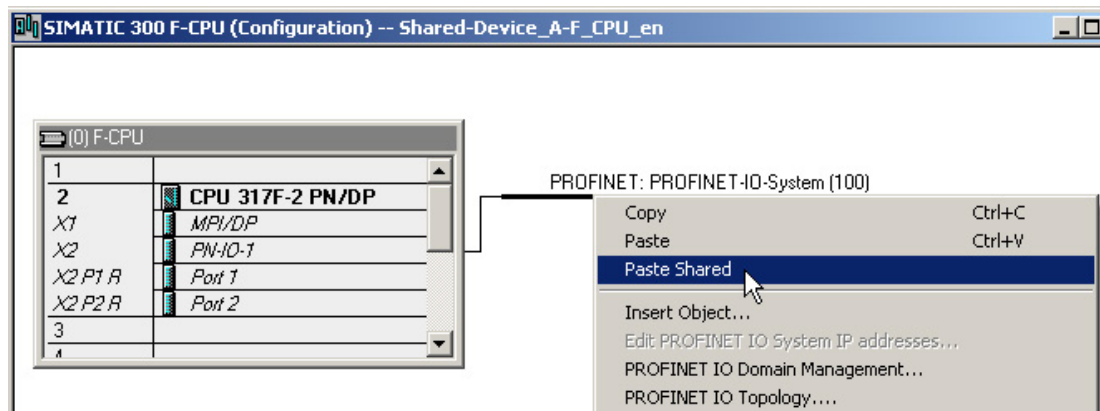
图 11-46 PROFI-safe 控制系统配置
