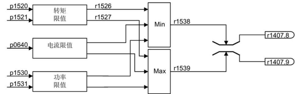
图 5-14 转矩限制
