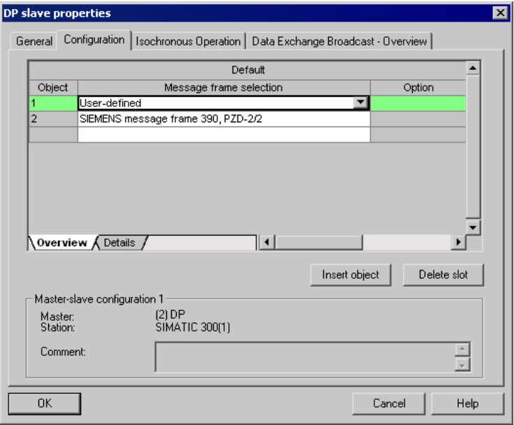
图 11-26 “从站-从站”通讯时的报文分配
