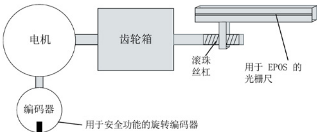
图 8-21 举例 2: EPOS和安全回参考点, 线性
