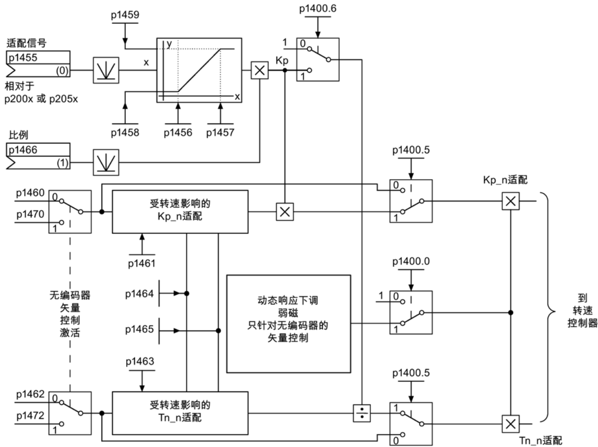
图 5-7 K_{p\_n}/T_{n\_n} 适配
