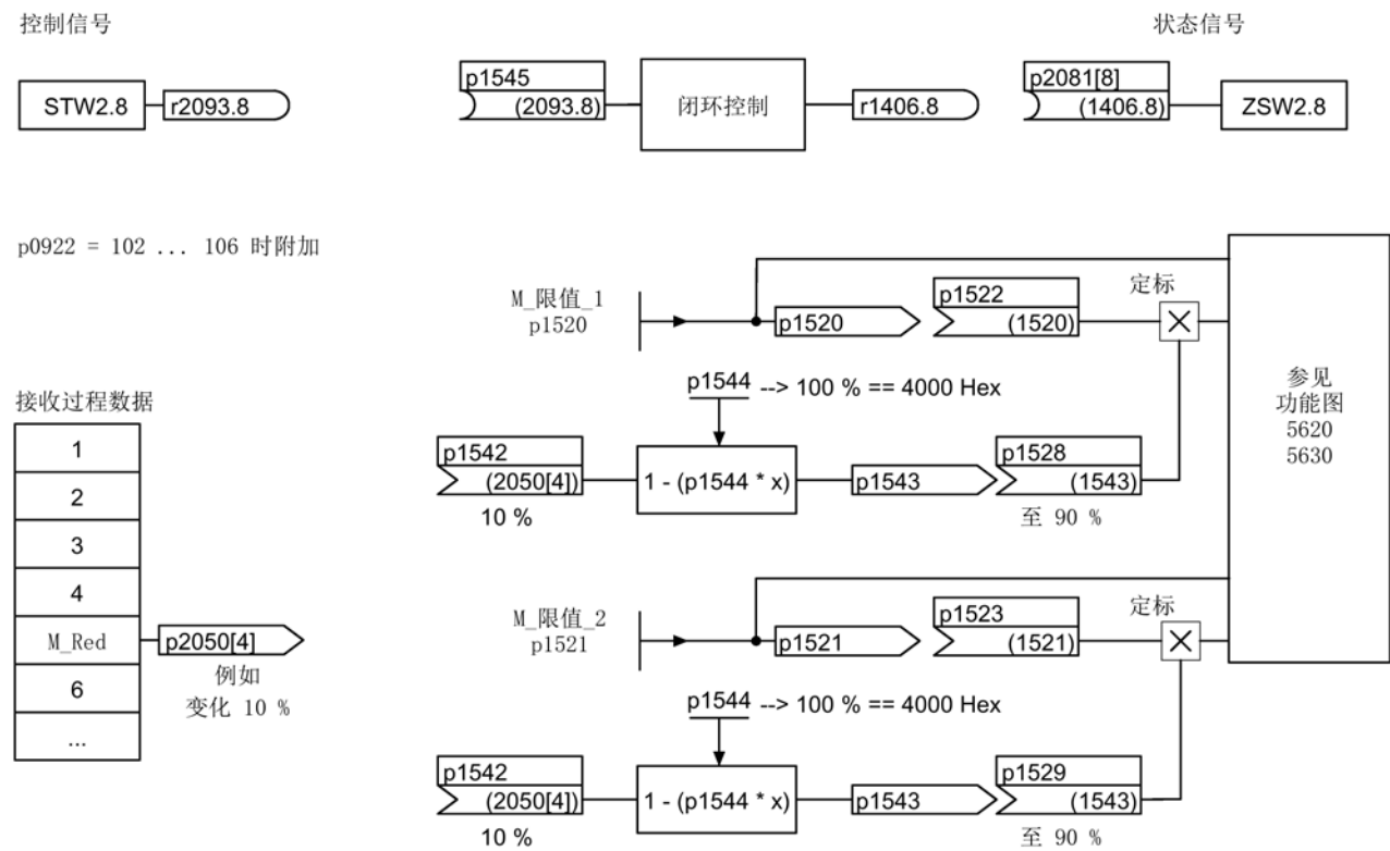
图 4-21 “运行到固定停止点”时的信号
