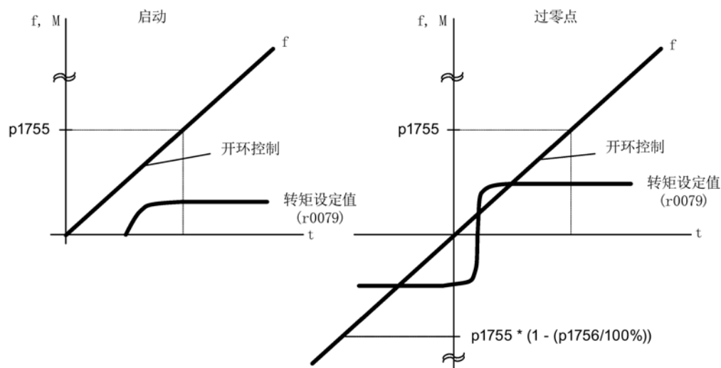
图 5-4 低速区内开环控制中的过零点和启动
