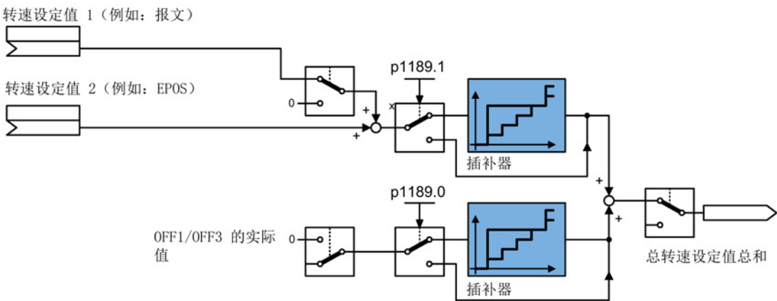
图 4-1 设定值相加
