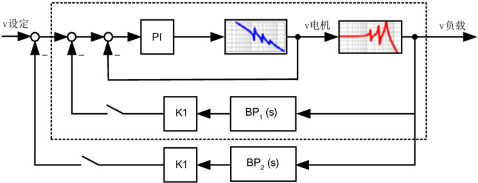
图 8-44 带 2 项 APC 反馈的控制环
