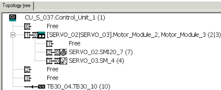
图 13-16 STARTER 中的拓扑结构视图
