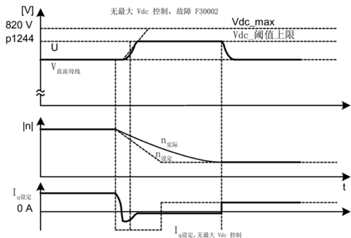
图 4-20 V dc_max 控制的激活/取消
