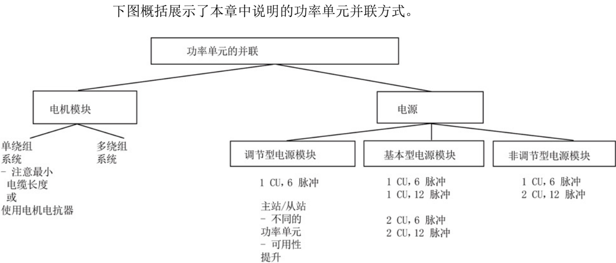
图 8-25 功率单元的并联 - 概览
