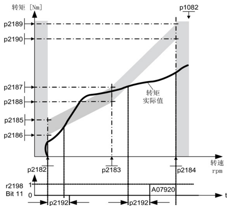
图 8-3 负载监控
