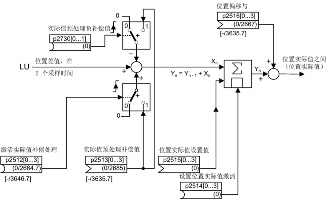
图 8-8 位置实际值处理
