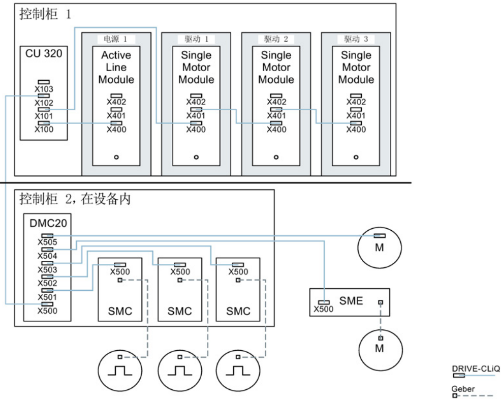
图 12-8 示例：带 DMC20 的分散拓扑结构
