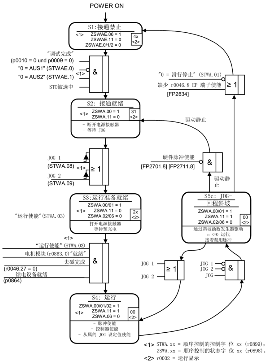
图 3-5 JOG 流程图
