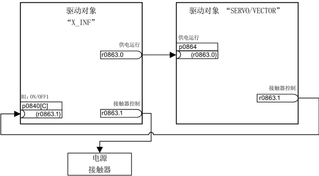
图 12-1 BICO 互联：通过驱动接通电源
