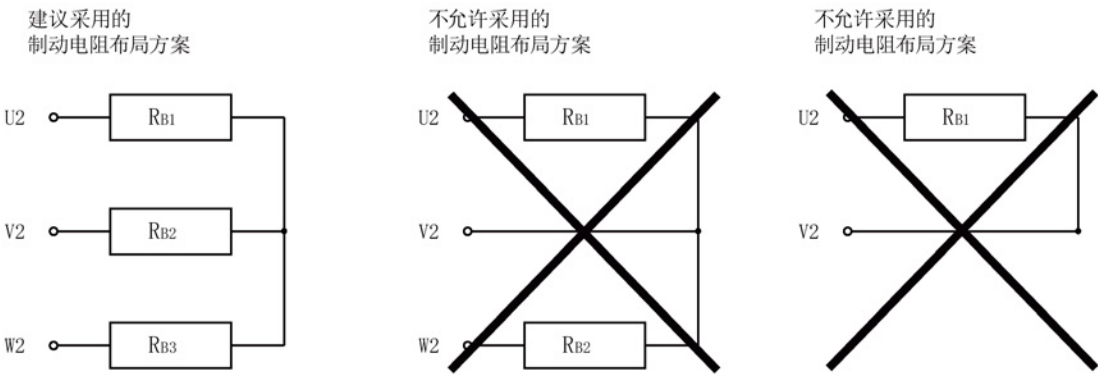
图 7-5 制动电阻
