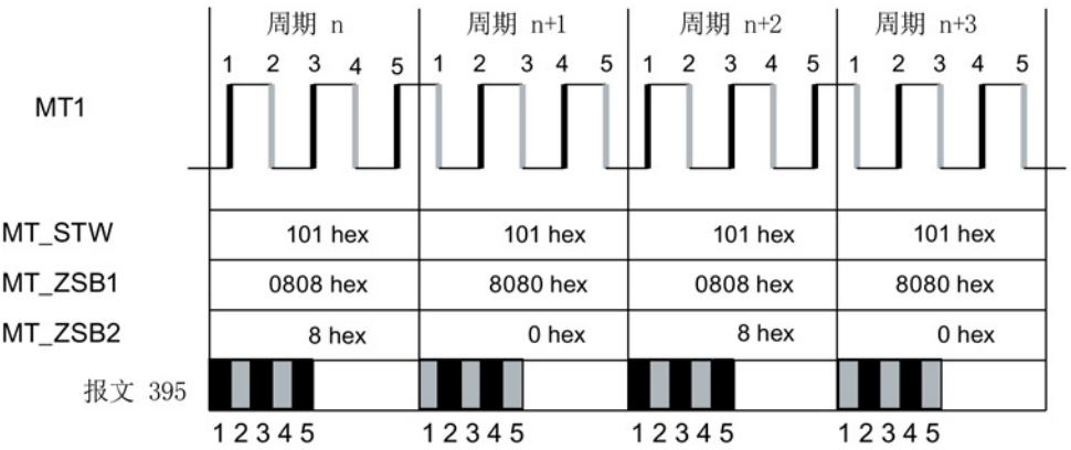
图 4-25 搜索测头 1 的上升沿和下降沿
