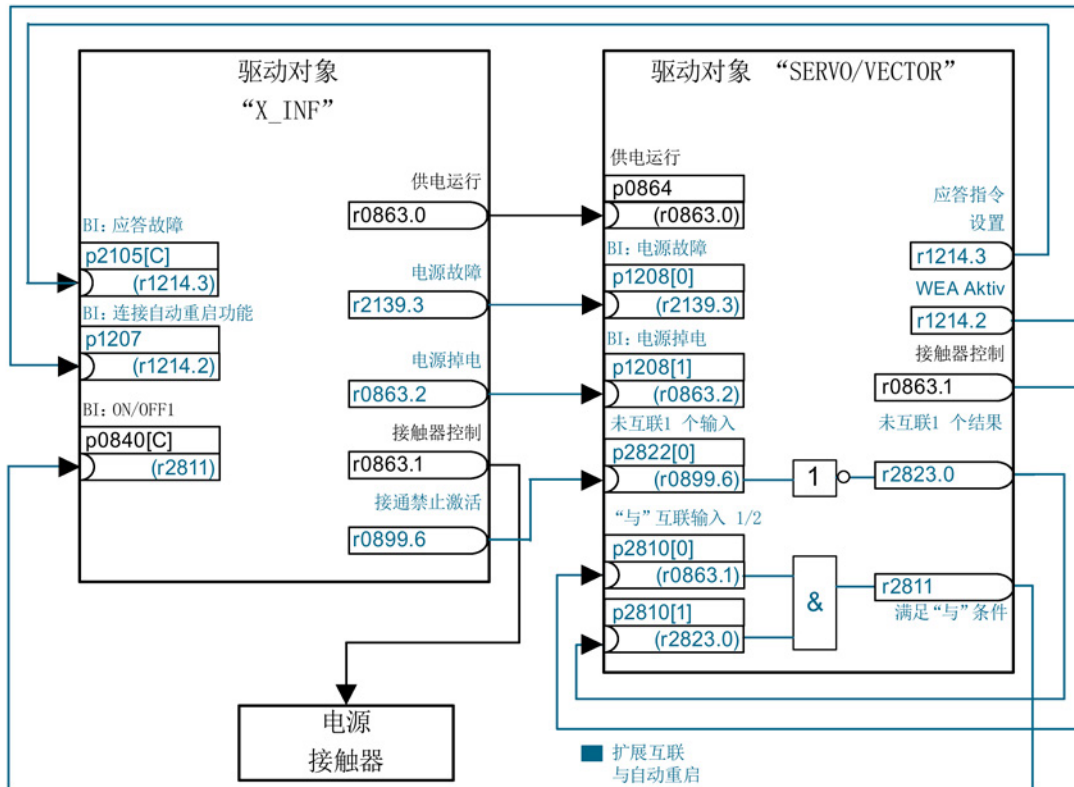
图 12-2 BICO 互联：通过驱动和自动重启接通电源
