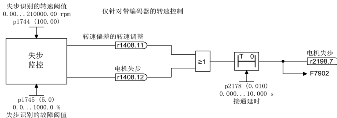
图 9-2 失速保护
