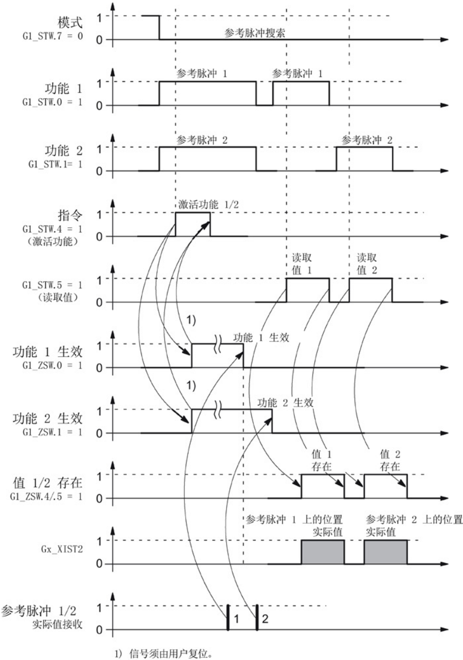
图 11-4 “参考脉冲搜索”功能的时序图
