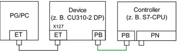
图 11-30 含 PG/PC 的以太网/PROFINET 拓扑结构
