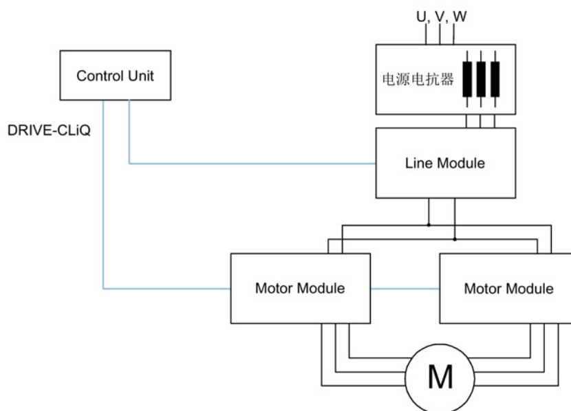
图 8-26 示例 1：并联
