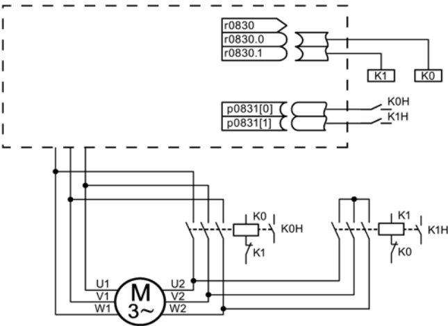
图 12-7 星形/三角形切换示例
