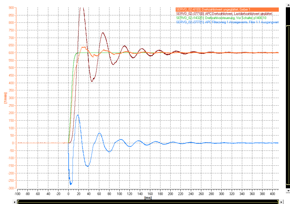
图 8-35 定位特性：不带 APC
