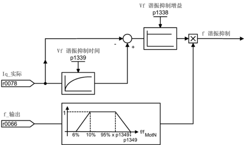
图 6-6 谐振抑制
