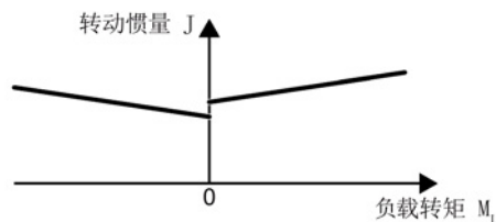
图 8-32 转动惯量前馈控制
