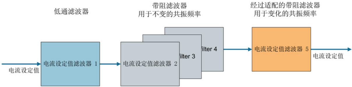
图 4-12 示例：电流设定值滤波器 5 是级联中最后使用的滤波器
