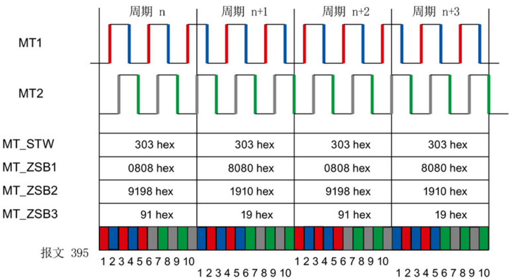
图 4-26 搜索测头 1 和 2 的上升沿和下降沿
