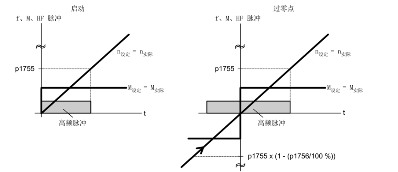
图 5-5 “零速前一直保持闭环控制”中的过零点
