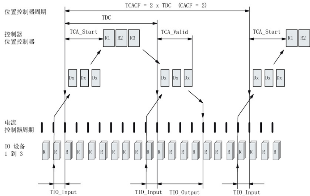
图 11-32 采用 PROFINET 的运动控制/等时同步驱动耦合，周期经过优化，CACF（Controller Application Cycle Factor，控制器应用循环系数）= 2
