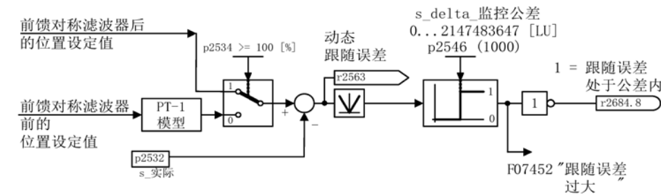
图 8-11 跟随误差监控
