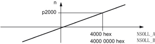
图 11-2 转速定标
