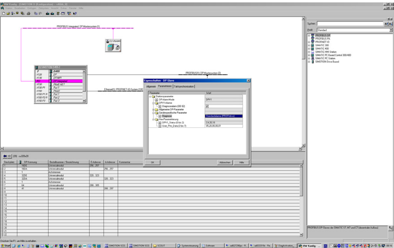
图 11-28 激活 PROFIBUS
