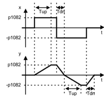
图 3-8 使用基本斜坡函数发生器时的斜坡上升/下降时间
