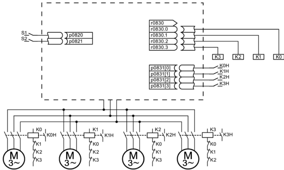
图 12-6 电机切换的示例
