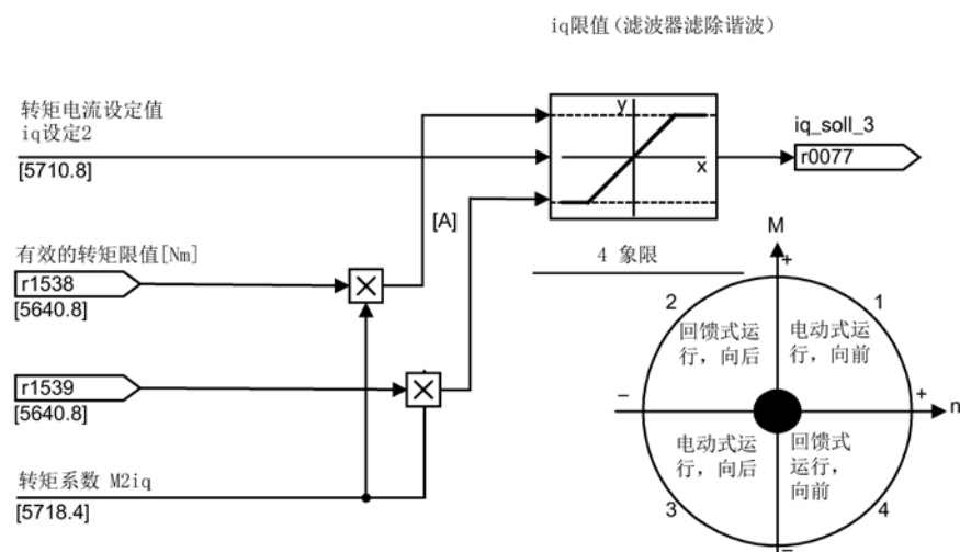
图 4-7 电流设定值限制/转矩设定值限制
