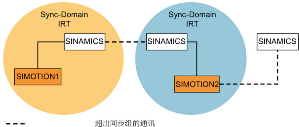
图 11-31 超出同步组极限实现实时同步
