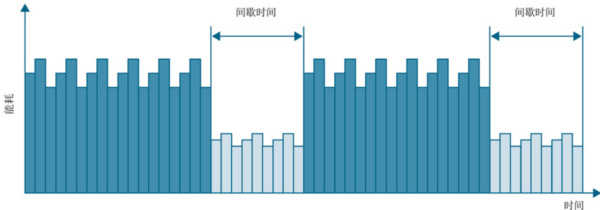
图 11-51 PROFlenergy 停机节能
