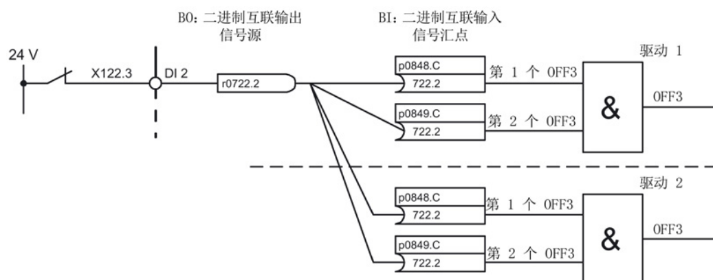
图 13-8 “OFF3”互联到多个驱动（示例）
