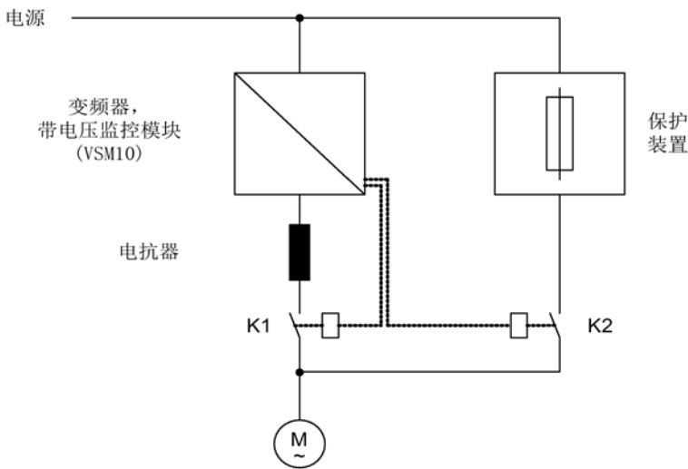
图 5-25 电路示例：带同步和重叠的旁路
