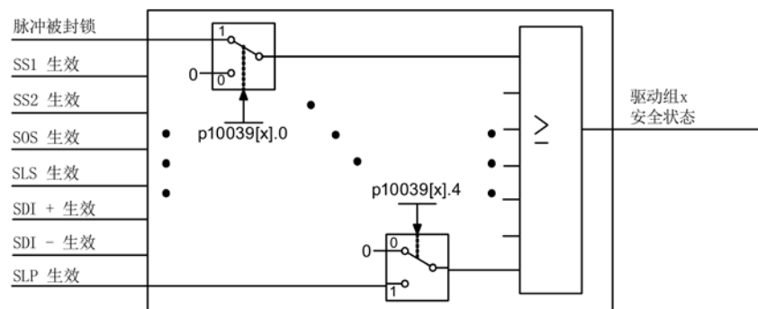
图 10-5 安全状态选择（扩展功能示例）
