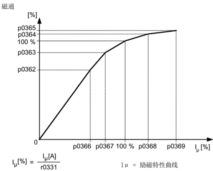
图 5-20 励磁特性曲线
