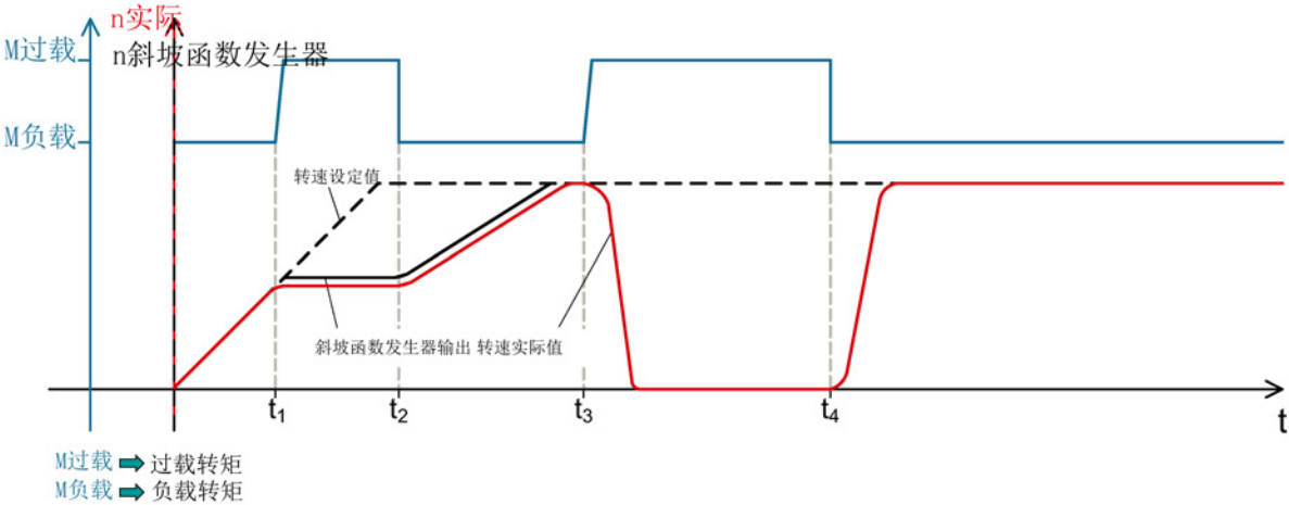
图 3-11 斜坡函数发生器跟踪标准
