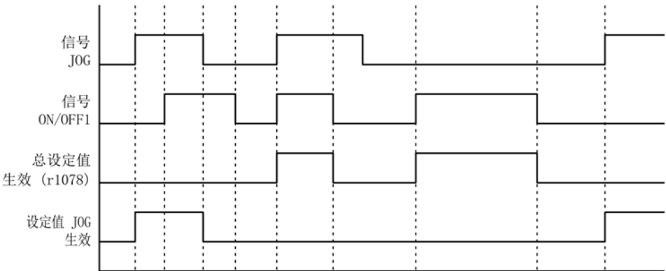
图 3-3 JOG 和 OFF1 的流程图
