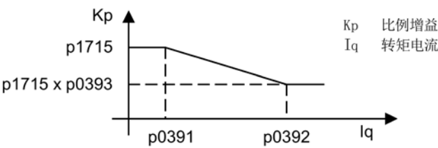
图 4-10 电流控制器适配
