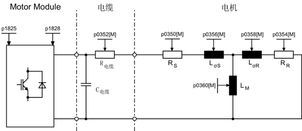
图 4-17 异步电机和电缆的等效电路图
