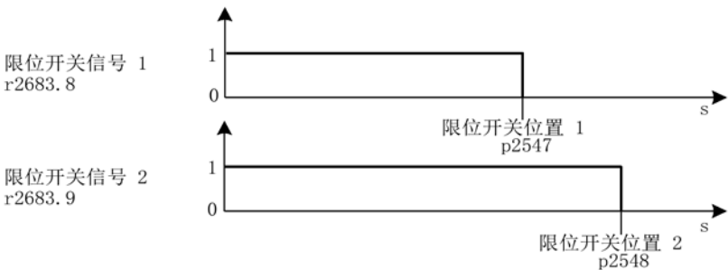
图 8-12 限位开关
