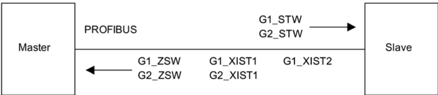
图 11-3 编码器接口示例（编码器 1：2 个实际值，编码器 2：1 个实际值）
