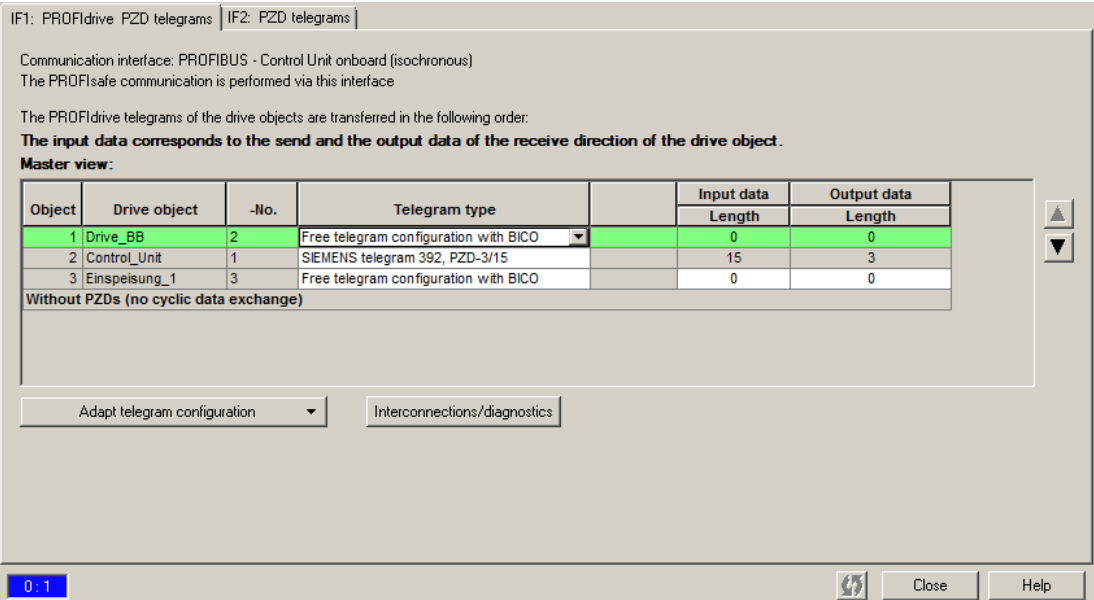
图 11-1 PZD 报文
