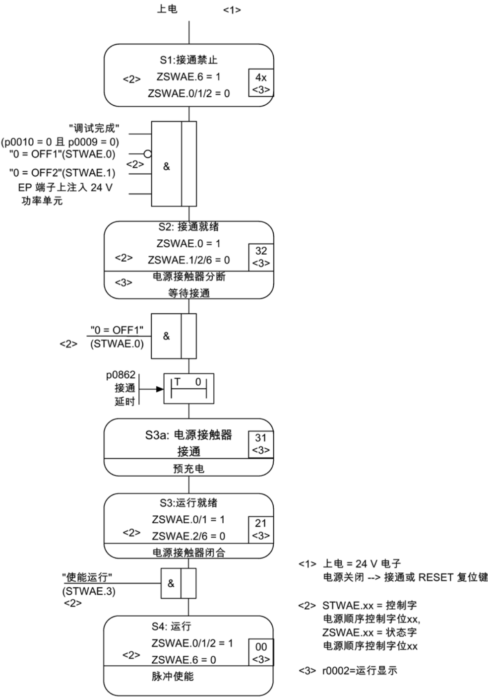
图 2-6 非调节型电源的启动过程
