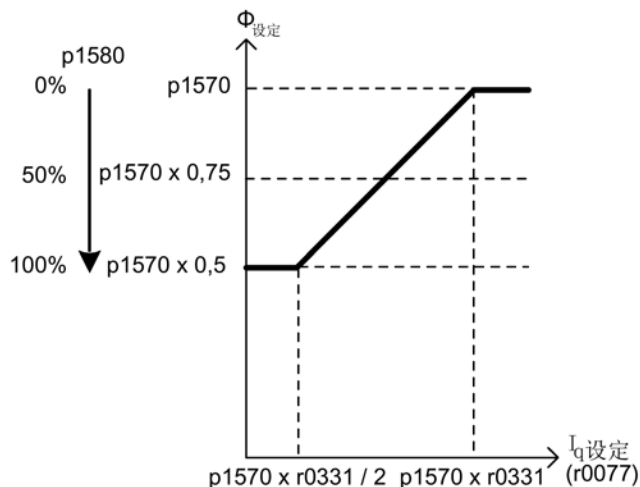
图 5-21 效率优化
