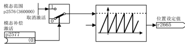
图 8-14 模态补偿
