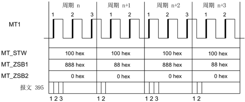
图 4-24 搜索测头 1 的上升沿
