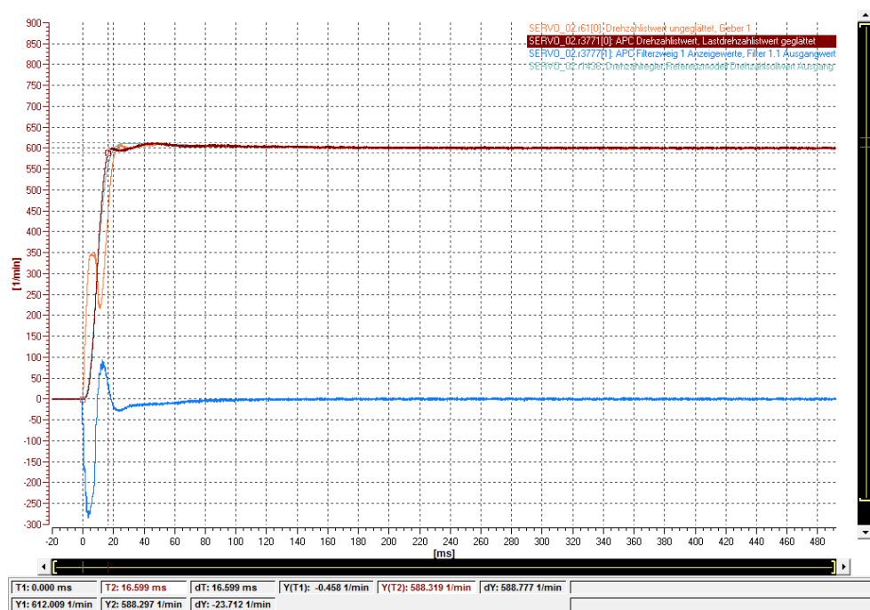
图 8-36 定位特性：APC 完美设置
