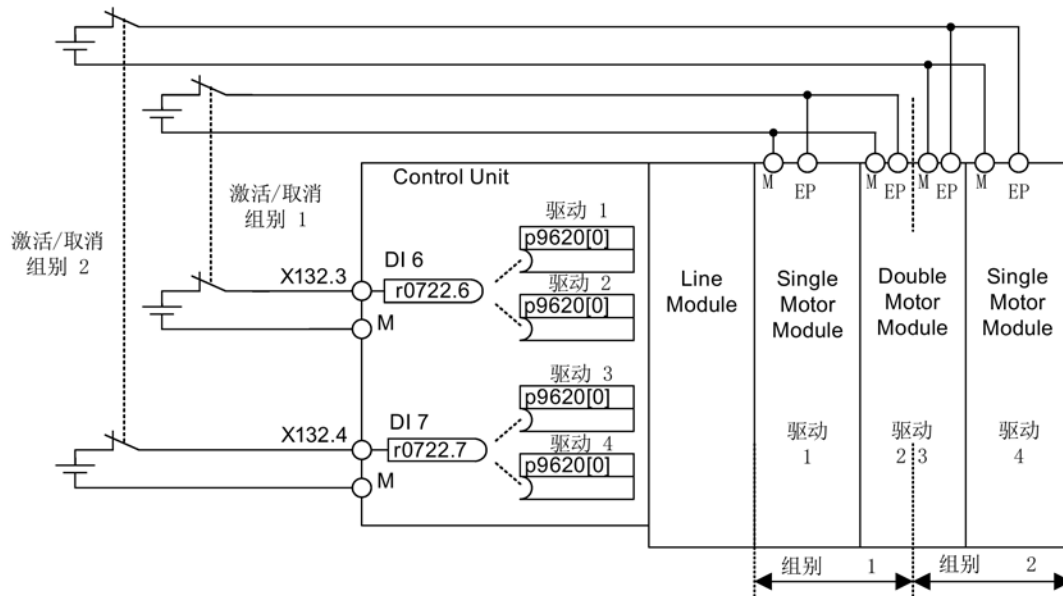
图 10-3 示例：端子分组：以书本型电机模块和 CU320-2 为例
