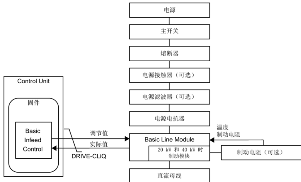
图 2-7 书本型基本型电源的结构框图
