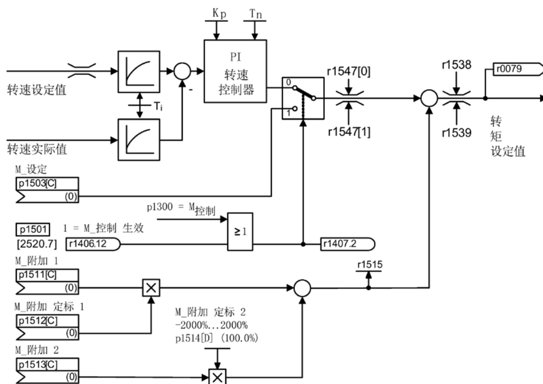
图 5-13 转速/转矩控制
