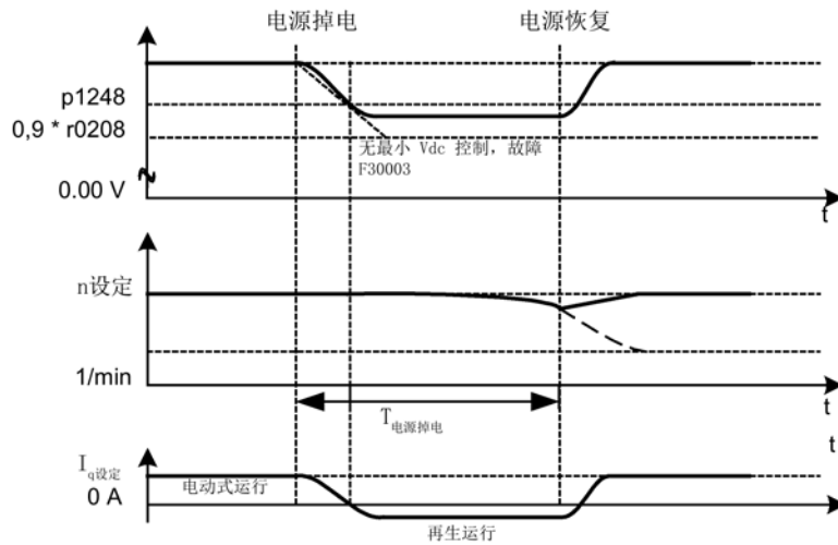
图 4-19 V dc_min 控制（动能缓冲）的激活/取消
