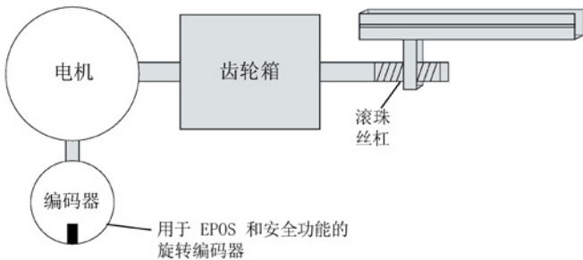
图 8-22 举例 3: EPOS和安全回参考点, 线性
