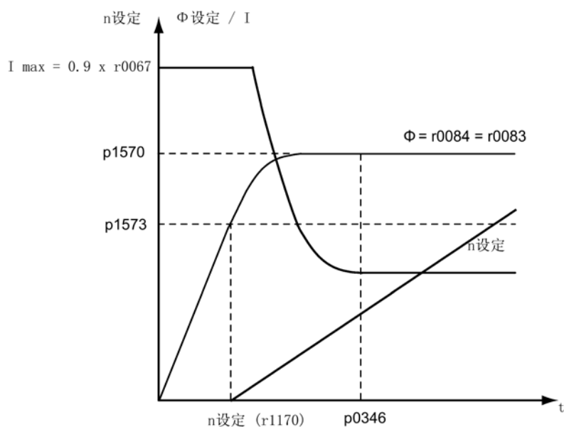
图 5-22 快速励磁的特性曲线
