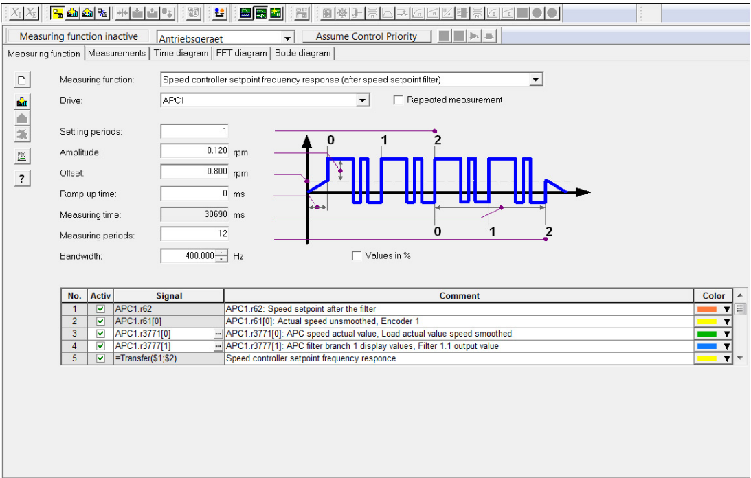
图 8-47 测量函数和信号
