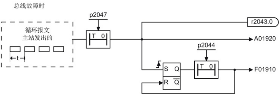
图 11-15 总线故障时的报文故障监控
