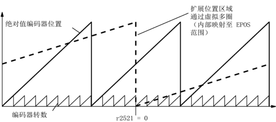
图 8-9 位置跟踪(p2721 = 24)、设置 p2504 = p2505 = 1 (传动比 = 1)
