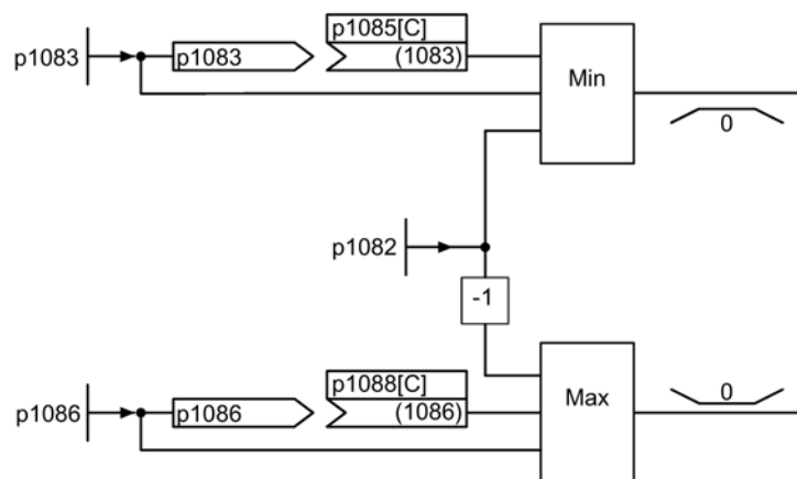
图 4-3 转速控制器限制
