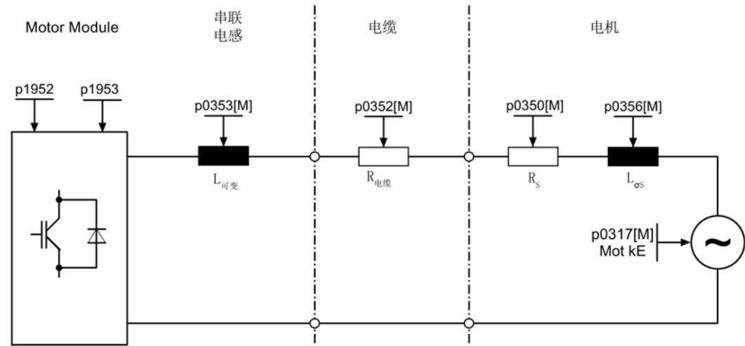
图 4-18 同步电机和电缆的等效电路图
