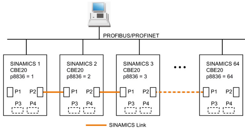
图 11-54 最大拓扑结构
