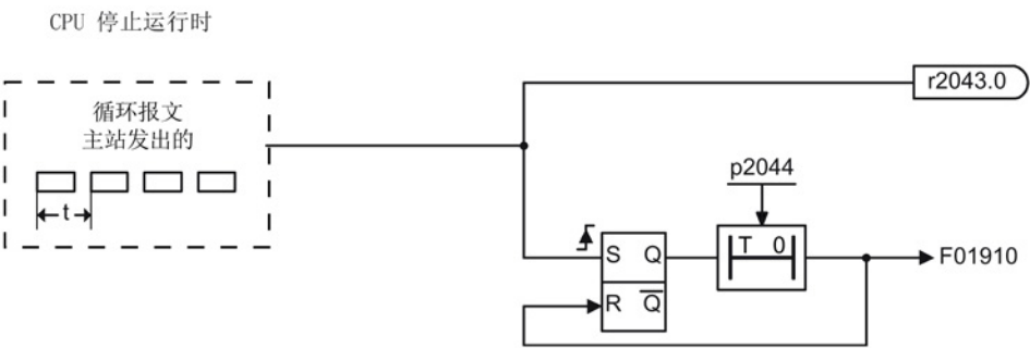
图 11-16 CPU 停止时的报文故障监控
