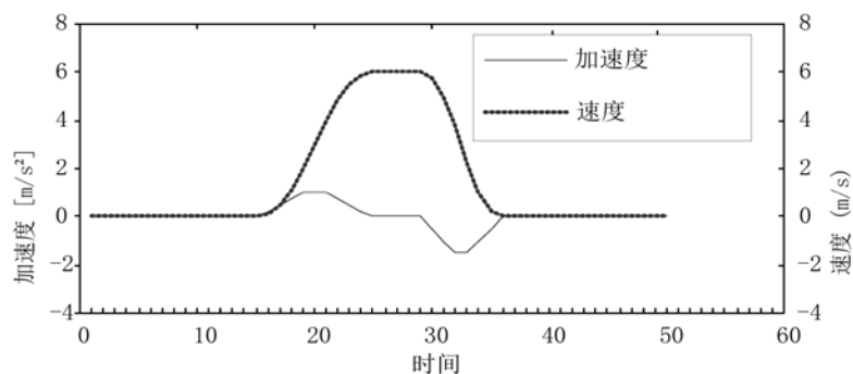
图 8-16 激活的加加速度限制
