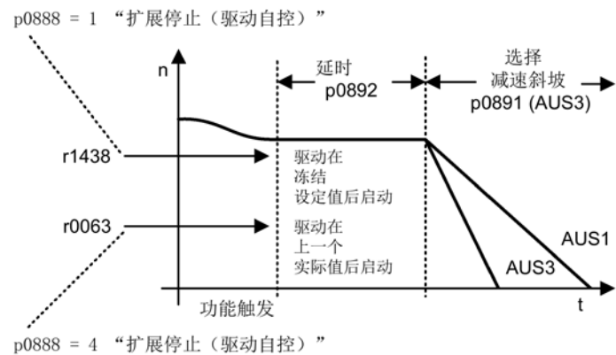
图 8-28 包含延时段 OFF 斜坡
