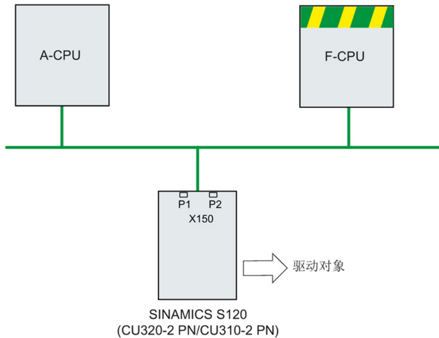
图 11-34 PROFINET 拓扑结构概览
