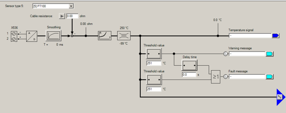
图 9-3 温度传感器/通道的平滑时间
