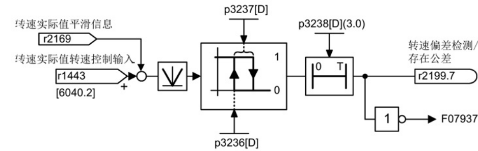
图 5-12 “模型/外部转速差”公差监控
