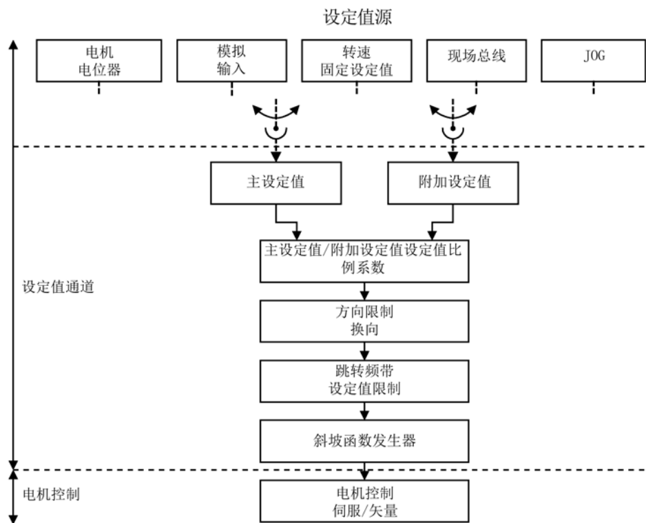
图 3-1 扩展的设定值通道
