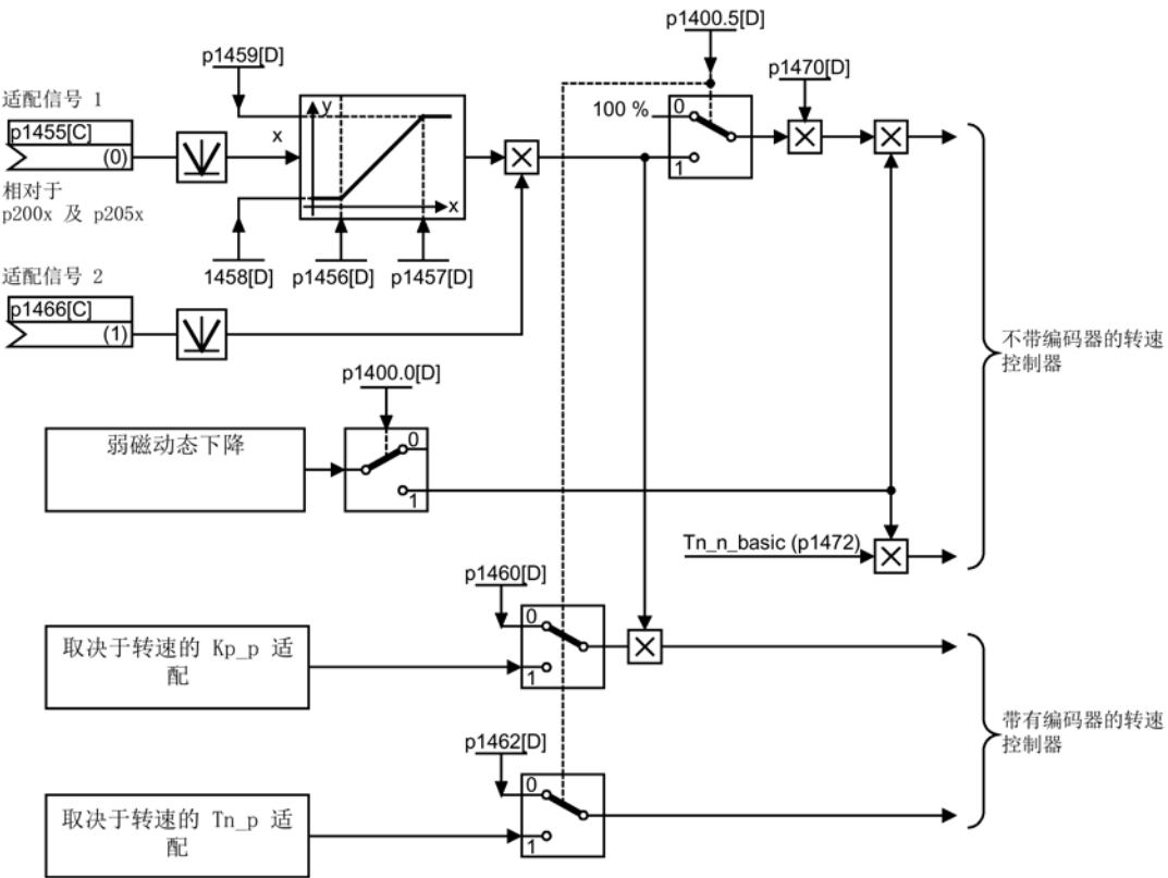
图 4-4 自由 K_{p\_n} 适配
