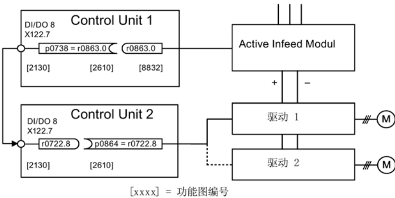
图 12-4 示例：多个控制单元的互联
