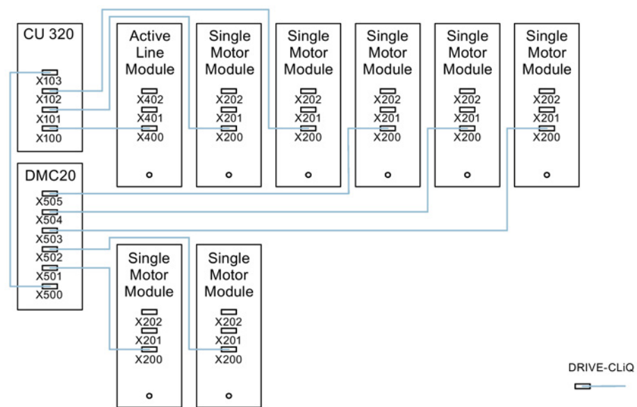
图 12-9 示例：矢量 V/f 控制中热插拔的拓扑结构
