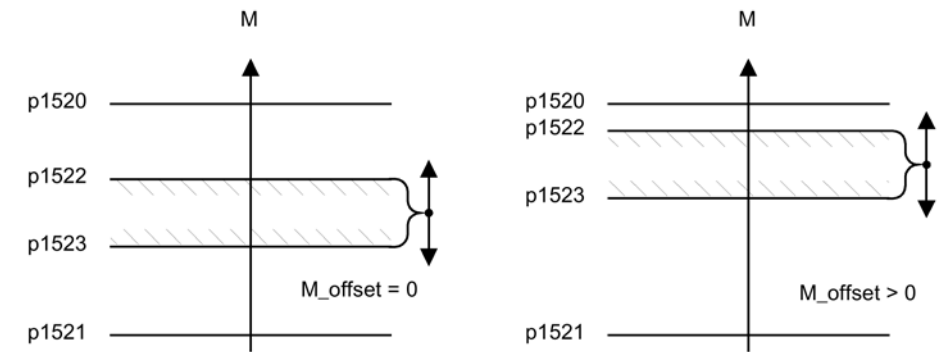
图 4-8 示例：带或不带偏移的转矩极限
