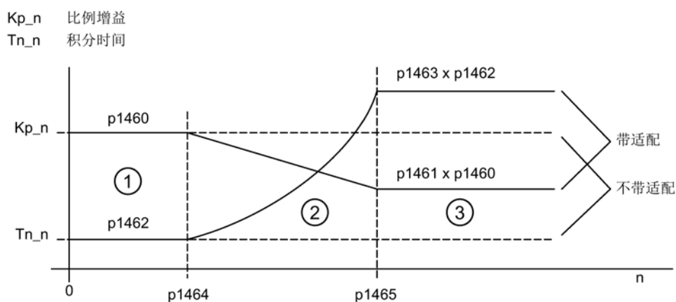
图 4-5 转速控制器 K_{p\_n}/T_{n\_n} 适配
