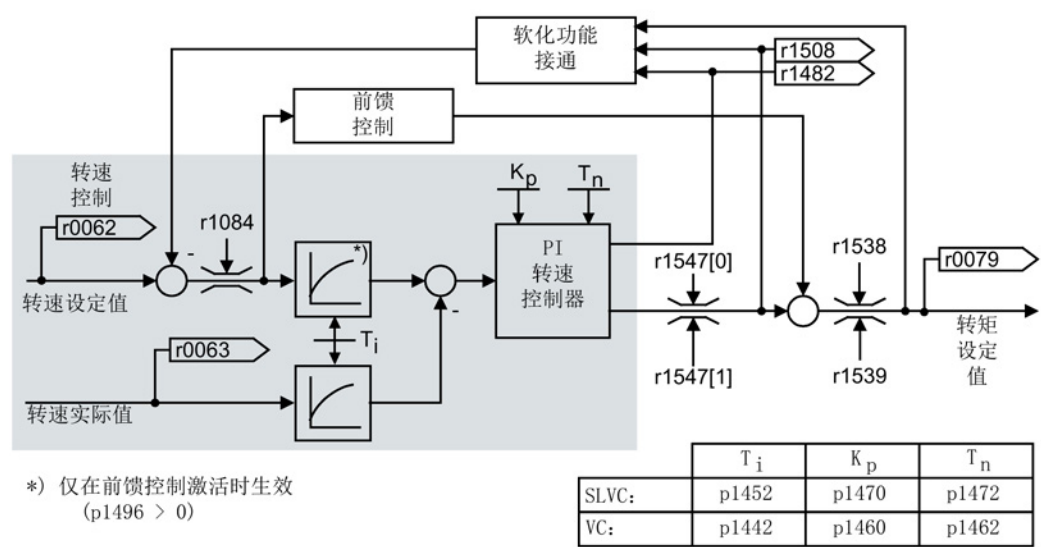
图 5-6 转速控制器
