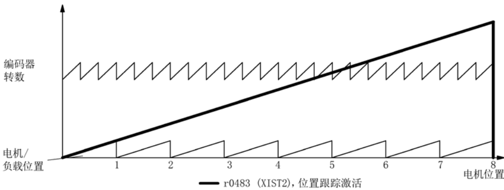
图 7-16 奇数传动比，有位置跟踪(p0412 = 8)
