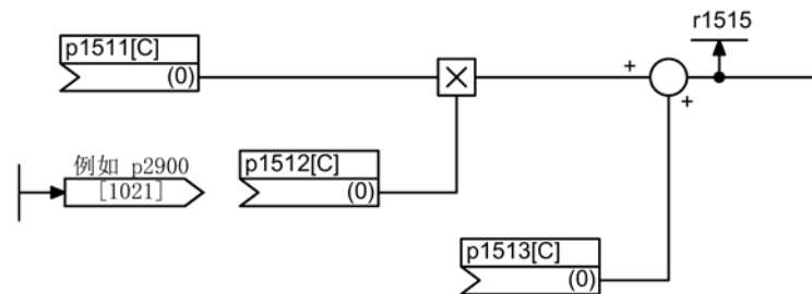
图 4-6 转矩设定值
