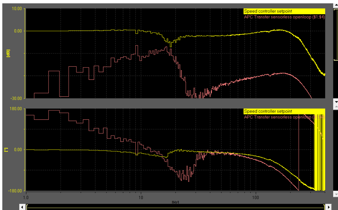
图 8-33 APC，无负载侧传感器（p3700 = 4）- 开环
