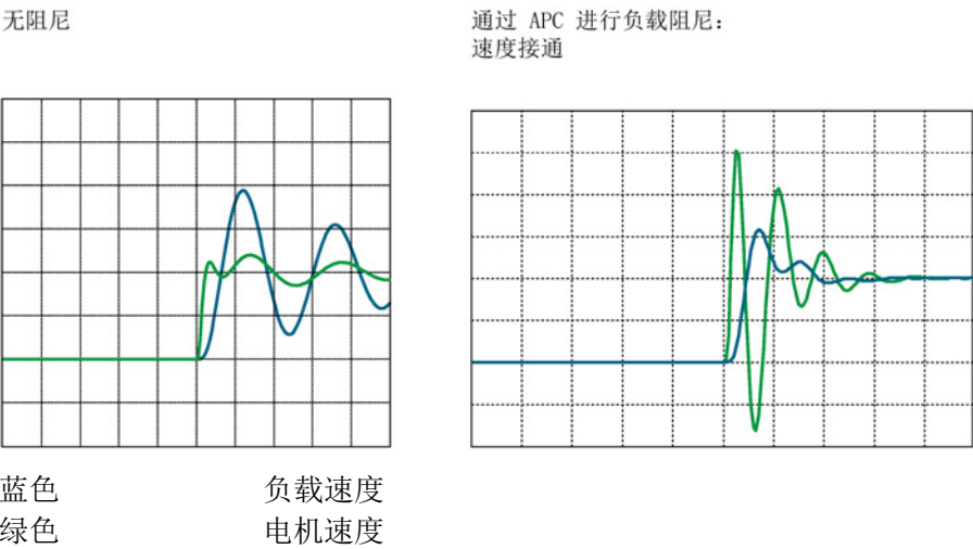
图 8-46 带速度接通的 APC（示例）
