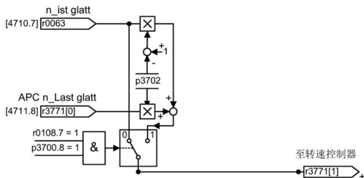
图 8-37 APC 编码器混合
