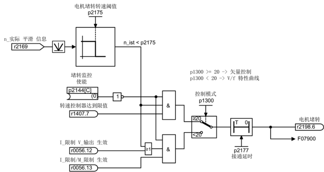
图 9-1 堵转保护
