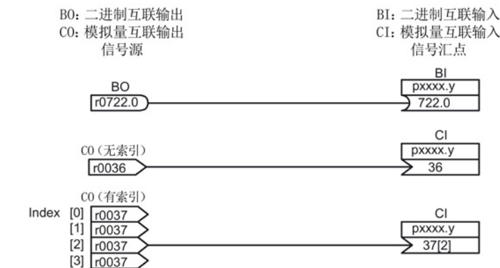
图 13-5 使用 BICO 技术互联信号
