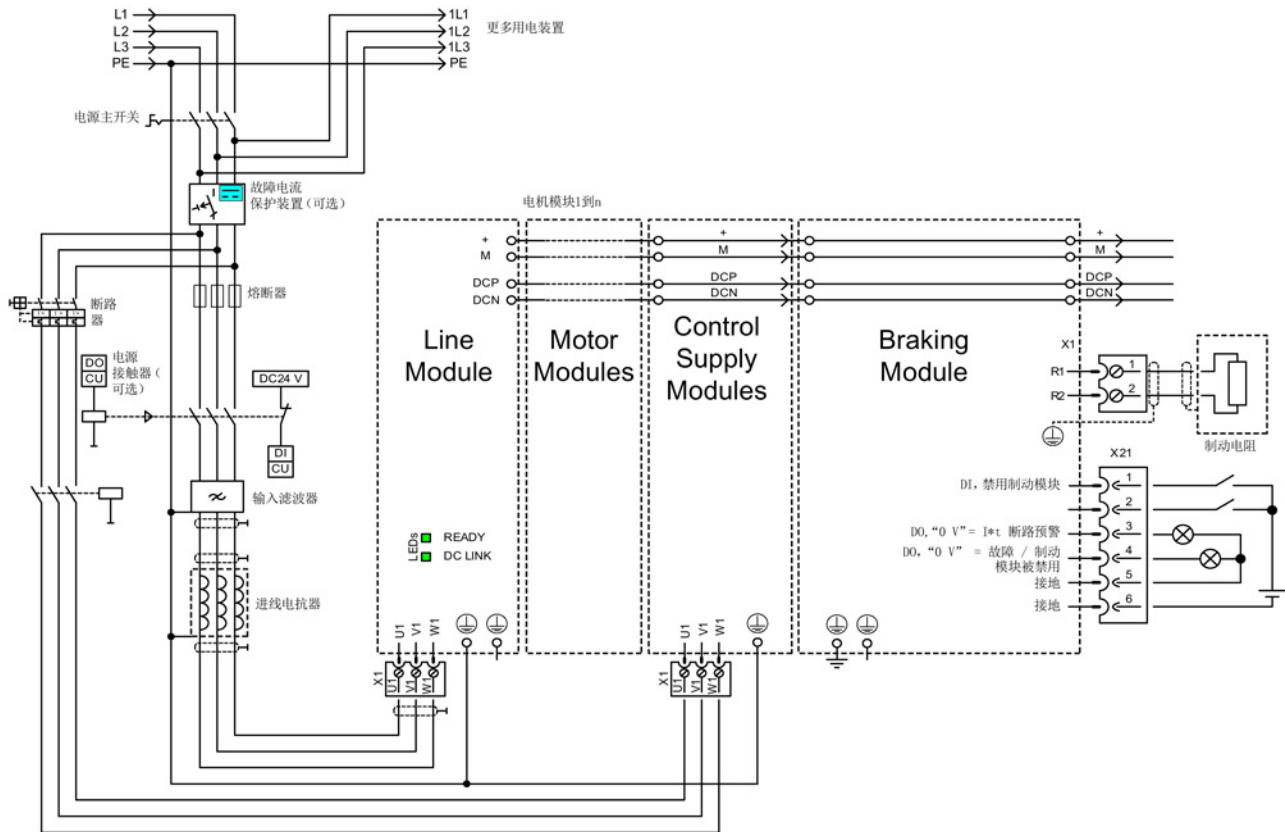
图 12-5 电源断电时紧急停止或紧急切断的连接示例
