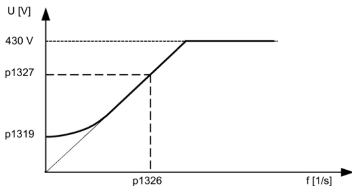
图 4-14 V/f 特性曲线
