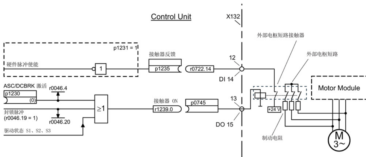
图 7-4 外部电枢短路制动示例
