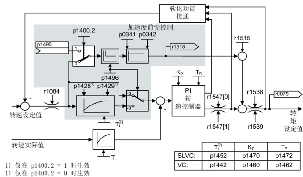
图 5-9 带前馈控制的转速控制器
