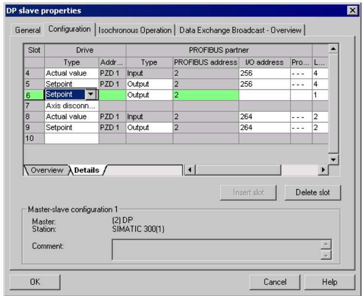
图 11-23 插入新的槽
