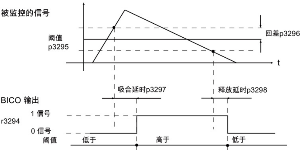
图 4-23 变量报告功能
