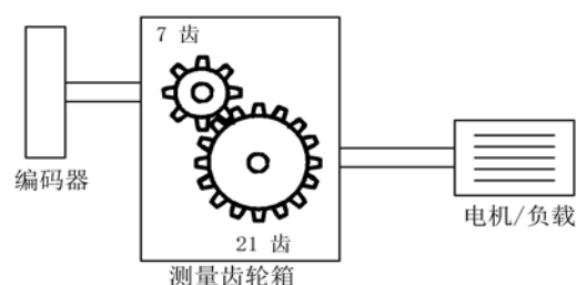
图 7-14 测量齿轮箱
