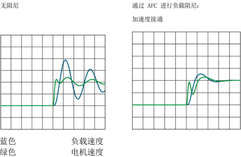
图 8-43 带加速度接通的 APC（示例）
