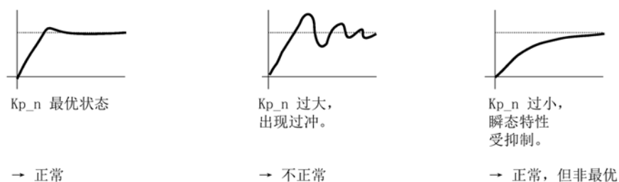
图 4-15 设置比例增益 K_p
