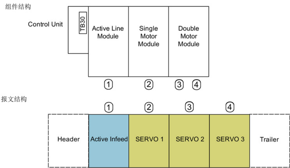
图 11-11 组件结构和报文结构
