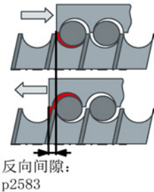
图 8-13 反向间隙补偿
