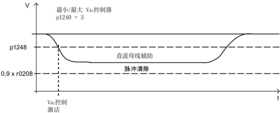
图 8-31 直流母线电压设定值
