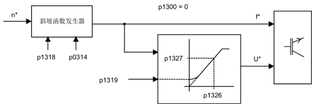
图 4-13 V/f 控制的结构
