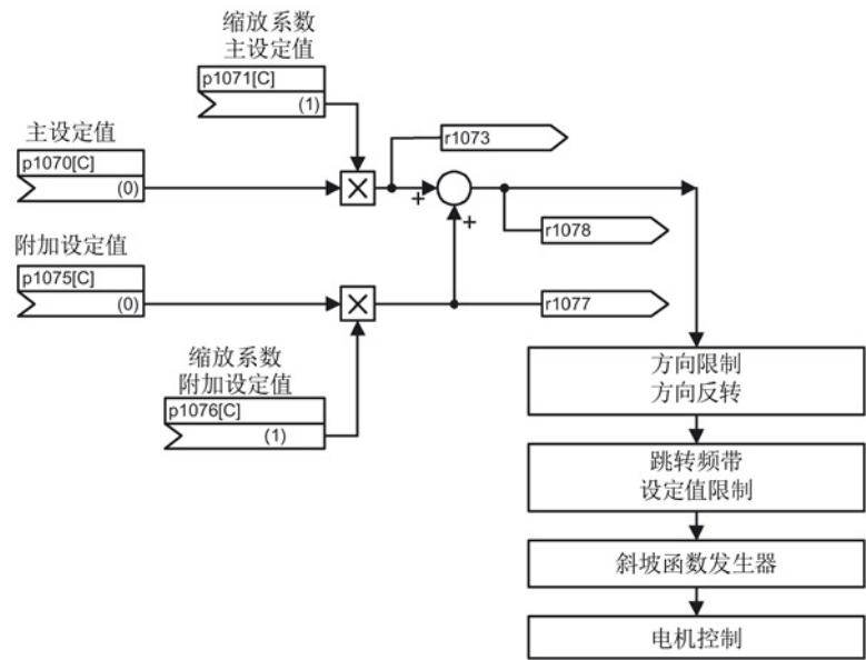
图 3-2 设定值相加，设定值比例系数
