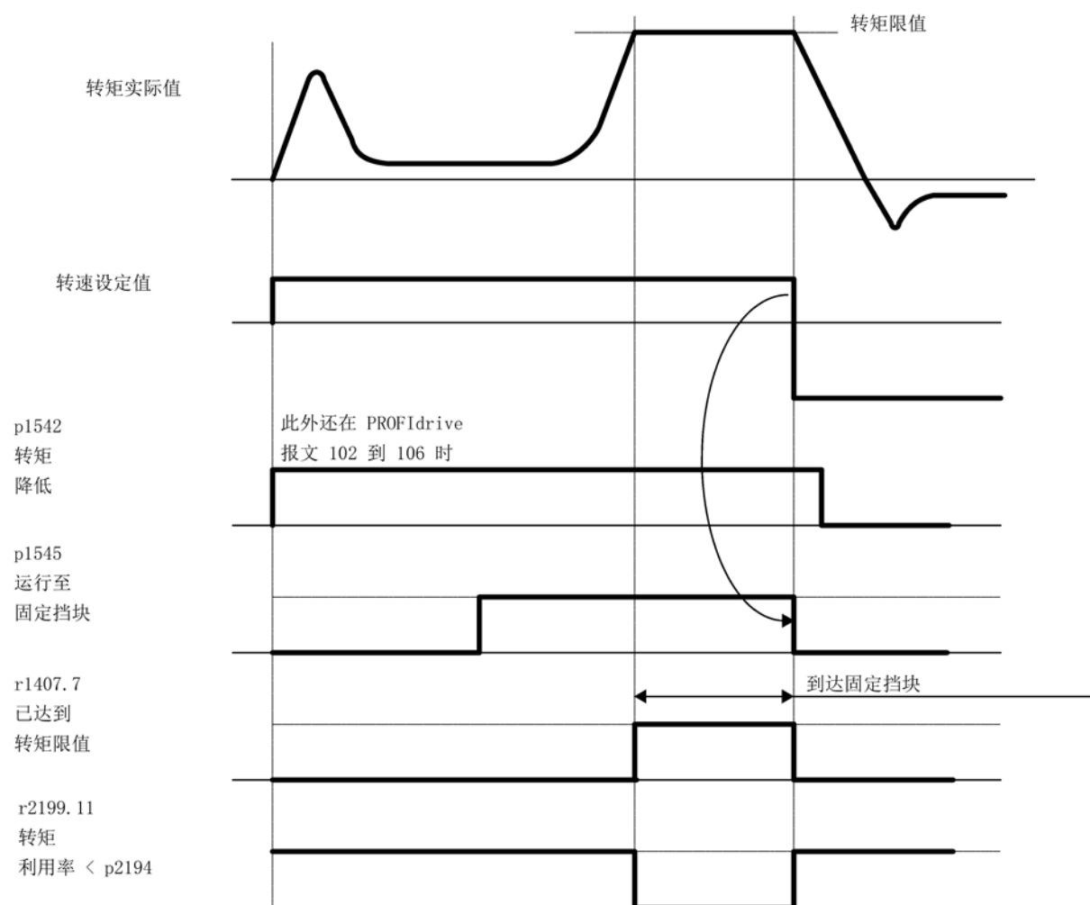
图 4-22 “运行到固定停止点”时的信号图
