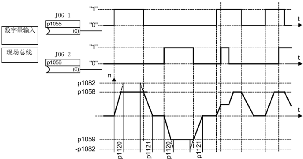
图 3-4 JOG 1 和 JOG 2 的流程图
