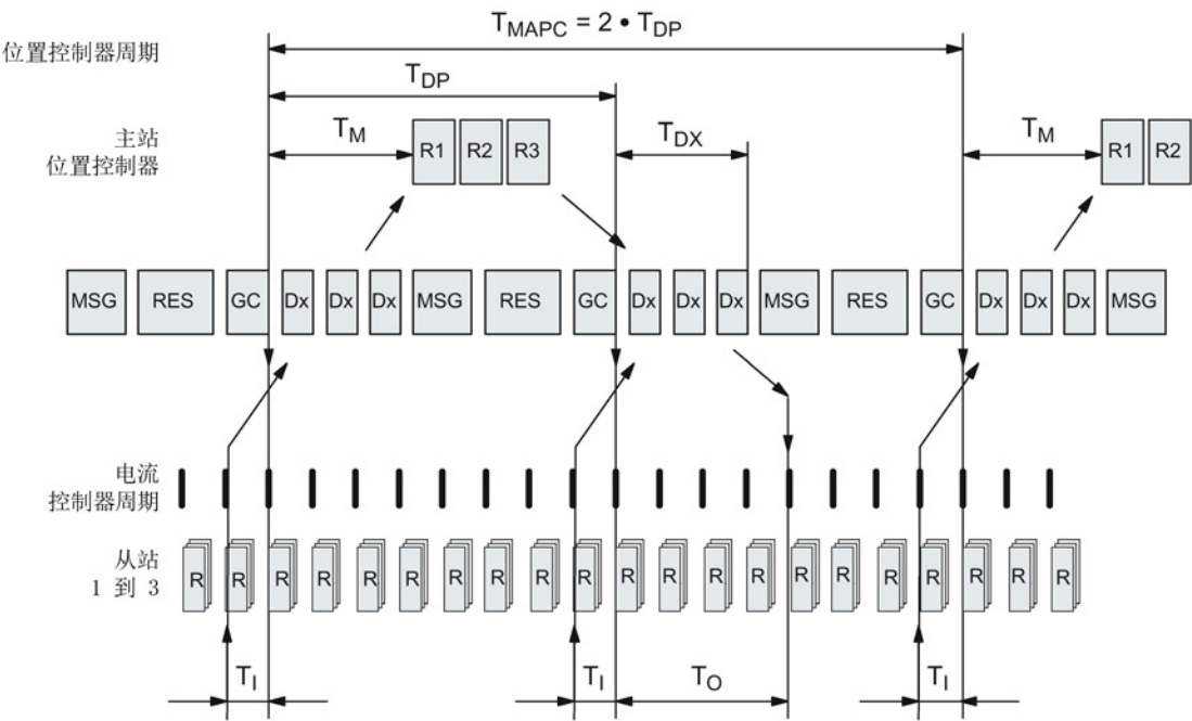
图 11-17 采用 PROFIBUS 的运动控制/等时同步驱动耦合，周期经过优化， T_{MAPC} = 2 \cdot T_{DP}
