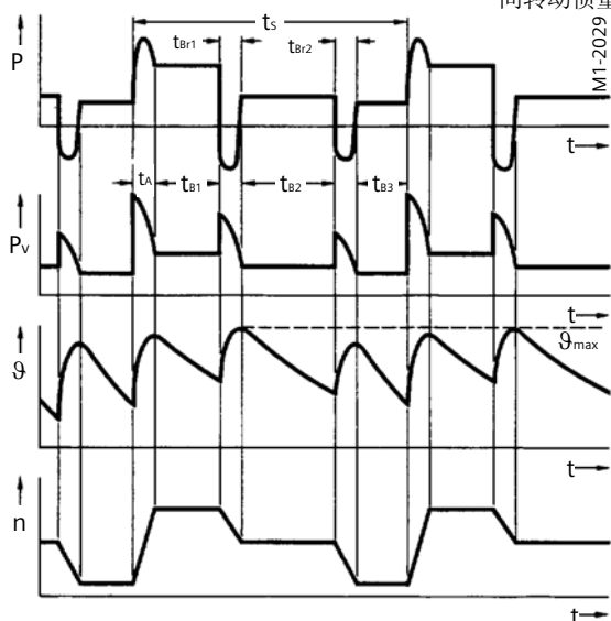
工作制 S8: 连续运行周期工作制，相关的负载/转速有变化
