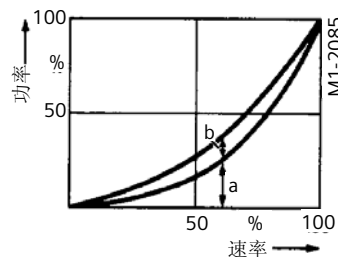
b. 功率损耗 在平方规律负载转矩下由于转速控制产生的起动可变电阻器损耗
