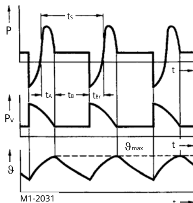
工作制 S7: 连续运行周期工作制，有起动和电制动
