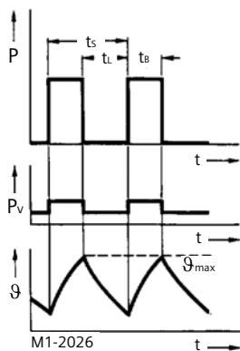
工作制 S6: 连续运行周期工作制
