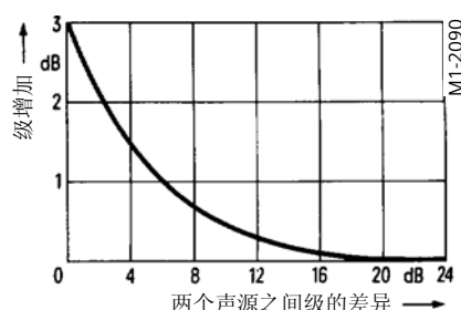
■ 两个不同级声源声功率级 L_{pA} 的增加。
