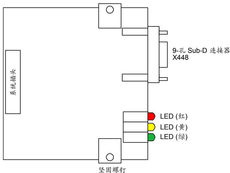
图 8.2-1 通讯板外观
