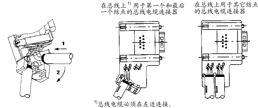
图 8.2-11 连接总线电缆到总线连接器
