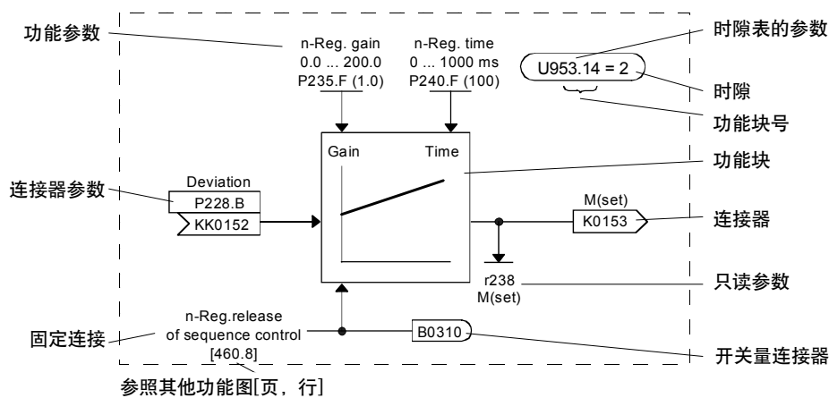
图 4-1 一个功能块
