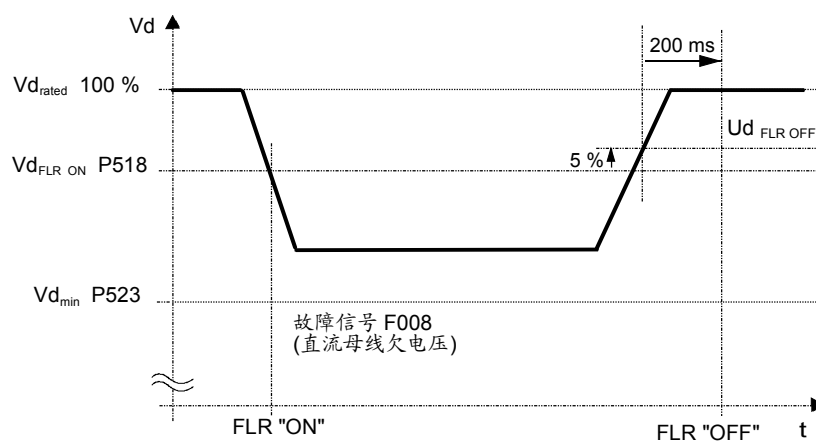
图 7-3 柔性响应
