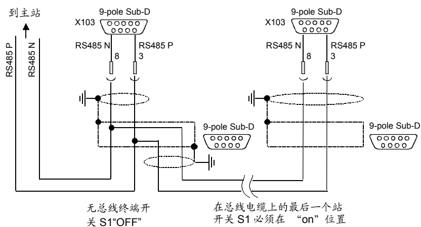
图 8.1-15 端子 X103 (增强书本型)2 线总线电缆连接
