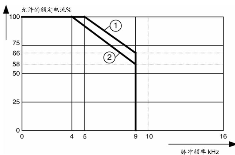
图 7-8 降额曲线
