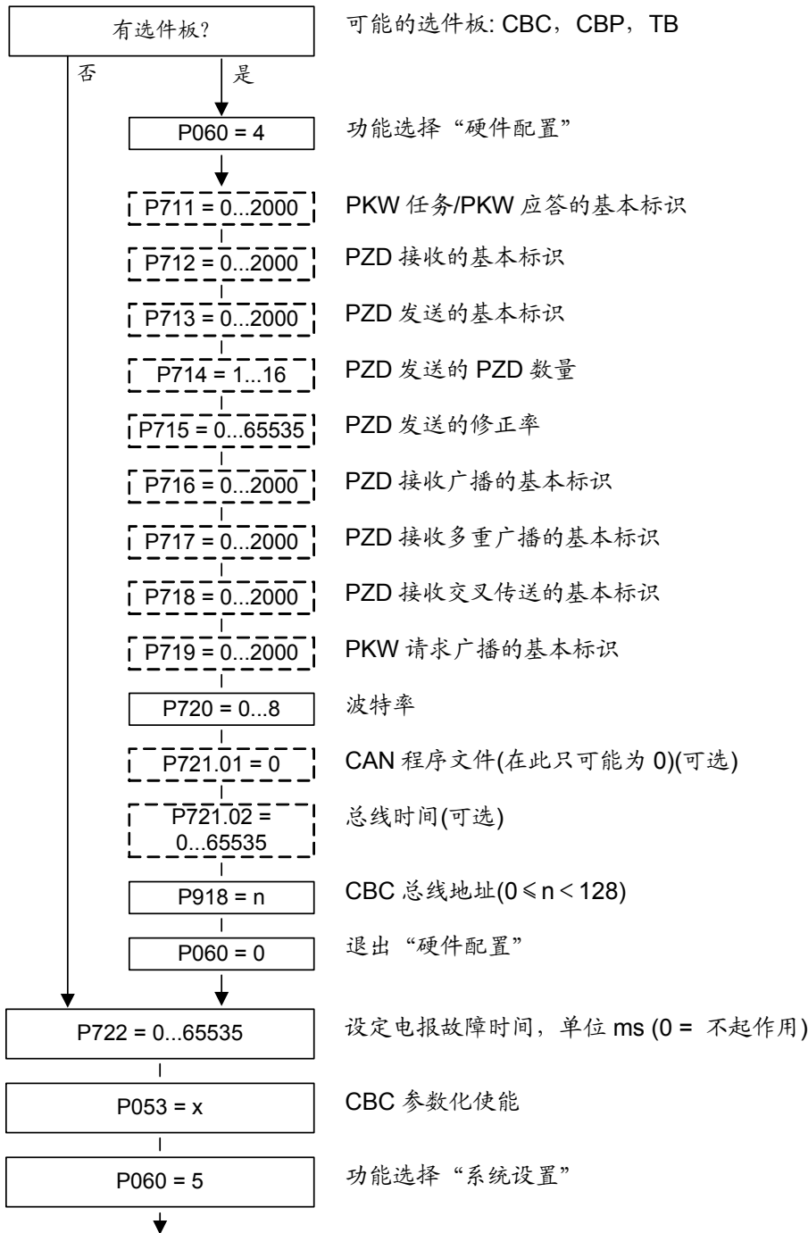
图 8.4-16 带 CUPM, CUMC 或 CUVC 的 MASTERDRIVES “硬件配置” 的参数化
