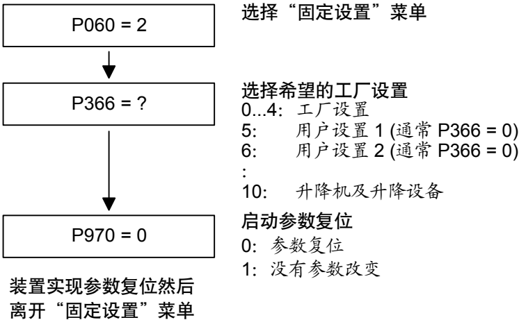
图 6-3 用用户的设定进行参数设置的顺序
