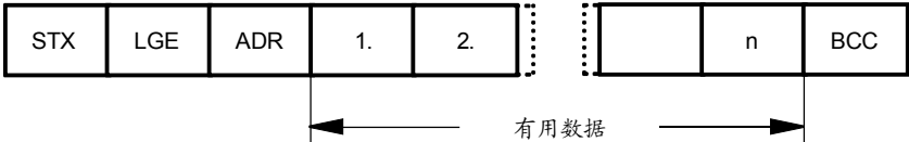
图 8.1-2 电报结构
