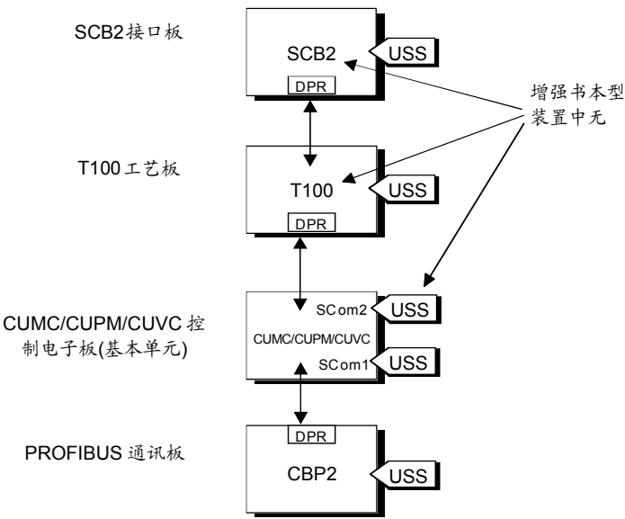
图 8.1-8 接口综述
