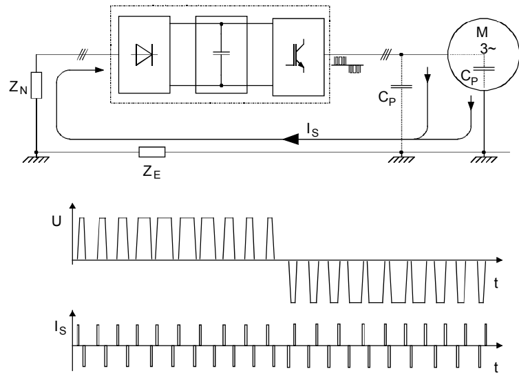
图 3-2 输出电压 V 和故障电流 I_S 的波形图
