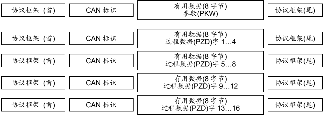
图 8.4-2 CAN 协议电报中的有用数据结构
