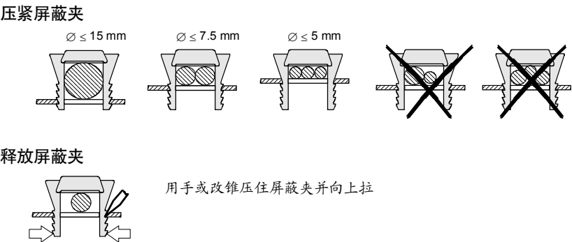
图 8.2-16 使用屏蔽夹
