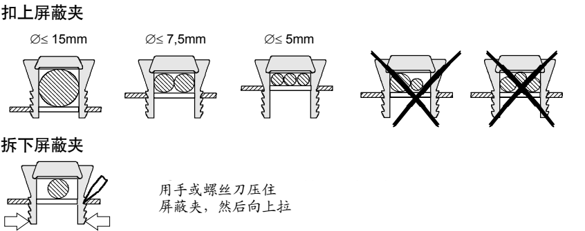
图 8.4-9 使用屏蔽夹
