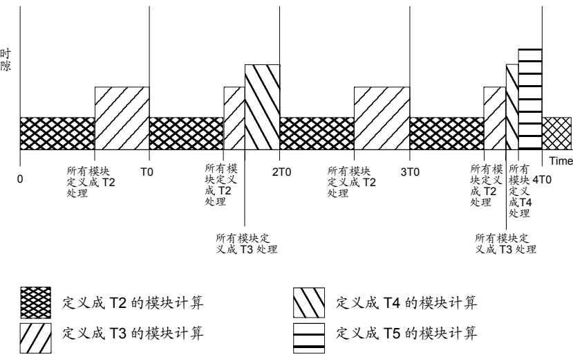
图 7-1 时隙处理顺序
