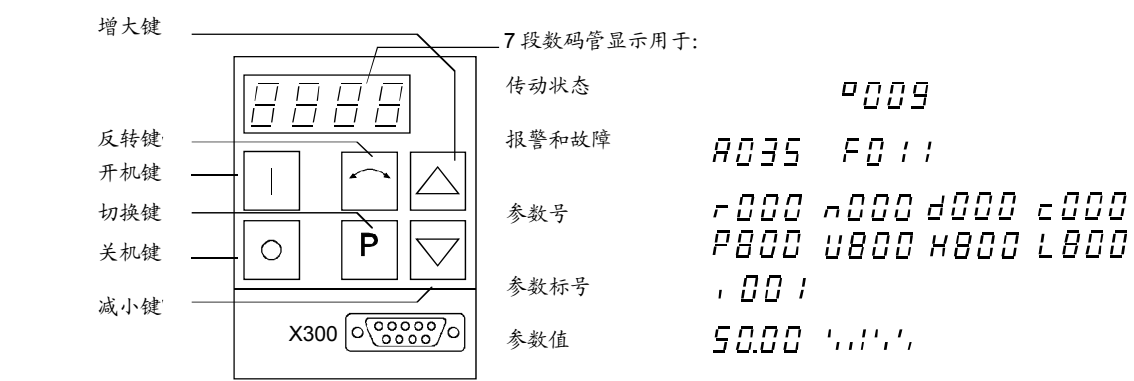
图 5-3 PMU 参数设置单元
