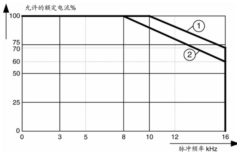
图 7-7 降额曲线
