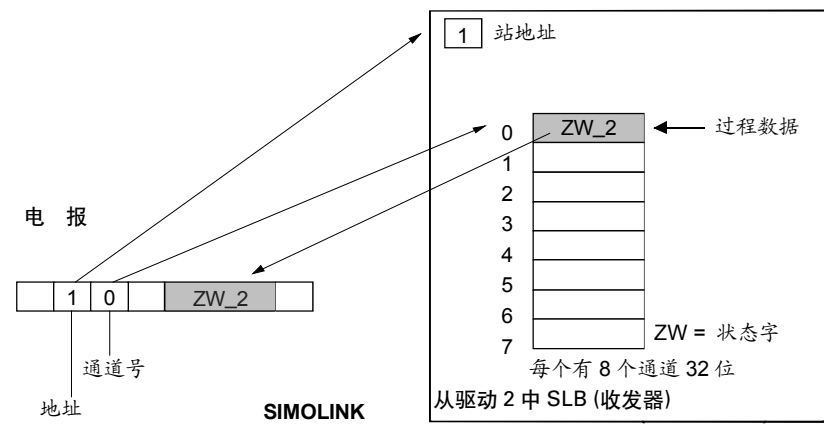
图 8.3-11 从驱动 2，写数据
