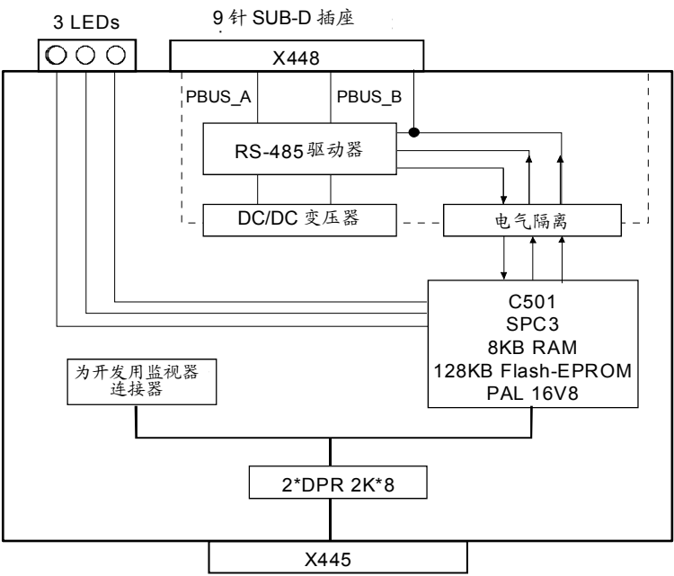
图 8.2-26 CBP 框图
