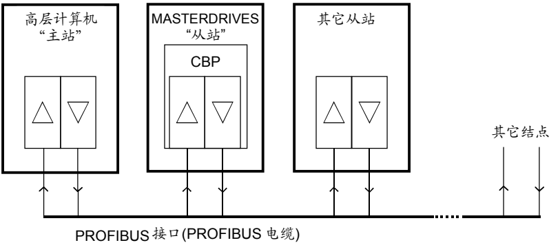
图 8.2-2 PROFIBUS 接口
