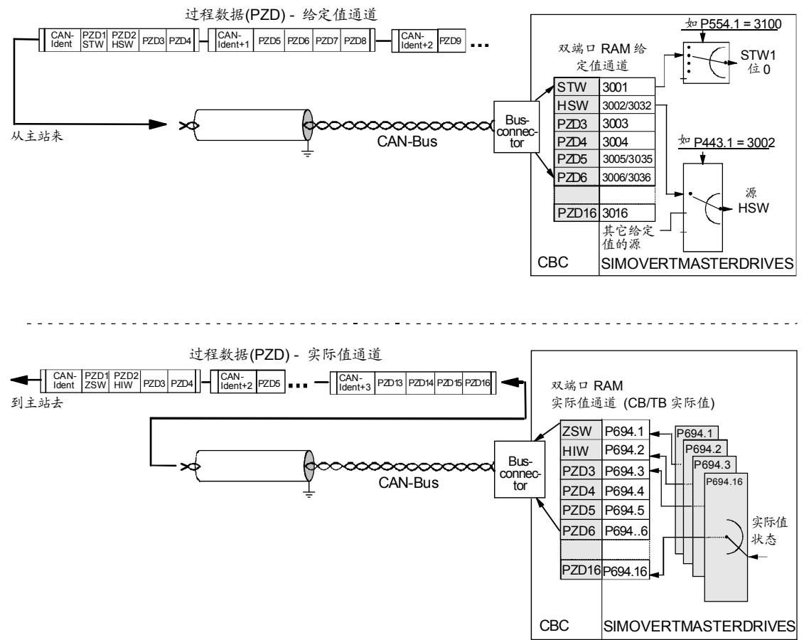
图 8.4-20 功能类型 CU1, CU2 或 CU3 的过程数据内部连接示例
