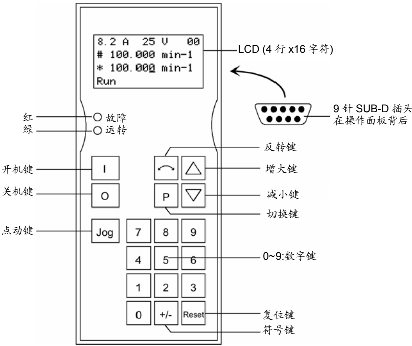
图 5-5 OP1S 正视图
