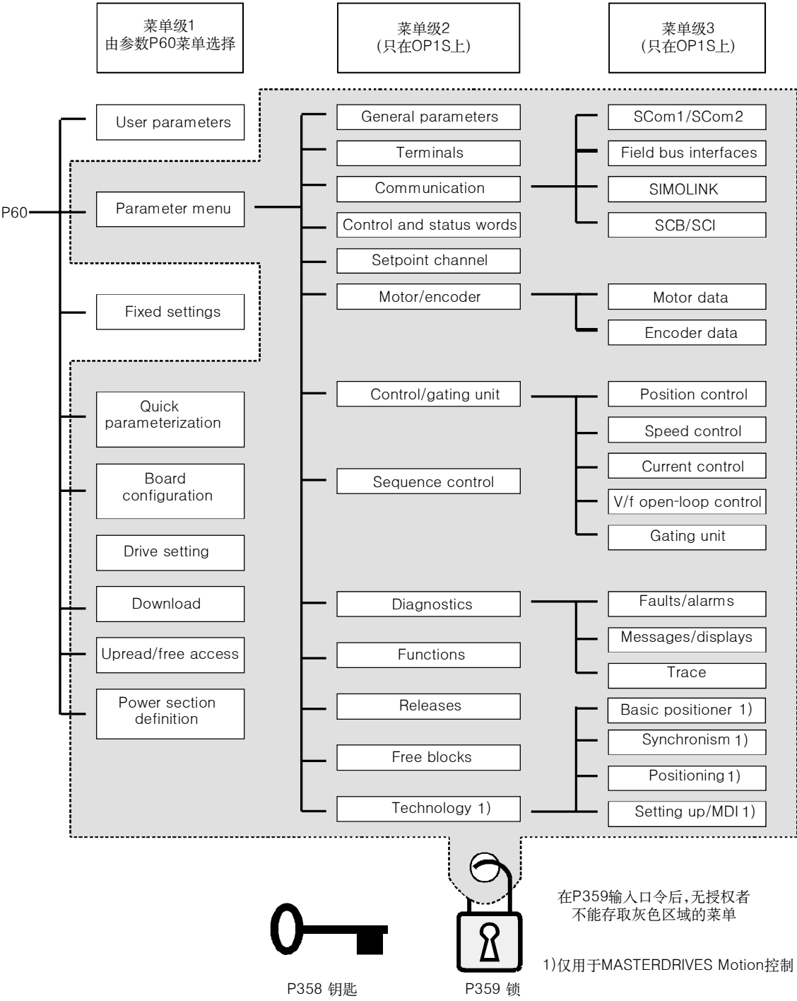
图 8-1 参数菜单
