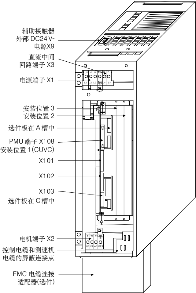
图 7-1 规格 A, B 和 C 的接线简图
