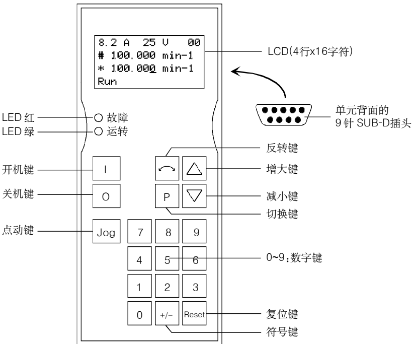
图 8-15 OP1S 正视图
