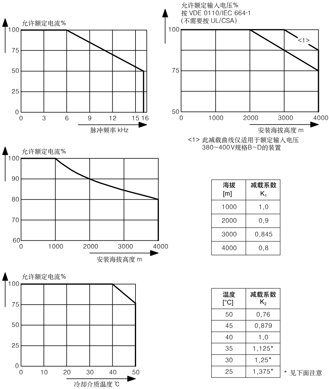
图 13-1 减载曲线
