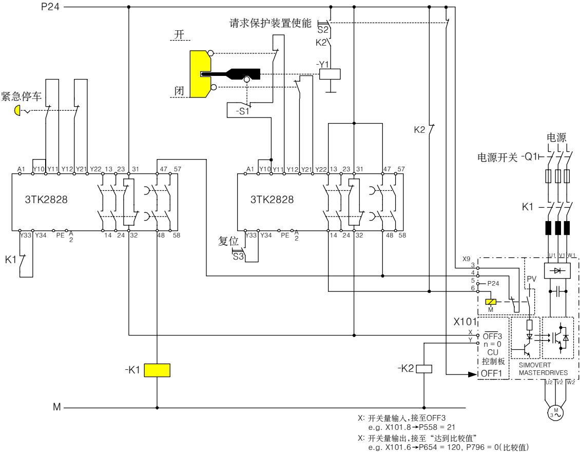
图 7-4 用接触器安全组合去监控按 EN 954-1 的安全级别 3，可移动保护装置的“安全停车”功能的实际应用图
