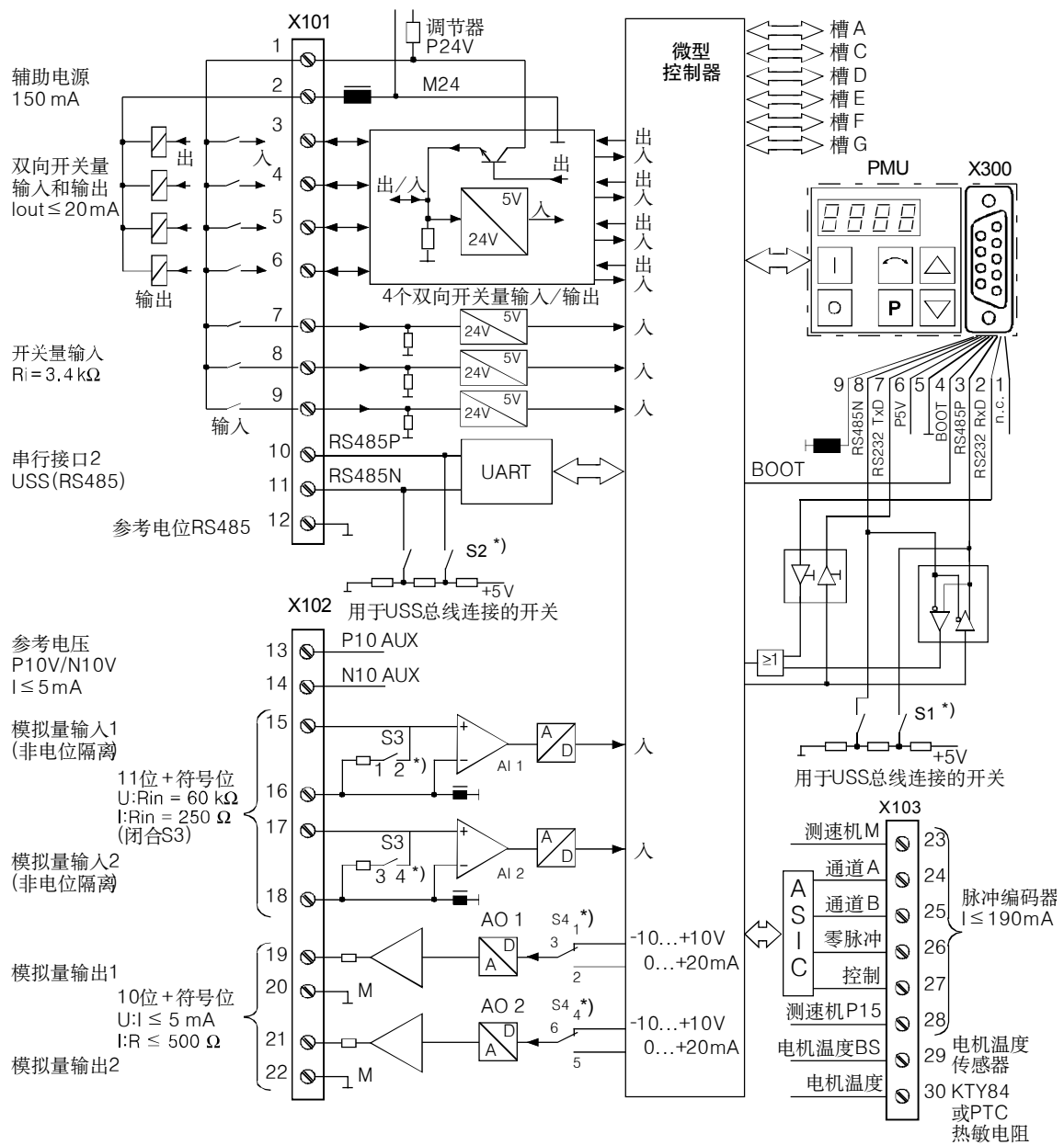
图 7-6 标准接线的简图
