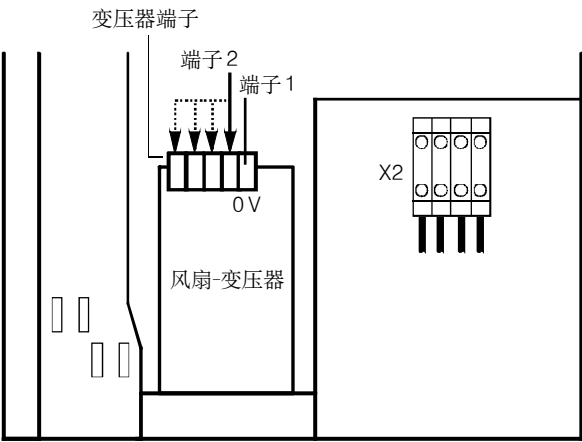
图 7-3 变压器位置(仅用于规格 D 的变频器)
