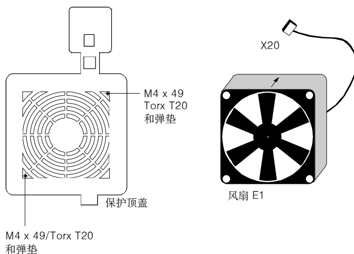
图 11-1 壳体尺寸 A~C 的顶盖和风扇
