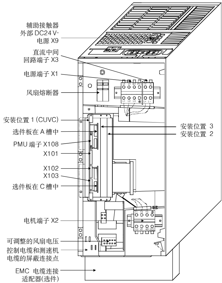
图 7-2 规格 D 的接线简图
