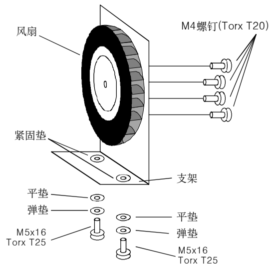
图 11-2 壳体尺寸 D 的带支架的风扇
