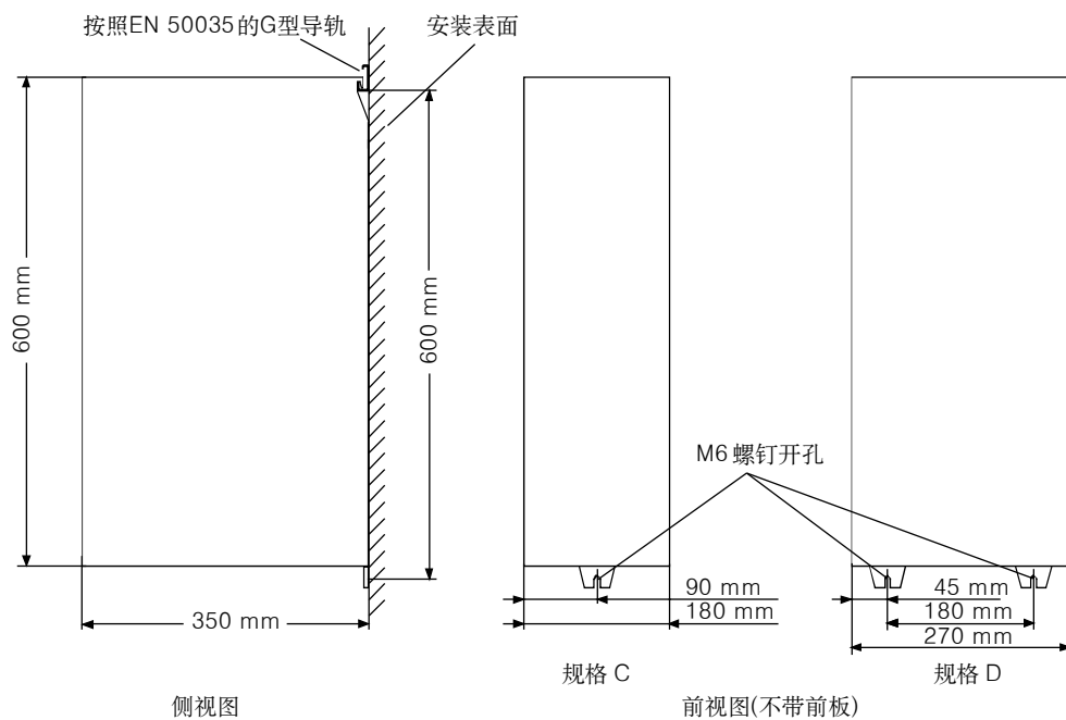
图 5-3 规格 C, D 安装尺寸图
