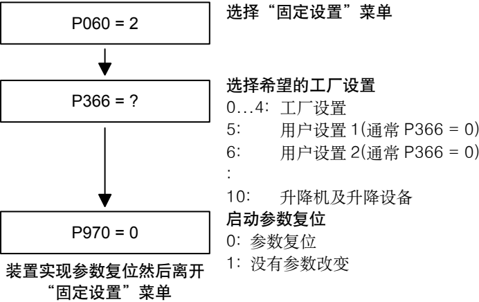
图 9-3 用用户的设定进行参数设置的顺序
