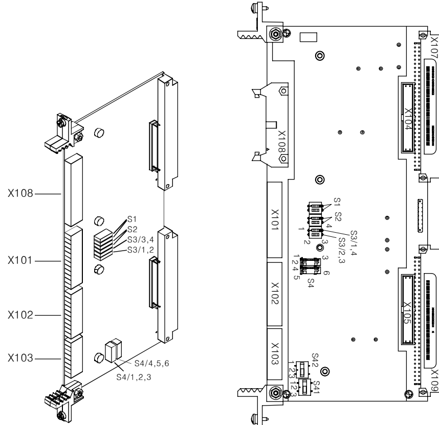
图 7-5 CUVC 板外观
