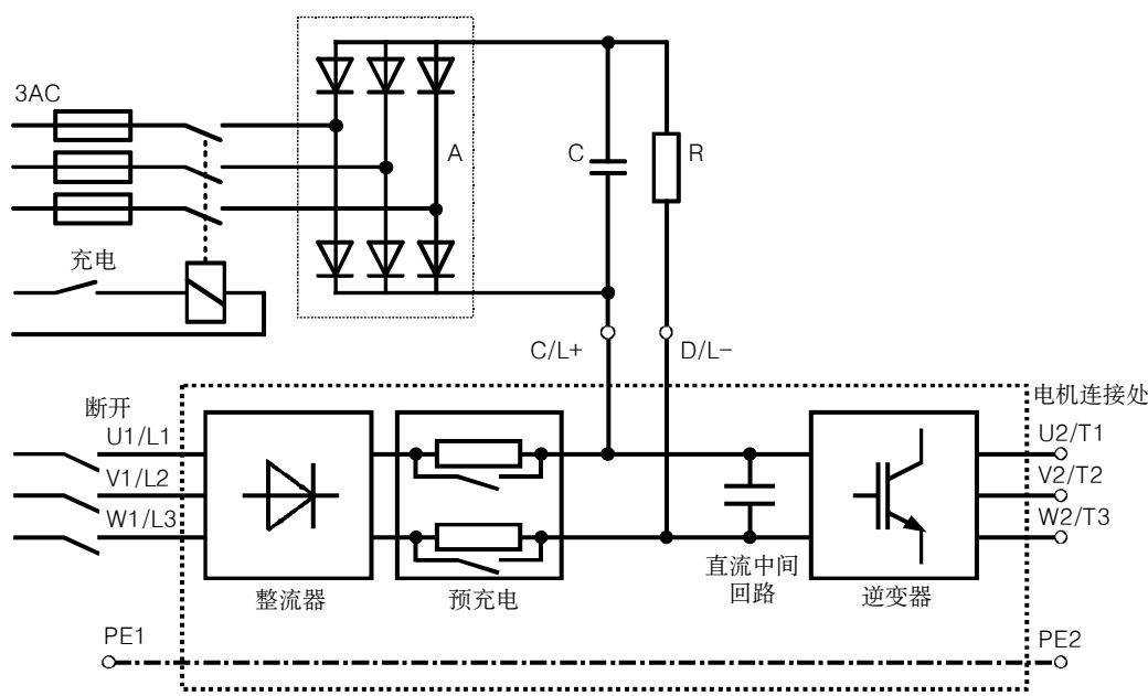
图 12-1 充电电路图
