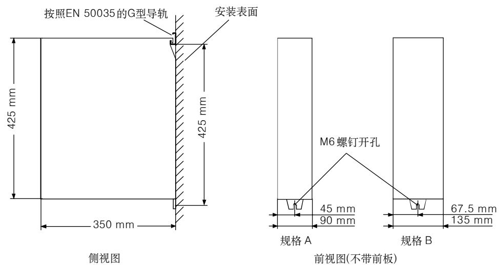
图 5-2 规格 A, B 安装尺寸图
