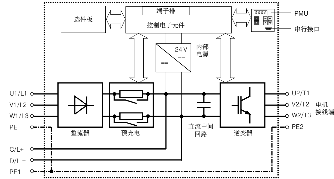
图 2-1 变频器的原理框图
