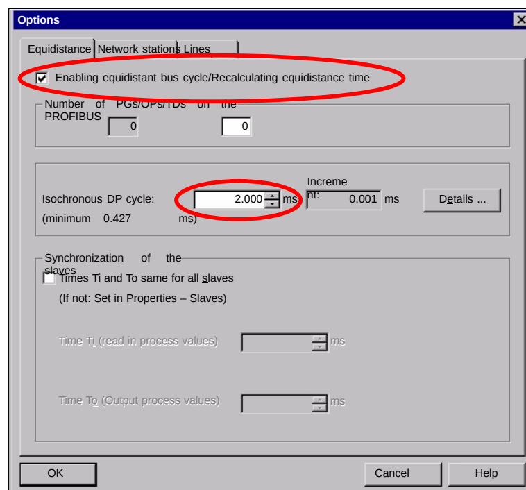
Fig. 3-9 Dialog: Options
