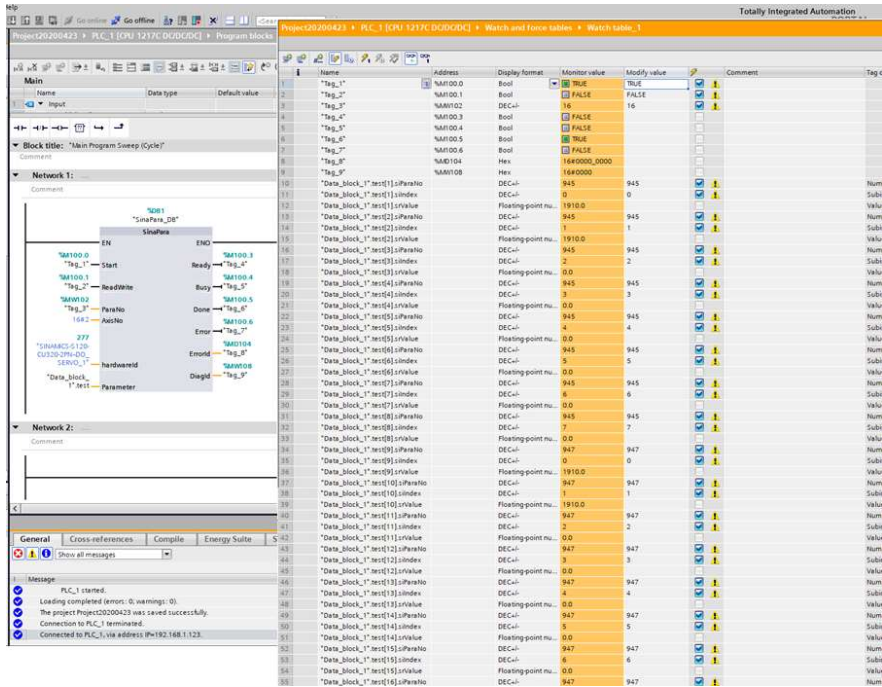
图 3-1 读取参数 r0945 和 r0947
