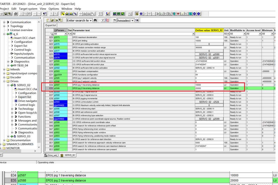
图 5-3 从 Starter 中查看参数修改
