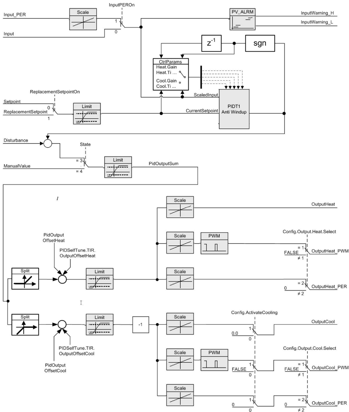
图 10-6 PID_Temp_Operation_Block_Diagram
