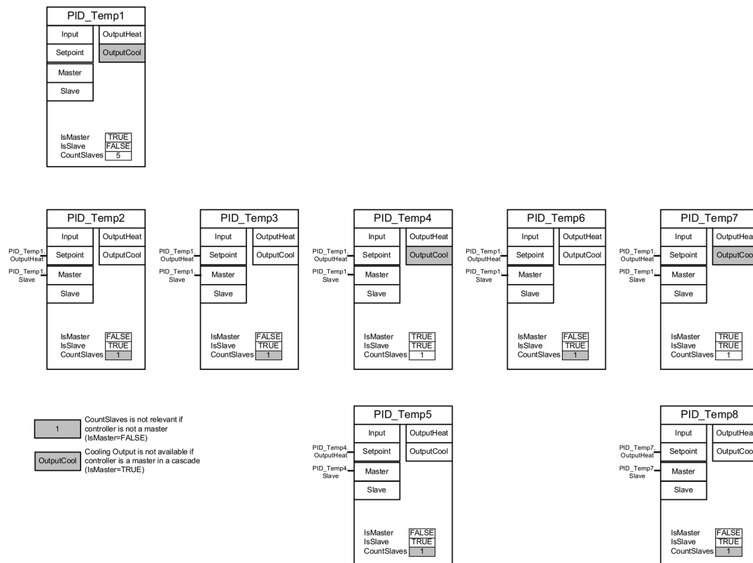
图 10-8 PID_Temp_Cascading_communication_connection
