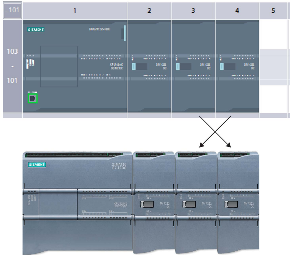
图 6-3 插槽 3 和 4 中的模块交换后，设备组态与实际安装的比较
