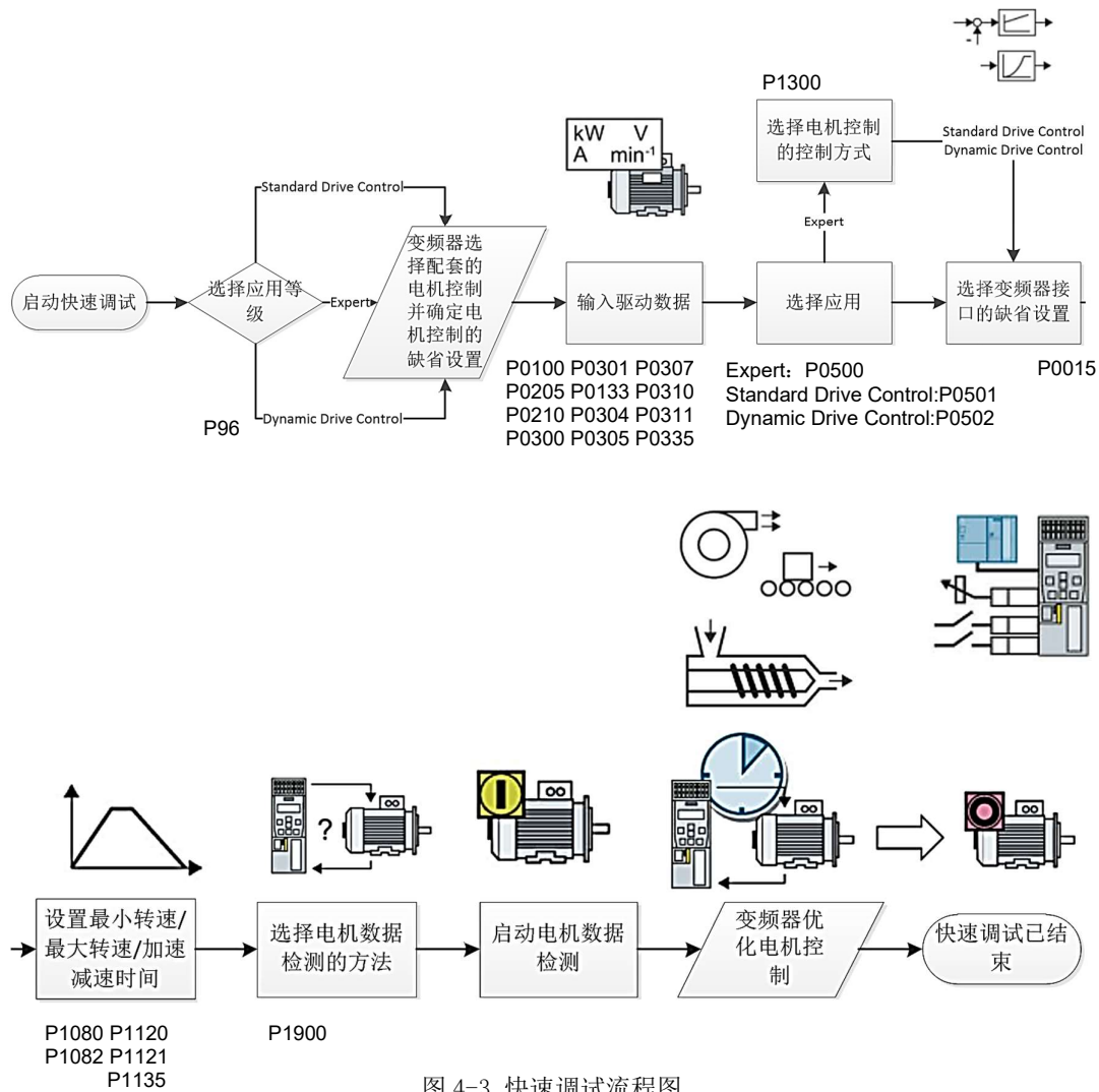
图 4-3 快速调试流程图
