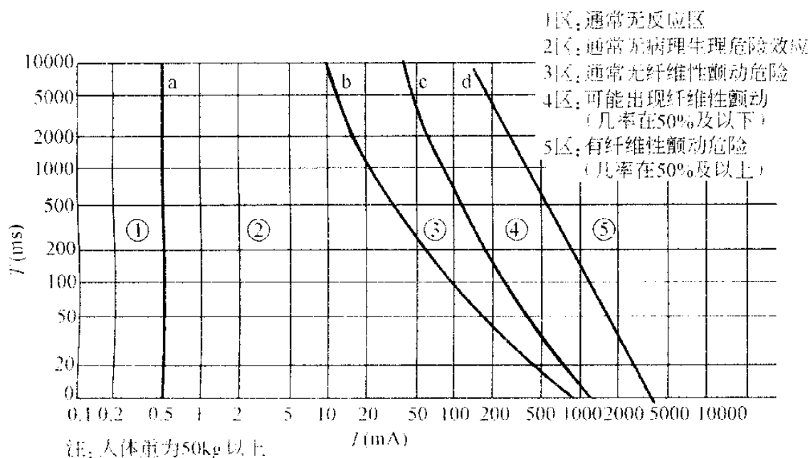
图 1 交流电流(50/60Hz)对成年人的效应区域
