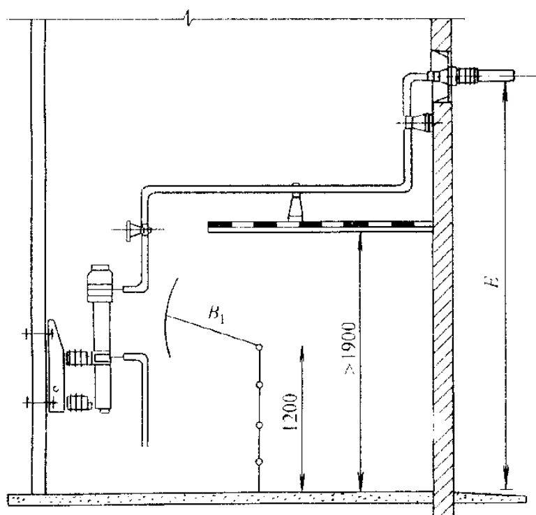
图 E.2 室内 B_1 、 E 值校验
