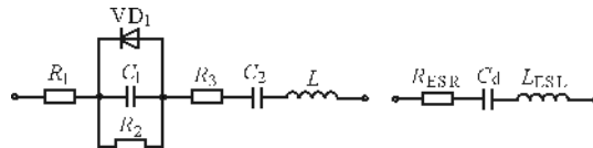
图 1 电解电容器实际等效电路和计算等效电路
