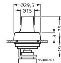
双按钮开关 凸型
