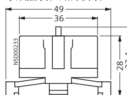
单触点块，底部安装
