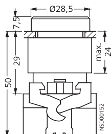
平形按钮或带灯按钮 带单触点块
