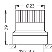
电位计旋钮
