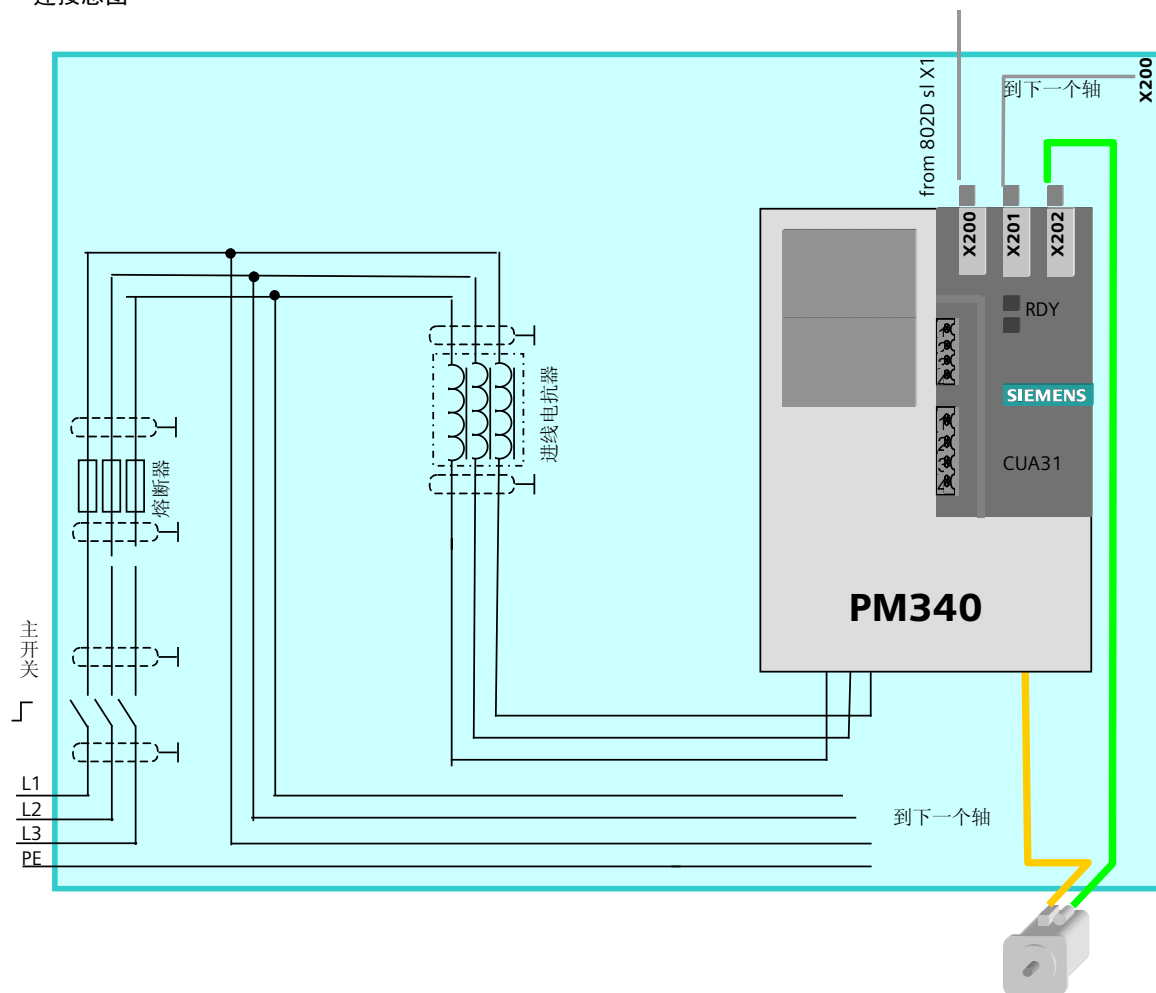
连接总图
