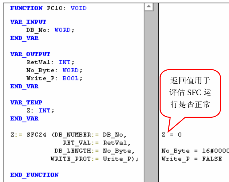
图 4-5: 调用带有返回值的 SFC
