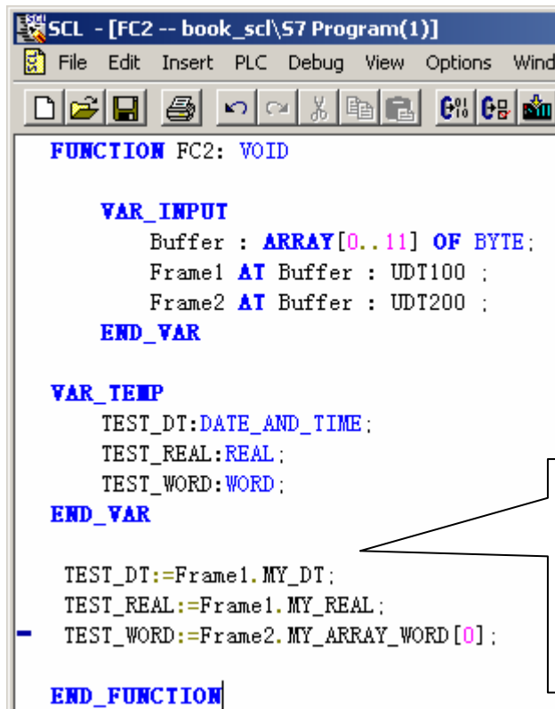
图 4-9: AT 指令特点说明 (b)
