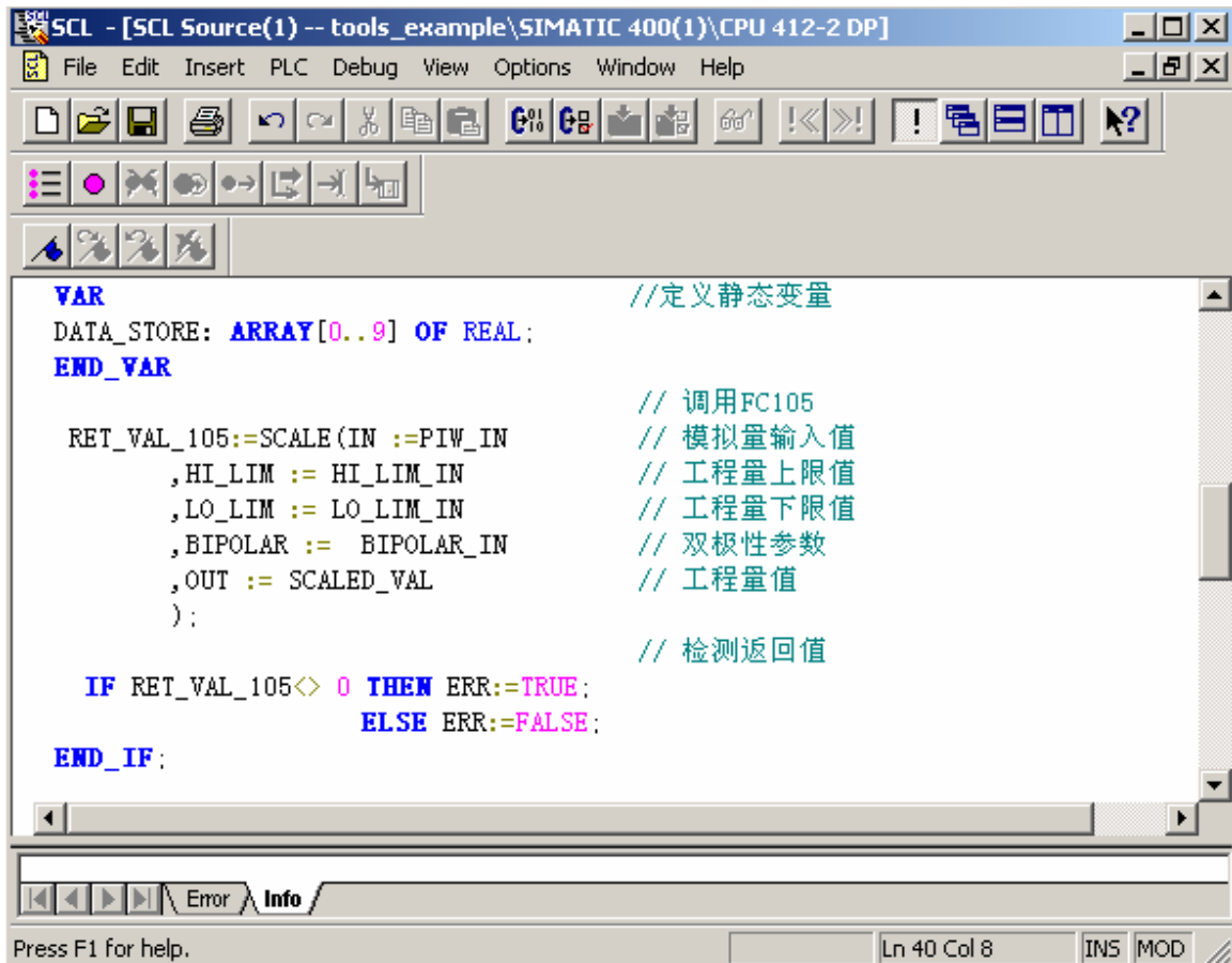
图 3-11: FC105 调用
