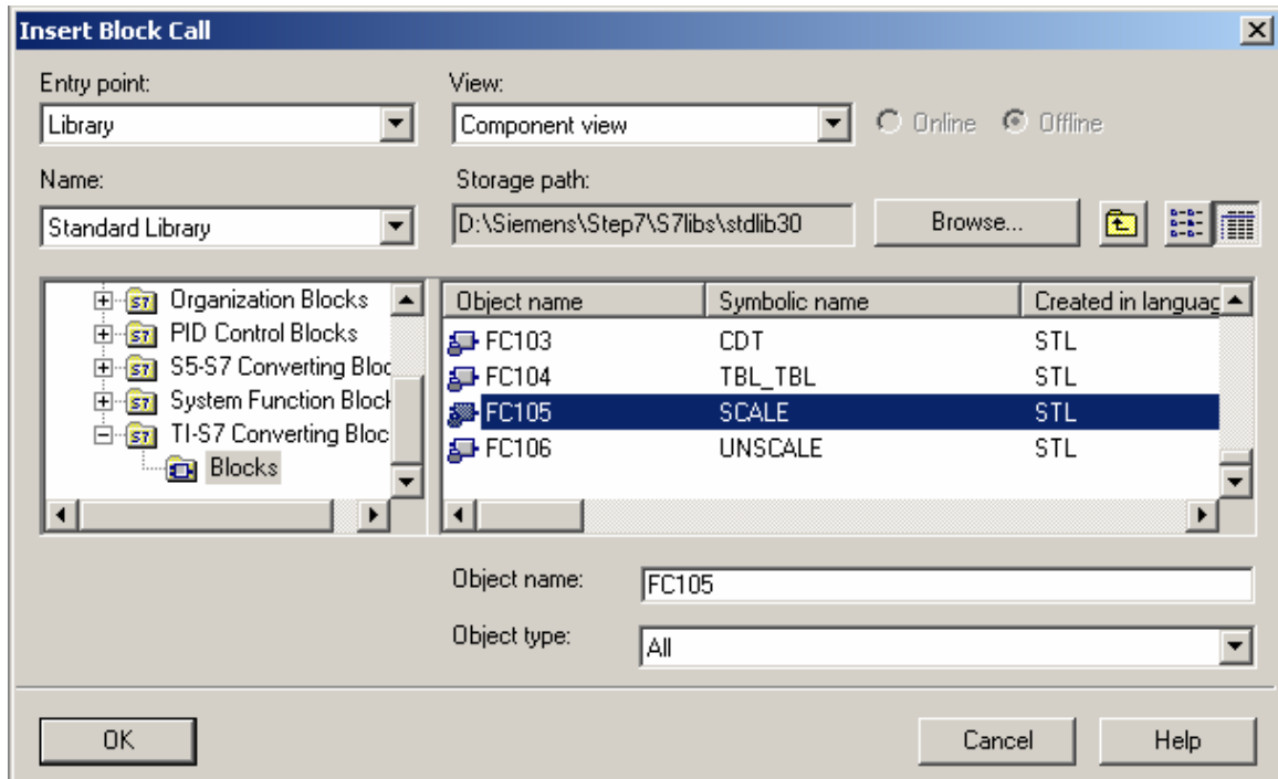
图 3-7: 调用 FC105
