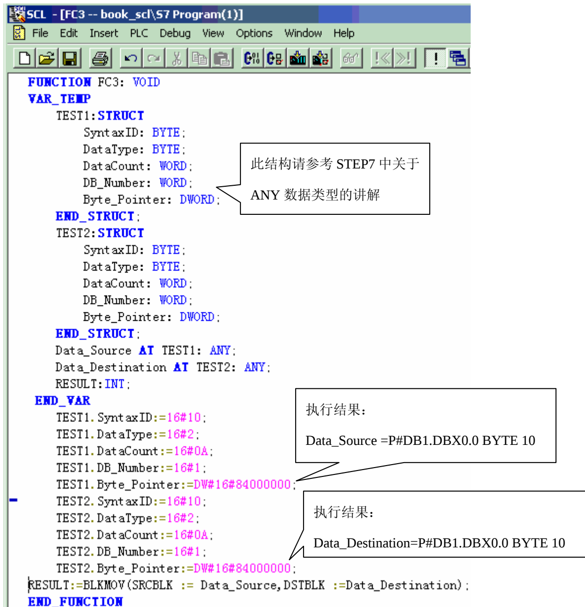
图 4-11: AT 指令应用 (b)
