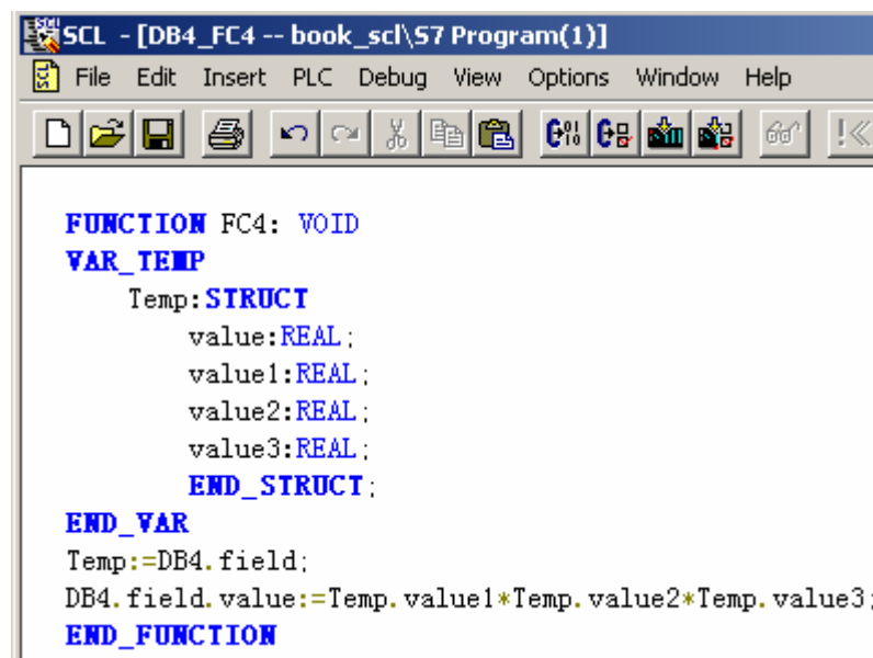
图 4-15：优化数据块访问
