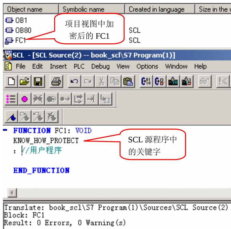
图 4-1: S7-SCL 源程序加密
