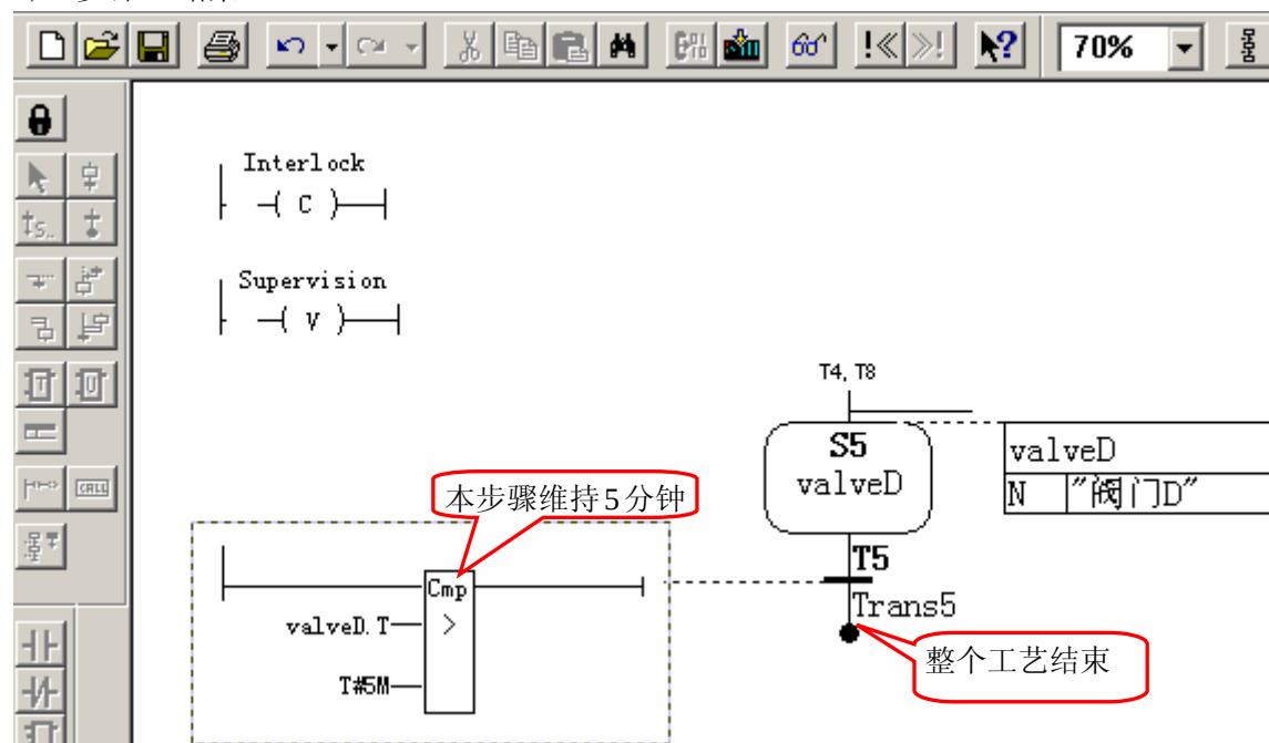
图 6-10: 流程结束
