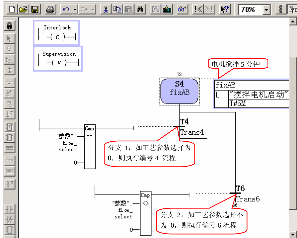
图 6-9: 流程分支
