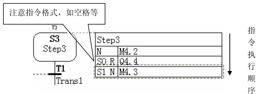
图 4-6：指令执行顺序
