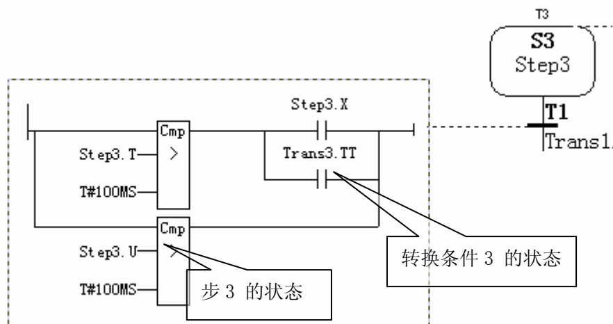
图 4-7：S7-GRAPH 特有地址的引用格式
