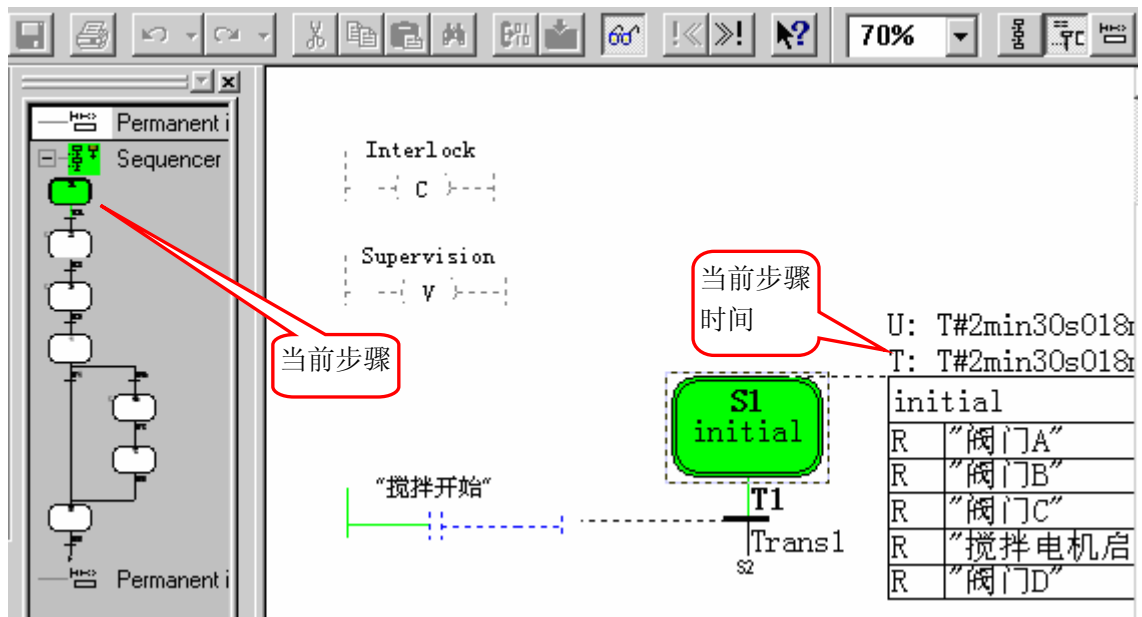
图 6-13: 监控 FB2
