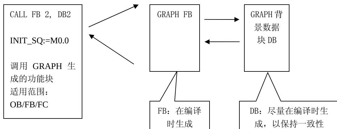
图 3-1: S7 程序构成
