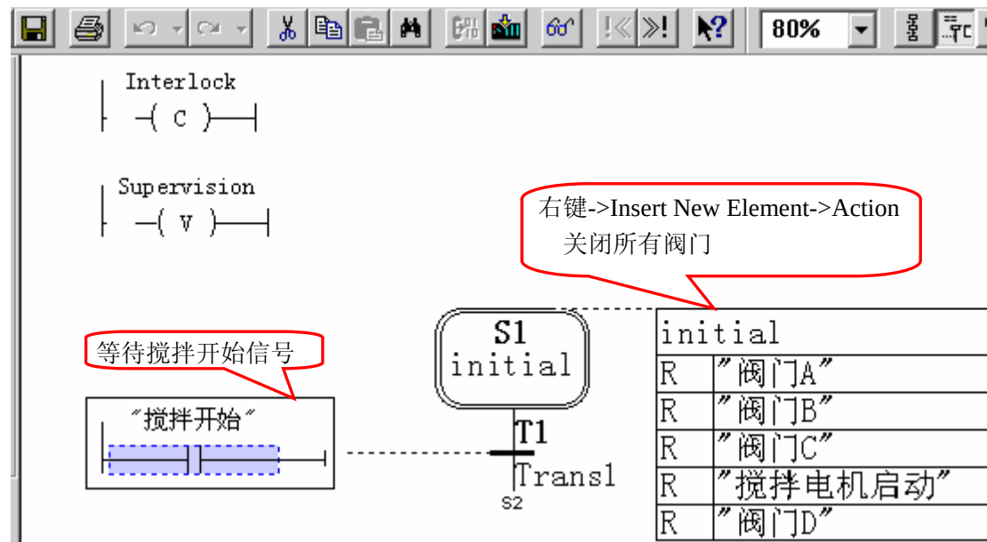
图 6-7：初始化
