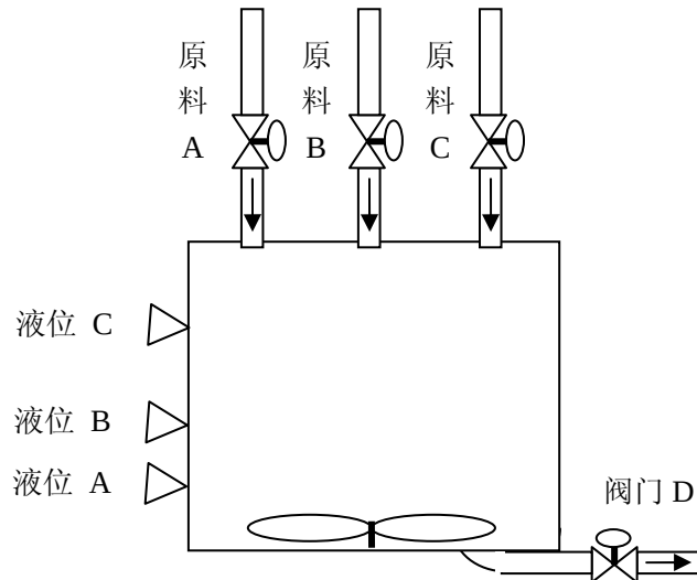
图 6-1：原料配比示意图
