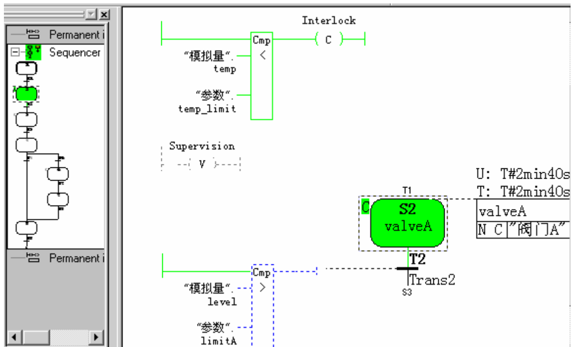
图 6-14: 测试 FB2
