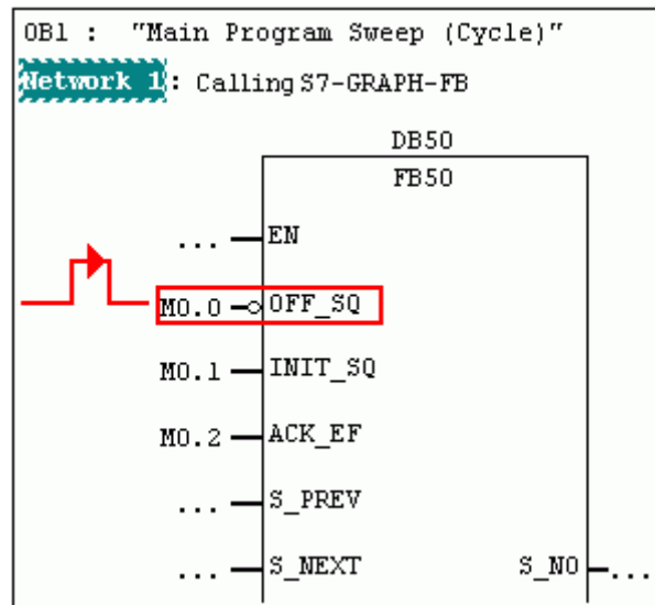
图 7-10: 关闭顺控器
