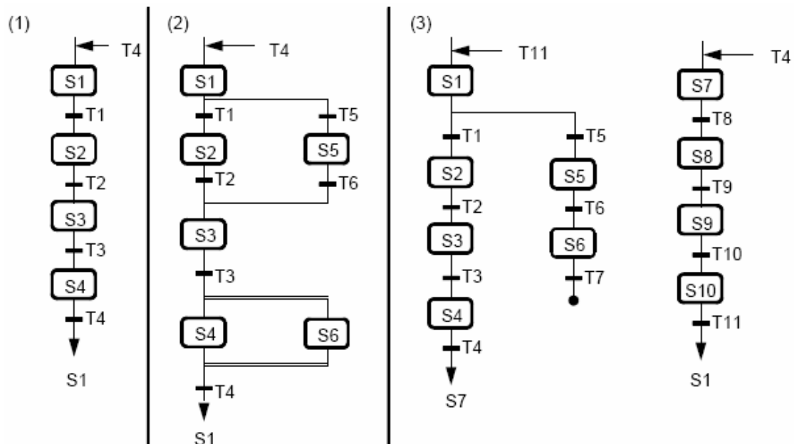
图4-1：顺控器结构
