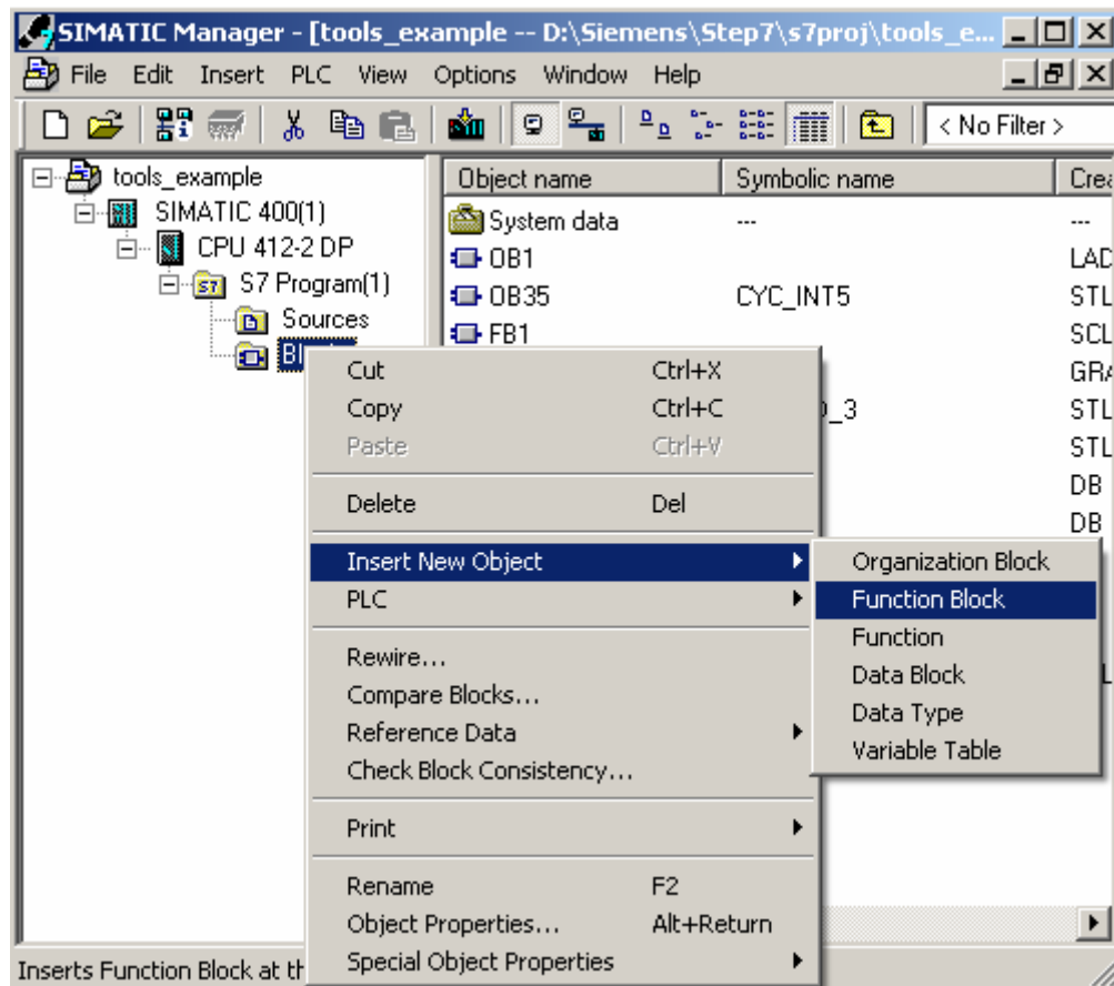
图 6-3：添加功能块
