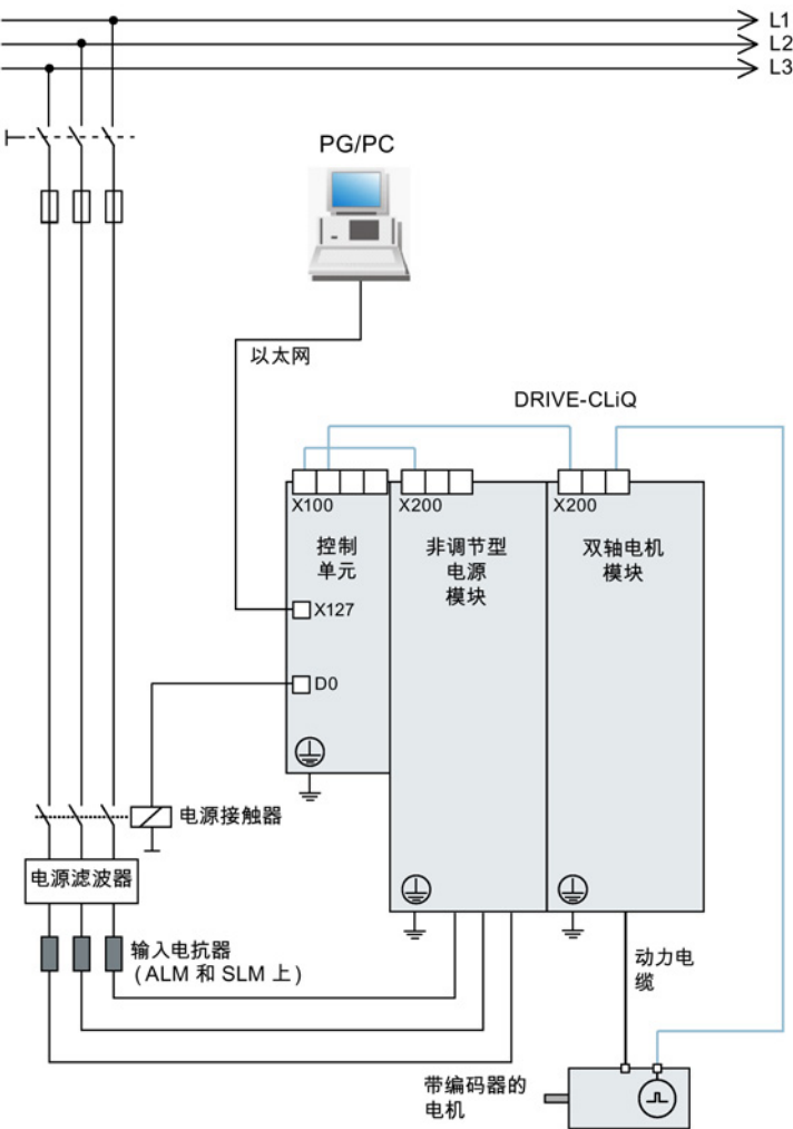
图 4-2 布线原理图
