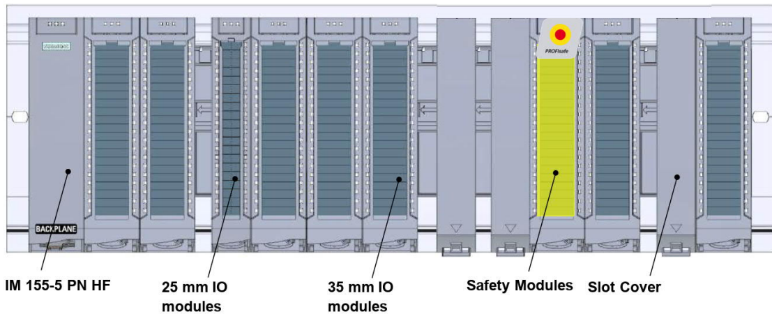
图 2 安装有源背板总线的 ET200MP 正面示意图
