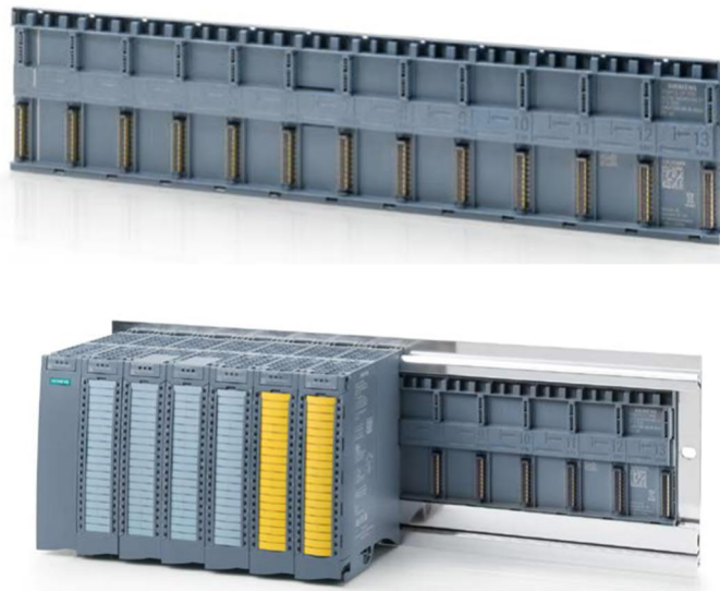
图 1 ET200MP 有源背板总线（12 槽）
